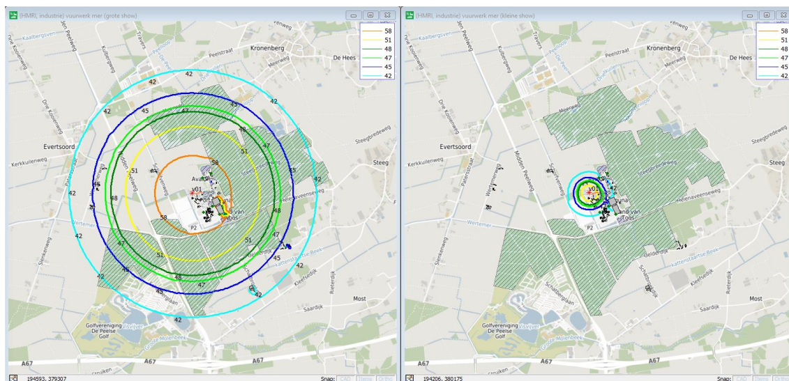
Afbeelding 1. Modelling geluid vuurwerk tijdens grote shows (links) en kleine shows (rechts).
