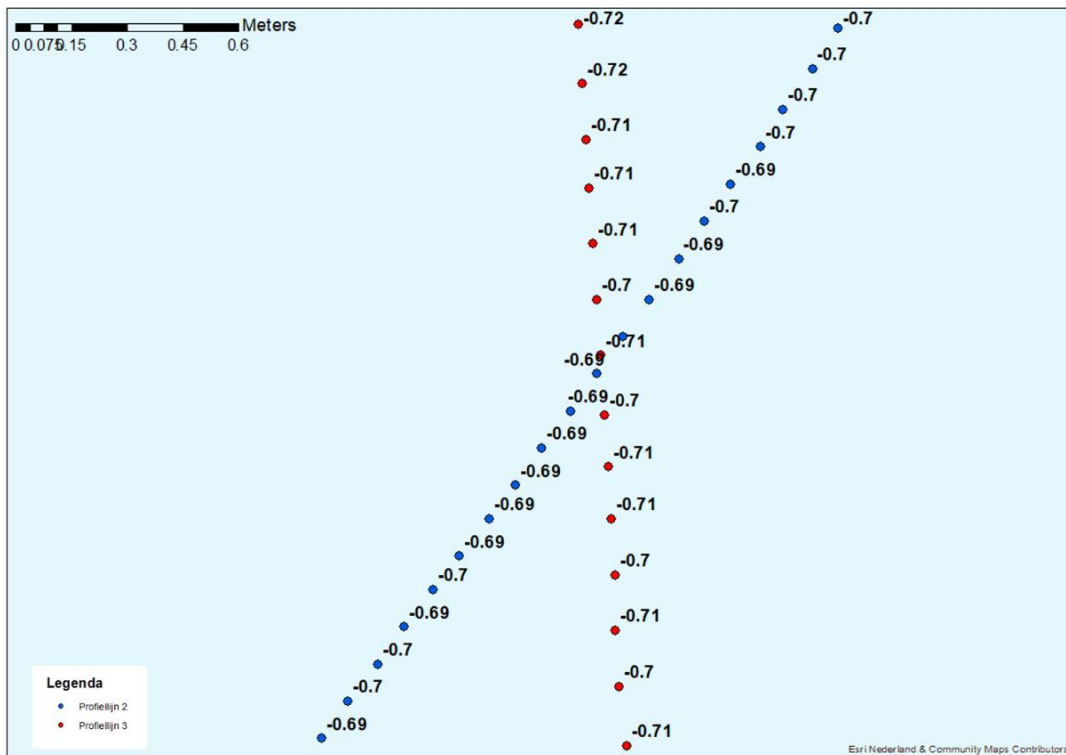
Figuur 9-44 Detailkaart controlepunt tussen profiellijn 2 en profiellijn 3 voor de hoogte/diepte raaien 2018, hoogtemetingen zijn weergegeven in m NAP.
