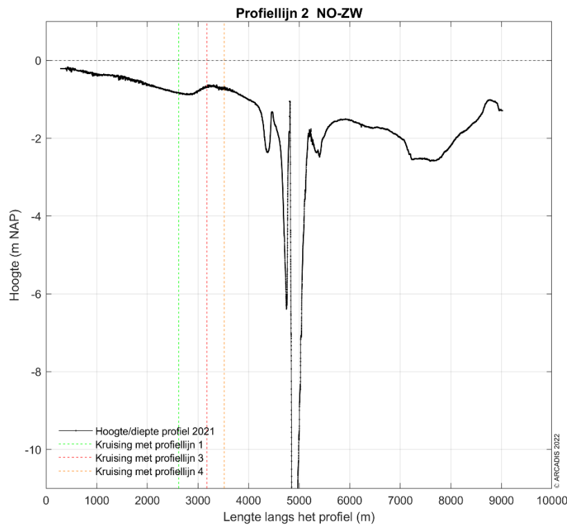
Figuur 9-64 Dwarsdoorsnede langs profiellijn 2 van noordoost naar zuidwest in 2021.
