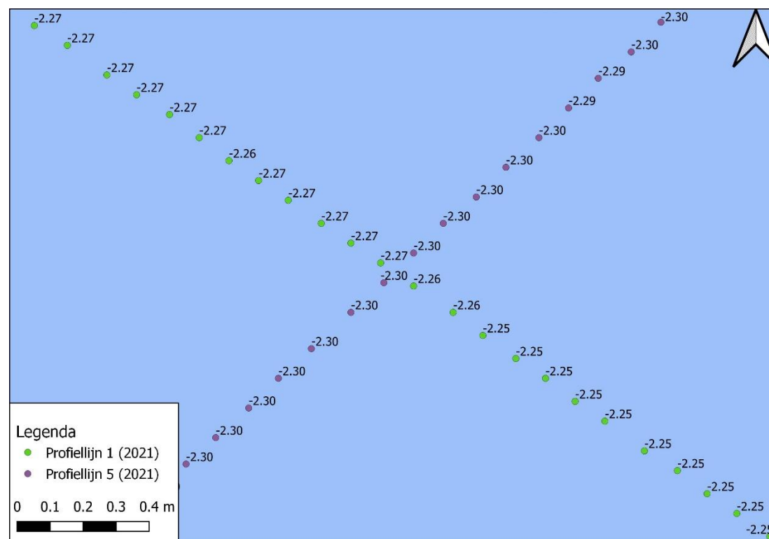
Figuur 9-71 Detailkaart controlepunt tussen profiellijn 1 en profiellijn 5 voor de hoogte/diepte raaien 2021, hoogtemetingen zijn weergegeven in m NAP.
