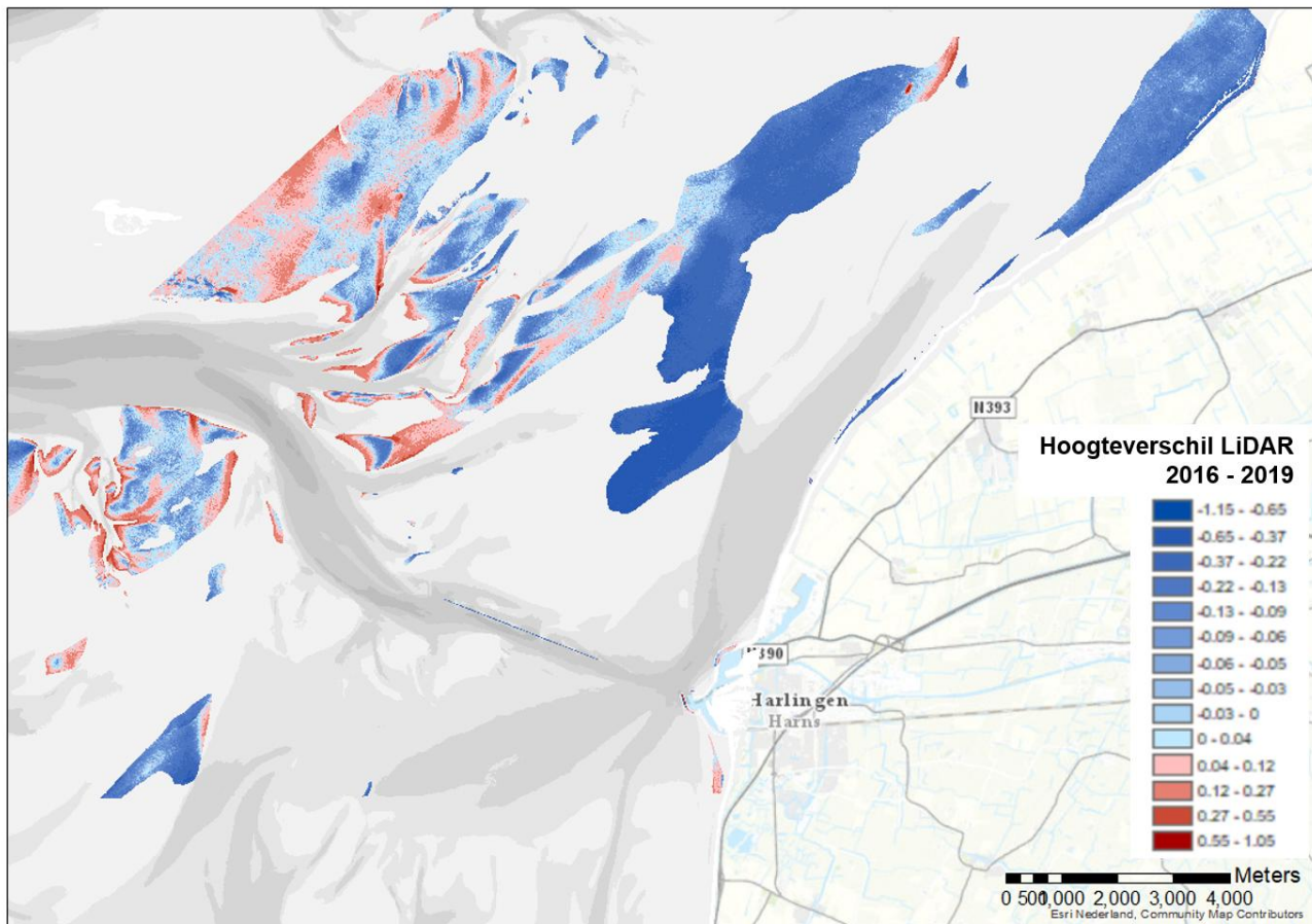
Figuur 9-26 Kaart met de hoogteverschillen in meters tussen de LiDAR hoogtemetingen van 2016 en 2019. De blauwe gebieden liggen lager in 2019 en de rode gebieden hoger.
