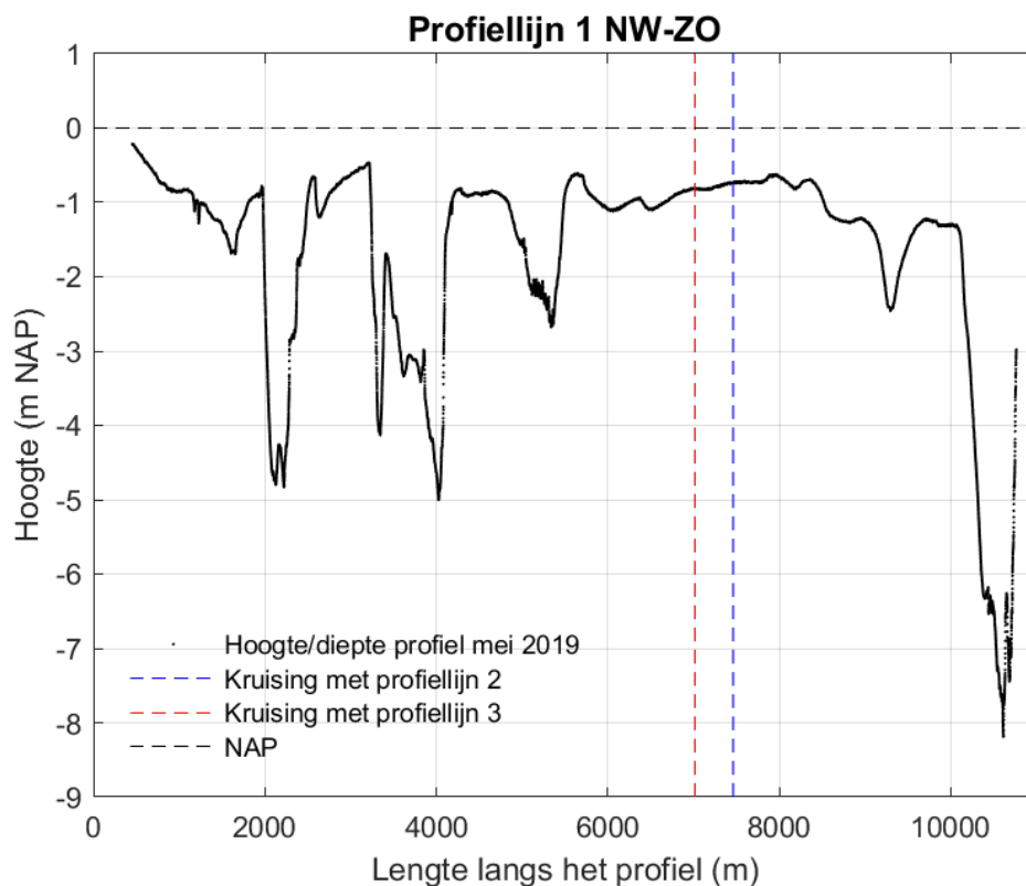
Figuur 9-51 Dwarsdoorsnede langs profiellijn 1 van noordwest naar zuidoost in mei 2019.
