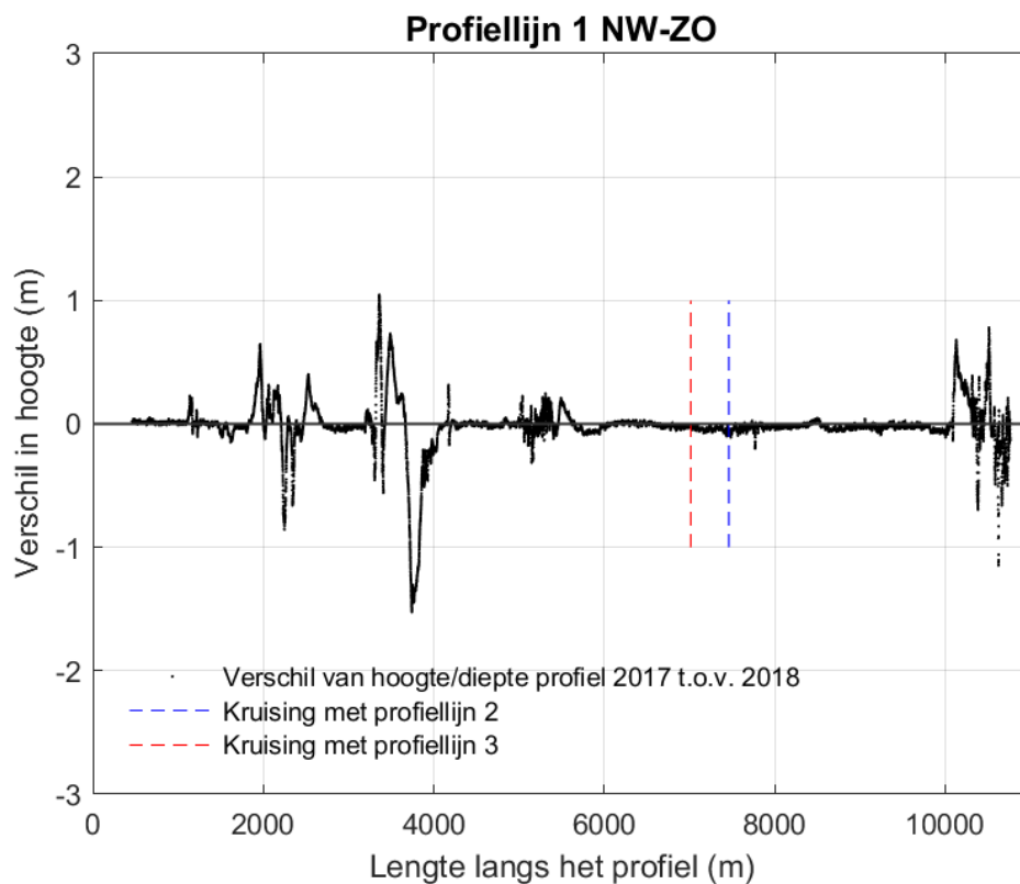
Figuur 9-129 Verschilplot langs profiellijn 1 van noordwest naar zuidoost voor de hoogte/diepte raai meetgegevens van 2017 en 2018. Een negatieve waarde betekent dat de hoogte/diepteraai van 2018 lager ligt dan de hoogte/diepteraai van 2017.
