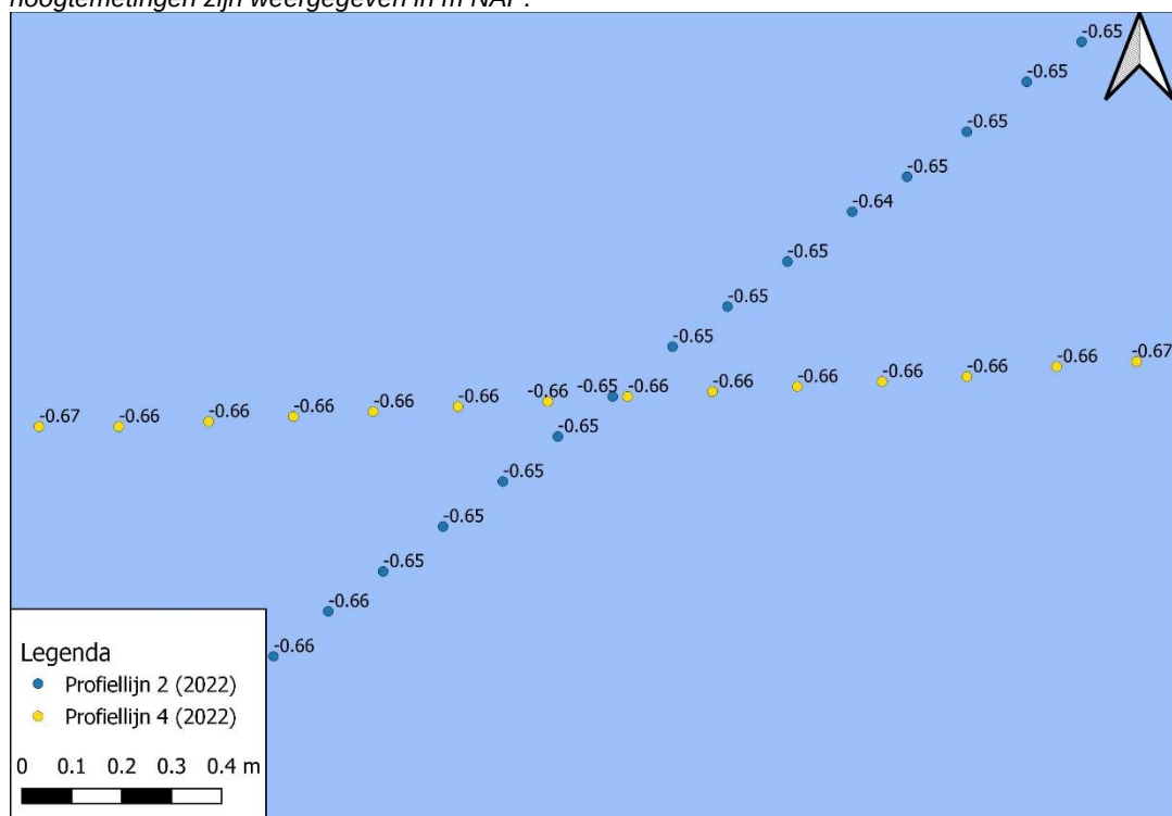
Figuur 9-87 Detailkaart controlepunt tussen profiellijn 2 en profiellijn 4 voor de hoogte/diepte raaien mei 2022, hoogtemetingen zijn weergegeven in m NAP.
