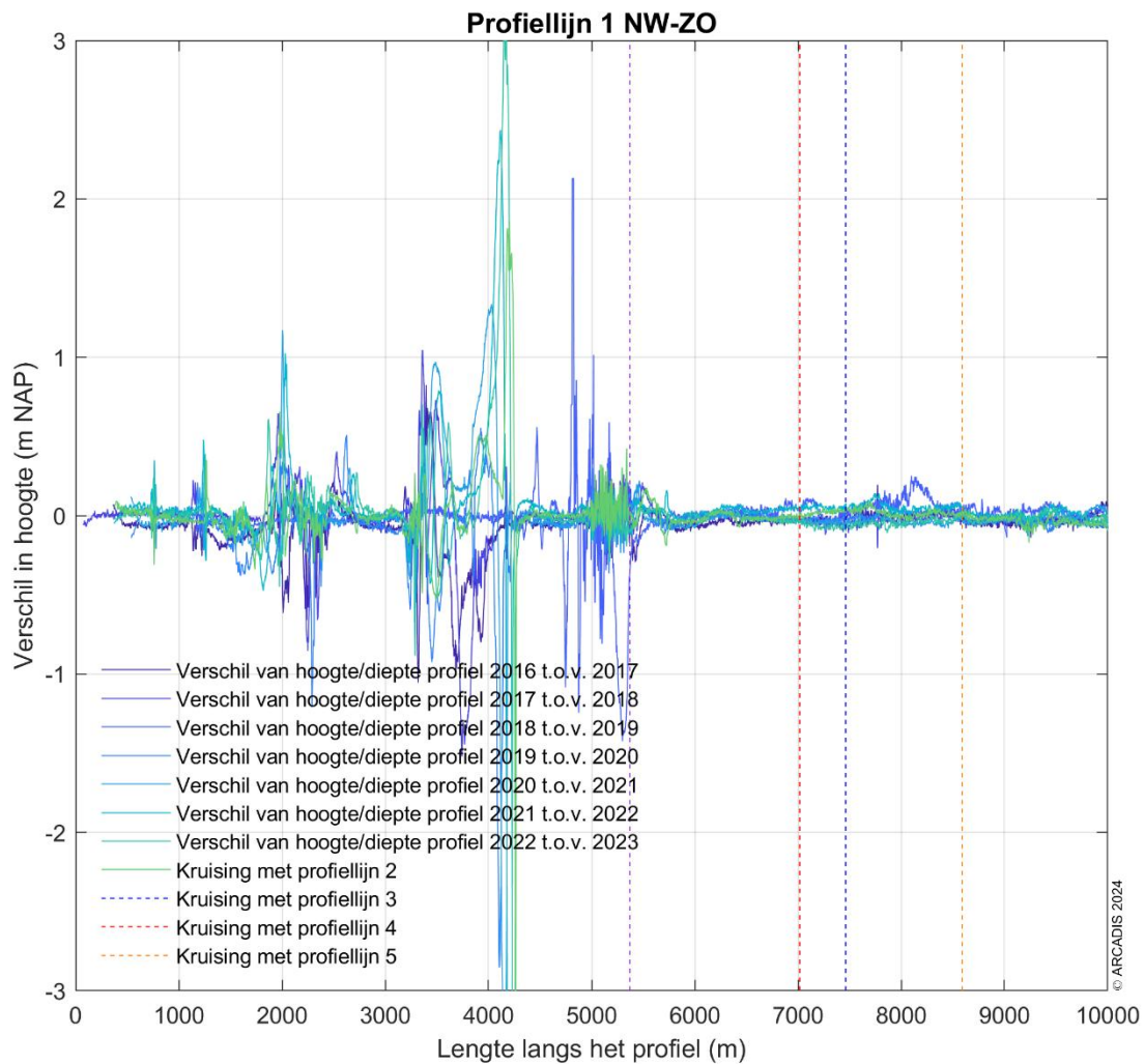
Figuur 4-3 Verschilplot langs profiellijn 1 van noordwest naar zuidoost voor de hoogte/diepte raai meetgegevens tussen 2016-2024. Een positieve waarde betekent dat de hoogte/diepteraai van het opvolgende jaar hoger ligt dan de hoogte/diepteraai van het eerdere jaar.
