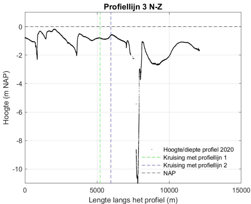
Figuur 9-59 Dwarsdoorsnede langs profiellijn 3 van noord naar zuid in 2020.
