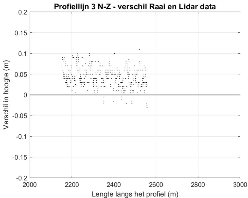
Figuur 9-14 Ingezoomde verschilplot langs profiellijn 3 van noord naar zuid voor de hoogte/diepte raai meetgegevens van 2016 en de LiDAR-data van 2016. Een positieve waarde betekent dat de LiDAR lager ligt dan de hoogte/diepteraai.
