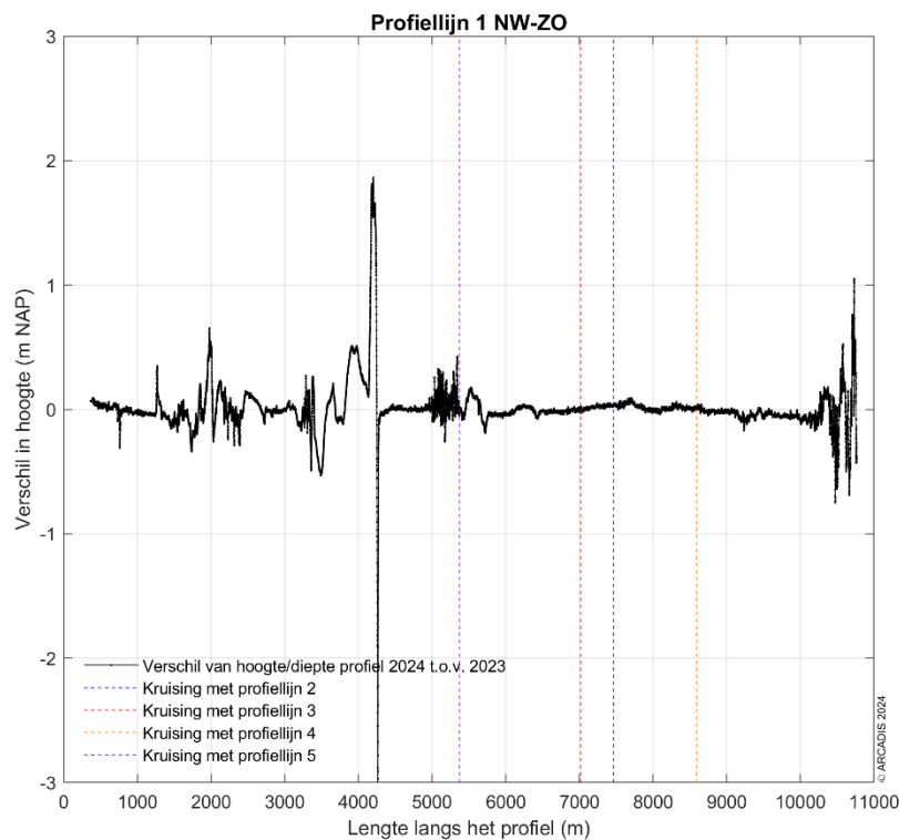
Figuur 3-5 Verschilplot langs profiellijn 1 van noordwest naar zuidoost voor de hoogte/diepte raai meetgegevens van 2023 en 2024. Een positieve waarde betekent dat de hoogte/diepteraai van 2024 hoger ligt dan de hoogte/diepteraai van 2023.
