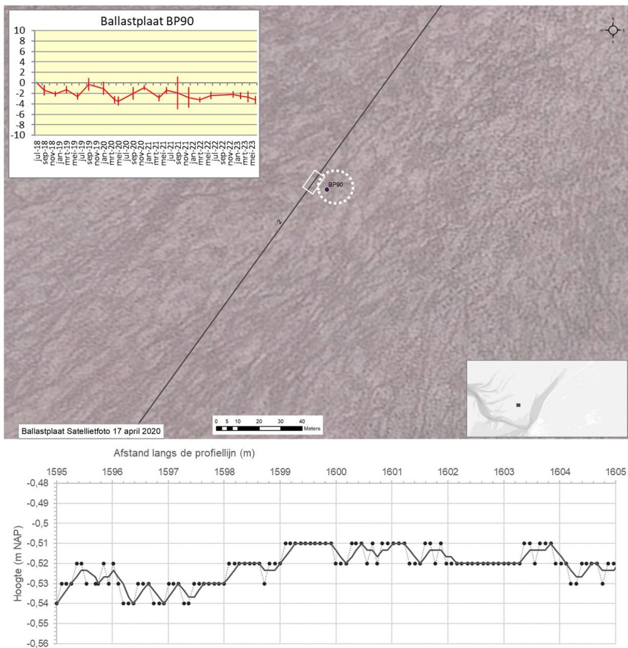
Figuur 9-208 Luchtfoto (17 april 2020) met de locatie van spijkermeting BP90 en raai 2, met daarbij linksboven de grafiek met de resultaten van de spijkermetingen bij BP90 en onder de dwarsdoorsnede van raai 2 van de raaimeting uit 2023.
