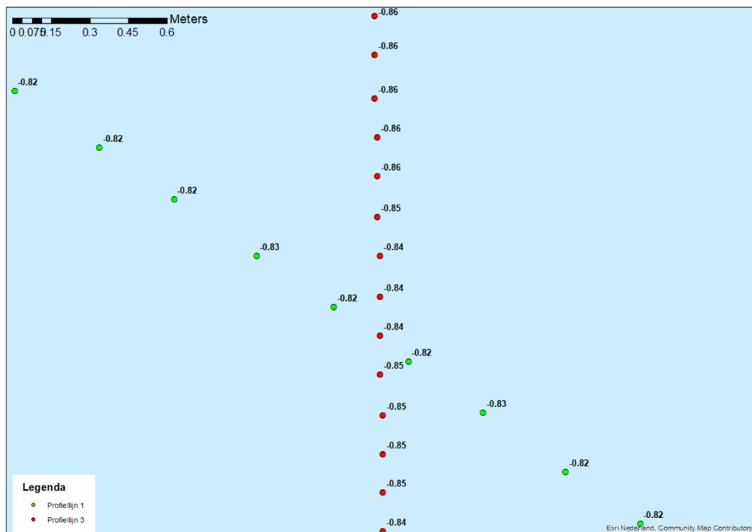
Figuur 9-49 Detailkaart controlepunt tussen profiellijn 1 en profiellijn 3 voor de hoogte/diepte raaien januari 2019, hoogtemetingen zijn weergegeven in m NAP.
