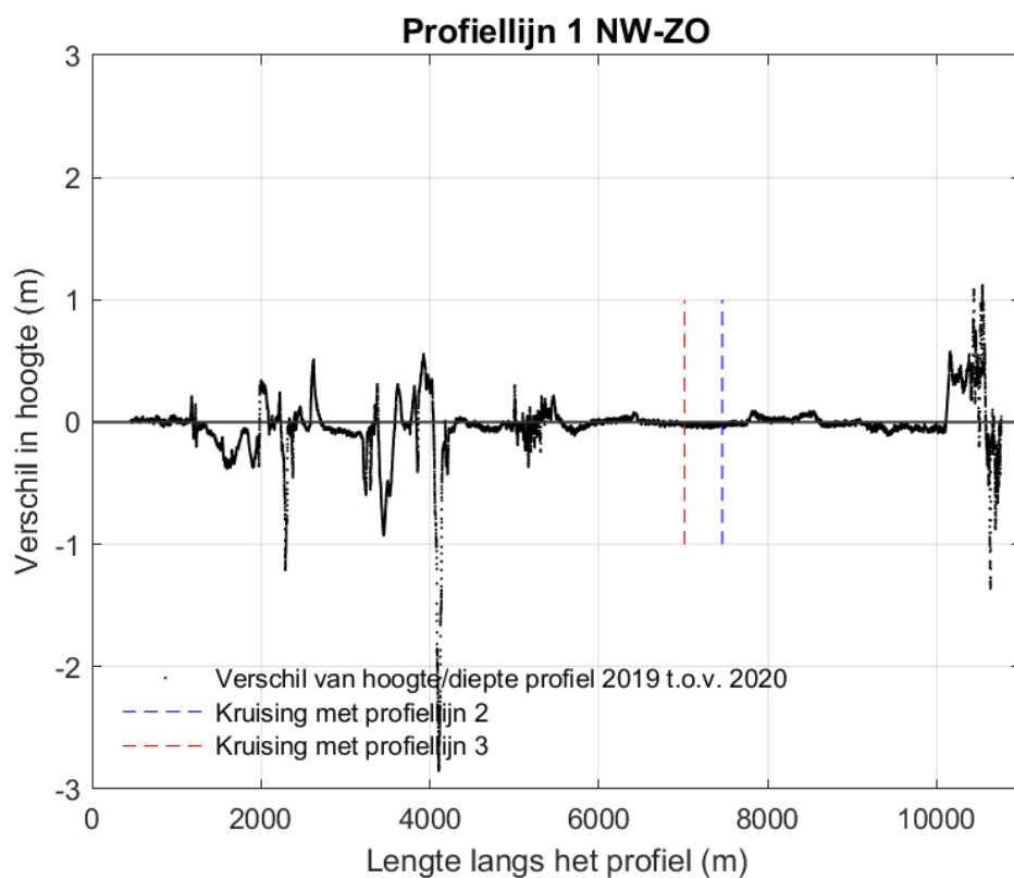
Figuur 9-156 Verschilplot langs profiel lijn 1 van noordwest naar zuidoost voor de hoogte/diepte raai meetgegevens van 2019 en 2020. Een positieve waarde betekent dat de hoogte/diepteraai van 2020 hoger ligt dan de hoogte/diepteraai van 2019.
