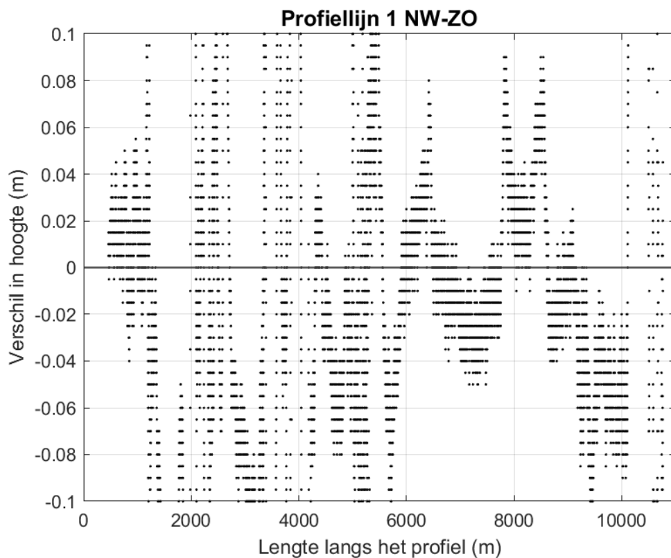
Figuur 9-157 Ingezoomde verschilplot langs profiel lijn 1 van noordwest naar zuidoost voor de hoogte/diepte raai meetgegevens van 2019 en 2020. Een positieve waarde betekent dat de hoogte/diepteraai van 2020 hoger ligt dan de hoogte/diepteraai van 2019.
