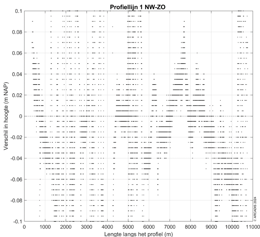
Figuur 3-5 Verschilplot langs profiellijn 1 van noordwest naar zuidoost voor de hoogte/diepte raai meetgegevens van 2023 en 2024. Een positieve waarde betekent dat de hoogte/diepteraai van 2024 hoger ligt dan de hoogte/diepteraai van 2023.
