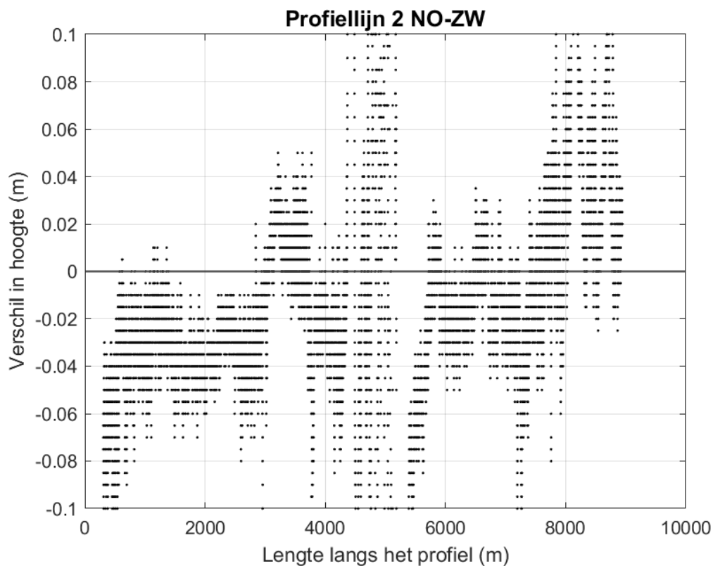
Figuur 9-133 Ingezoomde verschilplot langs profiellijn 2 van noordoost naar zuidwest voor de hoogte/diepte raai meetgegevens van 2017 en 2018. Een negatieve waarde betekent dat de hoogte/diepteraai van 2018 lager ligt dan de hoogte/diepteraai van 2017.
