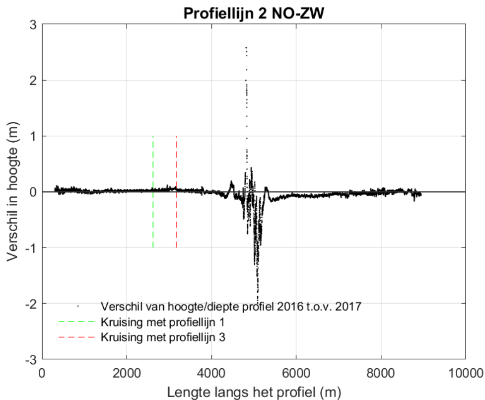
Figuur 9-123 Verschilplot langs profiellijn 2 van noordoost naar zuidwest voor de hoogte/diepte raai meetgegevens van 2016 en 2017. Een positieve waarde betekent dat de hoogte/diepteraai van 2017 hoger ligt dan de hoogte/diepteraai van 2016.
