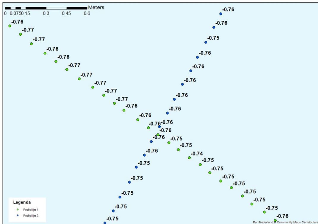
Figuur 9-42 Detailkaart controlepunt tussen profiellijn 1 en profiellijn 2 voor de hoogte/diepte raaien 2018, hoogtemetingen zijn weergegeven in m NAP.
