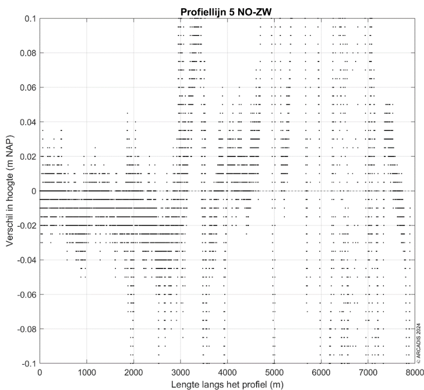
Figuur 3-18: Ingezoomde verschilplot langs profiellijn 5 van noordoost naar zuidwest voor de hoogte/diepte raai meetgegevens van 2023 en 2024. Een positieve waarde betekent dat de hoogte/diepteraai van 2024 hoger ligt dan de hoogte/diepteraai van 2023.
