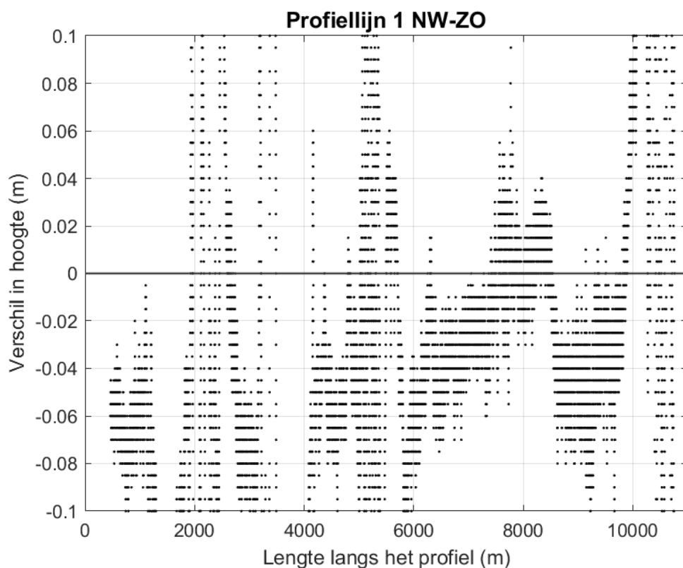
Figuur 9-121 Ingezoomde verschilplot langs profiellijn 1 van noordwest naar zuidoost voor de hoogte/diepte raai meetgegevens van 2016 en 2017. Een negatieve waarde betekent dat de hoogte/diepteraai van 2017 lager ligt dan de hoogte/diepteraai van 2016.
