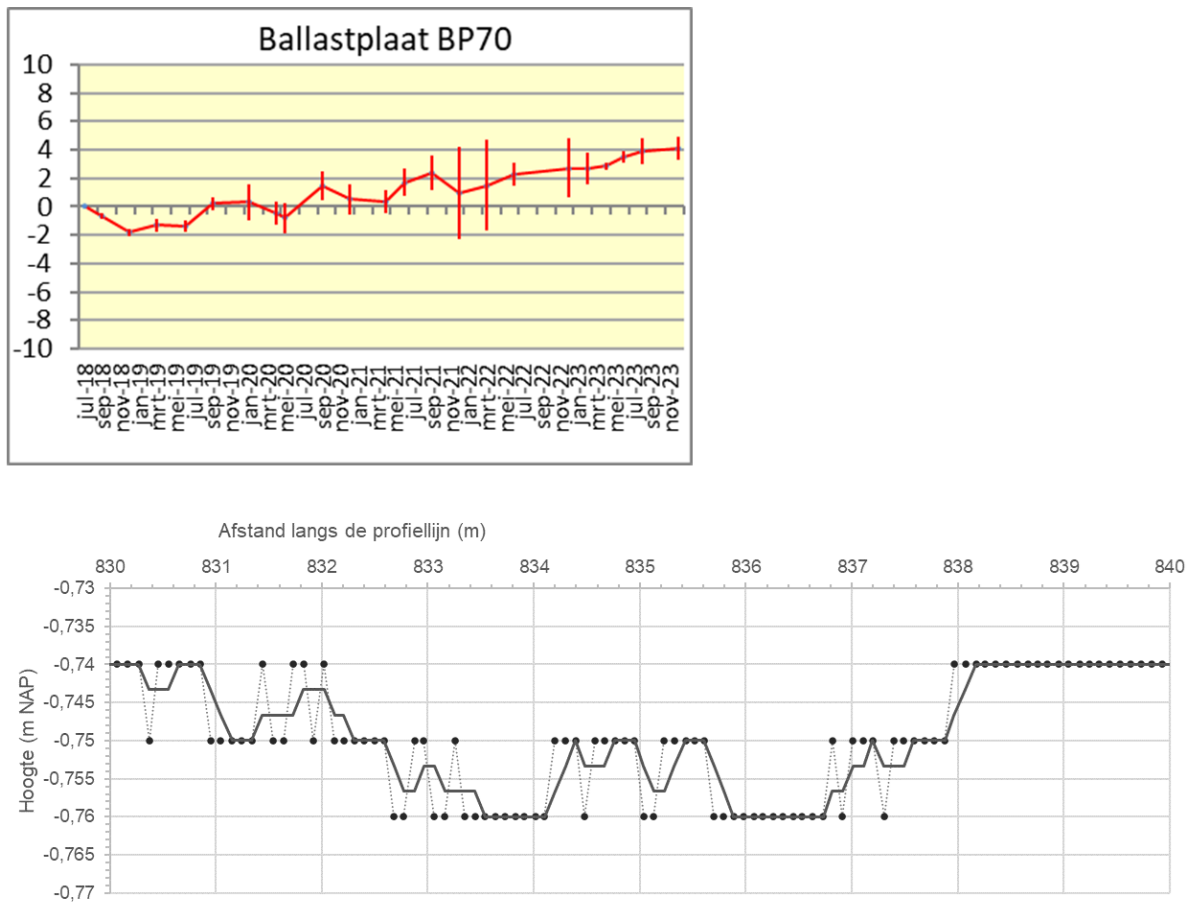
Figuur 9-210 Grafiek met de resultaten van de spijkermetingen bij BP70 en onder de dwarsdoorsnede van raai 2 ter plaatse van de spijkermeting van de raaimeting uit 2023.
