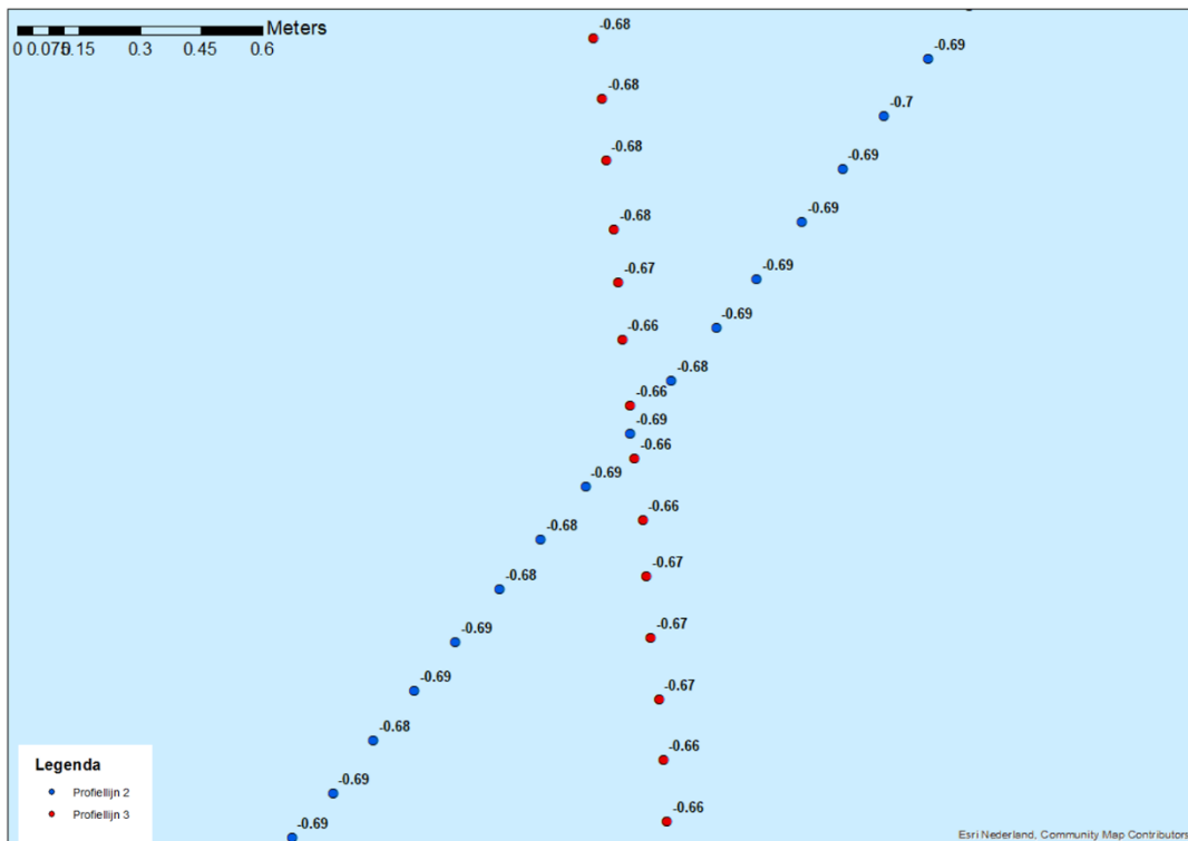
Figuur 9-56 Detailkaart controlepunt tussen profiellijn 2 en profiellijn 3 voor de hoogte/diepte raaien mei 2019, hoogtemetingen zijn weergegeven in m NAP.
