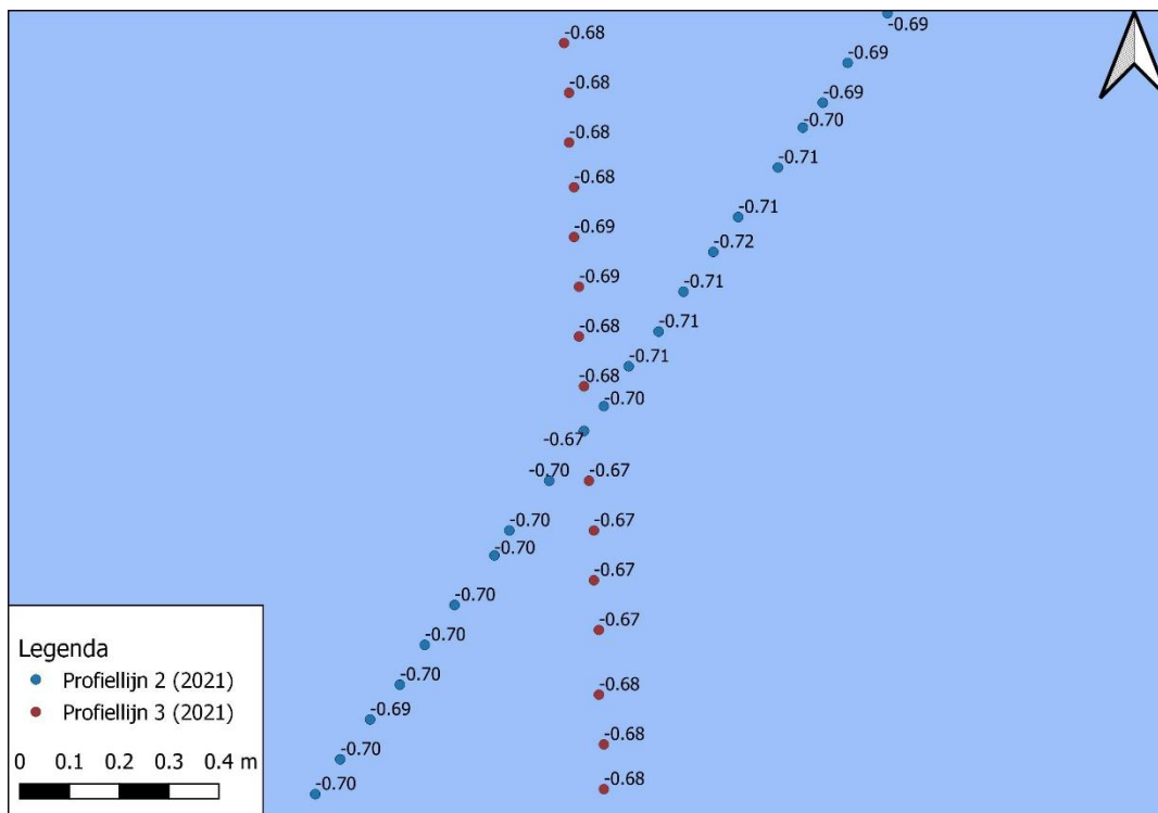
Figuur 9-72 Detailkaart controlepunt tussen profiellijn 2 en profiellijn 3 voor de hoogte/diepte raaien mei 2021, hoogtemetingen zijn weergegeven in m NAP.
