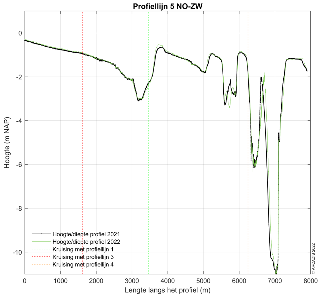
Figuur 9-185 Dwarsprofiel langs profiellijn 5 van noordoost naar zuidwest voor de hoogte/diepte raai meetgegevens van 2021 en 2022.
