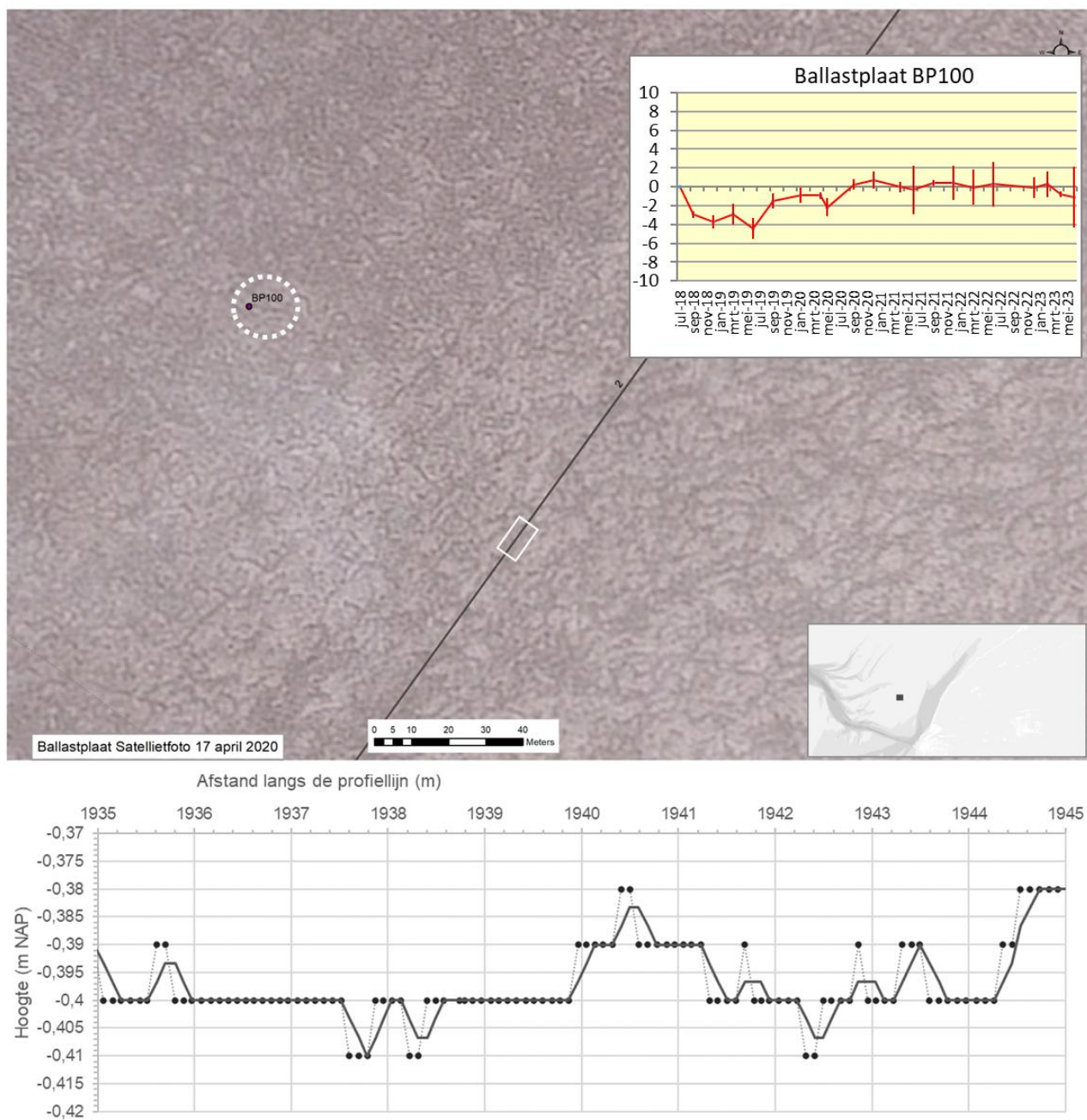
Figuur 9-207 Luchtfoto (17 april 2020) met de locatie van spijkermeting BP100 en raai 2, met daarbij rechtsboven de grafiek met de resultaten van de spijkermetingen bij BP100 en onder de dwarsdoorsnede van raai 2 van de raaimeting uit 2023.
