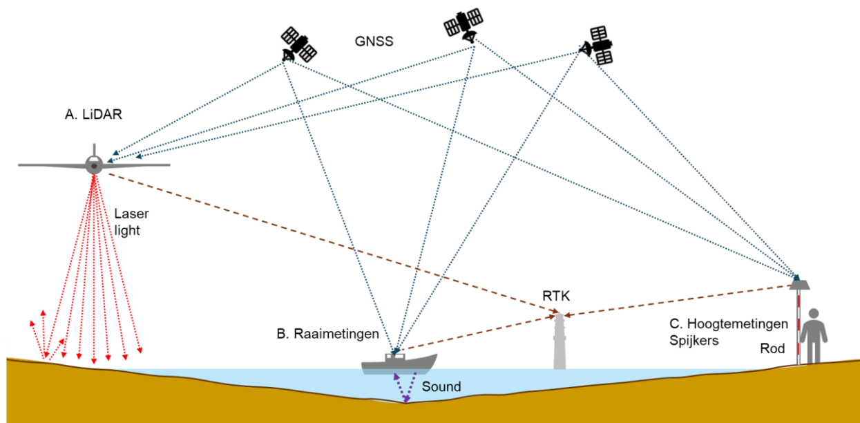
Figuur 6-1 Schematische weergave van de verschillende hoogtemetingen.
