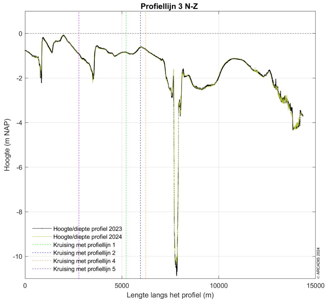
Figuur 3-10 Dwarsprofiel langs profiellijn 3 van noord naar zuid voor de hoogte/diepte raai meetgegevens van 2023 en 2024.
