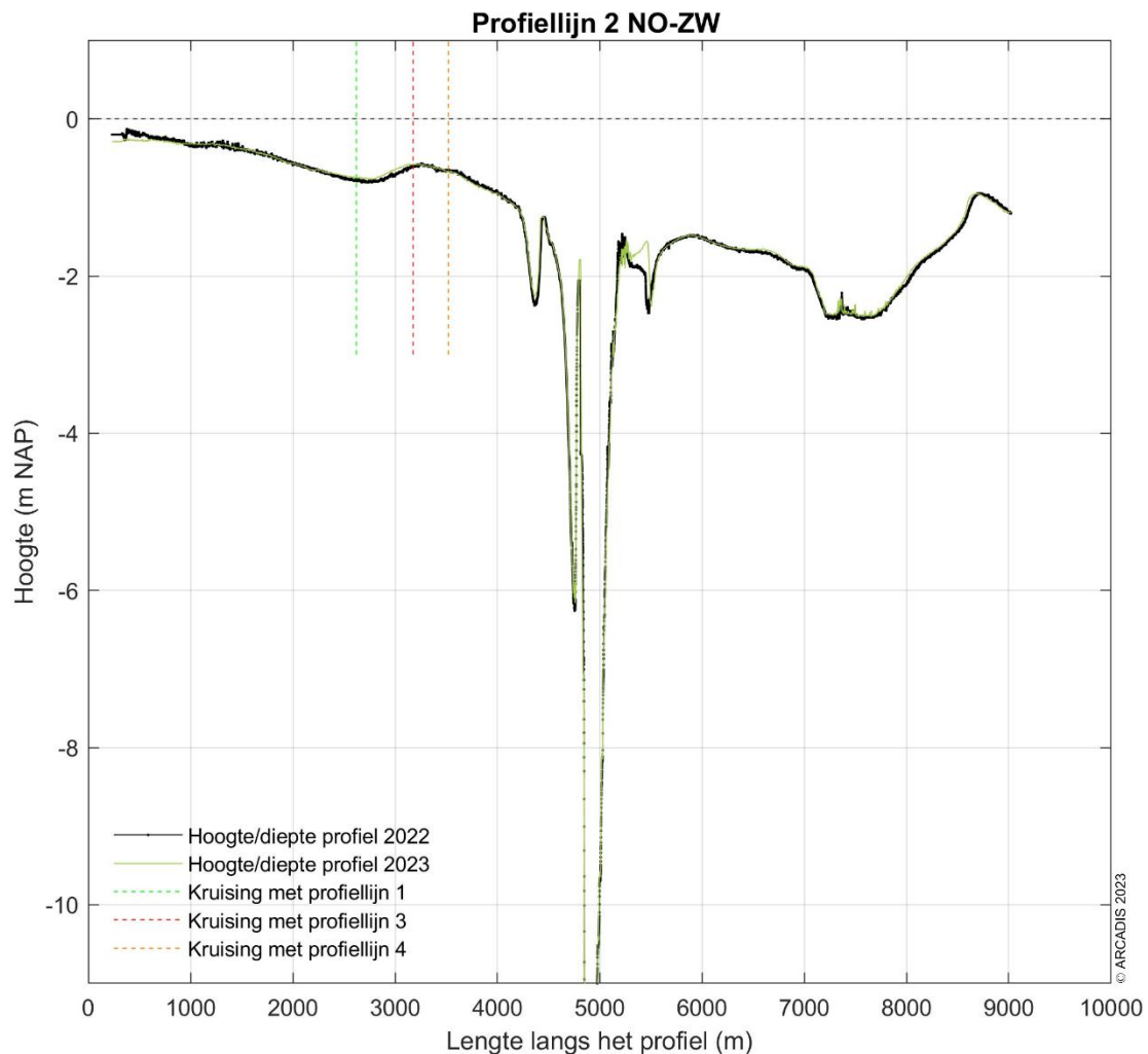
Figuur 9-191 Dwarsdoorsnede langs profiellijn 2 van noordoost naar zuidwest voor de hoogte/diepte raai meetgegevens van 2022 en 2023.
