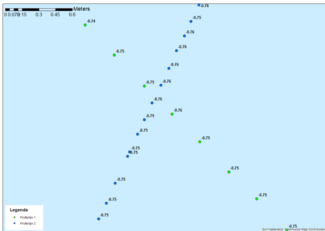
Figuur 9-48 Detailkaart controlepunt tussen profiellijn 1 en profiellijn 2 voor de hoogte/diepte raaien januari 2019, hoogtemetingen zijn weergegeven in m NAP.
