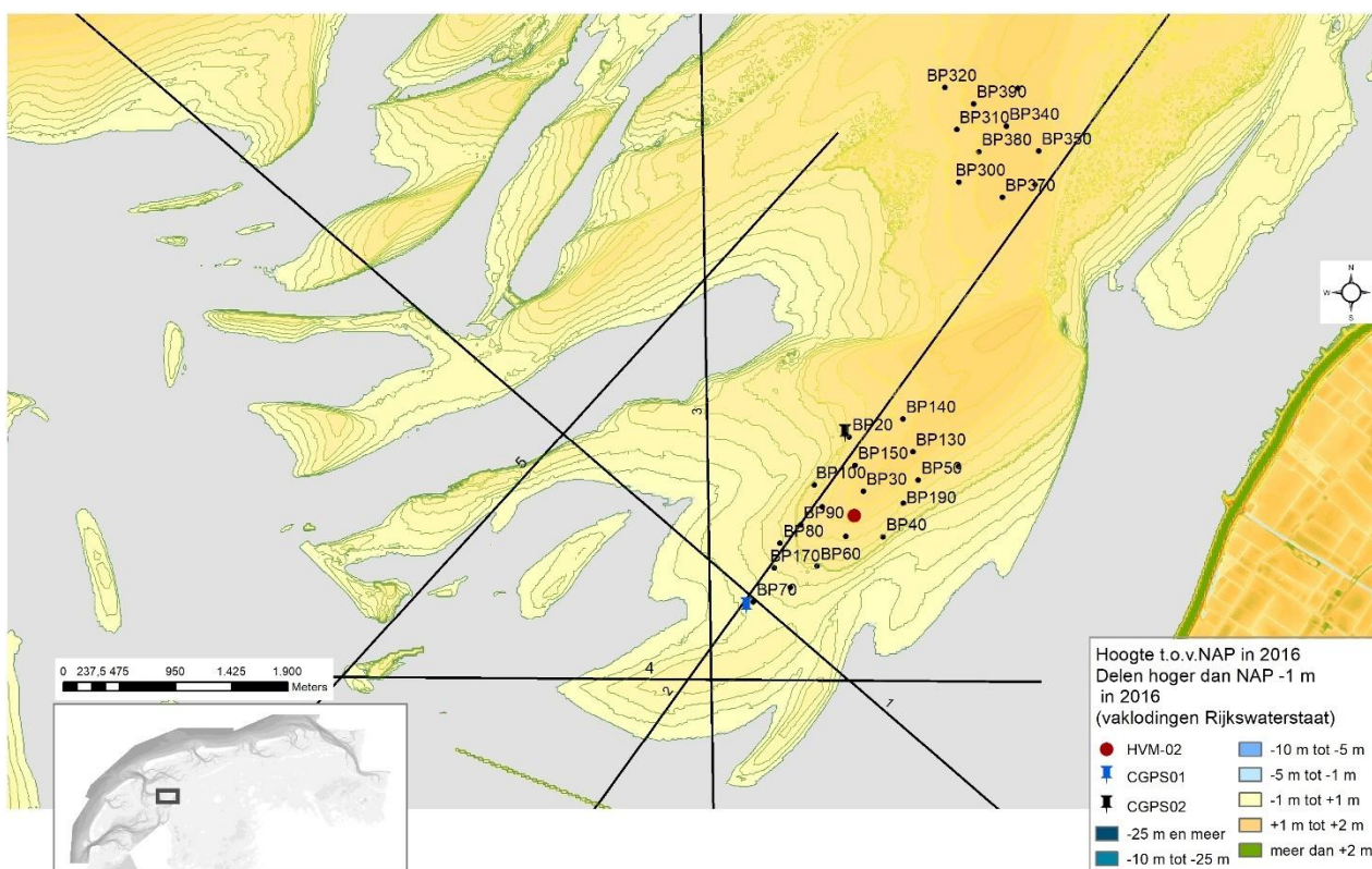
Figuur 7-3 Hoogte van de vakloding 2016, waarbij alleen de delen hoger dan NAP -1 m in 2016 zijn weergegeven.
