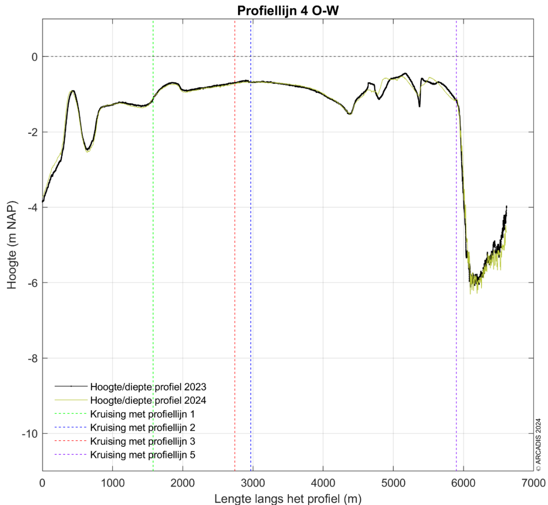
Figuur 3-13 Dwarsprofiel langs profiellijn 4 van oost naar west voor de hoogte/diepte raai meetgegevens van 2023 en 2024.
