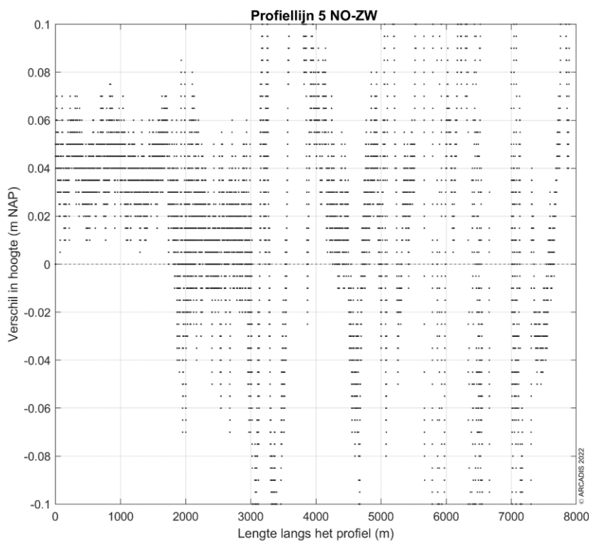
Figuur 9-187: Ingezoomde verschilplot langs profiellijn 5 van noordoost naar zuidwest voor de hoogte/diepte raai meetgegevens van 2021 en 2022. Een positieve waarde betekent dat de hoogte/diepteraai van 2022 hoger ligt dan de hoogte/diepteraai van 2021.
