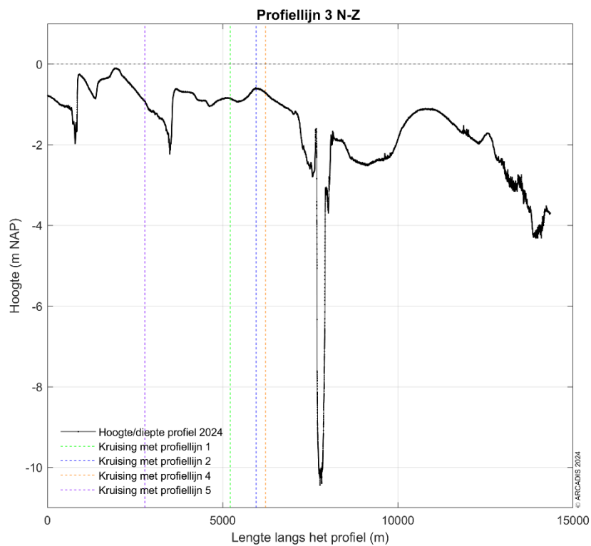
Figuur 9-107 Dwarsdoorsnede langs profiellijn 3 van noord naar zuid in 2024.
