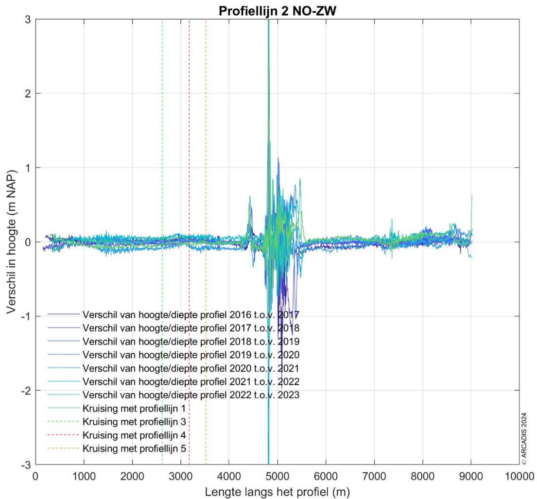
Figuur 4-6 Verschilplot langs profiellijn 2 van noordoost naar zuidwest voor de hoogte/diepte raai meetgegevens tussen 2016-2024. Een positieve waarde betekent dat de hoogte/diepteraai van het opvolgende jaar hoger ligt dan de hoogte/diepteraai van het eerdere jaar.
