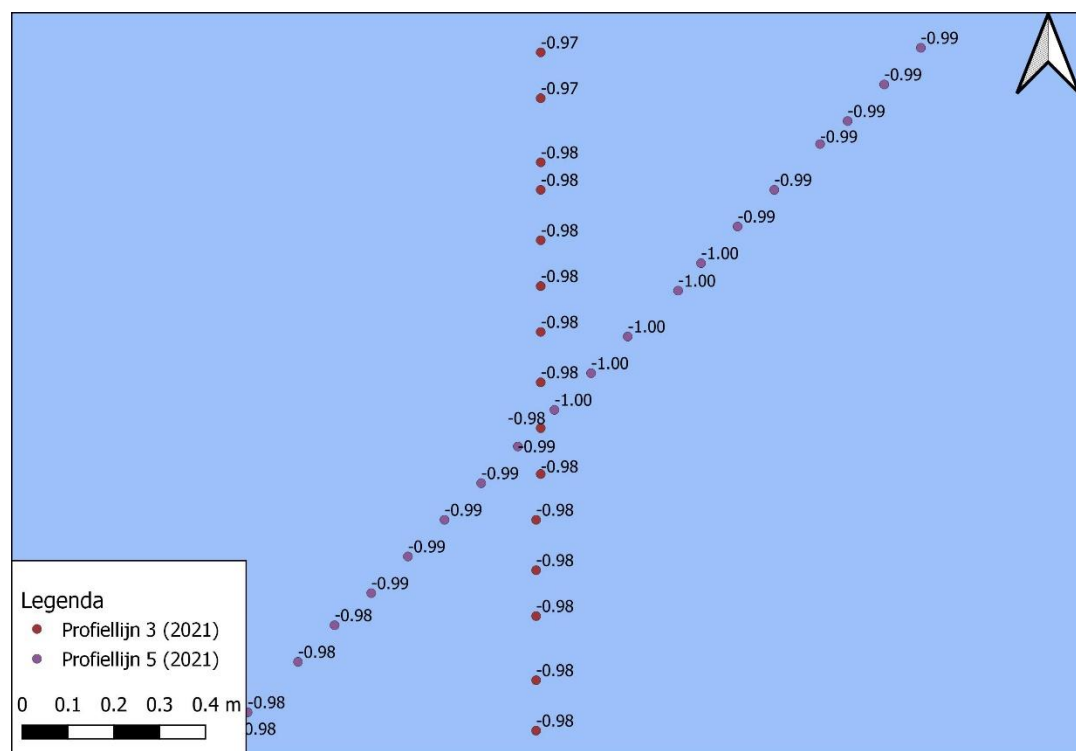
Figuur 9-75 Detailkaart controlepunt tussen profiellijn 3 en profiellijn 5 voor de hoogte/diepte raaien mei 2021, hoogtemetingen zijn weergegeven in m NAP.
