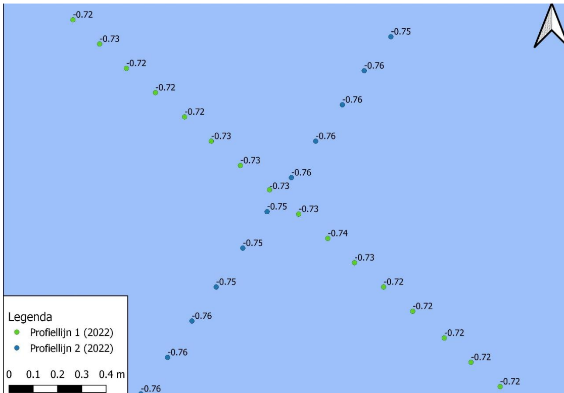
Figuur 9-82 Detailkaart controlepunt tussen profiellijn 1 en profiellijn 2 voor de hoogte/diepte raaien 2022, hoogtemetingen zijn weergegeven in m NAP.
