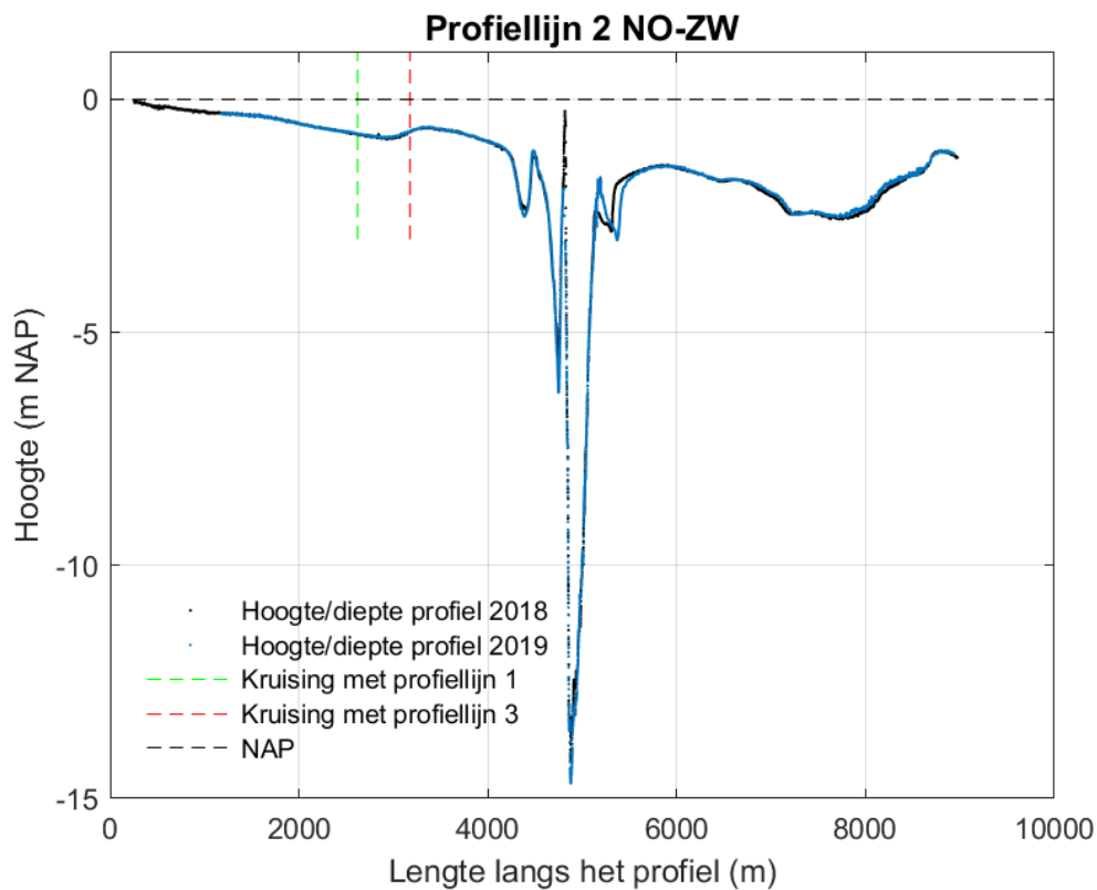
Figuur 9-140 Dwarsdoorsnede langs profiellijn 2 van noordoost naar zuidwest voor de hoogte/diepte raai meetgegevens van 2018 en mei 2019.
