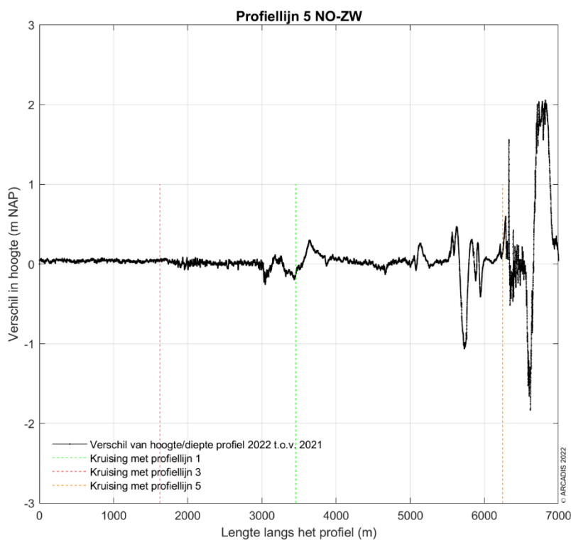
Figuur 9-186 Verschilplot langs profiellijn 5 van noordoost naar zuidwest voor de hoogte/diepte raai meetgegevens van 2021 en 2022. Een positieve waarde betekent dat de hoogte/diepteraai van mei 2022 hoger ligt dan de hoogte/diepteraai van 2021.
