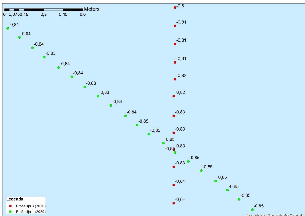
Figuur 9-55 Detailkaart controlepunt tussen profiellijn 1 en profiellijn 3 voor de hoogte/diepte raaien mei 2019, hoogtemetingen zijn weergegeven in m NAP.
