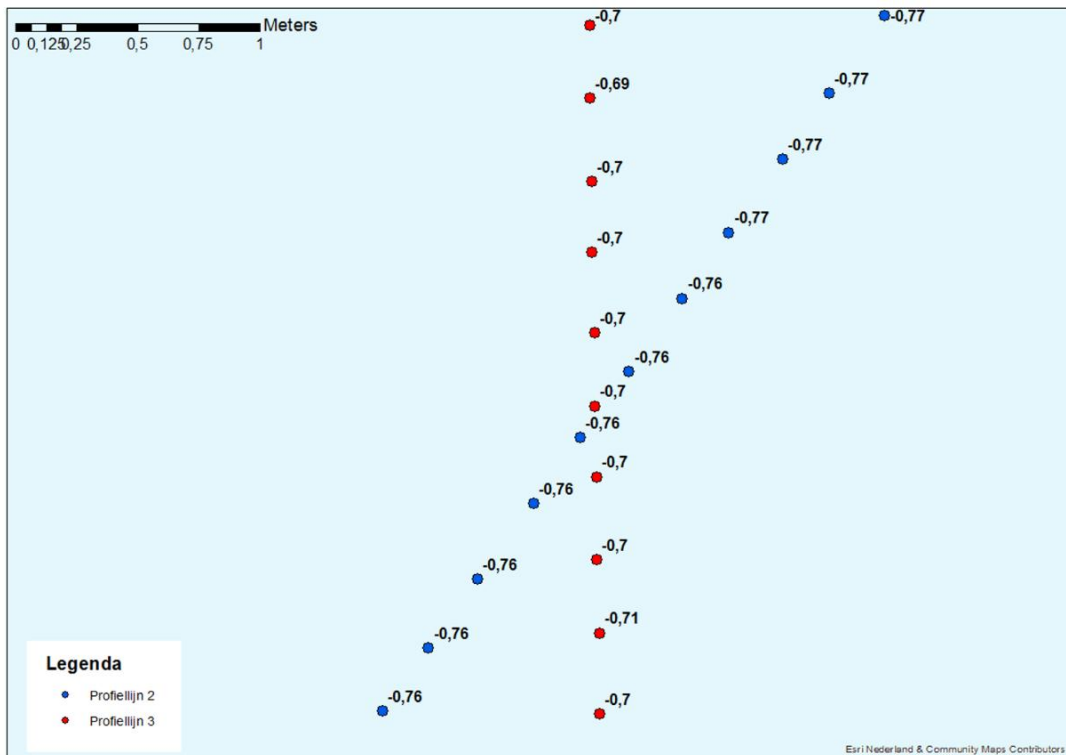
Figuur 9-32 Detailkaart controlepunt tussen profiellijn 2 en profiellijn 3 voor de hoogte/diepte raaien 2016, hoogtemetingen zijn weergegeven in m NAP.
