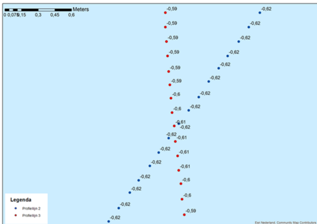
Figuur 9-62 Detailkaart controlepunt tussen profiel 2 en profiel 3 voor de hoogte/diepte raaien 2020, hoogtemetingen zijn weergegeven in m NAP.
