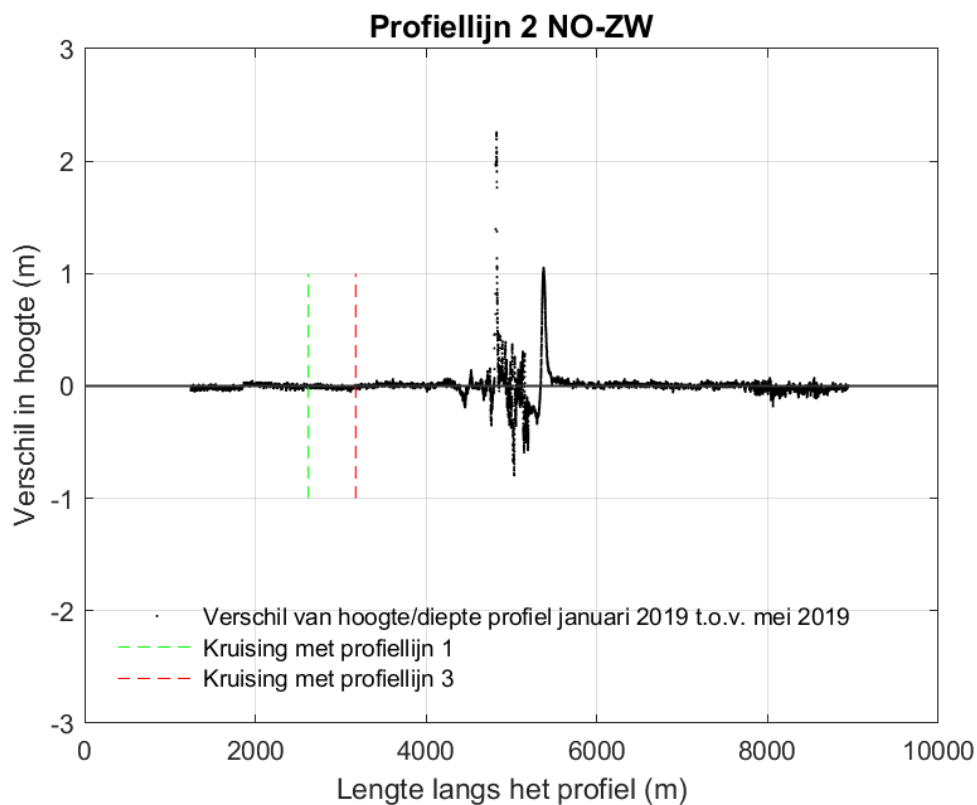
Figuur 9-150 Verschilplot langs profiellijn 2 van noordoost naar zuidwest voor de hoogte/diepte raai meetgegevens van januari 2019 en mei 2019. Een positieve waarde betekent dat de hoogte/diepteraai van mei 2019 hoger ligt dan de hoogte/diepteraai van januari 2019.
