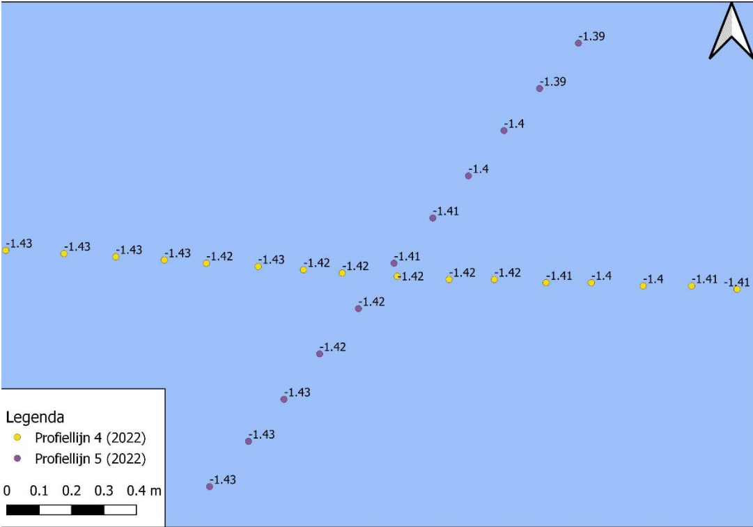
Figuur 9-90 Detailkaart controlepunt tussen profiellijn 4 en profiellijn 5 voor de hoogte/diepte raaien mei 2022, hoogtemetingen zijn weergegeven in m NAP.
