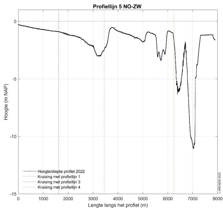
Figuur 9-81 Dwarsdoorsnede langs profiellijn 5 van noordoost naar zuidwest in 2022.
