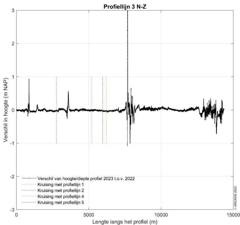
Figuur 9-195 Verschilplot langs profiellijn 3 van noord naar zuid voor de hoogte/diepte raai meetgegevens van 2022 en 2023. Een positieve waarde betekent dat de hoogte/diepteraai van mei 2023 hoger ligt dan de hoogte/diepteraai van 2022.
