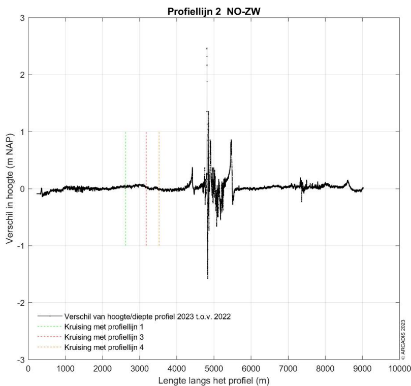
Figuur 9-192 Verschilplot langs profiellijn 2 van noordoost naar zuidwest voor de hoogte/diepte raai meetgegevens van 2022 en 2023. Een positieve waarde betekent dat de hoogte/diepteraai van mei 2023 hoger ligt dan de hoogte/diepteraai van 2022.
