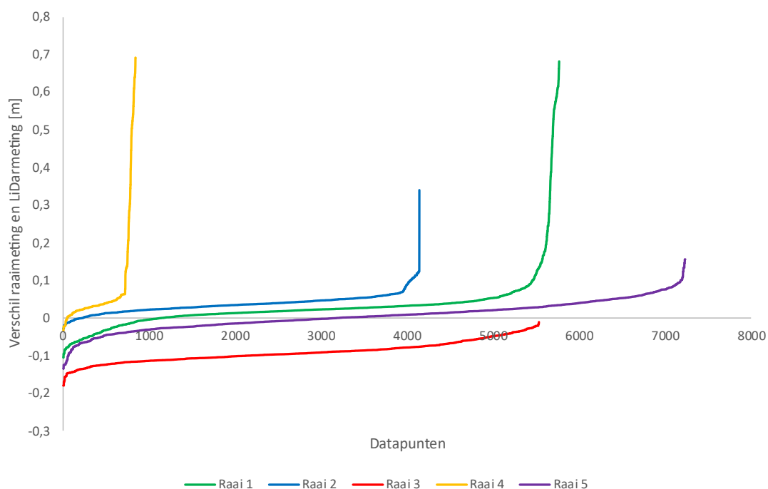
Figuur 9-216: Vergelijking raaimetingen en LiDarmetingen 2022.
