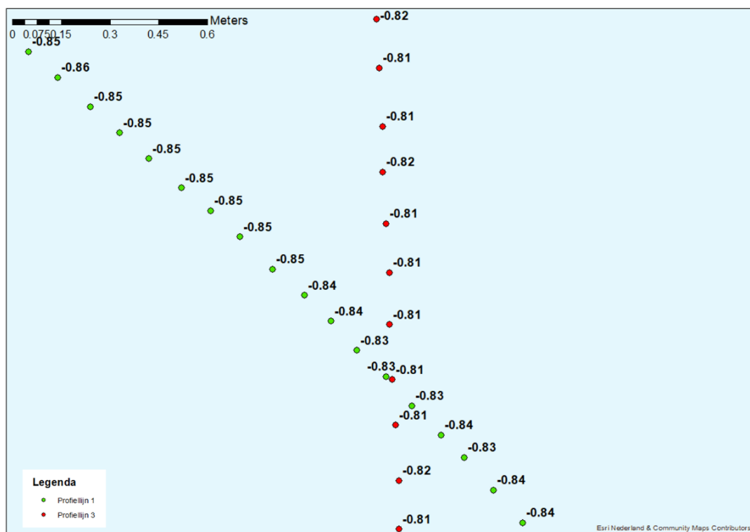
Figuur 9-43 Detailkaart controlepunt tussen profiellijn 1 en profiellijn 3 voor de hoogte/diepte raaien 2018, hoogtemetingen zijn weergegeven in m NAP.
