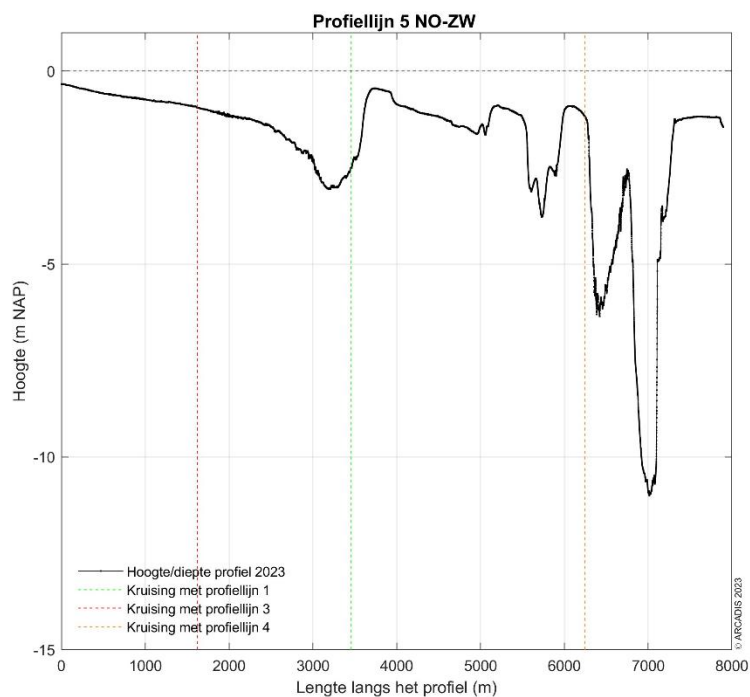
Figuur 9-95 Dwarsdoorsnede langs profiellijn 5 van noordoost naar zuidwest in 2023.
