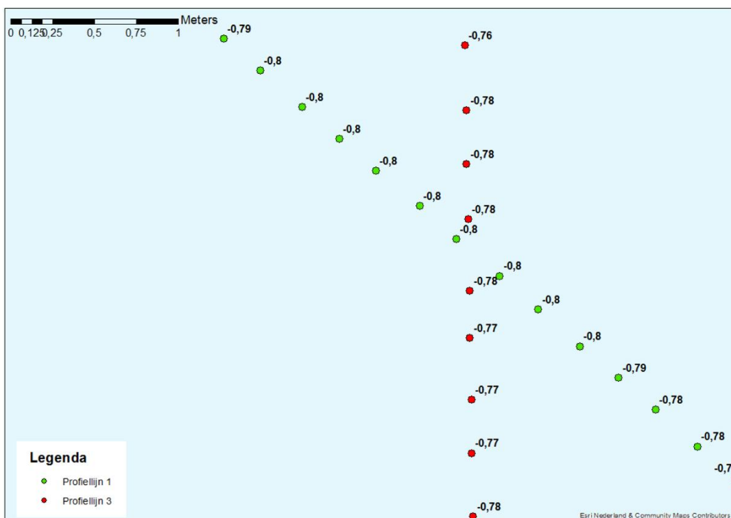
Figuur 9-31 Detailkaart controlepunt tussen profiellijn 1 en profiellijn 3 voor de hoogte/diepte raaien 2016, hoogtemetingen zijn weergegeven in m NAP.
