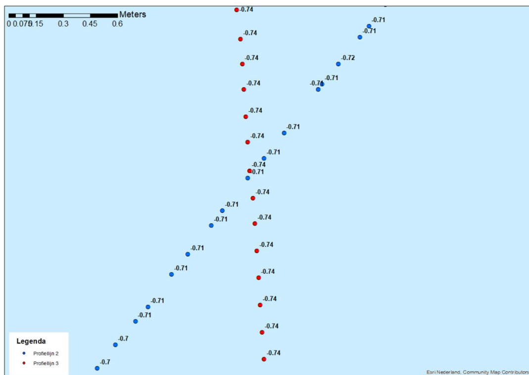
Figuur 9-50 Detailkaart controlepunt tussen profiellijn 2 en profiellijn 3 voor de hoogte/diepte raaien januari 2019, hoogtemetingen zijn weergegeven in m NAP.
