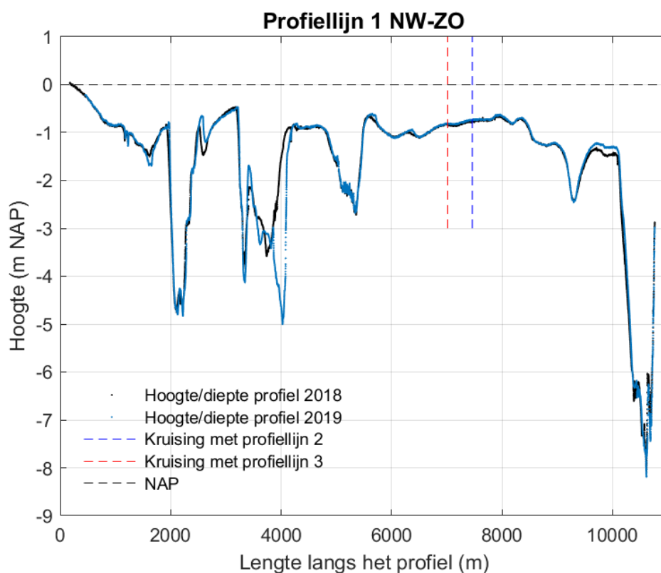
Figuur 9-137 Dwarsdoorsnede langs profiellijn 1 van noordwest naar zuidoost voor de hoogte/diepte raai meetgegevens van 2018 en mei 2019.
