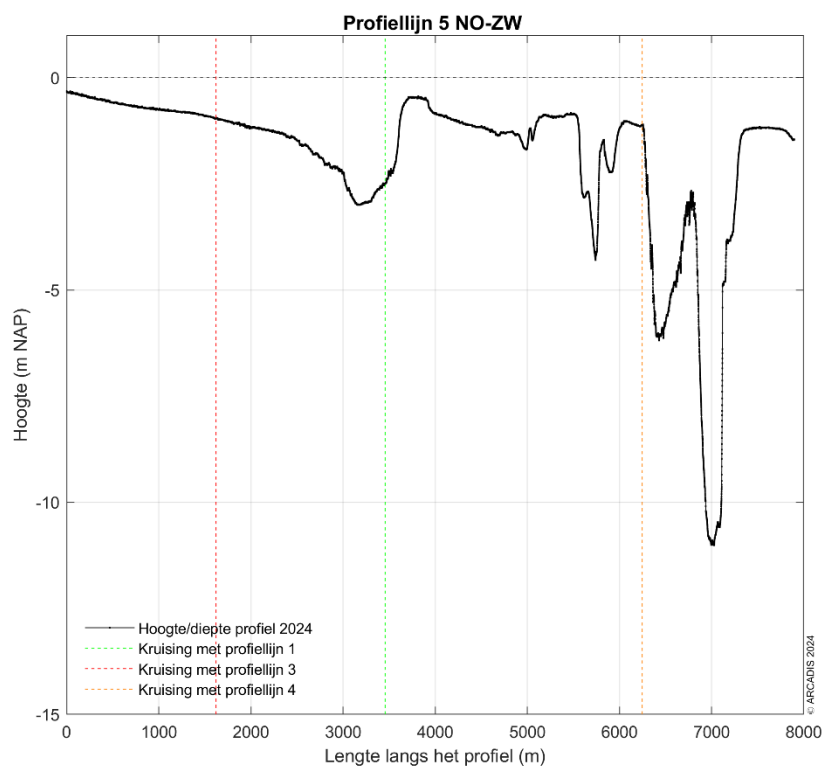
Figuur 9-109 Dwarsdoorsnede langs profiellijn 5 van noordoost naar zuidwest in 2024.
