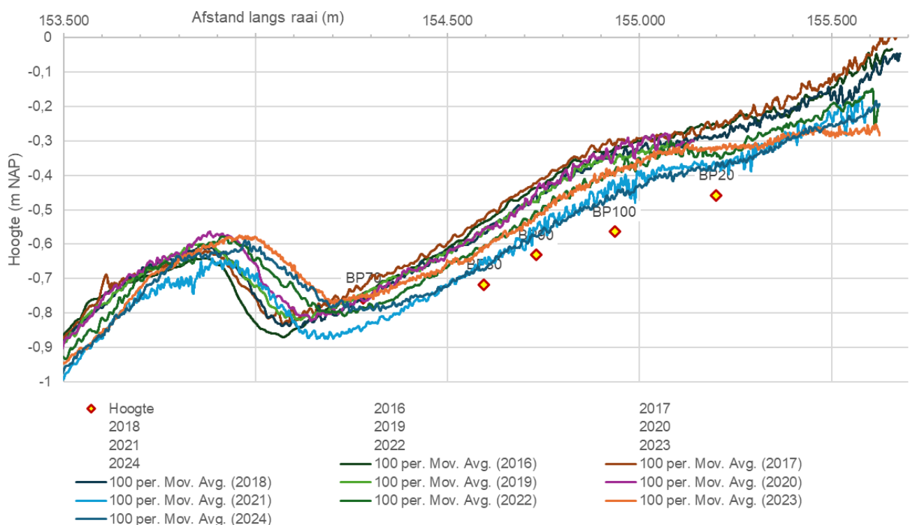
Figuur 6-3 Hoogtemetingen raai 2 en NAP hoogte van de spijkermetingen (25 maart 2024).
