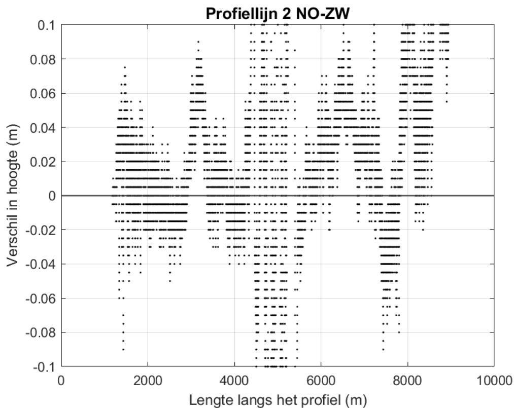
Figuur 9-160 Ingezoomde verschilplot langs profiellijn 2 van noordoost naar zuidwest voor de hoogte/diepte raai meetgegevens van 2019 en 2020. Een positieve waarde betekent dat de hoogte/diepteraai van 2020 hoger ligt dan de hoogte/diepteraai van 2019.
