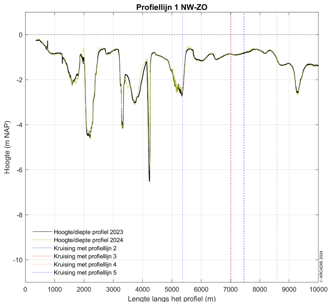
Figuur 3-4 Dwarsdoorsnede langs profiellijn 1 van noordwest naar zuidoost voor de hoogte/diepte raai meetgegevens van 2023 en 2024.
