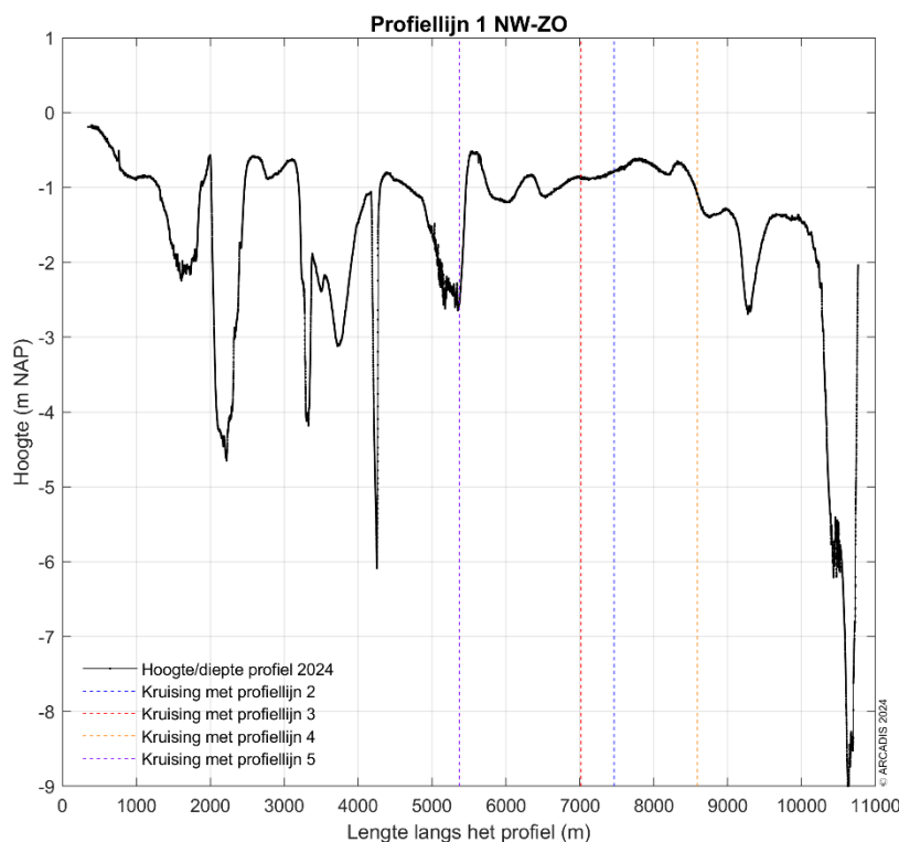
Figuur 9-105 Dwarsdoorsnede langs profiellijn 1 van noordwest naar zuidoost in 2024.
