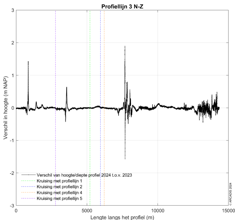
Figuur 3-11 Verschilplot langs profiellijn 3 van noord naar zuid voor de hoogte/diepte raai meetgegevens van 2023 en 2024. Een positieve waarde betekent dat de hoogte/diepteraai van 2024 hoger ligt dan de hoogte/diepteraai van 2023.
