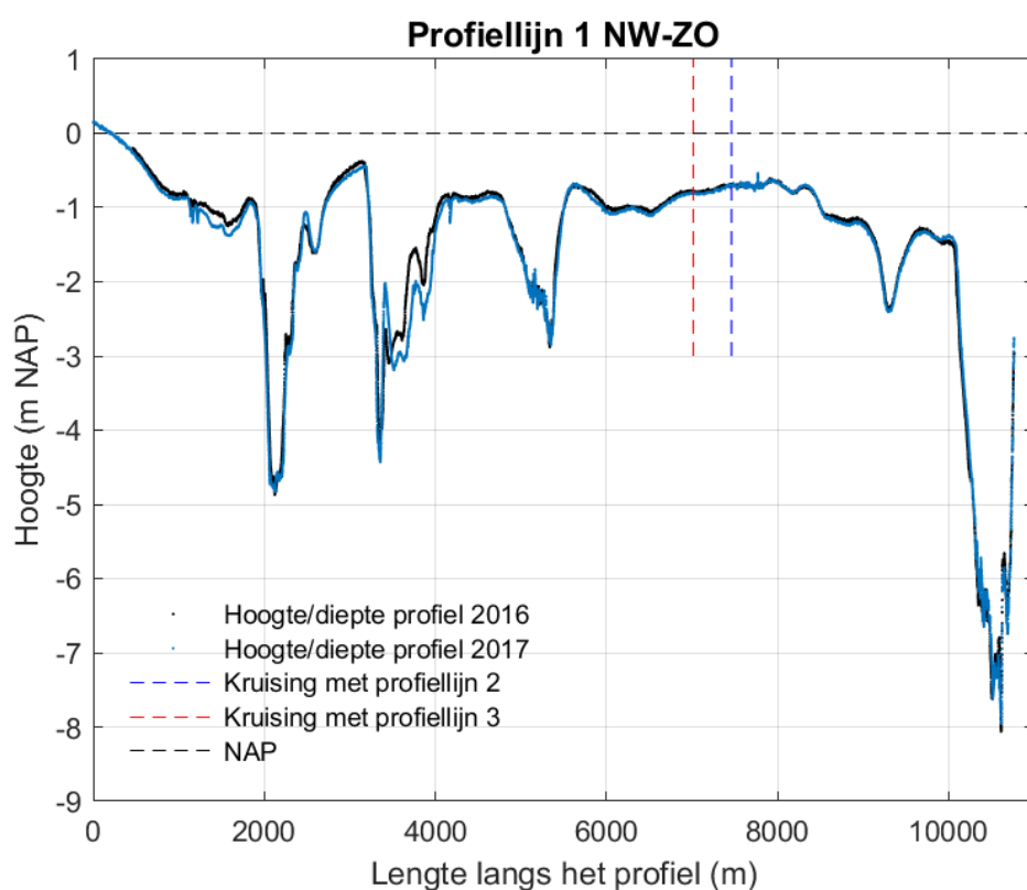
Figuur 9-119 Dwarsdoorsnede langs profiellijn 1 van noordwest naar zuidoost voor de hoogte/diepte raai meetgegevens van 2016 en 2017.
