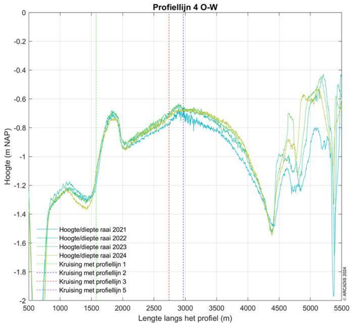
Figuur 4-11 Ingezoomd dwarsprofiel langs profiellijn 4 van noord naar zuid voor de hoogte/diepte raai meetgegevens van 2016 - 2024 (Detail van Figuur 4-10 Figuur 4-7).
