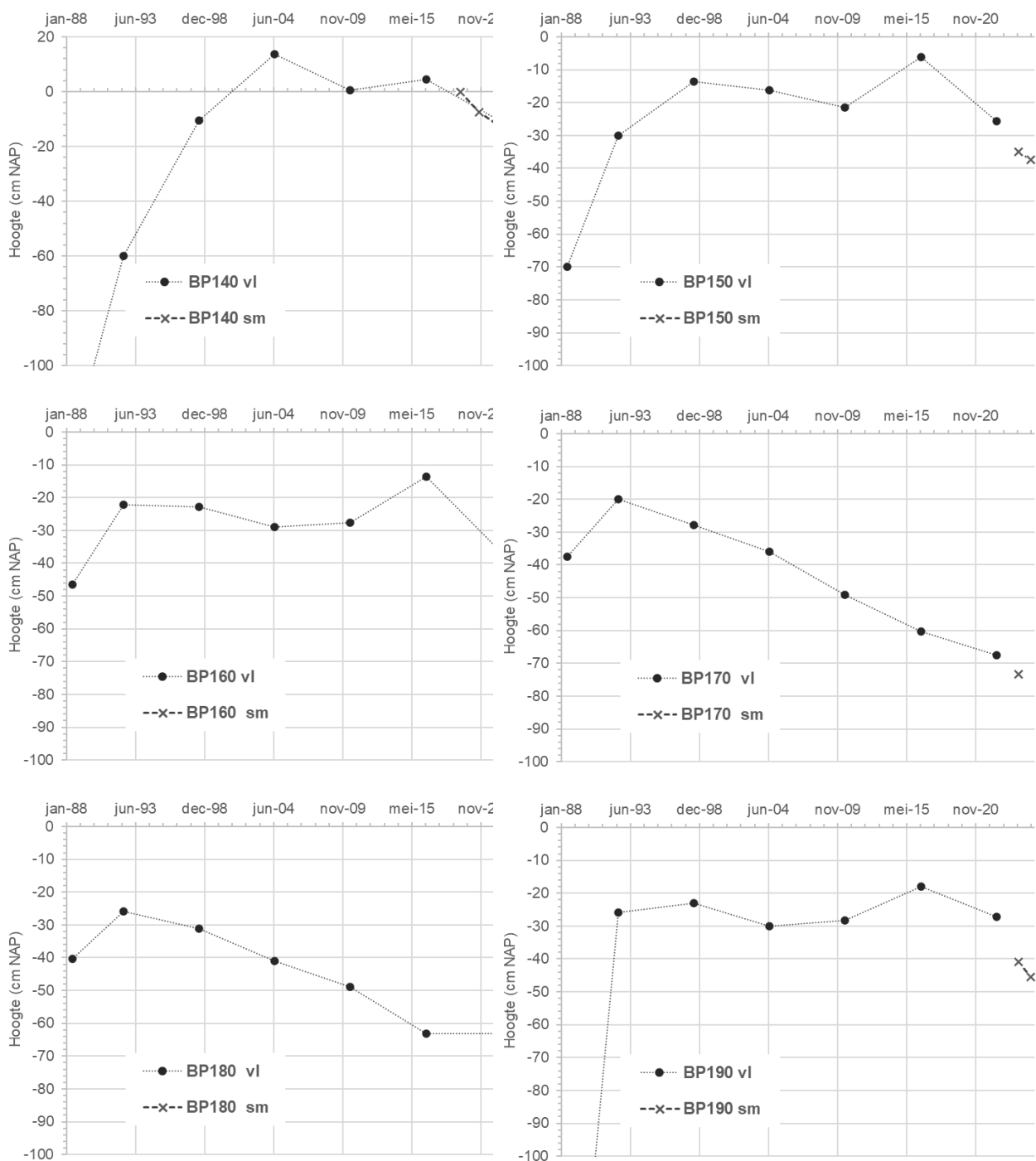
Vervolg van Figuur 6-14. Hoogte ter plaatse van de Spijkermetingen op basis de vakkelingen (vl) en de hoogtemetingen van de locaties van de Spijkermetingen (sm) van de meetpunten op de Ballastplaat Zuid.
