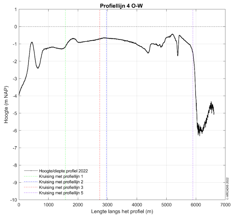
Figuur 9-80 Dwarsdoorsnede langs profiellijn 4 van oost naar west in 2022.
