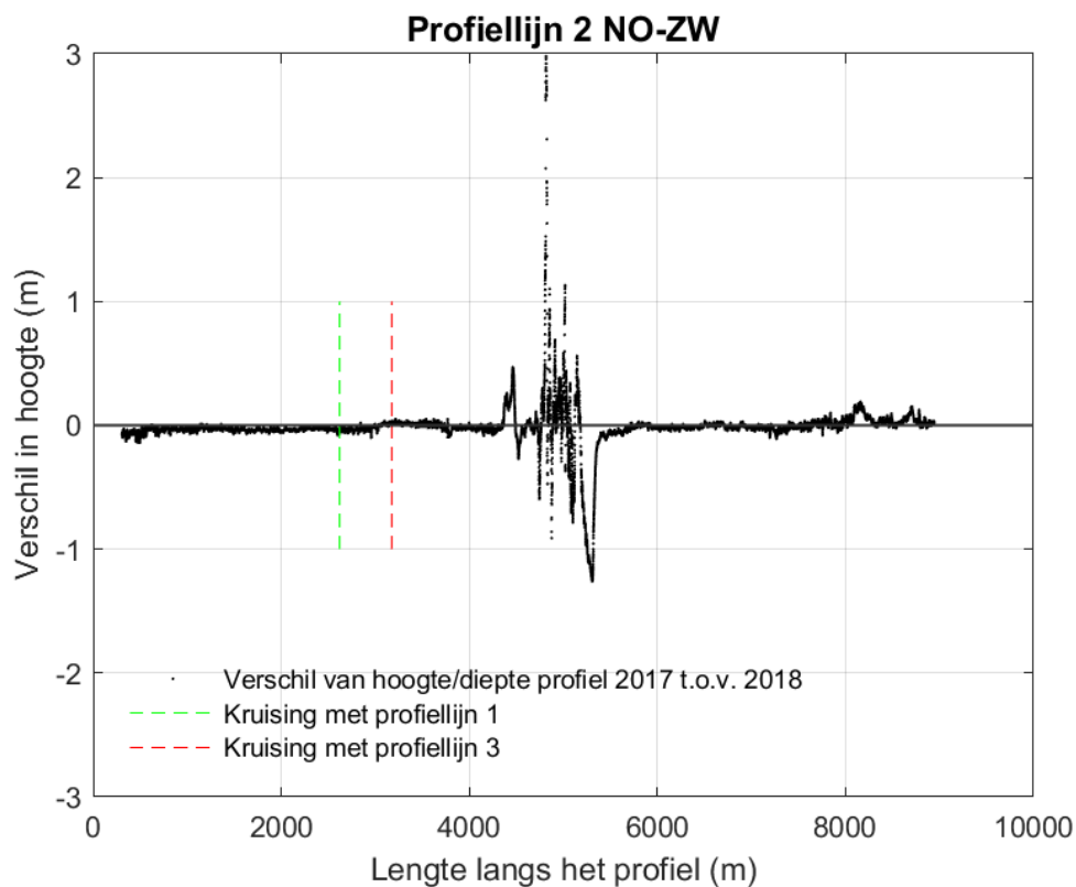
Figuur 9-132 Verschilplot langs profiellijn 2 van noordoost naar zuidwest voor de hoogte/diepte raai meetgegevens van 2017 en 2018. Een negatieve waarde betekent dat de hoogte/diepteraai van 2018 lager ligt dan de hoogte/diepteraai van 2017.
