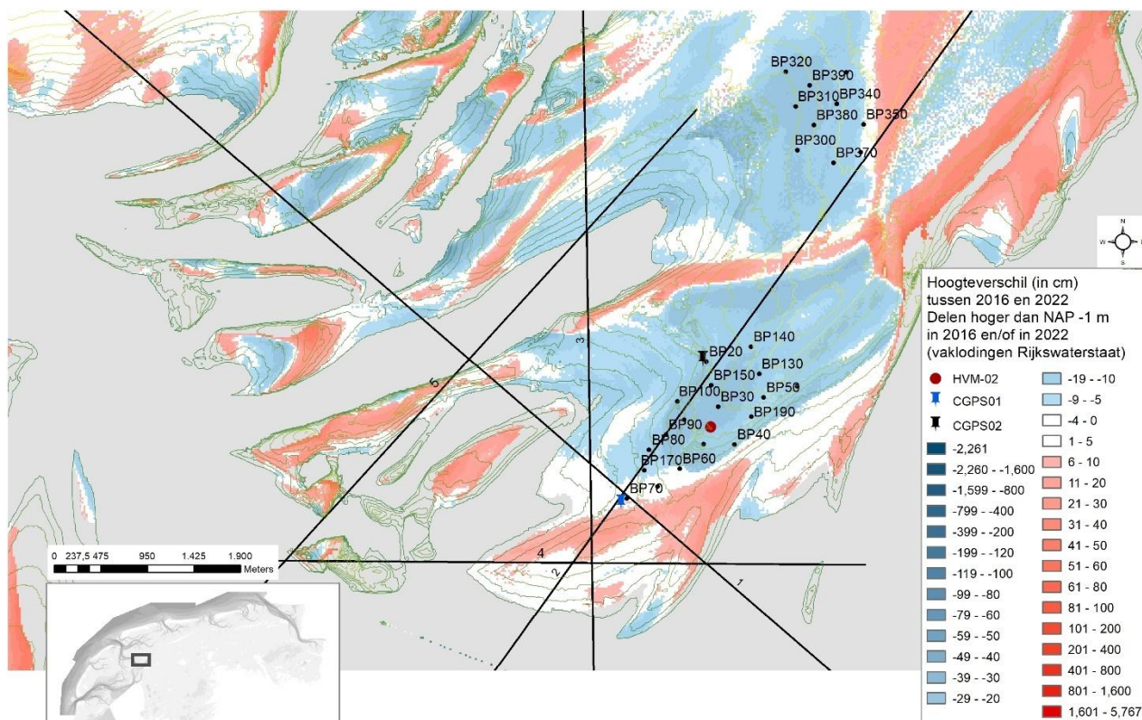
Figuur 7-2 Kaart met het hoogteverschil tussen de vaklodingen 2016 en 2022, waarbij alleen de delen hoger dan NAP -1 m in 2016 en/of 2022 zijn weergegeven.
