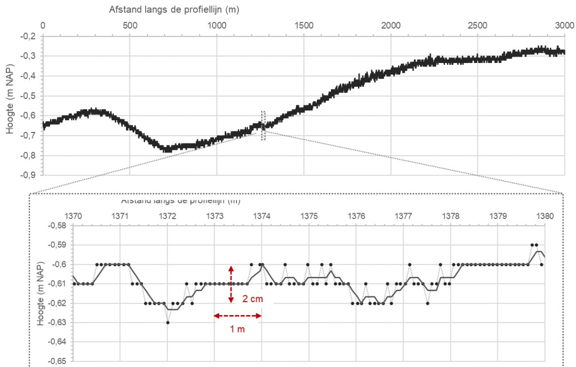
Figuur 9-203 Boven een voorbeeld van de hoogte van de Ballastplaat zoals gemeten in dwarsprofiel langs een stuk van raai 2 van zuidoost naar noordwest. Onder een detail van 10 meter, waarin de bolletjes de meetpunten zijn en de doorgetrokken lijn het 3-punt lopende gemiddelde (meetgegevens 2023).
