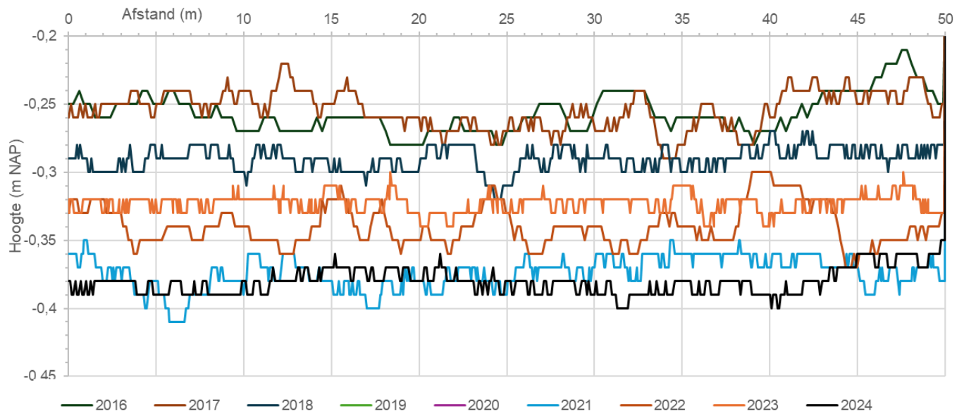
Figuur 6-12 Raaimetingen over afstand van 50 m rond het middelpunt ter hoogte van BP20 (projectie op de raailijn).
