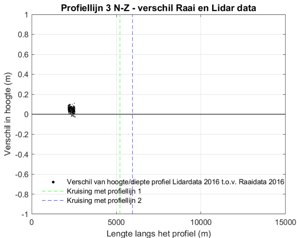
Figuur 9-13 Verschilplot langs profiellijn 3 van noord naar zuid voor de hoogte/diepte raai meetgegevens van 2016 en de LiDAR-data van 2016. Een positieve waarde betekent dat de LiDAR lager ligt dan de hoogte/diepteraai.
