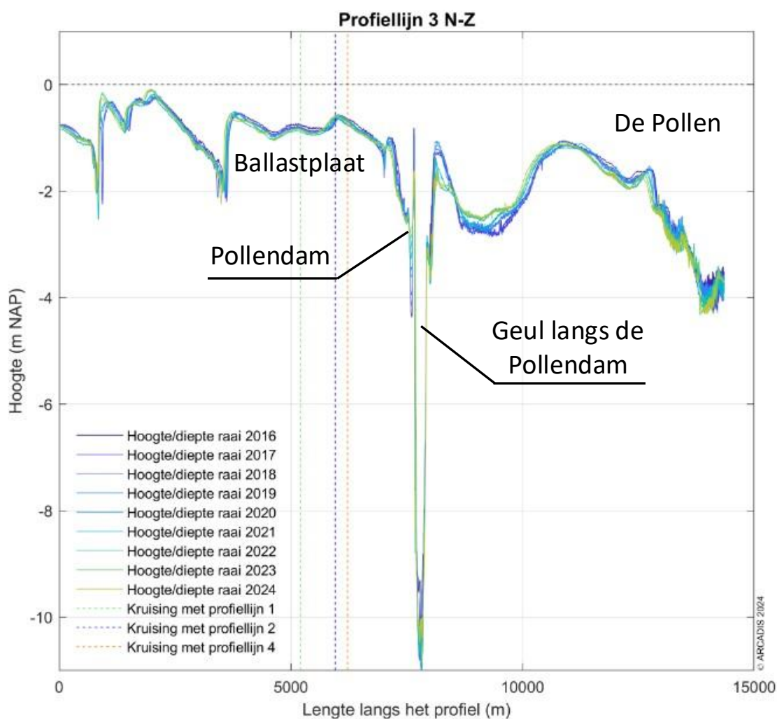
Figuur 4-7 Dwarsprofiel langs profiellijn 3 van noord naar zuid voor de hoogte/diepte raai meetgegevens van 2016 - 2024.
