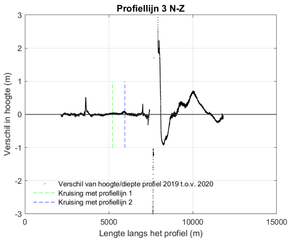
Figuur 9-162 Vershilplot langs profiellijn 3 van noord naar zuid voor de hoogte/diepte raai meetgegevens van 2019 en 2020. Een positieve waarde betekent dat de hoogte/diepteraai van 2020 hoger ligt dan de hoogte/diepteraai van 2019.
