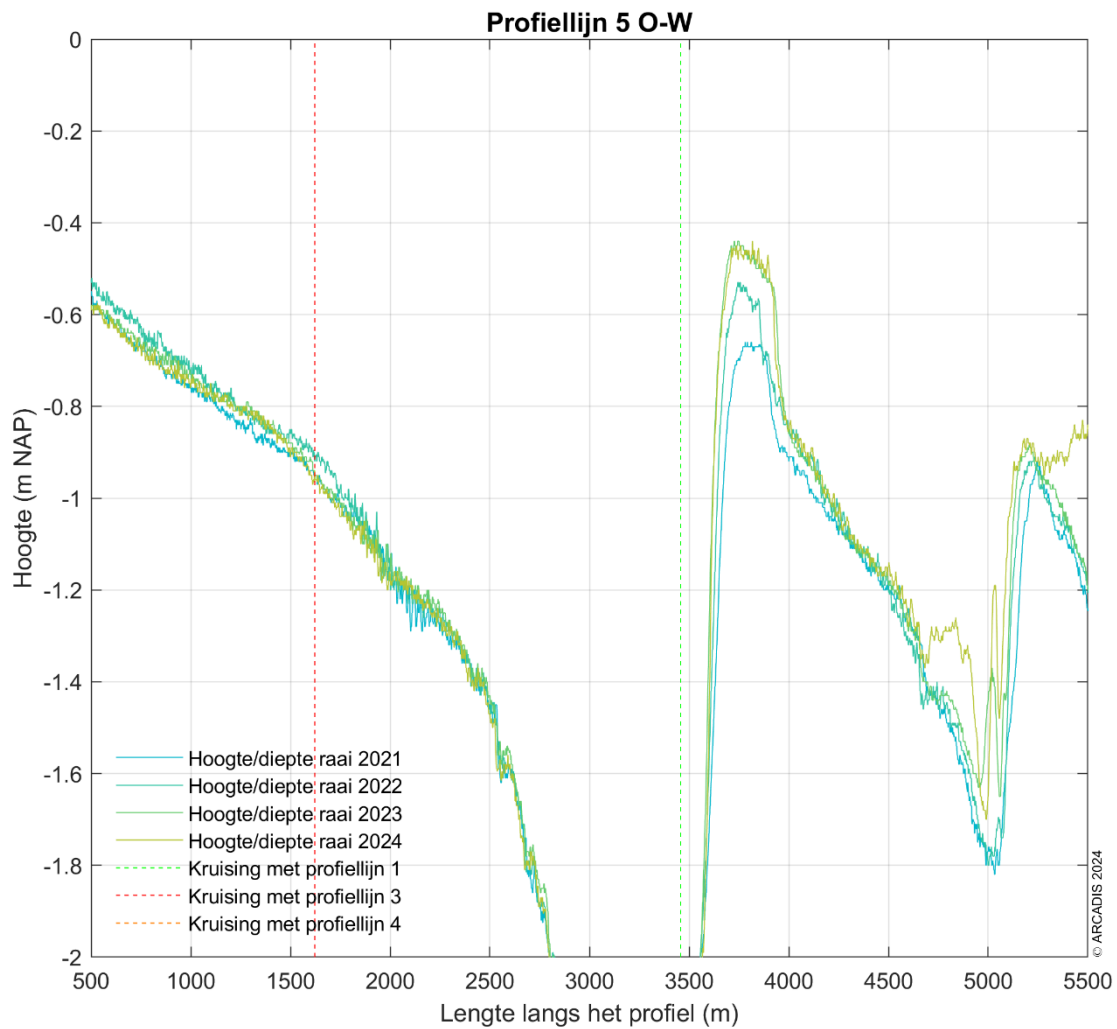
Figuur 4-14 Ingezoomd dwarsprofiel langs profiellijn 5 van noord naar zuid voor de hoogte/diepte raai meetgegevens van 2016 - 2024 (Detail van Figuur 4-13).
