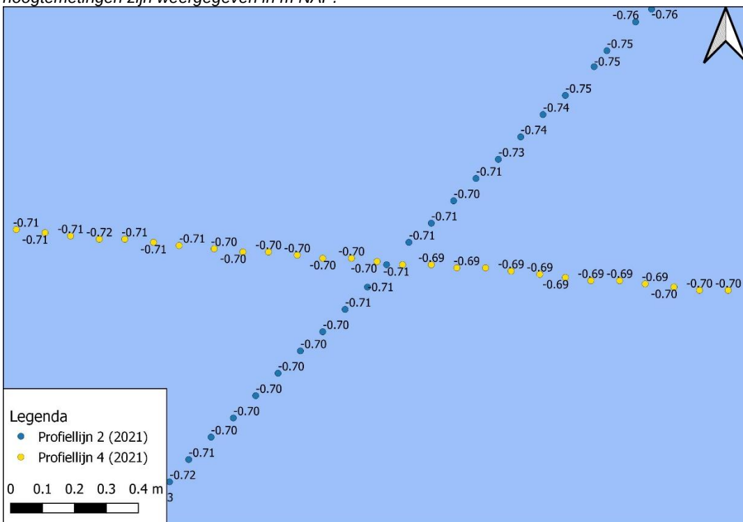
Figuur 9-73 Detailkaart controlepunt tussen profiellijn 2 en profiellijn 4 voor de hoogte/diepte raaien mei 2021, hoogtemetingen zijn weergegeven in m NAP.
