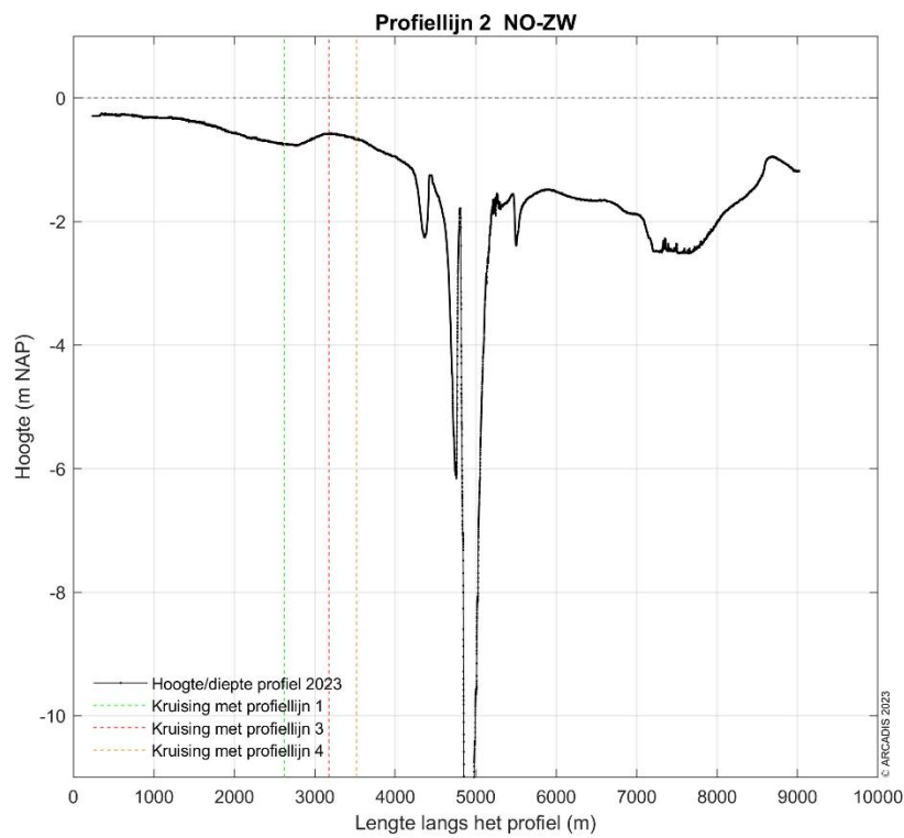
Figuur 9-92 Dwarsdoorsnede langs profiellijn 2 van noordoost naar zuidwest in 2023.
