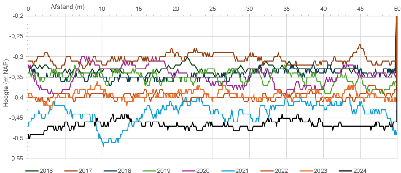
Figuur 6-10 Raaimetingen over afstand van 50 m rond het middelpunt ter hoogte van BP100 (projectie op de raailijn).
