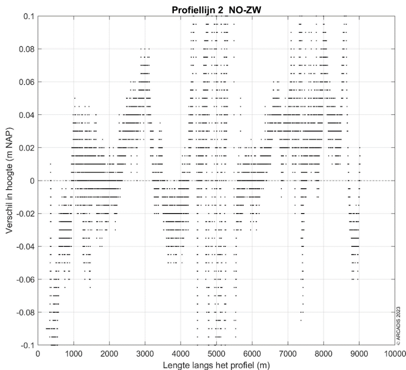
Figuur 9-193 Ingezoomde verschilplot langs profiellijn 2 van noordoost naar zuidwest voor de hoogte/diepte raai meetgegevens van 2022 en 2023. Een positieve waarde betekent dat de hoogte/diepteraai van 2023 hoger ligt dan de hoogte/diepteraai van 2022.
