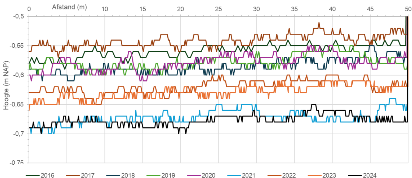
Figuur 6-6 Raaimetingen over afstand van 50 m rond het middelpunt ter hoogte van BP80 (projectie op de raailijn).
