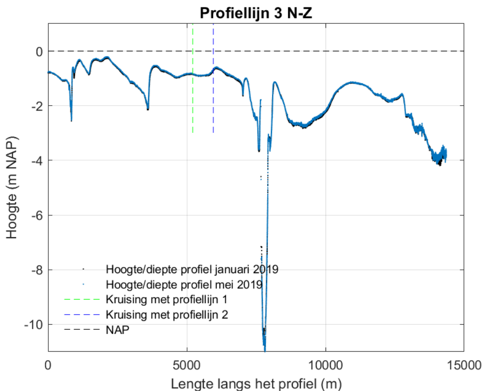
Figuur 9-152 Dwarsprofiel langs profiellijn 3 van noord naar zuid voor de hoogte/diepte raai meetgegevens van januari 2019 en mei 2019.
