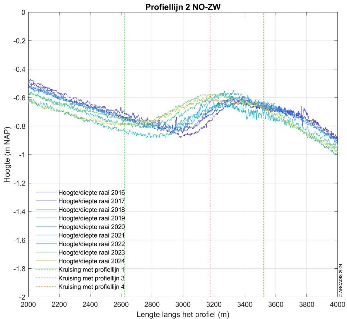
Figuur 4-5 Ingezoomd dwarsprofiel langs profiellijn 2 van noordoost naar zuidwest voor de hoogte/diepte raai meetgegevens van 2016 – 2024 (Detail van Figuur 4-4).
