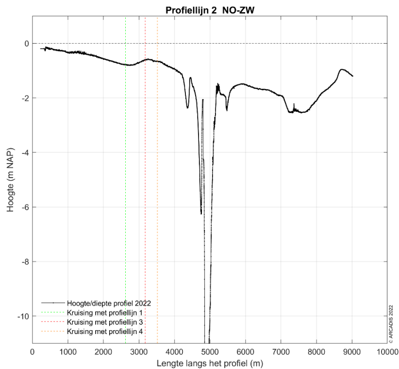
Figuur 9-78 Dwarsdoorsnede langs profiellijn 2 van noordoost naar zuidwest in 2022.
