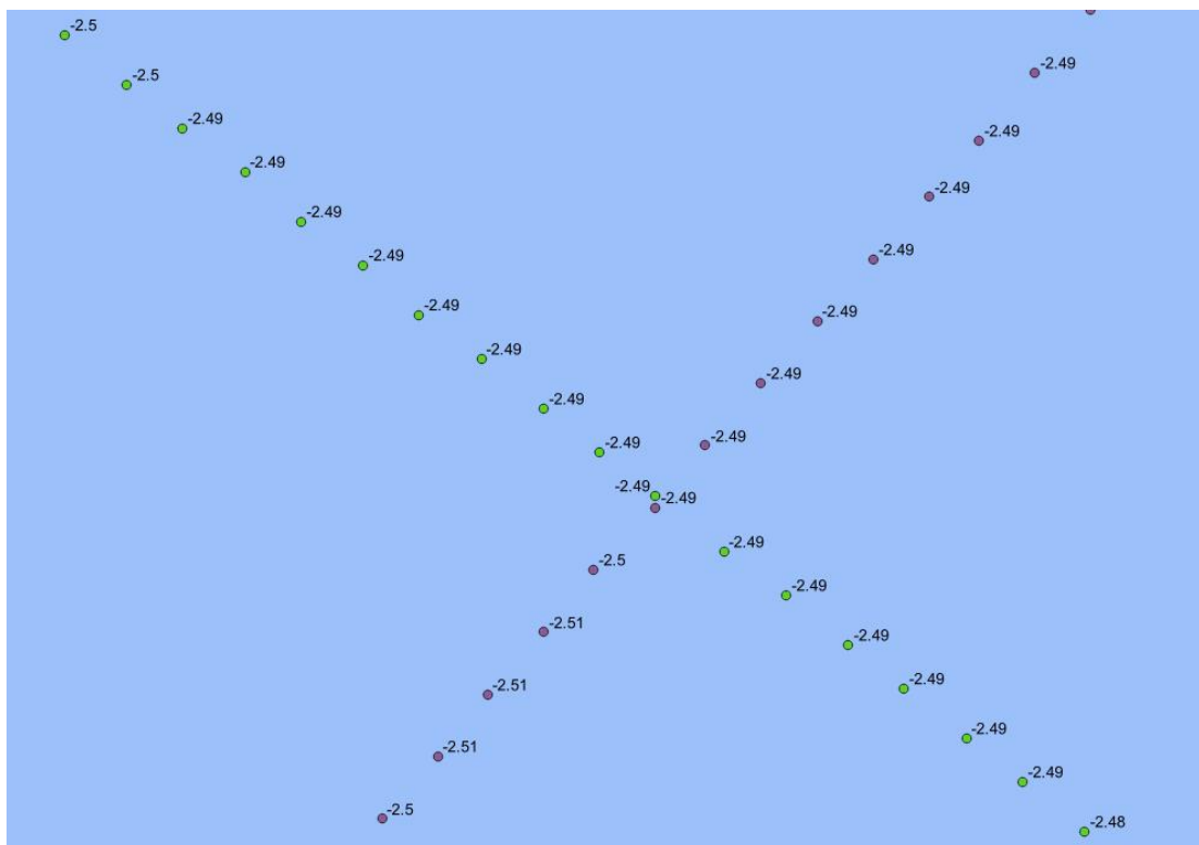
Figuur 9-99 Detailkaart controlepunt tussen profiellijn 1 en profiellijn 5 voor de hoogte/diepte raaien 2023, hoogtemetingen zijn weergegeven in m NAP.
