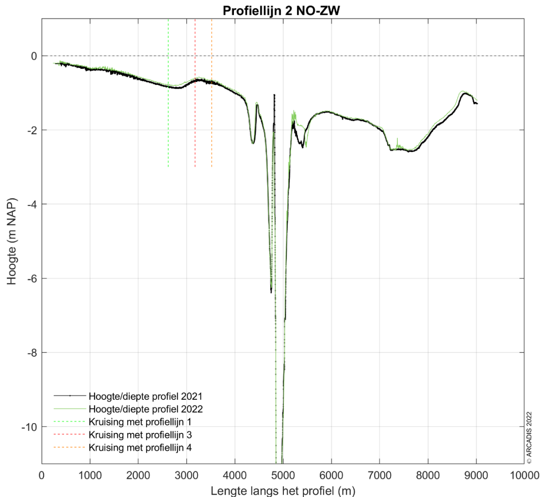
Figuur 9-176 Dwarsdoorsnede langs profiellijn 2 van noordoost naar zuidwest voor de hoogte/diepte raai meetgegevens van 2021 en 2022.
