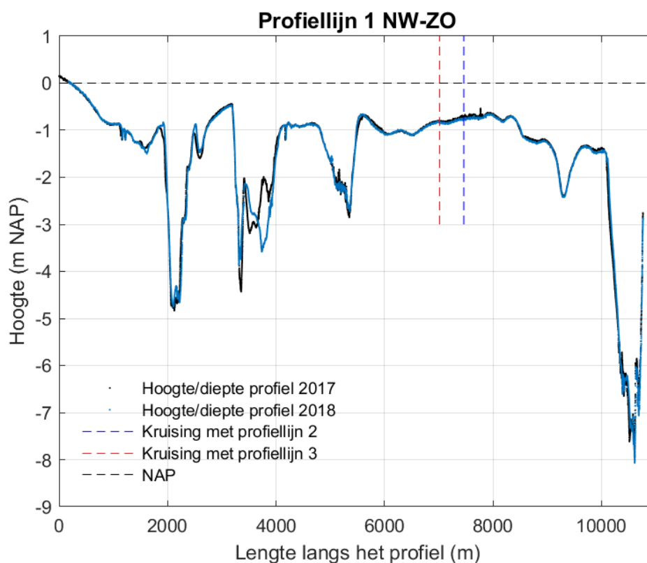
Figuur 9-128 Dwarsdoorsnede langs profiellijn 1 van noordwest naar zuidoost voor de hoogte/diepte raai meetgegevens van 2017 en 2018.
