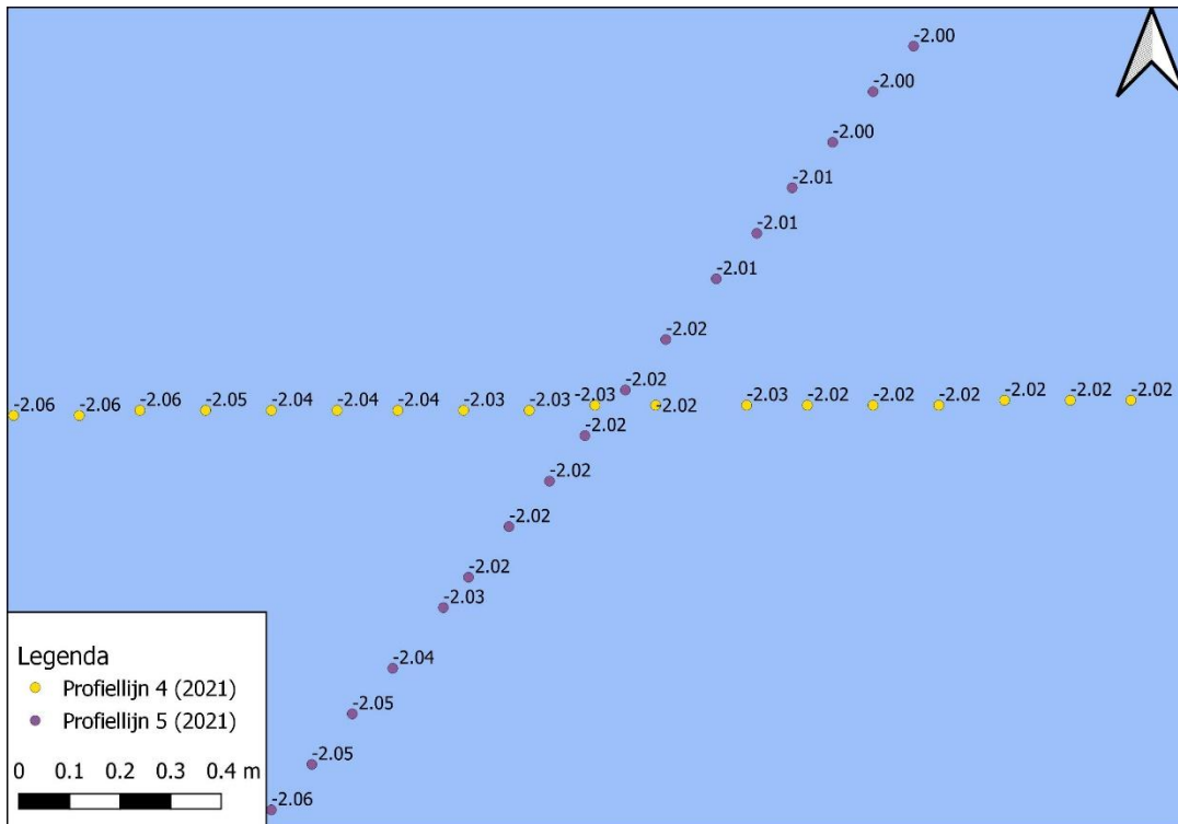
Figuur 9-76 Detailkaart controlepunt tussen profiellijn 4 en profiellijn 5 voor de hoogte/diepte raaien mei 2021, hoogtemetingen zijn weergegeven in m NAP.
