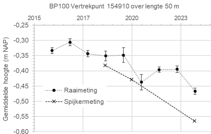
Figuur 6-11 Hoogte van de raaimetingen en de Spijkermetingen bij BP100.
