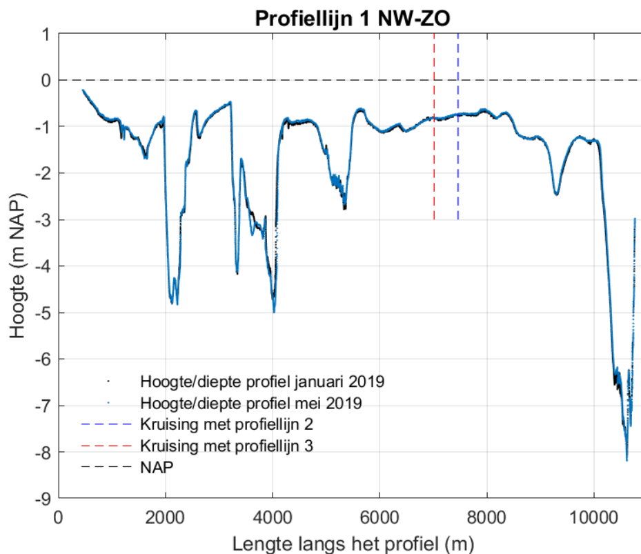
Figuur 9-146 Dwarsdoorsnede langs profiellijn 1 van noordwest naar zuidoost voor de hoogte/diepte raai meetgegevens van januari 2019 en mei 2019.
