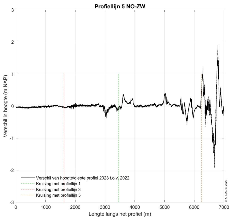
Figuur 9-201 Verschilplot langs profiellijn 5 van noordoost naar zuidwest voor de hoogte/diepte raai meetgegevens van 2022 en 2023. Een positieve waarde betekent dat de hoogte/diepteraai van mei 2023 hoger ligt dan de hoogte/diepteraai van 2022.
