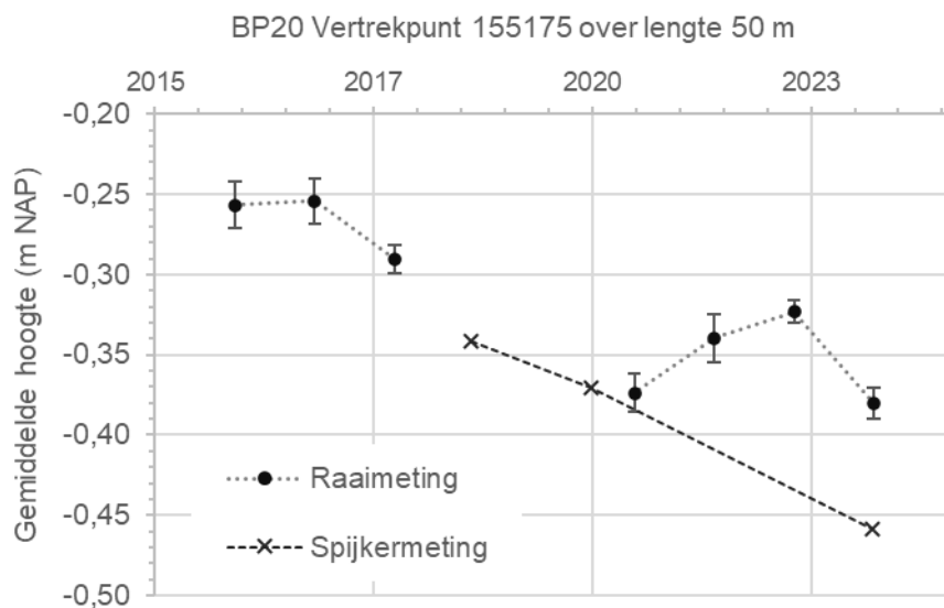
Figuur 6-13 Hoogte van de raaimetingen en de Spijkermetingen bij BP20.
