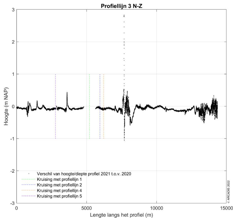
Figuur 9-171 Verskilplot langs profiellijn 3 van noord naar zuid voor de hoogte/diepte raai meetgegevens van 2020 en 2021. Een positieve waarde betekent dat de hoogte/diepteraai van mei 2021 hoger ligt dan de hoogte/diepteraai van 2020.
