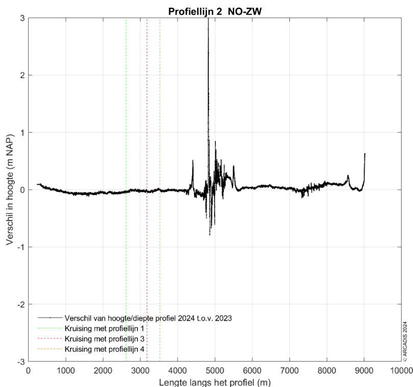
Figuur 3-8 Verschilplot langs profiellijn 2 van noordoost naar zuidwest voor de hoogte/diepte raai meetgegevens van 2023 en 2024. Een positieve waarde betekent dat de hoogte/diepteraai van 2024 hoger ligt dan de hoogte/diepteraai van 2023.
