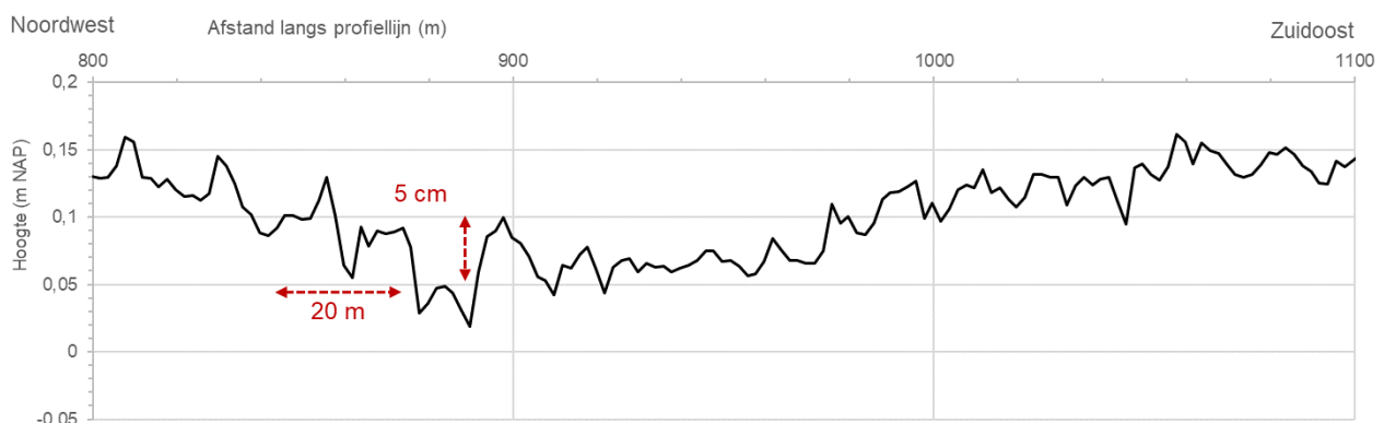
Figuur 9-219 Boven: Hoogte van de Ballastplaat volgens de LiDAR 2022 in dwarsprofiel DD' (locatie in Figuur 9-217) van noordwest naar zuidoost. Onder: Detail van 300 meter (bron gegevens Rijkswaterstaat).
