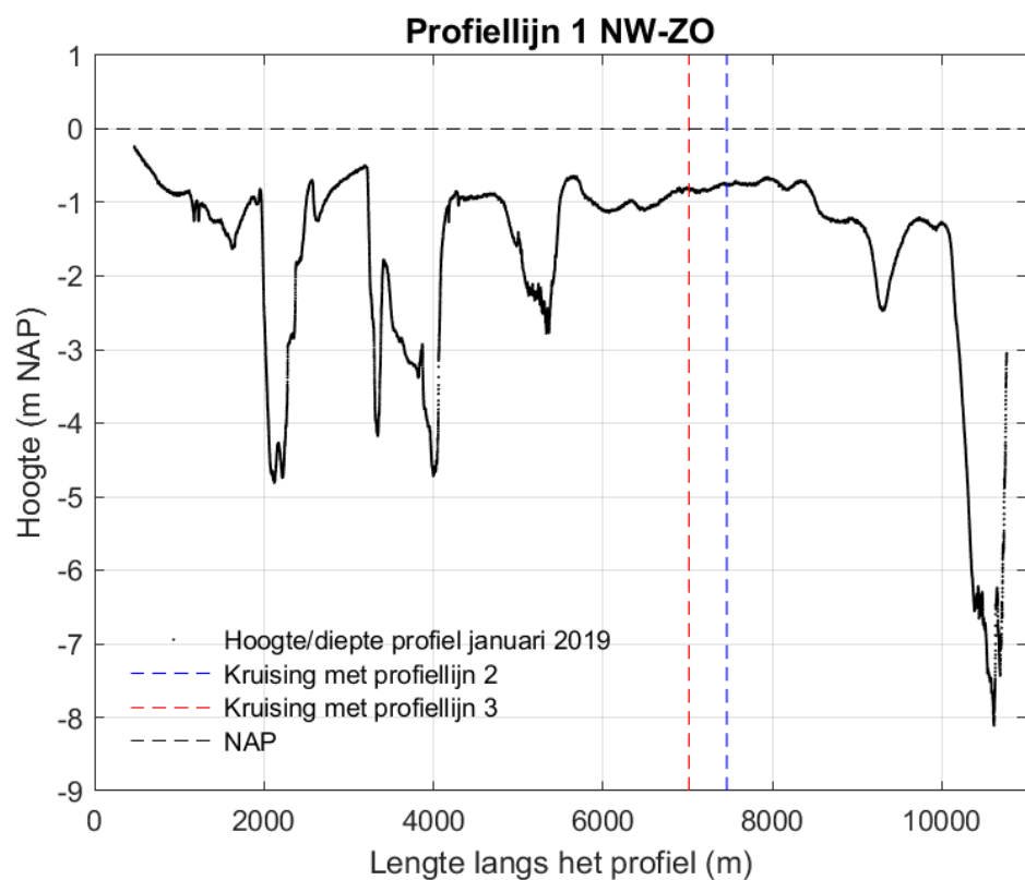
Figuur 9-45 Dwarsdoorsnede langs profiel 1 van noordwest naar zuidoost in januari 2019.
