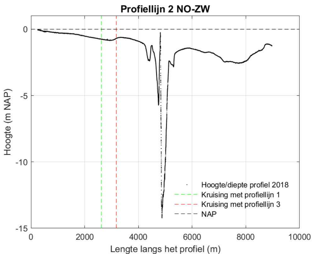
Figuur 9-40 Dwarsdoorsnede langs profiellijn 2 van noordoost naar zuidwest in 2018.
