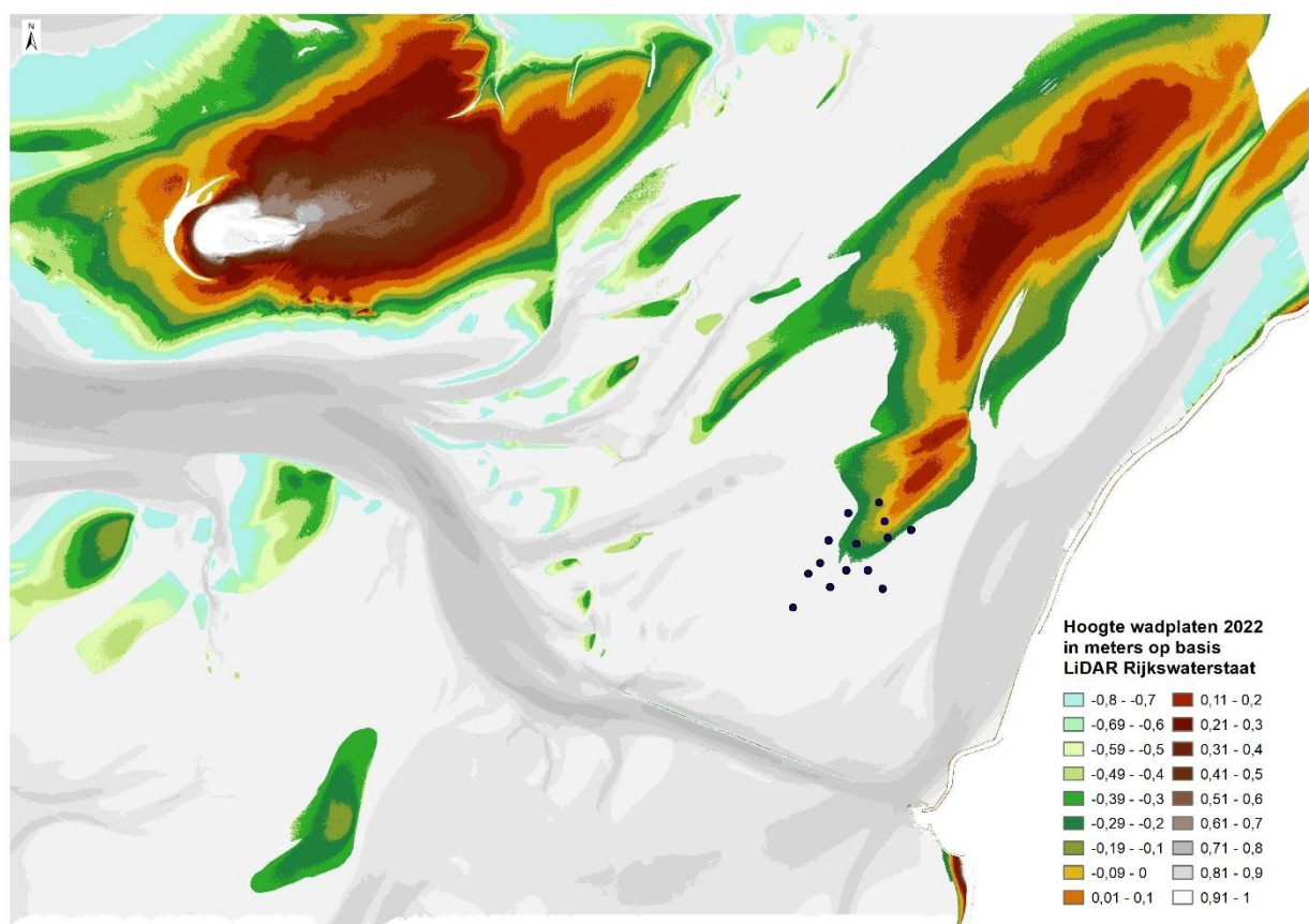
Figuur 9-212 Kaart met de hoogte van de wadplaten, zoals in 2022 ingemeten met LiDAR voor de vaklodingen. De zwarte stippen zijn de locaties van de Spijkermetingen op de Ballastplaat.
