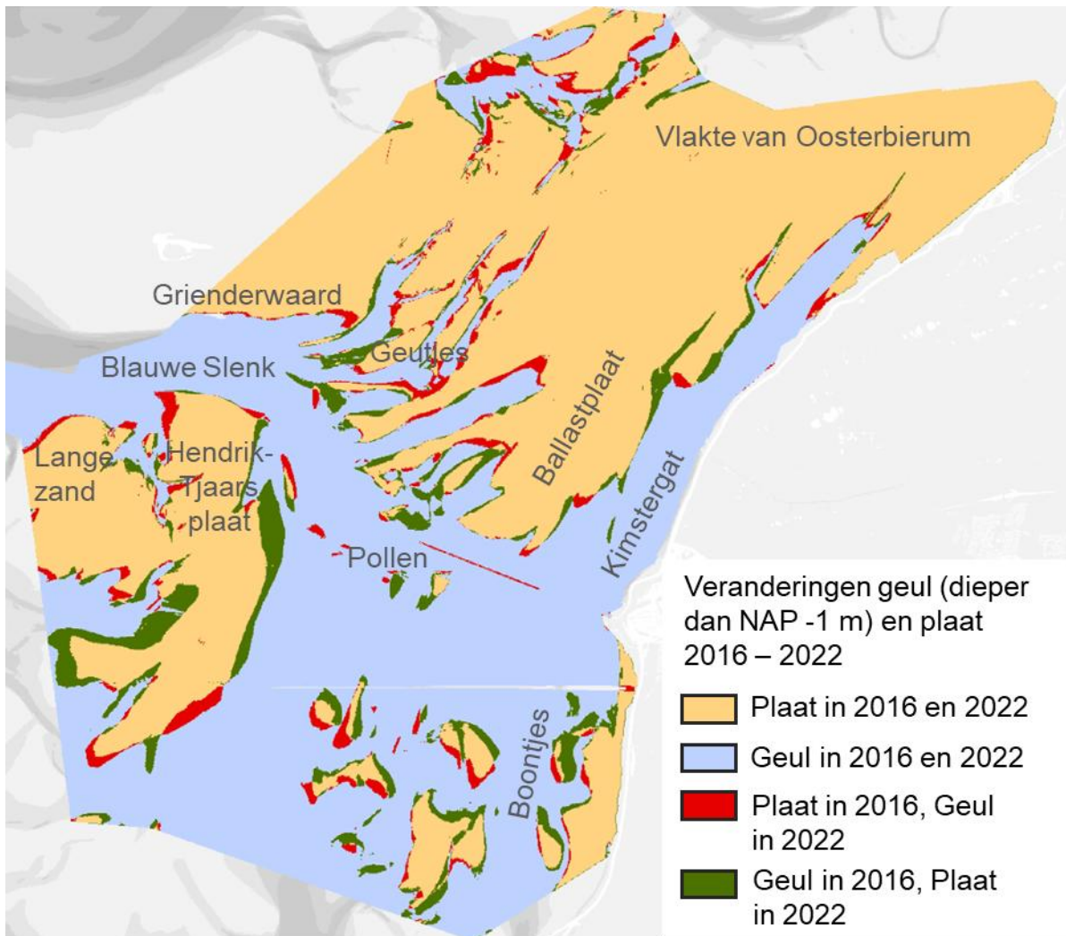
Figuur 5-4 Kaart met de stabiliteit van de wadplaten (delen hoger dan NAP -1 m) van het studiegebied (het gebied met de heldere kleuren).
