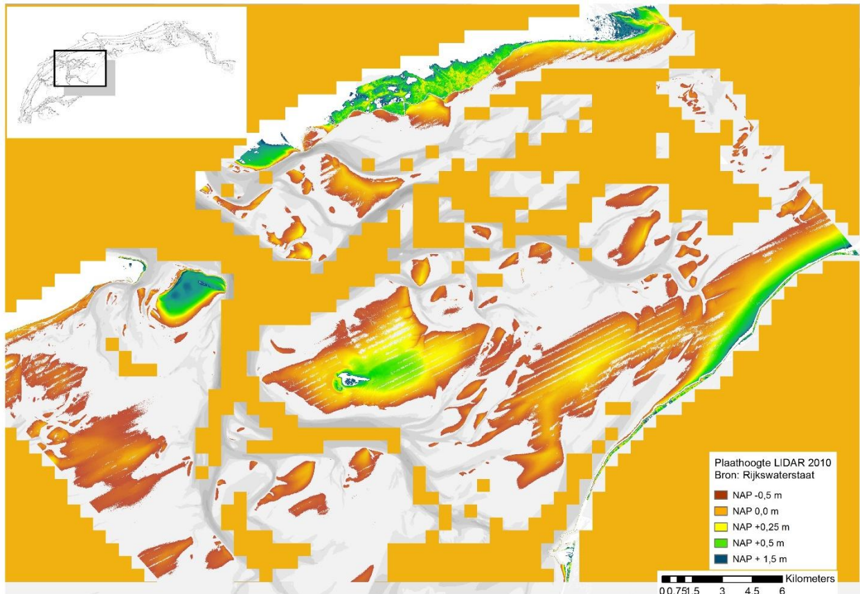
Figuur 9-2 Overzichtskartaal van het kombergingsgebied van het Vlie, met de LiDAR opname van 2010.
