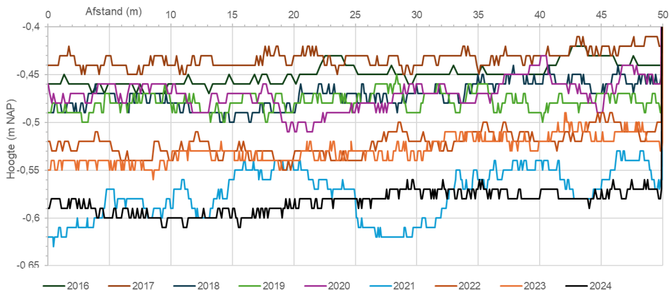
Figuur 6-8 Raaimetingen over afstand van 50 m rond het middelpunt ter hoogte van BP90 (projectie op de raailijn).
