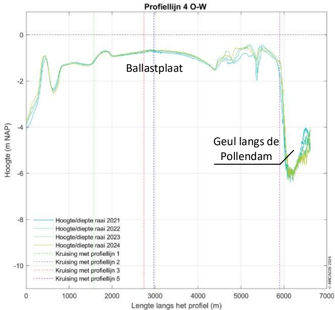
Figuur 4-10 Dwarsprofiel langs profiellijn 4 van noord naar zuid voor de hoogte/diepte raai meetgegevens van 2016 - 2024.
