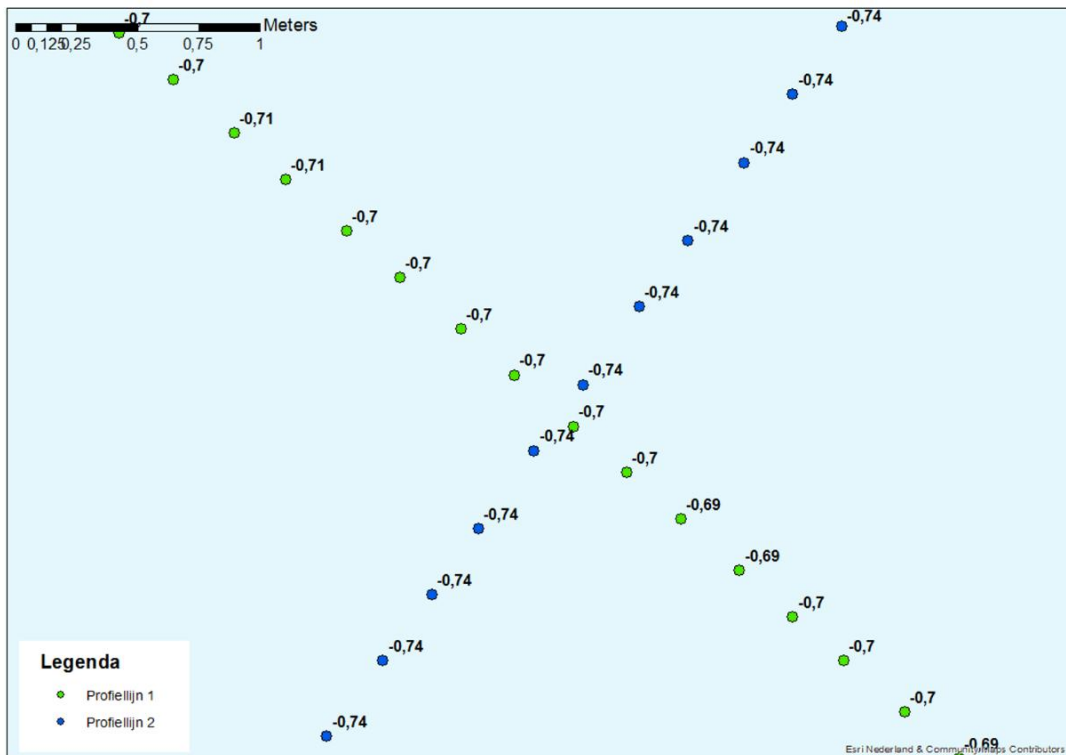
Figuur 9-30 Detailkaart controlepunt tussen profiellijn 1 en profiellijn 2 voor de hoogte/diepte raaien 2016, hoogtemetingen zijn weergegeven in m NAP.
