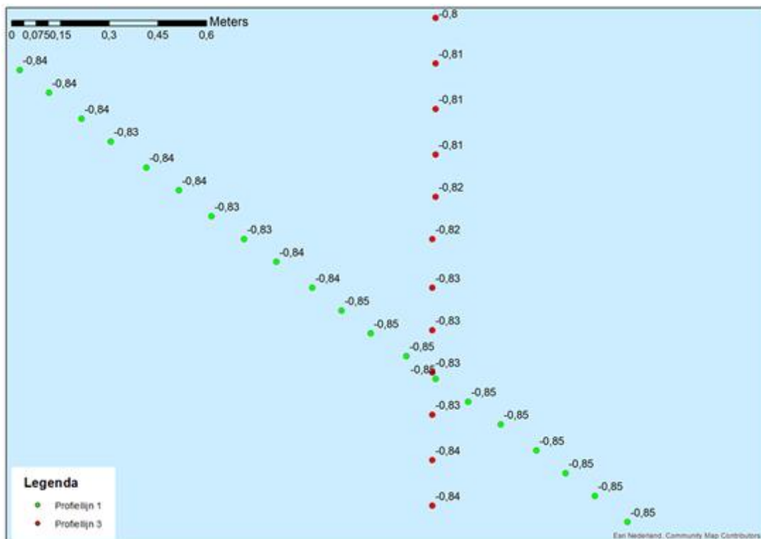
Figuur 9-61 Detailkaart controlepunt tussen profiel 1 en profiel 3 voor de hoogte/diepte raaien 2020, hoogtemetingen zijn weergegeven in m NAP.
