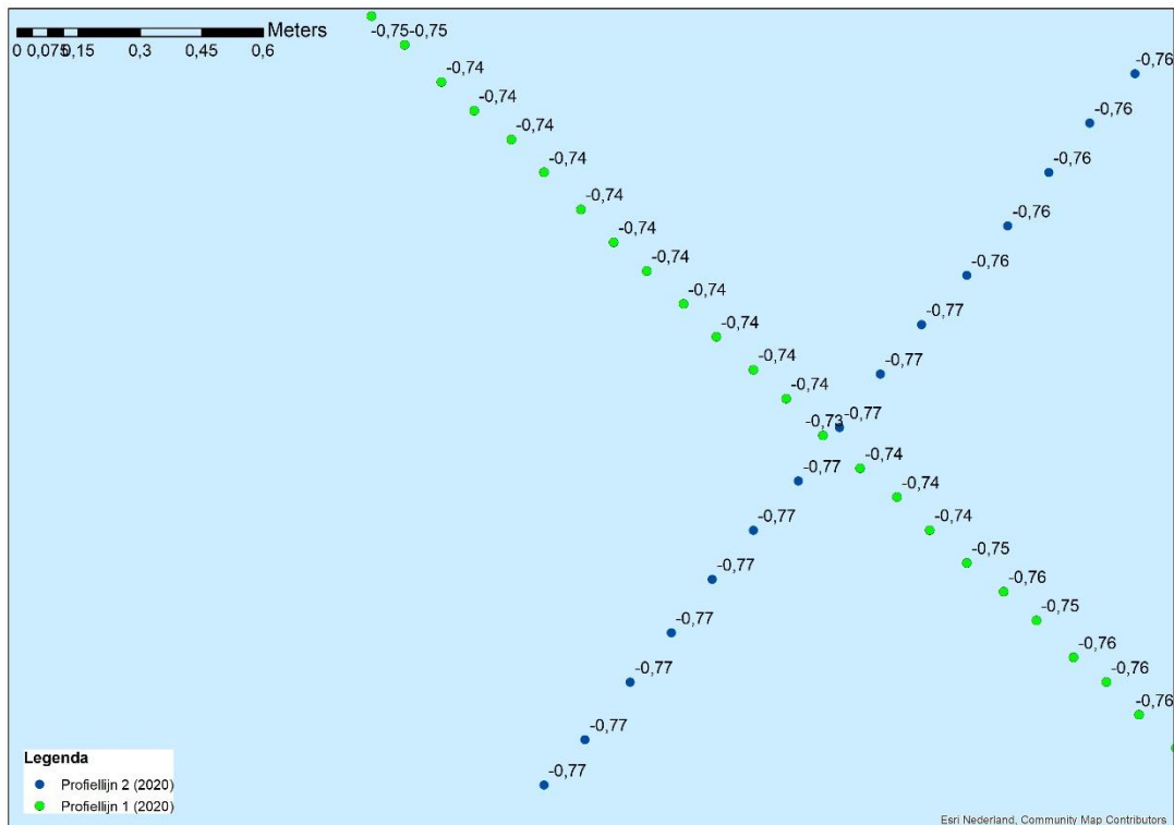
Figuur 9-54 Detailkaart controlepunt tussen profiellijn 1 en profiellijn 2 voor de hoogte/diepte raaien mei 2019, hoogtemetingen zijn weergegeven in m NAP.
