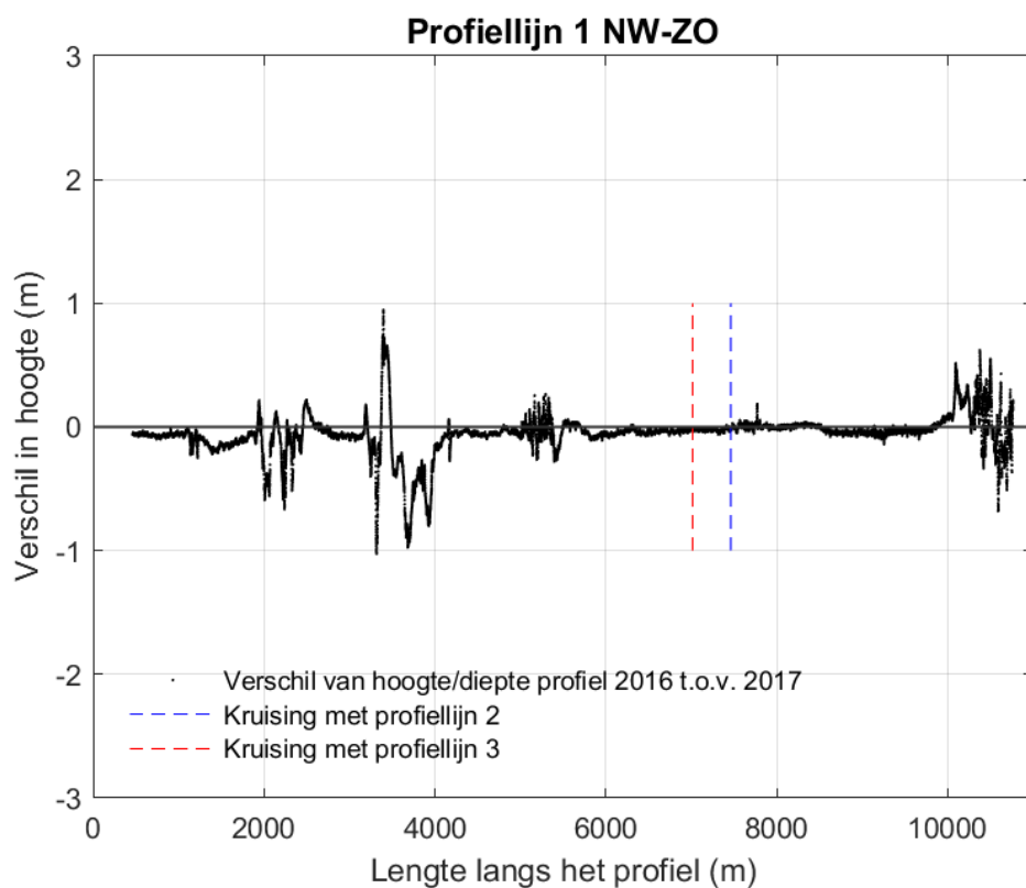
Figuur 9-120 Verschilplot langs profiellijn 1 van noordwest naar zuidoost voor de hoogte/diepte raai meetgegevens van 2016 en 2017. Een negatieve waarde betekent dat de hoogte/diepteraai van 2017 lager ligt dan de hoogte/diepteraai van 2016.
