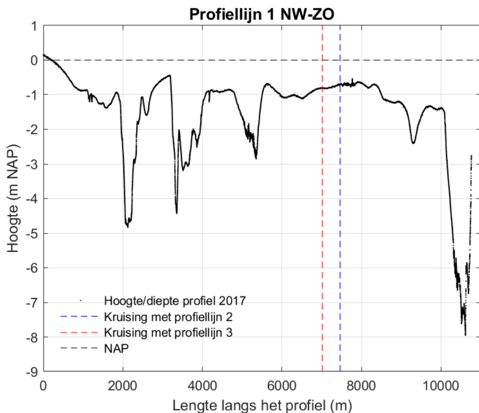
Figuur 9-33 Dwarsdoorsnede langs profiellijn 1 van noordwest naar zuidoost in 2017.
