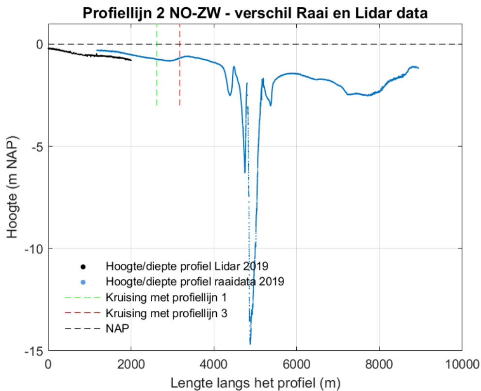
Figuur 9-18 Profiellijn 2 van noordoost naar zuidwest voor de hoogte/diepte raai meetgegevens van 2019 en de LiDAR-data van 2019.
