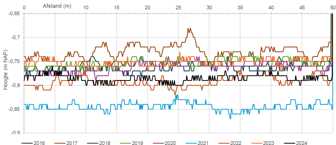
Figuur 6-4 Raaimetingen over afstand van 50 m rond het middelpunt ter hoogte van BP70 (projectie op de raailijn).
