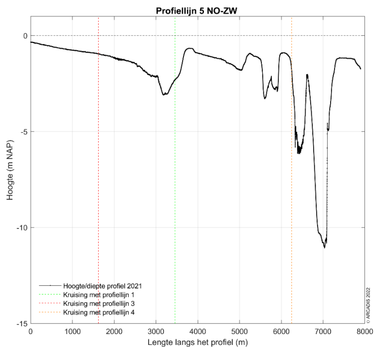
Figuur 9-67 Dwarsdoorsnede langs profiellijn 5 van noordoost naar zuidwest in 2021.
