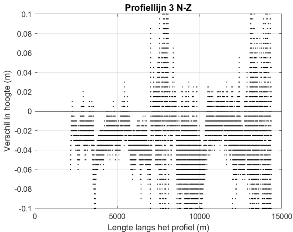
Figuur 9-154 Ingezoomde verschilplot langs profiellijn 3 van noord naar zuid voor de hoogte/diepte raai meetgegevens van januari 2019 en mei 2019. Een negatieve waarde betekent dat de hoogte/diepteraai van mei 2019 lager ligt dan de hoogte/diepteraai van januari 2019.
