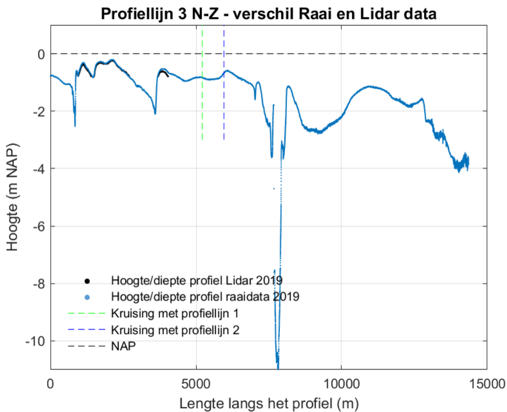
Figuur 9-21 Profiellijn 3 van noord naar zuid voor de hoogte/diepte raai meetgegevens van 2019 en de LiDAR-data van 2019.
