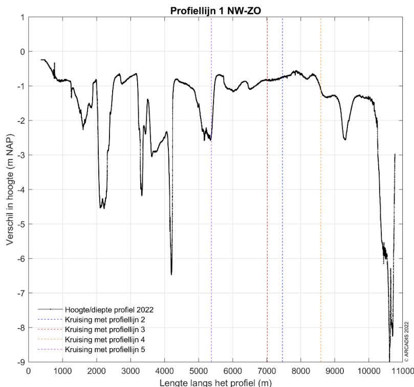
Figuur 9-77 Dwarsdoorsnede langs profiellijn 1 van noordwest naar zuidoost in 2022.
