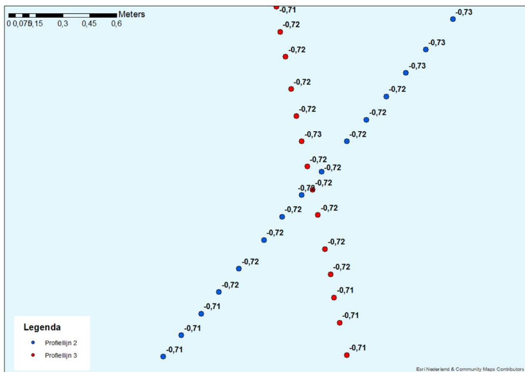
Figuur 9-38 Detailkaart controlepunt tussen profiellijn 2 en profiellijn 3 voor de hoogte/diepte raaien 2017, hoogtemetingen zijn weergegeven in m NAP.
