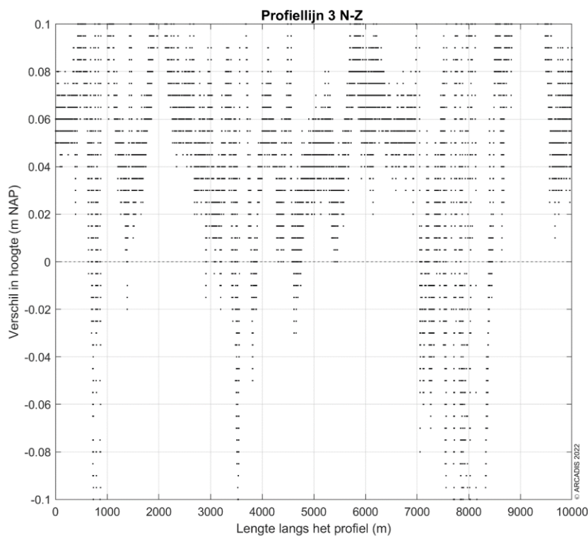
Figuur 9-181: Ingezoomde vershilplot langs profielijn 3 van noord naar zuid voor de hoogte/diepte raai meetgegevens van 2021 en 2022. Een positieve waarde betekent dat de hoogte/diepteraai van 2022 hoger ligt dan de hoogte/diepteraai van 2021.
