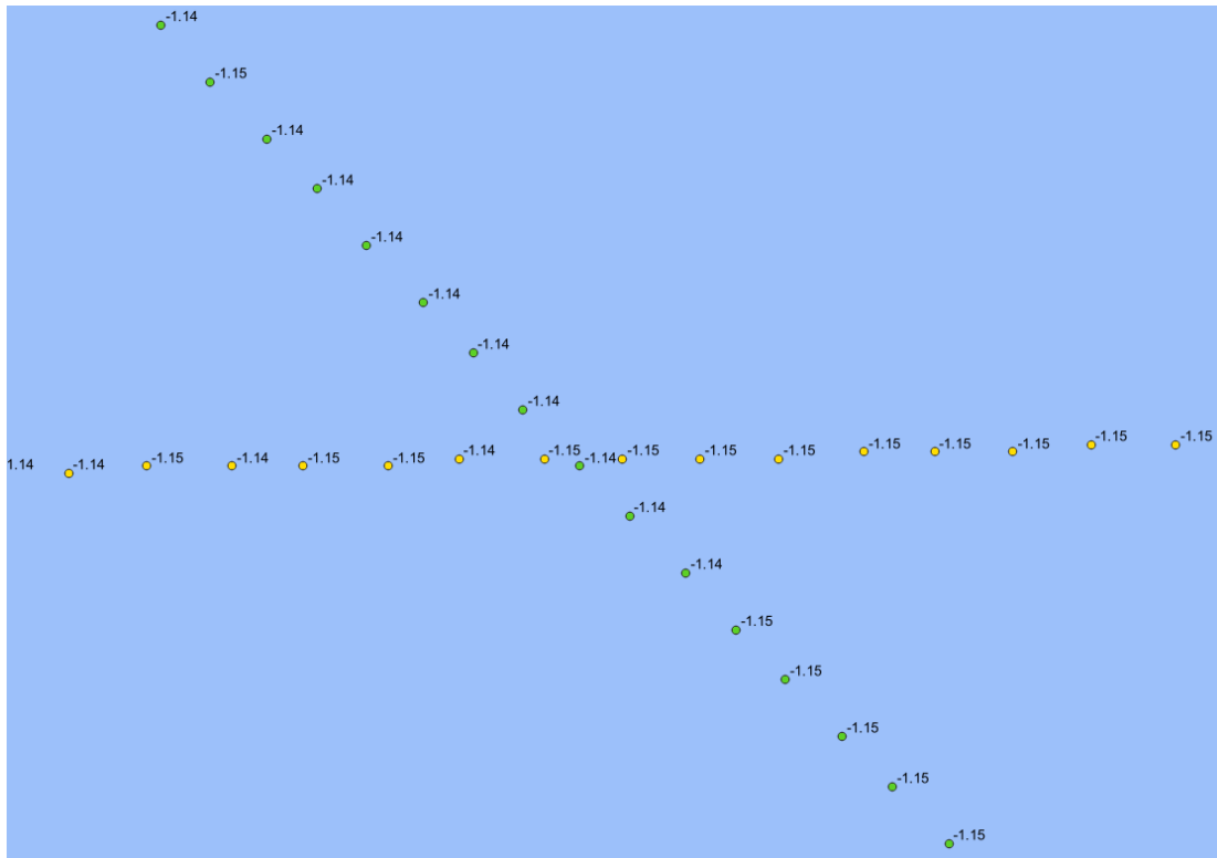
Figuur 9-98 Detailkaart controlepunt tussen profiellijn 1 en profiellijn 4 voor de hoogte/diepte raaien 2023, hoogtemetingen zijn weergegeven in m NAP.
