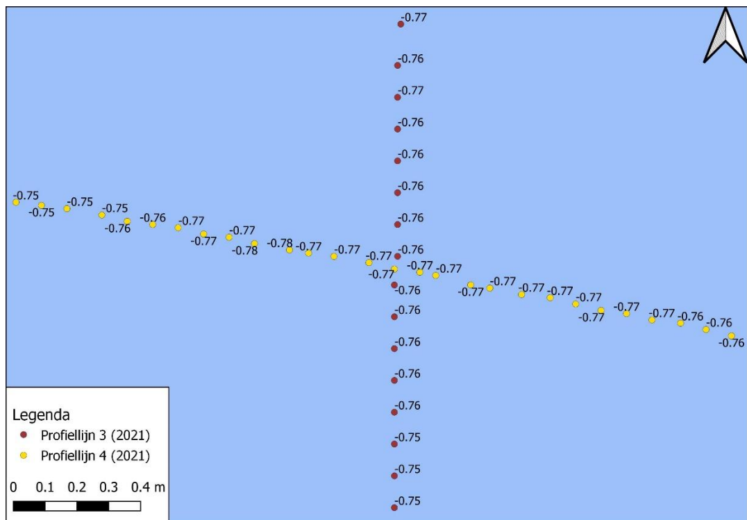
Figuur 9-74 Detailkaart controlepunt tussen profiellijn 3 en profiellijn 4 voor de hoogte/diepte raaien mei 2021, hoogtemetingen zijn weergegeven in m NAP.
