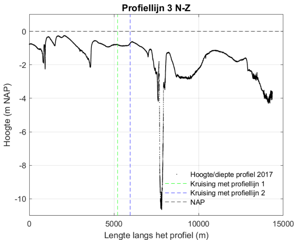
Figuur 9-35 Dwarsdoorsnede langs profiellijn 3 van noord naar zuid in 2017.
