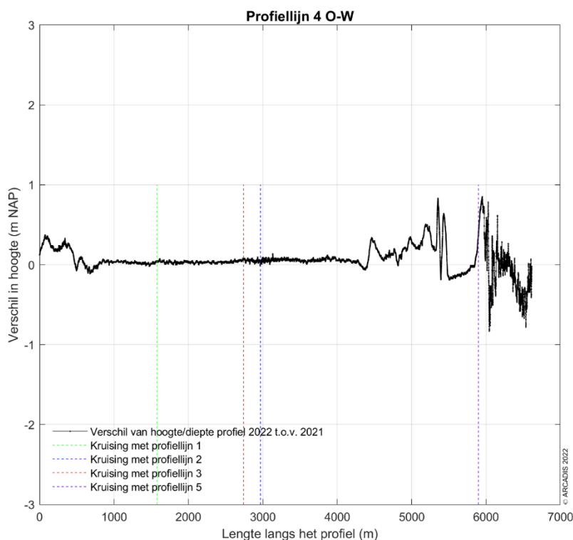
Figuur 9-183 Verschilplot langs profiellijn 4 van oost naar west voor de hoogte/diepte raai meetgegevens van 2021 en 2022. Een positieve waarde betekent dat de hoogte/diepteraai van mei 2022 hoger ligt dan de hoogte/diepteraai van 2021.
