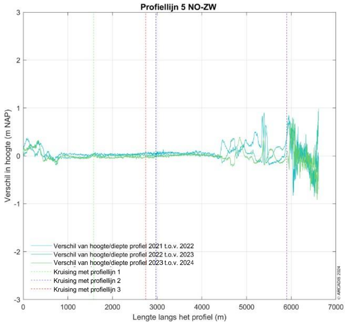
Figuur 4-12 Vershilplot langs profiellijn 4 van noord naar zuid voor de hoogte/diepte raai meetgegevens tussen 2021-2024. Een positieve waarde betekent dat de hoogte/diepteraai van het opvolgende jaar hoger ligt dan de hoogte/diepteraai van het eerdere jaar.
