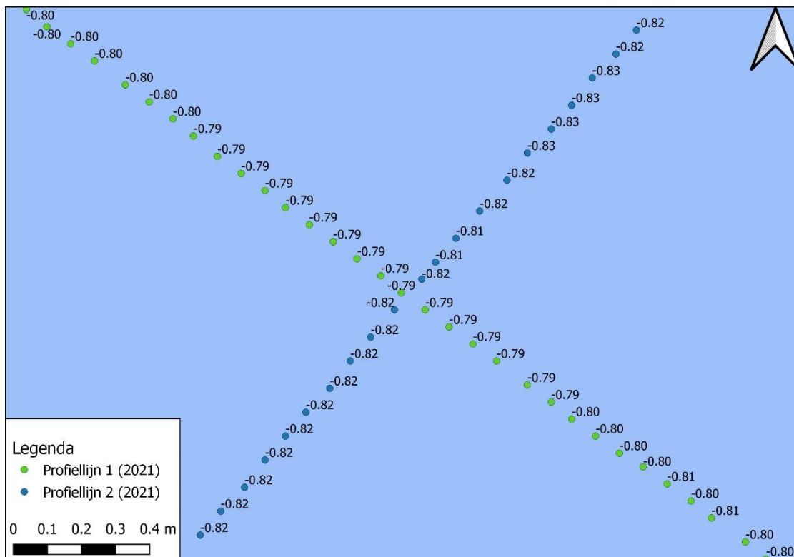
Figuur 9-68 Detailkaart controlepunt tussen profiellijn 1 en profiellijn 2 voor de hoogte/diepte raaien 2021, hoogtemetingen zijn weergegeven in m NAP.
