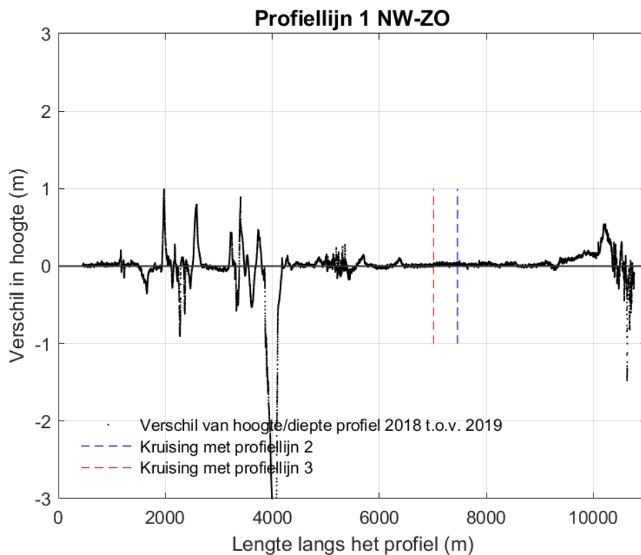
Figuur 9-138 Verschilplot langs profiellijn 1 van noordwest naar zuidoost voor de hoogte/diepte raai meetgegevens van 2018 en mei 2019. Een positieve waarde betekent dat de hoogte/diepteraai van mei 2019 hoger ligt dan de hoogte/diepteraai van 2018.
