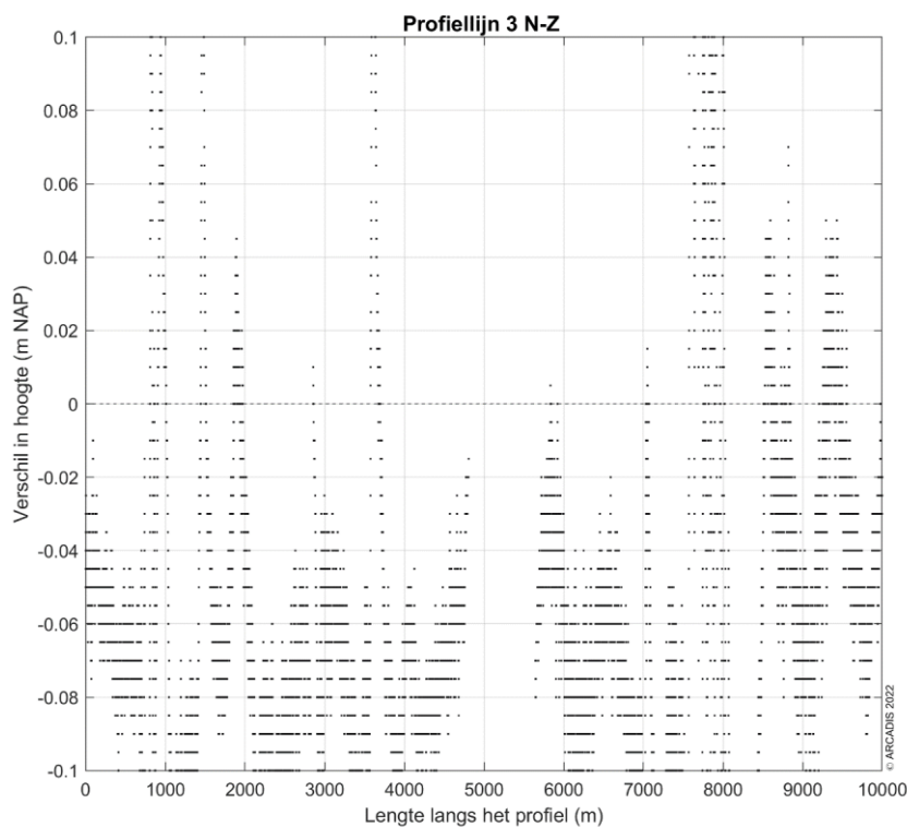
Figuur 9-172: Ingezoomde verskilplot langs profiellijn 3 van noord naar zuid voor de hoogte/diepte raai meetgegevens van 2020 en 2021. Een positieve waarde betekent dat de hoogte/diepteraai van 2021 hoger ligt dan de hoogte/diepteraai van 2020.
