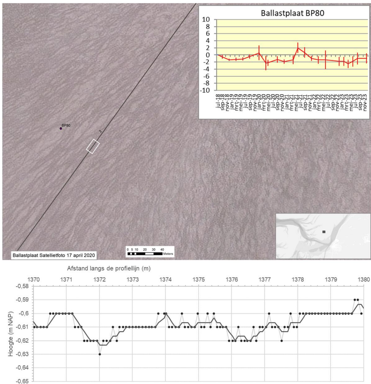
Figuur 9-209 Luchtfoto (17 april 2020) met de locatie van spijkermeting BP80 en raai 2, met daarbij rechtsboven de grafiek met de resultaten van de spijkermetingen bij BP80 en onder de dwarsdoorsnede van raai 2 van de raaimeting uit 2023.
