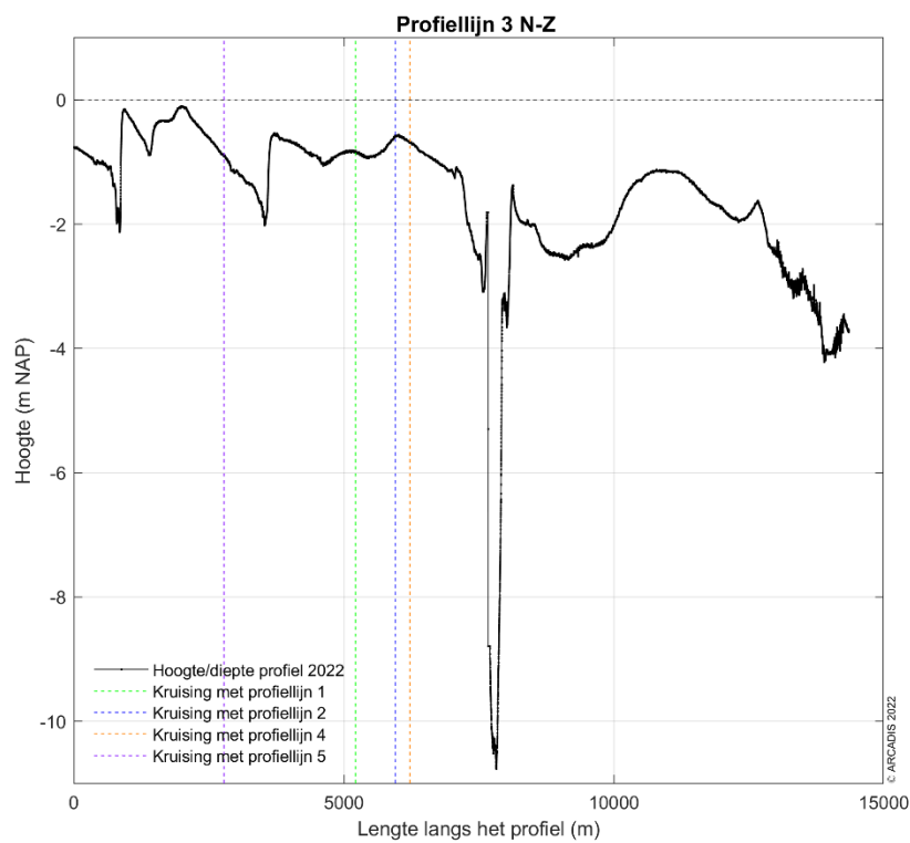
Figuur 9-79 Dwarsdoorsnede langs profiellijn 3 van noord naar zuid in 2022.
