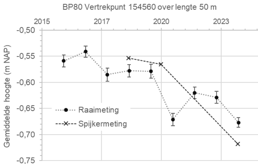
Figuur 6-7 Hoogte van de raaimetingen en de Spijkermetingen bij BP80.
