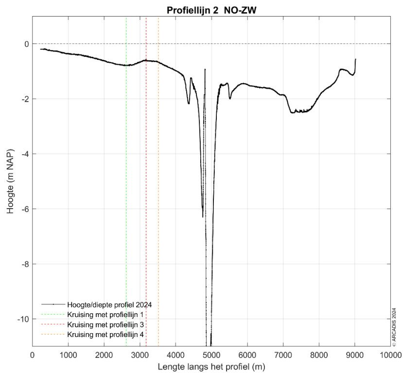
Figuur 9-106 Dwarsdoorsnede langs profiellijn 2 van noordoost naar zuidwest in 2024.
