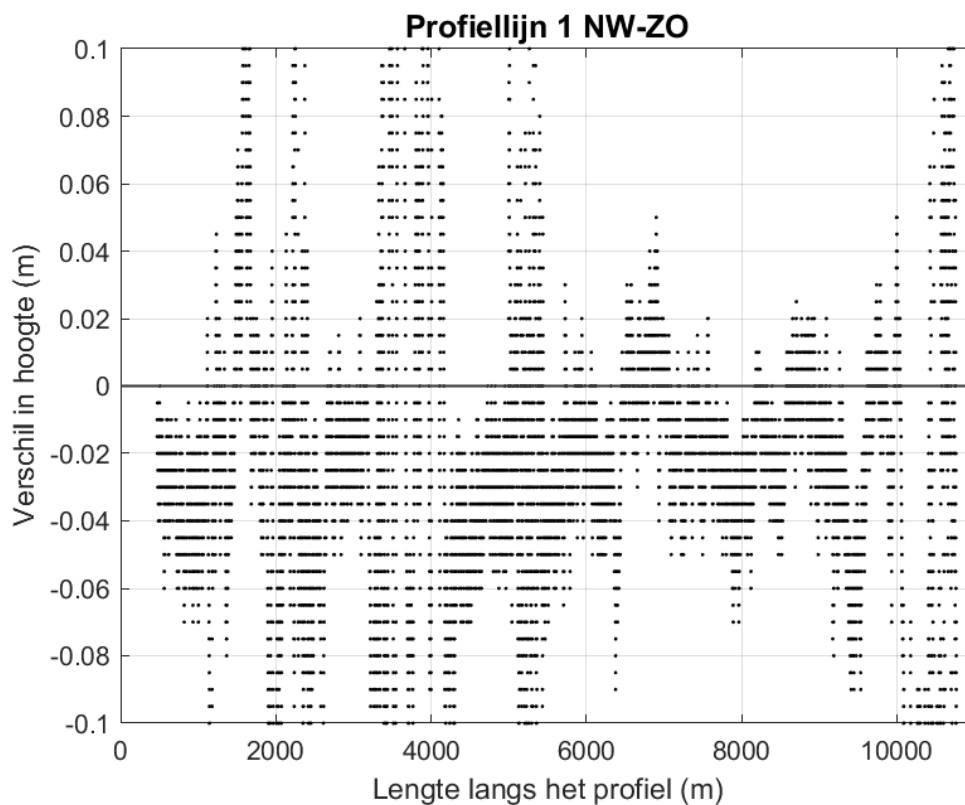
Figuur 9-148 Ingezoomde verschilplot langs profiellijn 1 van noordwest naar zuidoost voor de hoogte/diepte raai meetgegevens van januari 2019 en mei 2019. Een negatieve waarde betekent dat de hoogte/diepteraai van mei 2019 lager ligt dan de hoogte/diepteraai van januari 2019.
