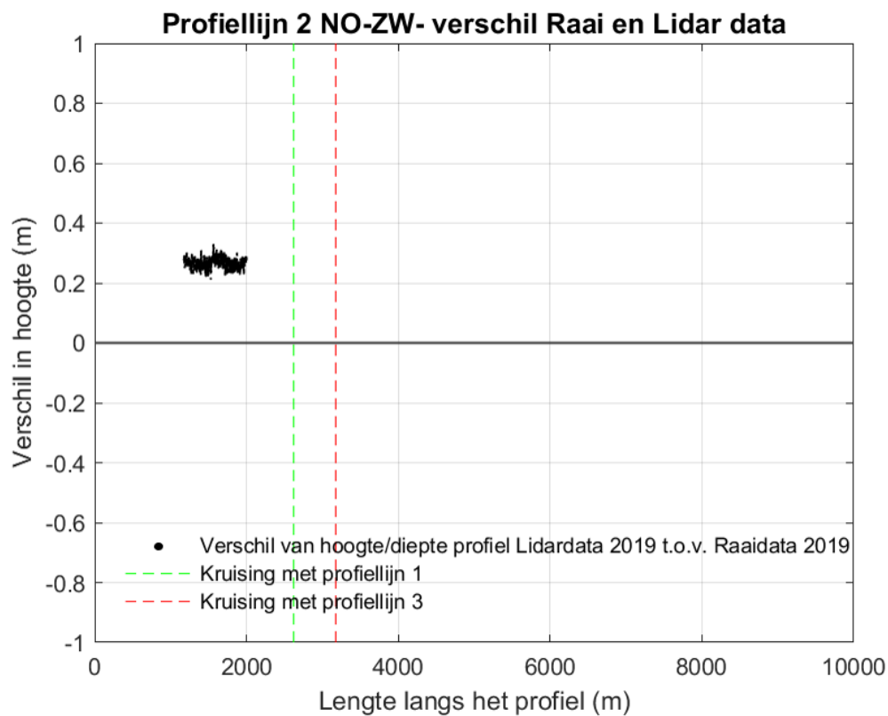
Figuur 9-19 Verskilplot langs profiellijn 2 van noordoost naar zuidwest voor de hoogte/diepte raai meetgegevens van 2019 en de LiDAR-data van 2019. Een positieve waarde betekent dat de LiDAR lager ligt dan de hoogte/diepteraai.
