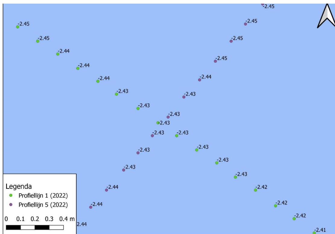
Figuur 9-85 Detailkaart controlepunt tussen profiellijn 1 en profiellijn 5 voor de hoogte/diepte raaien 2022, hoogtemetingen zijn weergegeven in m NAP.
