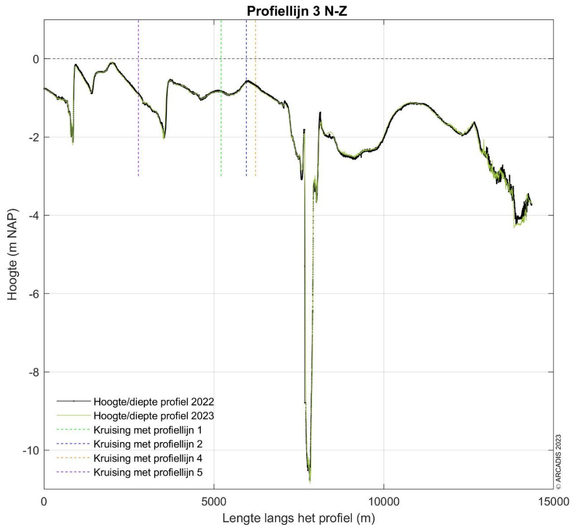
Figuur 9-194 Dwarsprofiel langs profiellijn 3 van noord naar zuid voor de hoogte/diepte raai meetgegevens van 2022 en 2023.
