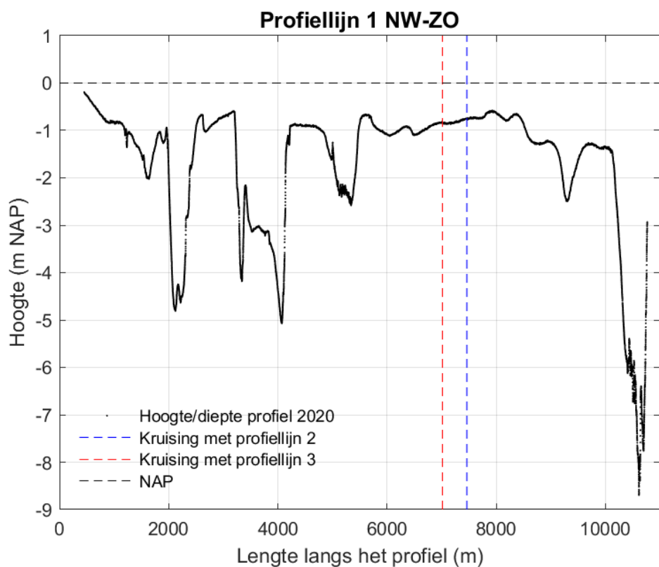
Figuur 9-57 Dwarsdoorsnede langs profiel 1 van noordwest naar zuidoost in 2020.
