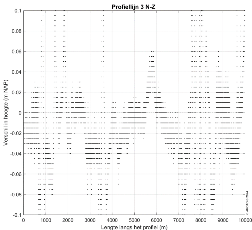
Figuur 3-12: Ingezoomde verschilplot langs profiellijn 3 van noord naar zuid voor de hoogte/diepte raai meetgegevens van 2023 en 2024. Een positieve waarde betekent dat de hoogte/diepteraai van 2024 hoger ligt dan de hoogte/diepteraai van 2023.
