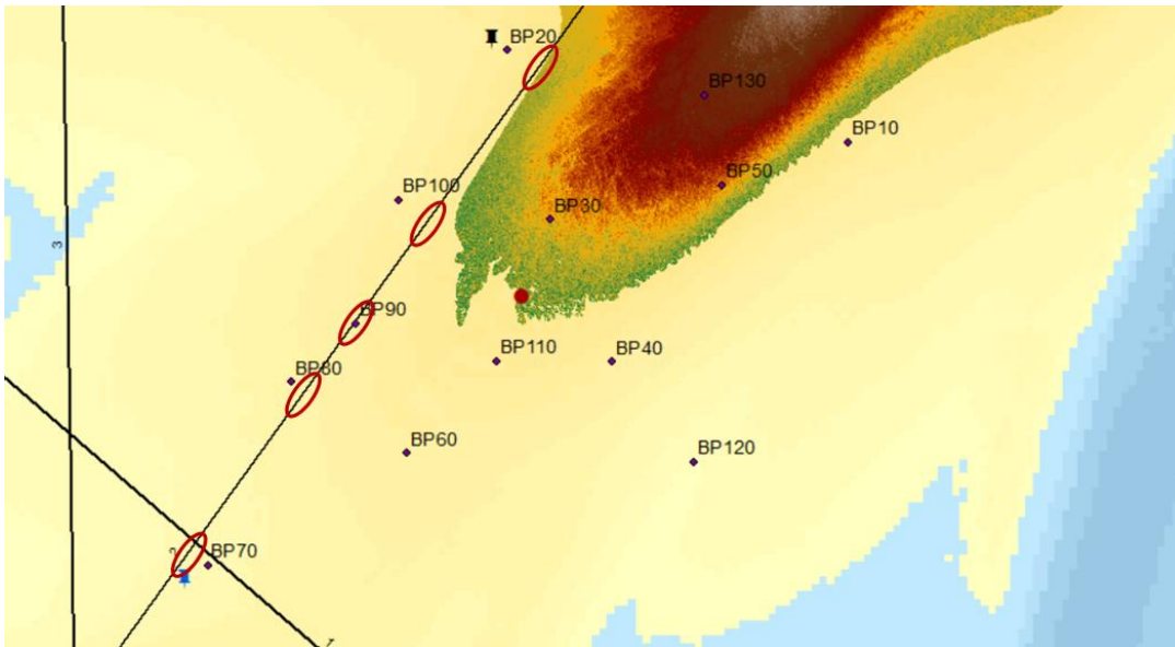
Figuur 6-2 Locaties van de Raaimetingen en de Spijkermetingen.
