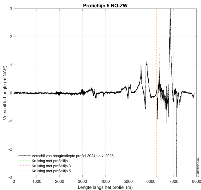
Figuur 3-17 Verschilplot langs profiellijn 5 van noordoost naar zuidwest voor de hoogte/diepte raai meetgegevens van 2023 en 2024. Een positieve waarde betekent dat de hoogte/diepteraai van 2024 hoger ligt dan de hoogte/diepteraai van 2023.
