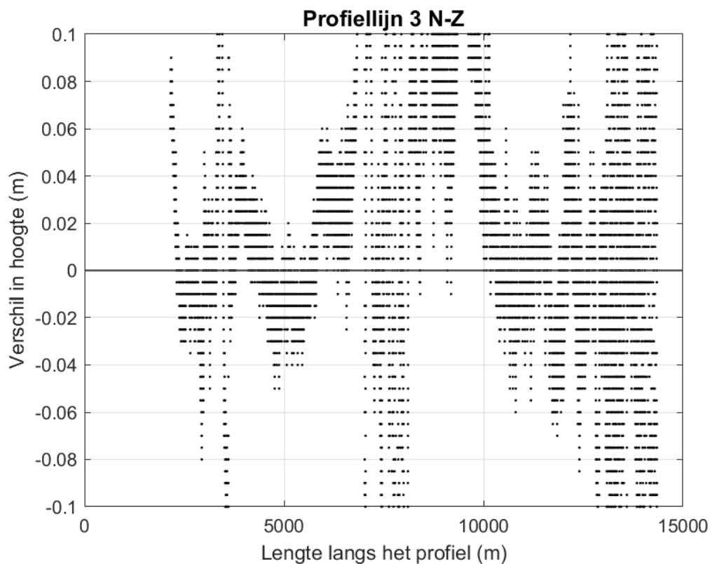
Figuur 9-145 Ingezoomde verschilplot langs profiellijn 3 van noord naar zuid voor de hoogte/diepte raai meetgegevens van 2018 en mei 2019. Een positieve waarde betekent dat de hoogte/diepteraai van mei 2019 hoger ligt dan de hoogte/diepteraai van 2018.
