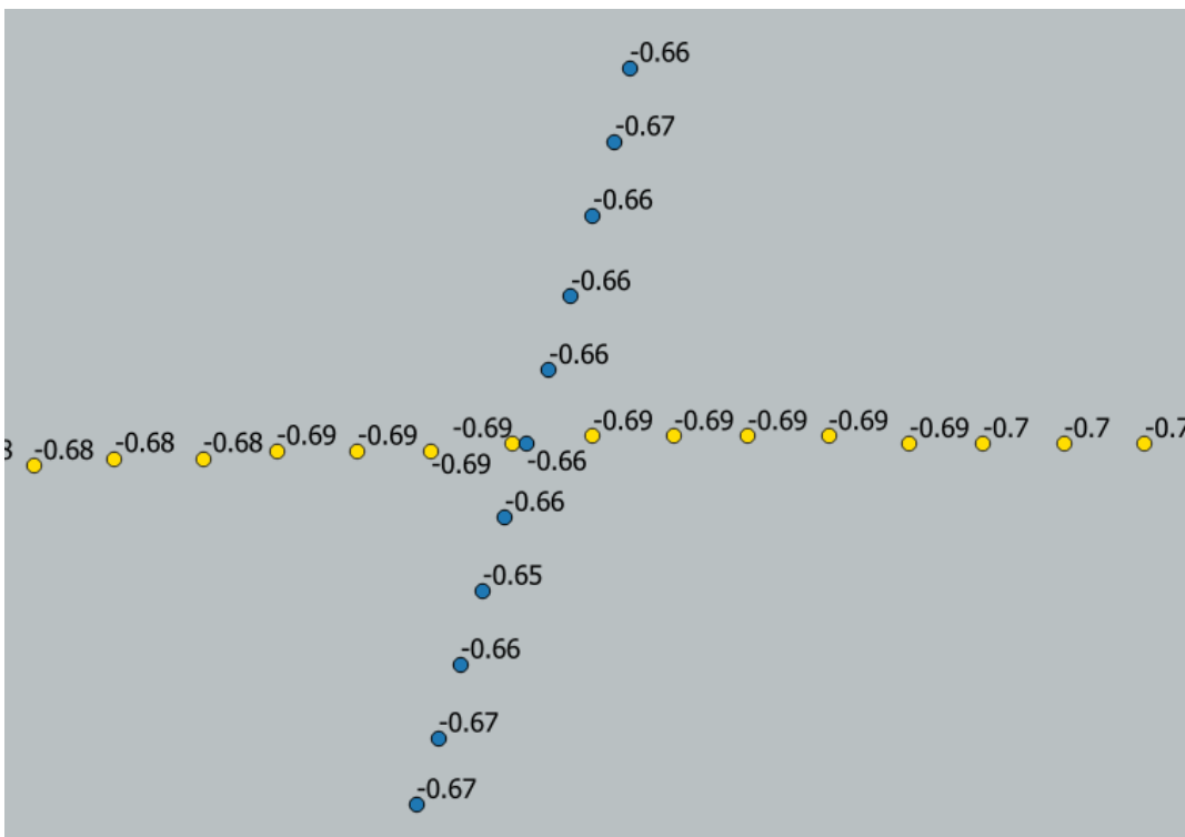
Figuur 9-115 Detailkaart controlepunt tussen profiellijn 2 en profiellijn 4 voor de hoogte/diepte raaien mei 2024, hoogtemetingen zijn weergegeven in m NAP.
