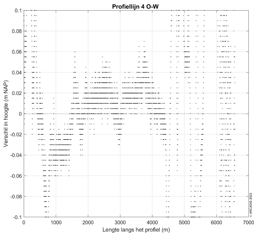
Figuur 9-199: Ingezoomde verschilplot langs profiellijn 4 van oost naar west voor de hoogte/diepte raai meetgegevens van 2022 en 2023. Een positieve waarde betekent dat de hoogte/diepteraai van 2023 hoger ligt dan de hoogte/diepteraai van 2022.
