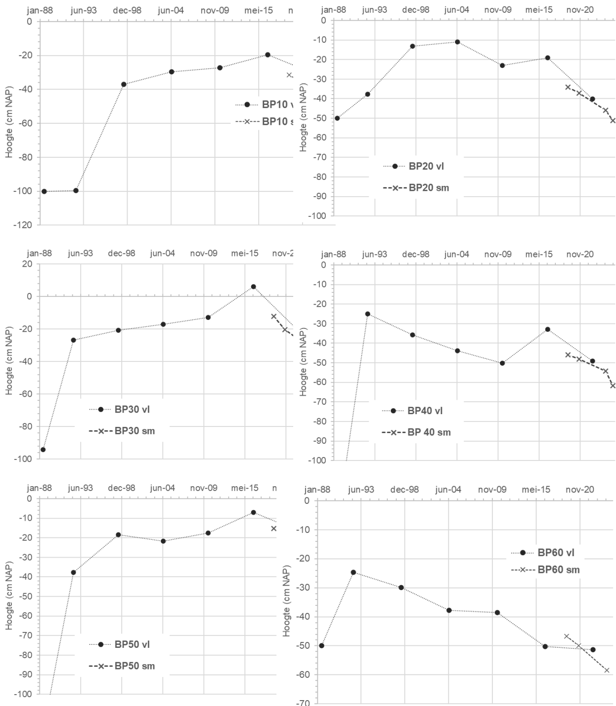
Figuur 6-14 Hoogte ter plaatse van de Spijkermetingen op basis de vaklodingen (vl) en de hoogtemetingen van de locaties van de Spijkermetingen (sm) van de meetpunten op de Ballastplaat Zuid. Vervolg op de volgende pagina.
