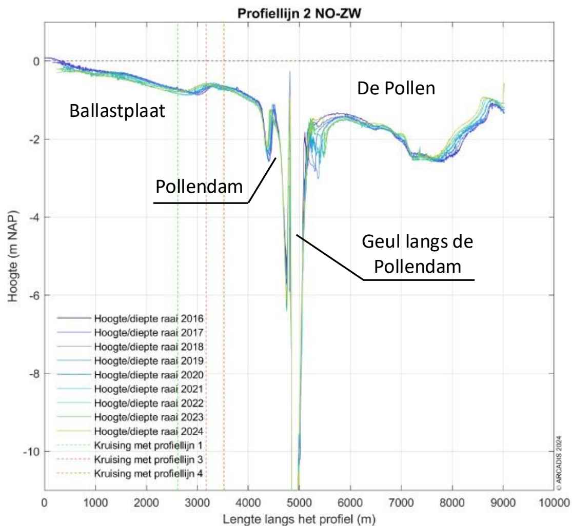
Figuur 4-4 Dwarsprofiel langs profiellijn 2 van noordoost naar zuidwest voor de hoogte/diepte raai meetgegevens van 2016 - 2024.
