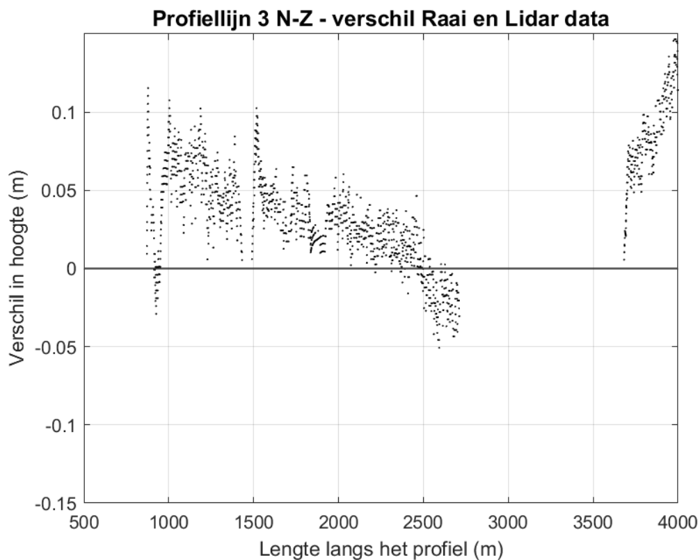
Figuur 9-23 Ingezoomde verschilplot langs profiellijn 3 van noord naar zuid voor de hoogte/diepte raai meetgegevens van 2019 en de LiDAR-data van 2019. Een positieve waarde betekent dat de LiDAR lager ligt dan de hoogte/diepteraai.
