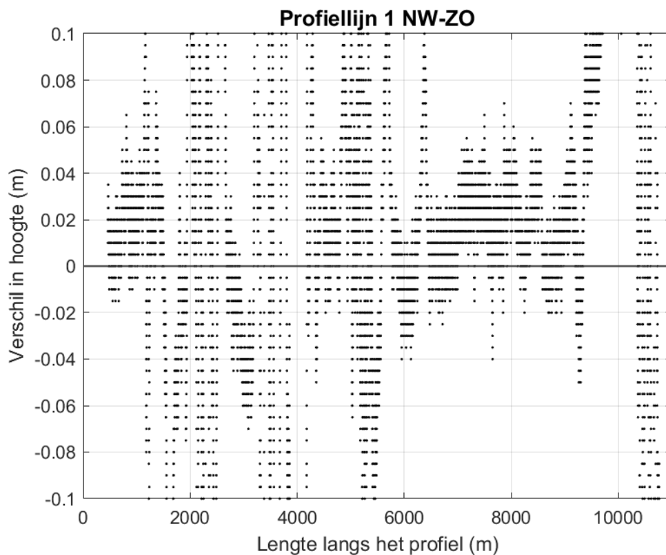
Figuur 9-139 Ingezoomde verschilplot langs profiellijn 1 van noordwest naar zuidoost voor de hoogte/diepte raai meetgegevens van 2018 en mei 2019. Een positieve waarde betekent dat de hoogte/diepteraai van mei 2019 hoger ligt dan de hoogte/diepteraai van 2018.
