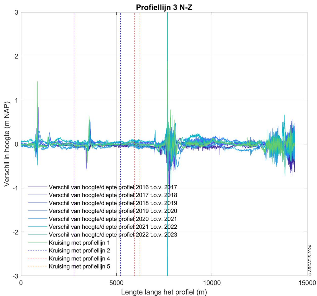
Figuur 4-9 Verschilplot langs profiellijn 3 van noord naar zuid voor de hoogte/diepte raai meetgegevens tussen 2016-2024. Een positieve waarde betekent dat de hoogte/diepteraai van het opvolgende jaar hoger ligt dan de hoogte/diepteraai van het eerdere jaar.
