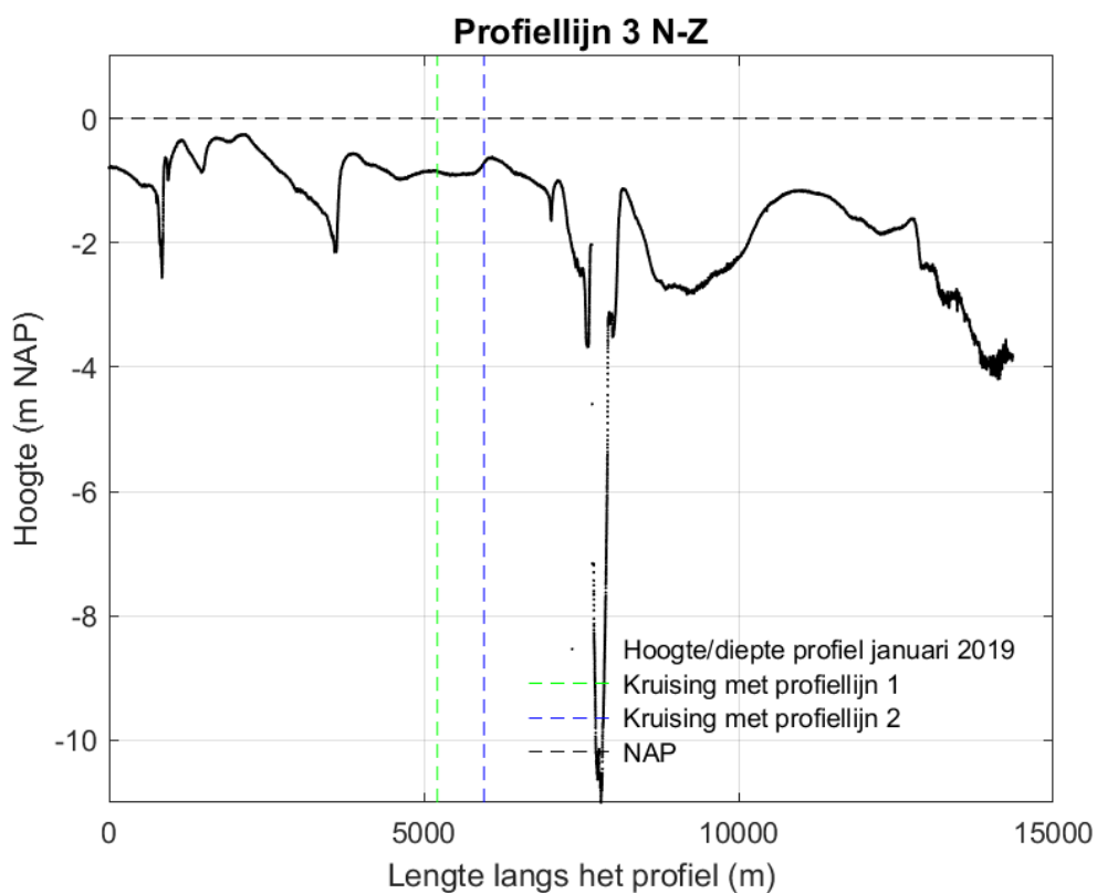
Figuur 9-47 Dwarsdoorsnede langs profiellijn 3 van noord naar zuid in januari 2019.
