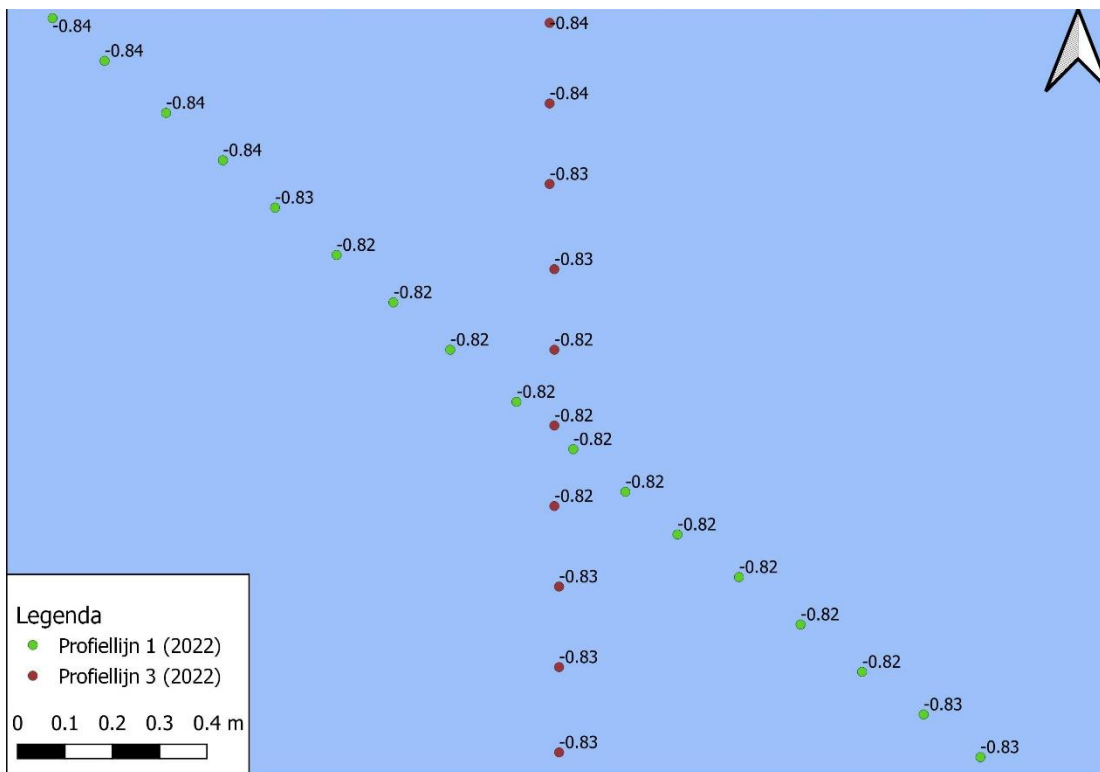
Figuur 9-83 Detailkaart controlepunt tussen profiellijn 1 en profiellijn 3 voor de hoogte/diepte raaien 2022, hoogtemetingen zijn weergegeven in m NAP.
