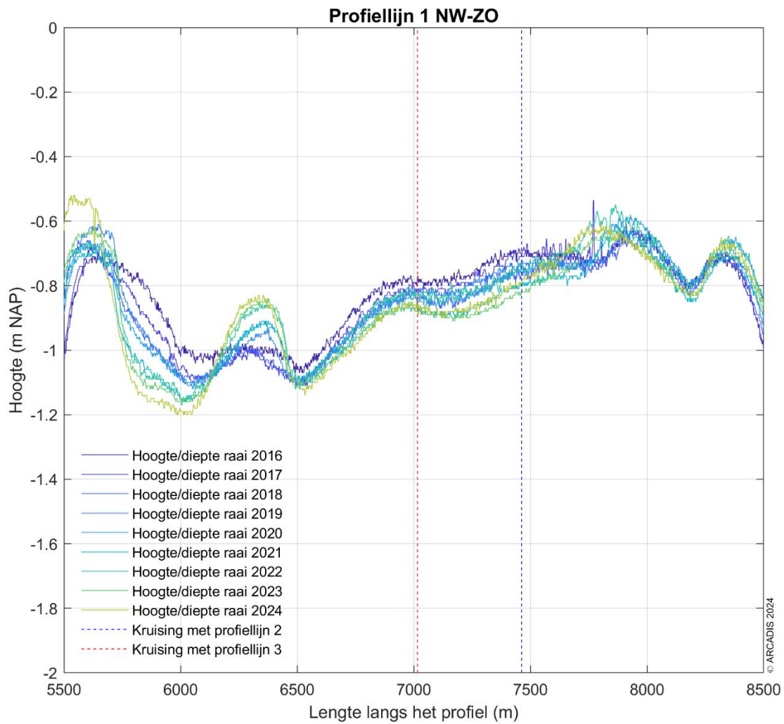
Figuur 4-2 Ingezoomd dwarsprofiel van de Ballastplaat langs profiellijn 2 van noordwest naar zuidoost voor de hoogte/diepte raai meetgegevens van 2016 -2024 (Detail van Figuur 4-1).
