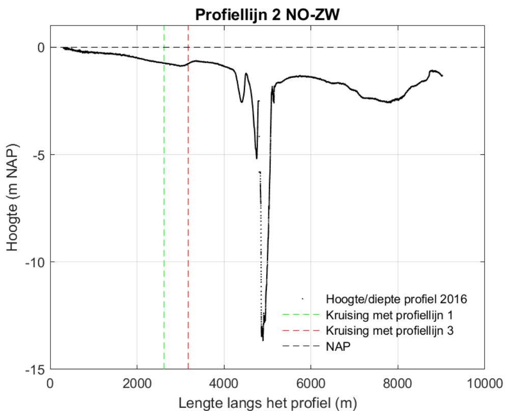
Figuur 9-28 Dwarsdoorsnede langs profiellijn 2 van noordoost naar zuidwest in 2016.
