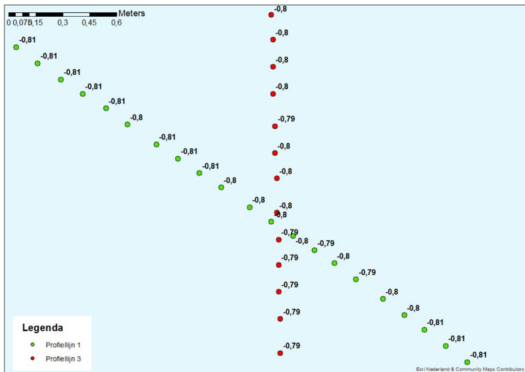
Figuur 9-37 Detailkaart controlepunt tussen profiellijn 1 en profiellijn 3 voor de hoogte/diepte raaien 2017, hoogtemetingen zijn weergegeven in m NAP.
