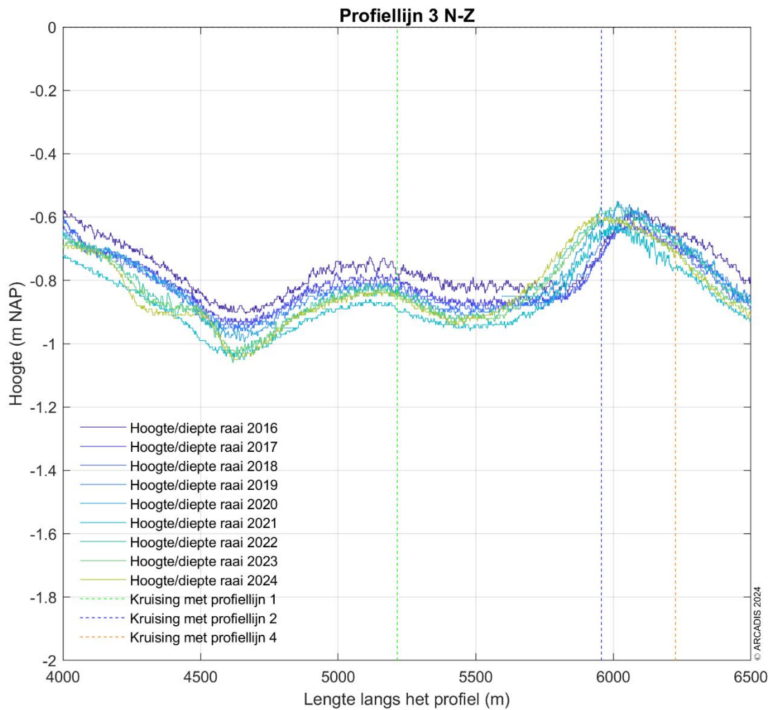
Figuur 4-8 Ingezoomd dwarsprofiel van de Ballastplaat langs profiellijn 3 van noord naar zuid voor de hoogte/diepte raai meetgegevens van 2016 - 2024 (Detail van Figuur 4-7).
