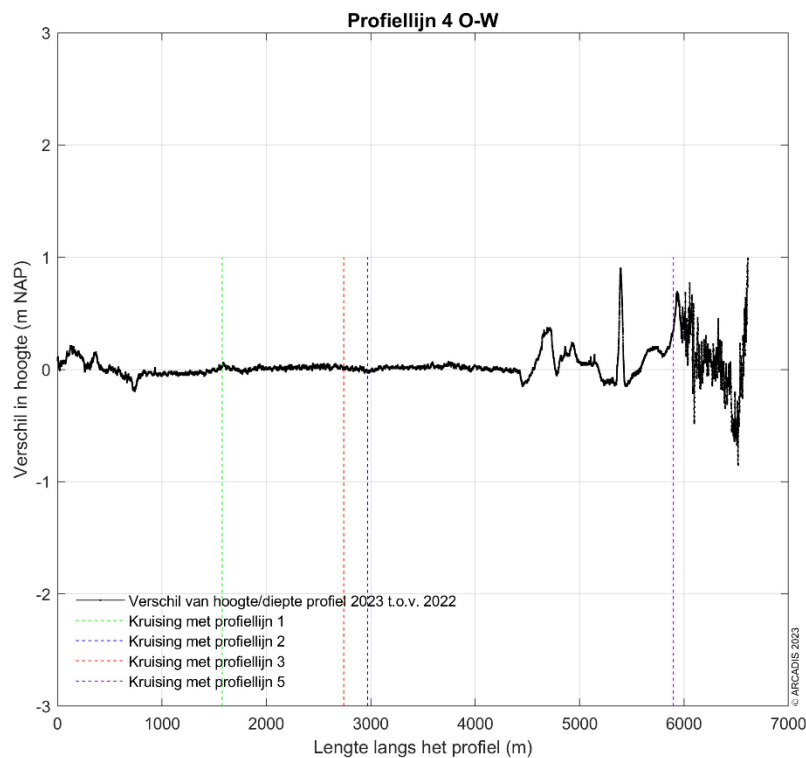
Figuur 9-198 Verschilplot langs profiellijn 4 van oost naar west voor de hoogte/diepte raai meetgegevens van 2022 en 2023. Een positieve waarde betekent dat de hoogte/diepteraai van mei 2023 hoger ligt dan de hoogte/diepteraai van 2022.
