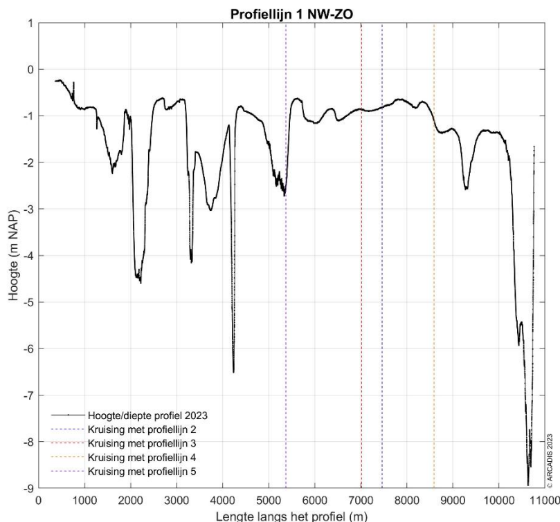
Figuur 9-91 Dwarsdoorsnede langs profiellijn 1 van noordwest naar zuidoost in 2023.
