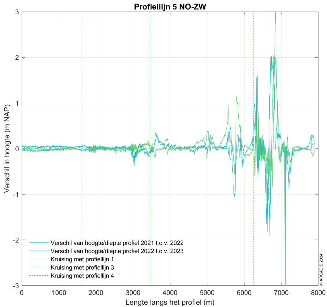
Figuur 4-15 Vershilplot langs profiellijn 5 van noord naar zuid voor de hoogte/diepte raai meetgegevens tussen 2021-2024. Een positieve waarde betekent dat de hoogte/diepteraai van het opvolgende jaar hoger ligt dan de hoogte/diepteraai van het eerdere jaar.
