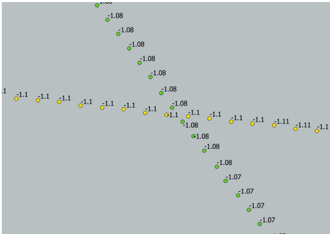
Figuur 9-112 Detailkaart controlepunt tussen profiellijn 1 en profiellijn 4 voor de hoogte/diepte raaien 2024, hoogtemetingen zijn weergegeven in m NAP.
