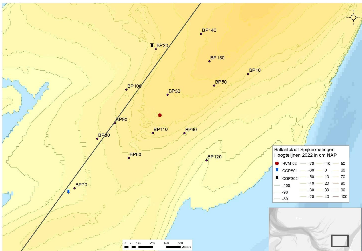
Figuur 9-205 Kaart met de ligging van de spijkermetingen ten opzichte van de raaimetingen in profiellijn 2.
