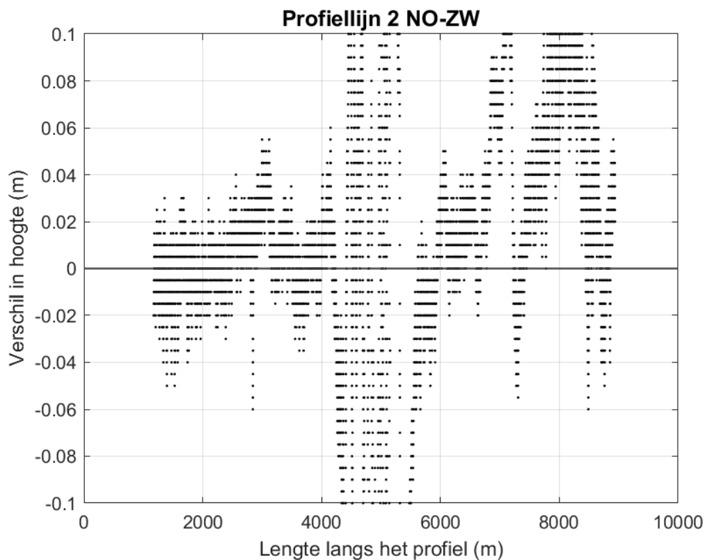
Figuur 9-142 Ingezoomde verschilplot langs profiellijn 2 van noordoost naar zuidwest voor de hoogte/diepte raai meetgegevens van 2018 en mei 2019. Een positieve waarde betekent dat de hoogte/diepteraai van mei 2019 hoger ligt dan de hoogte/diepteraai van 2018.
