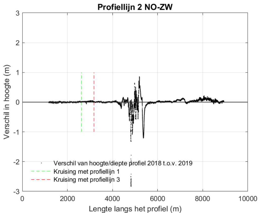
Figuur 9-141 Verschilplot langs profiellijn 2 van noordoost naar zuidwest voor de hoogte/diepte raai meetgegevens van 2018 en mei 2019. Een positieve waarde betekent dat de hoogte/diepteraai van mei 2019 hoger ligt dan de hoogte/diepteraai van 2018.
