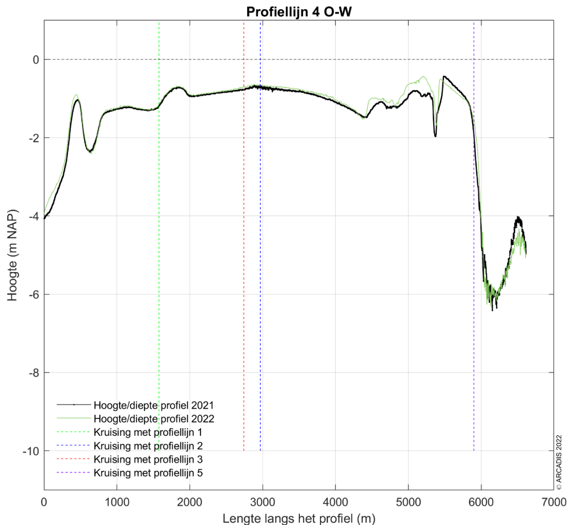
Figuur 9-182 Dwarsprofiel langs profiellijn 4 van oost naar west voor de hoogte/diepte raai meetgegevens van 2021 en 2022.
