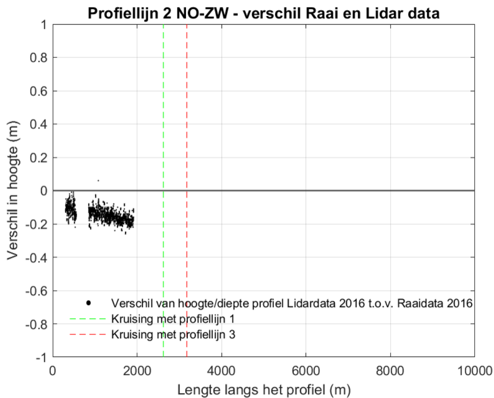
Figuur 9-10 Verschilplot langs profiellijn 2 van noordoost naar zuidwest voor de hoogte/diepte raai meetgegevens van 2016 en de LiDAR-data van 2016. Een positieve waarde betekent dat de LiDAR lager ligt dan de hoogte/diepteraai.
