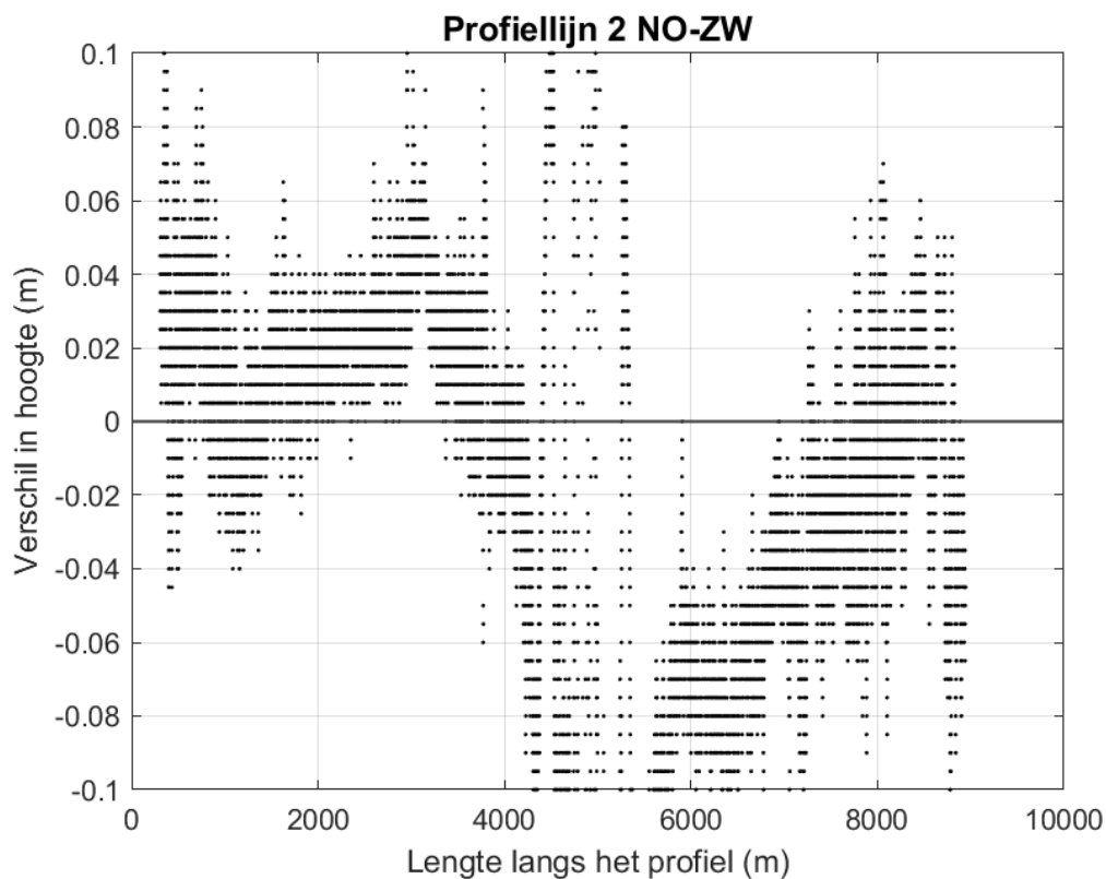
Figuur 9-124: Ingezoomde verschilplot langs profiellijn 2 van noordoost naar zuidwest voor de hoogte/diepte raai meetgegevens van 2016 en 2017. Een positieve waarde betekent dat de hoogte/diepteraai van 2017 hoger ligt dan de hoogte/diepteraai van 2016.
