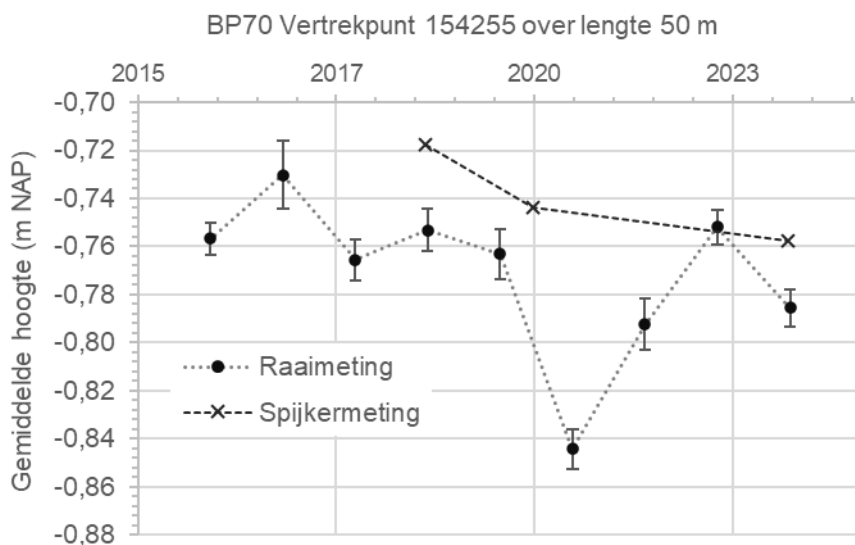
Figuur 6-5 Hoogte van de raaimetingen en de Spijkermetingen bij BP70.
