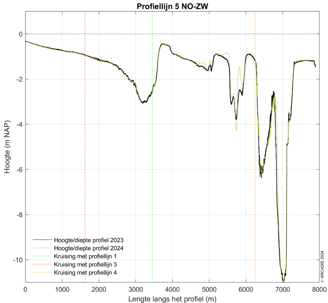
Figuur 3-16 Dwarsprofiel langs profiellijn 5 van noordoost naar zuidwest voor de hoogte/diepte raai meetgegevens van 2023 en 2024.
