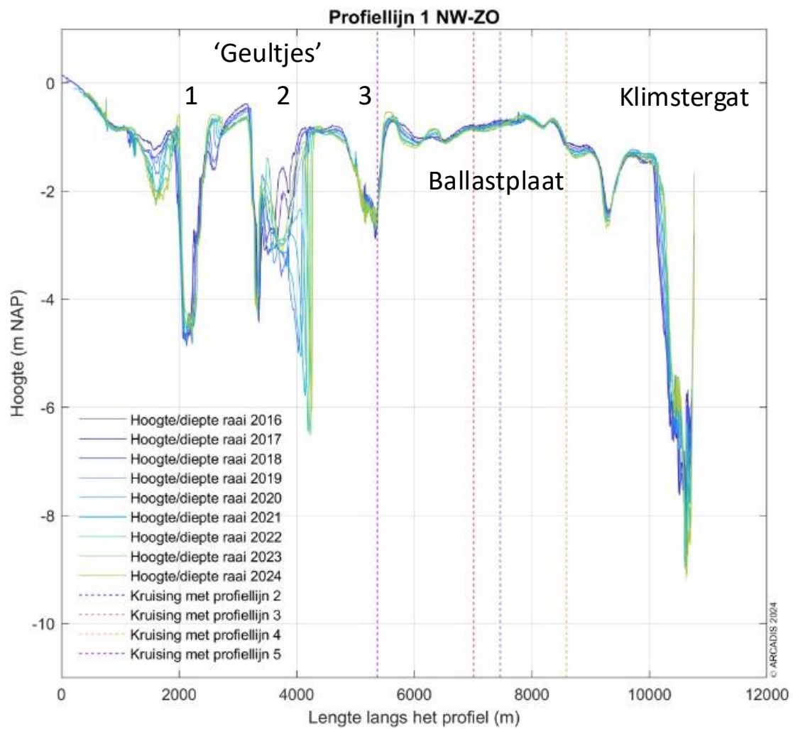
Figuur 4-1 Dwarsprofiel langs profiellijn 1 van noordwest naar zuidoost voor de hoogte/diepte raai meetgegevens van 2016 – 2024.
