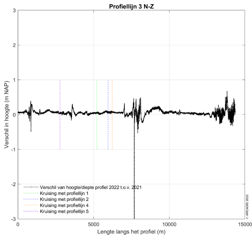
Figuur 9-180 Vershilplot langs profielijn 3 van noord naar zuid voor de hoogte/diepte raai meetgegevens van 2021 en 2022. Een positieve waarde betekent dat de hoogte/diepteraai van mei 2022 hoger ligt dan de hoogte/diepteraai van 2021.
