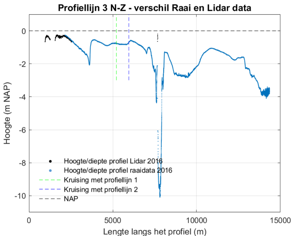
Figuur 9-12 Profiellijn 3 van noord naar zuid voor de hoogte/diepte raai meetgegevens van 2016 en de LiDAR-data van 2016.
