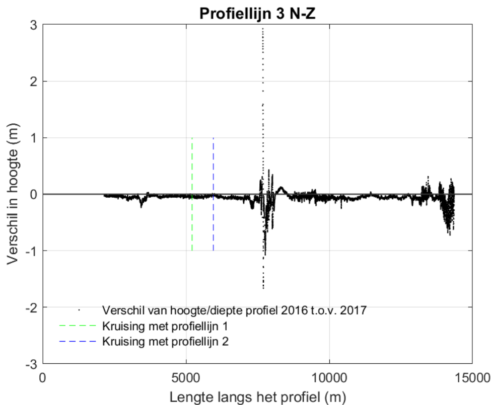
Figuur 9-126 Verschilplot langs profiellijn 3 van noord naar zuid voor de hoogte/diepte raai meetgegevens van 2016 en 2017. Een negatieve waarde betekent dat de hoogte/diepteraai van 2017 lager ligt dan de hoogte/diepteraai van 2016.
