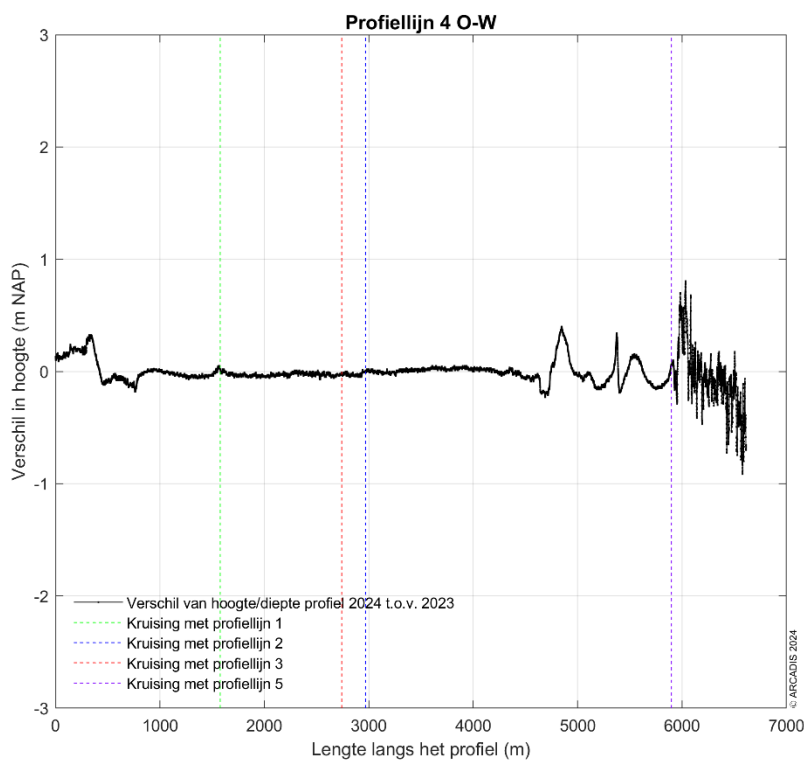
Figuur 3-14 Verschilplot langs profiellijn 4 van oost naar west voor de hoogte/diepte raai meetgegevens van 2023 en 2024. Een positieve waarde betekent dat de hoogte/diepteraai van 2024 hoger ligt dan de hoogte/diepteraai van 2023.
