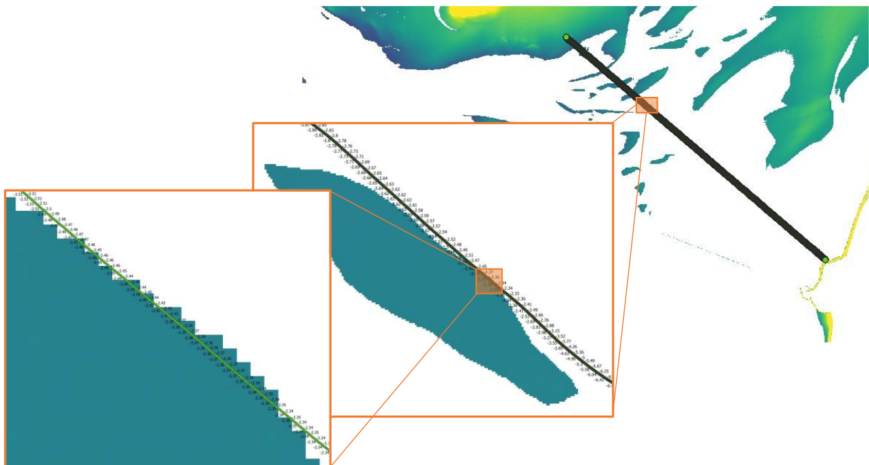
Figuur 9-214: Ligging van de extreme meetwaarden voor raai 1. De extreme waarden zijn precies op de rand van een relatief kleine blootliggende plaat gemeten. Het is niet ongebruikelijk dat hier grotere hoogteverschillen optreden als gevolg van natuurlijke morfologische processen.
