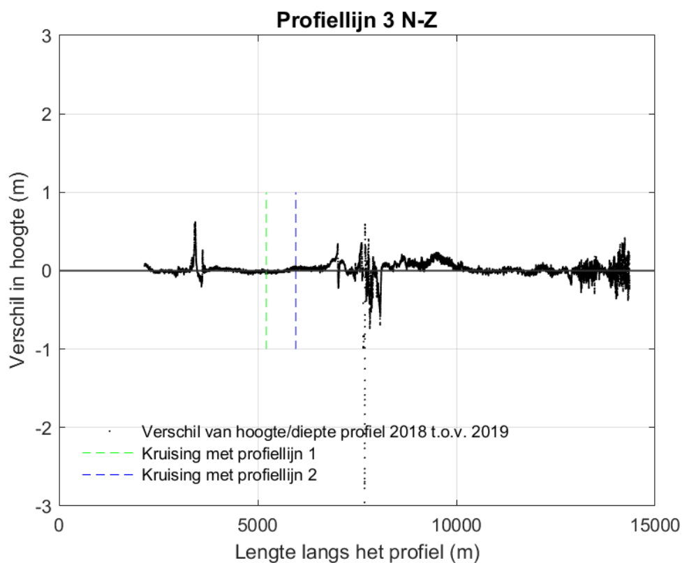
Figuur 9-144 Verschilplot langs profiellijn 3 van noord naar zuid voor de hoogte/diepte raai meetgegevens van 2018 en mei 2019. Een positieve waarde betekent dat de hoogte/diepteraai van mei 2019 hoger ligt dan de hoogte/diepteraai van 2018.
