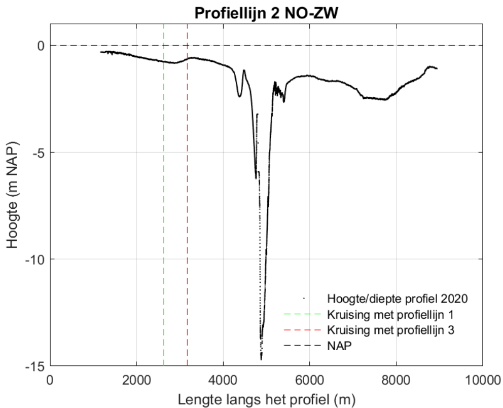
Figuur 9-58 Dwarsdoorsnede langs profiel 2 van noordoost naar zuidwest in 2020.
