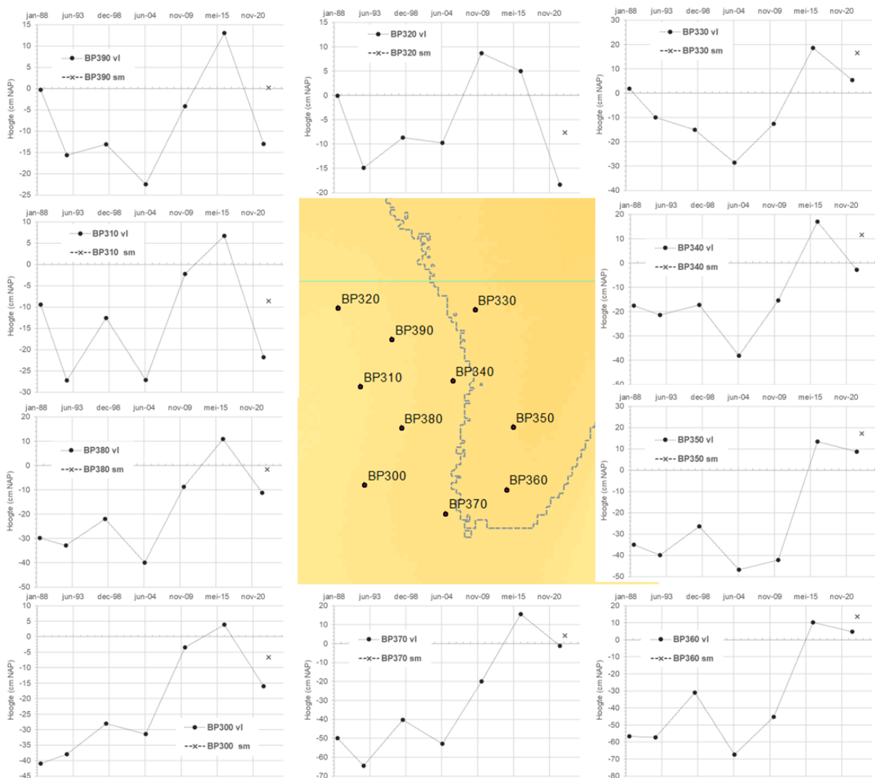
Figuur 7-6 Overzicht van de grafieken van de hoogteontwikkeling op de Ballastplaat Midden.
