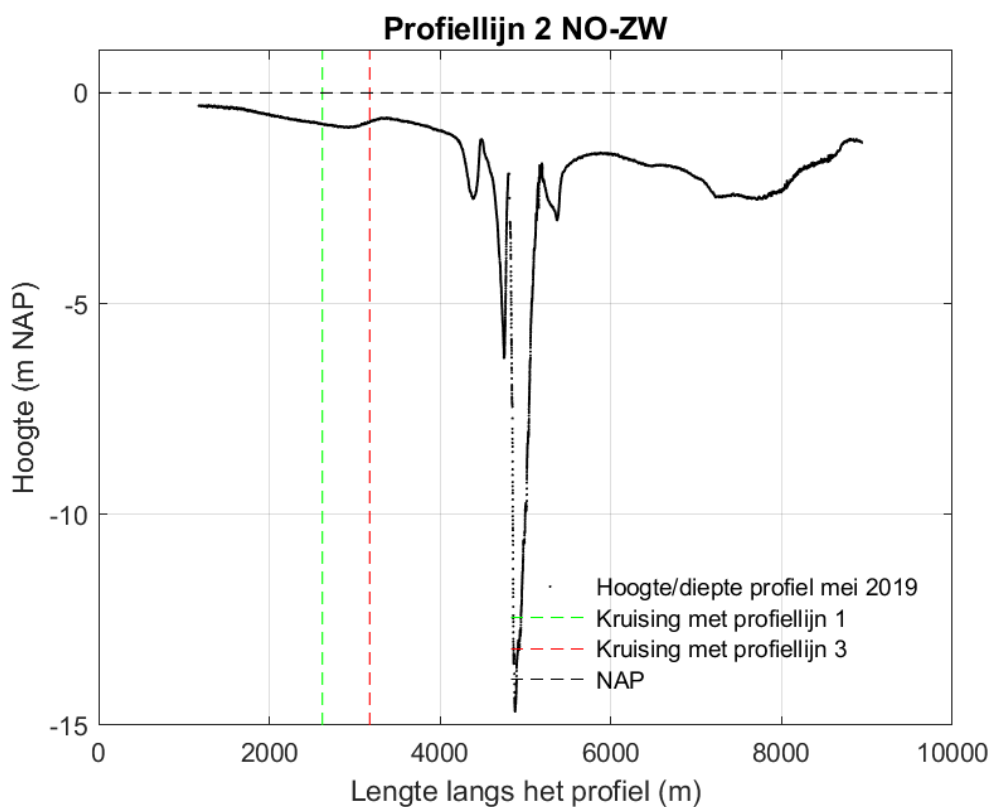
Figuur 9-52 Dwarsdoorsnede langs profiellijn 2 van noordoost naar zuidwest in mei 2019.
