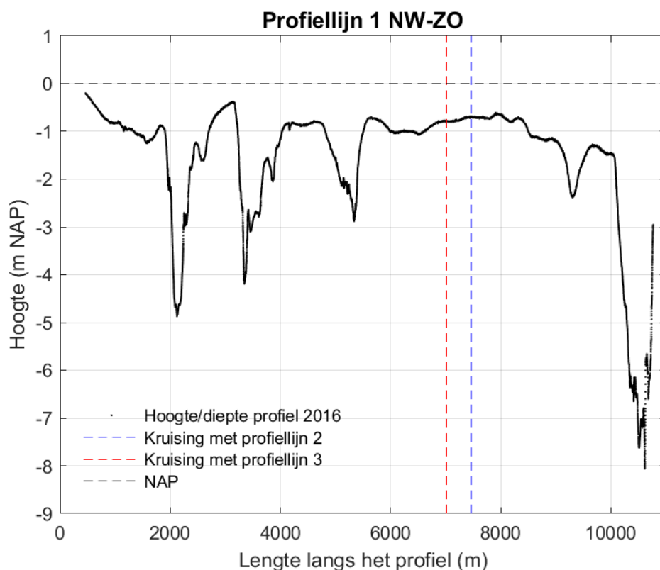
Figuur 9-27 Dwarsdoorsnede langs profiellijn 1 van noordwest naar zuidoost in 2016.
