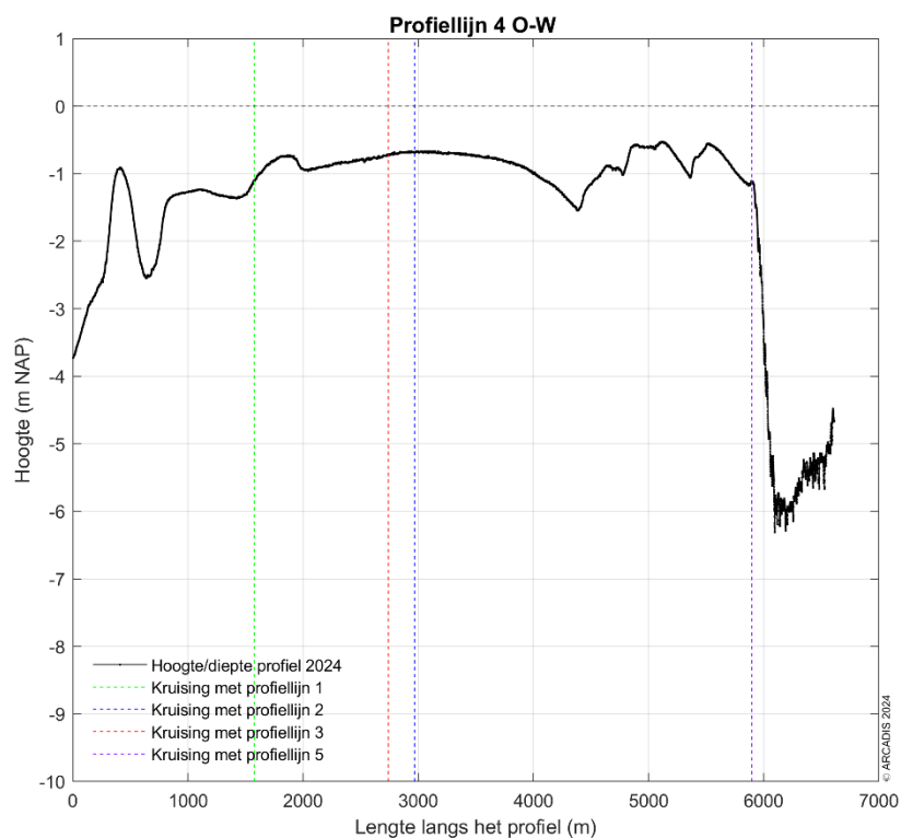
Figuur 9-108 Dwarsdoorsnede langs profiellijn 4 van oost naar west in 2024.
