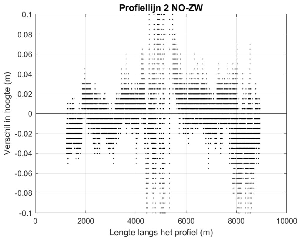
Figuur 9-151 Ingezoomde verschilplot langs profiellijn 2 van noordoost naar zuidwest voor de hoogte/diepte raai meetgegevens van januari 2019 en mei 2019. Een positieve waarde betekent dat de hoogte/diepteraai van mei 2019 hoger ligt dan de hoogte/diepteraai van januari 2019.
