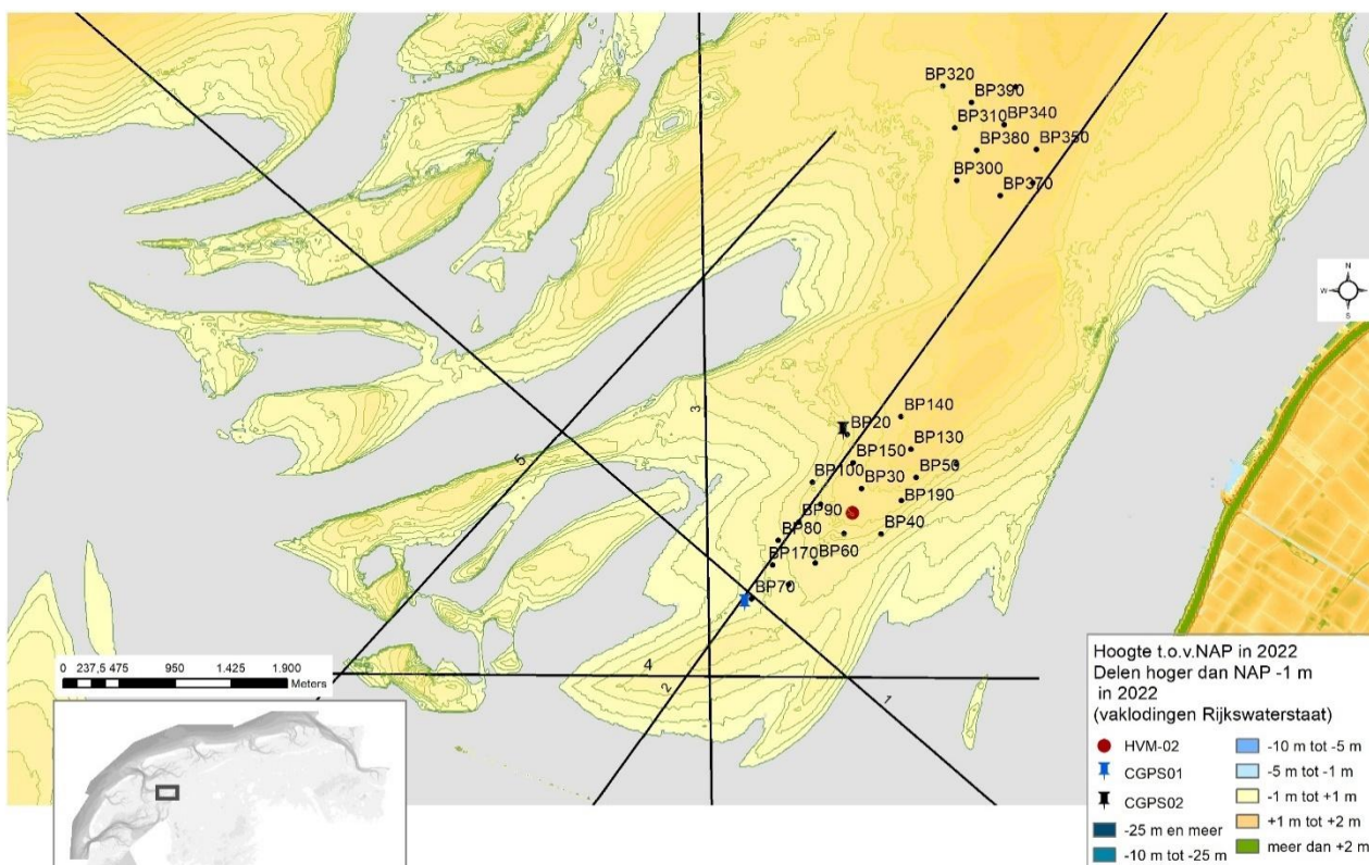
Figuur 7-4 Hoogte van de vakloding 2022, waarbij alleen de delen hoger dan NAP -1 m in 2022 zijn weergegeven.
