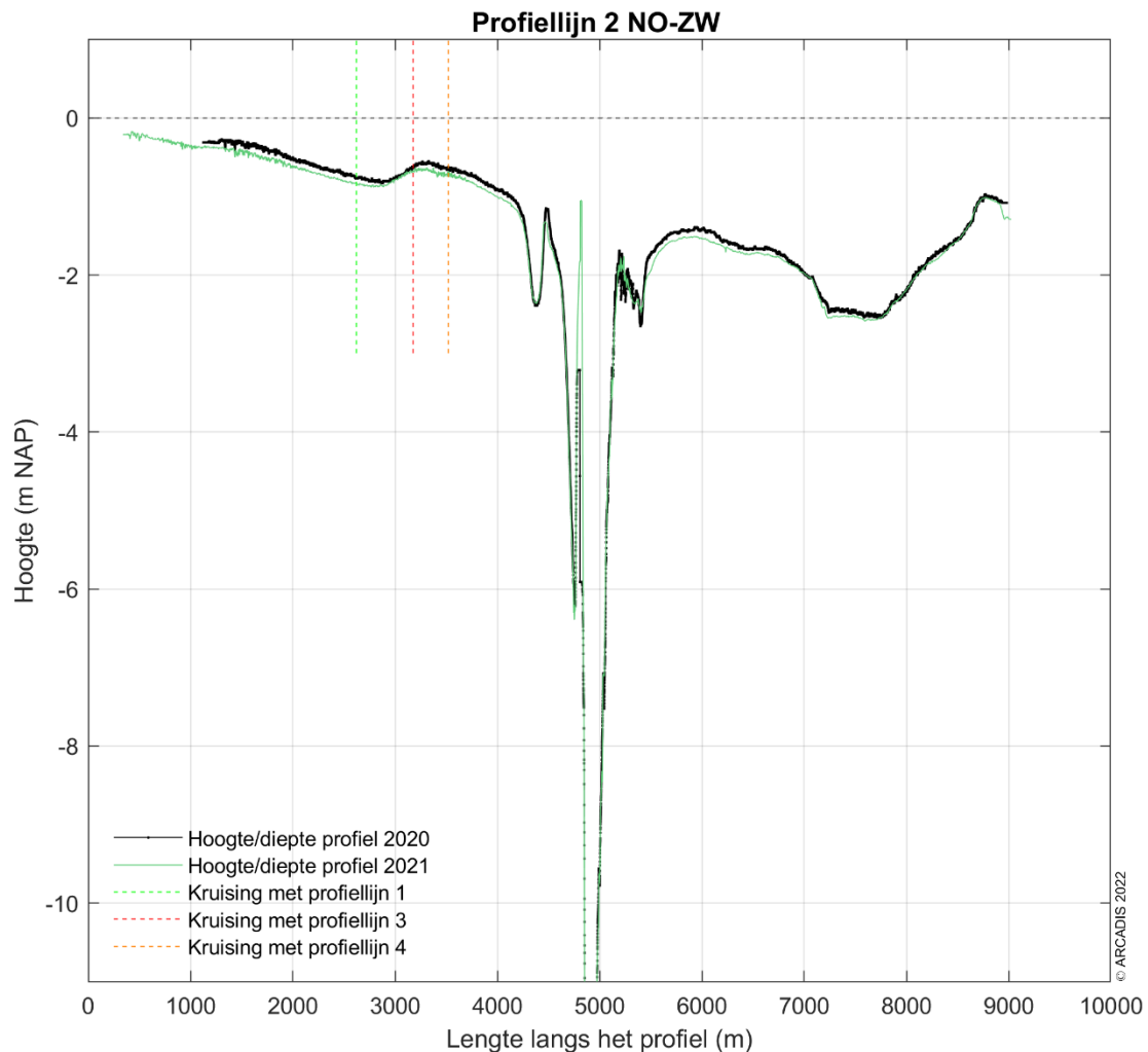
Figuur 9-167 Dwarsdoorsnede langs profiellijn 2 van noordoost naar zuidwest voor de hoogte/diepte raai meetgegevens van 2020 en 2021.
