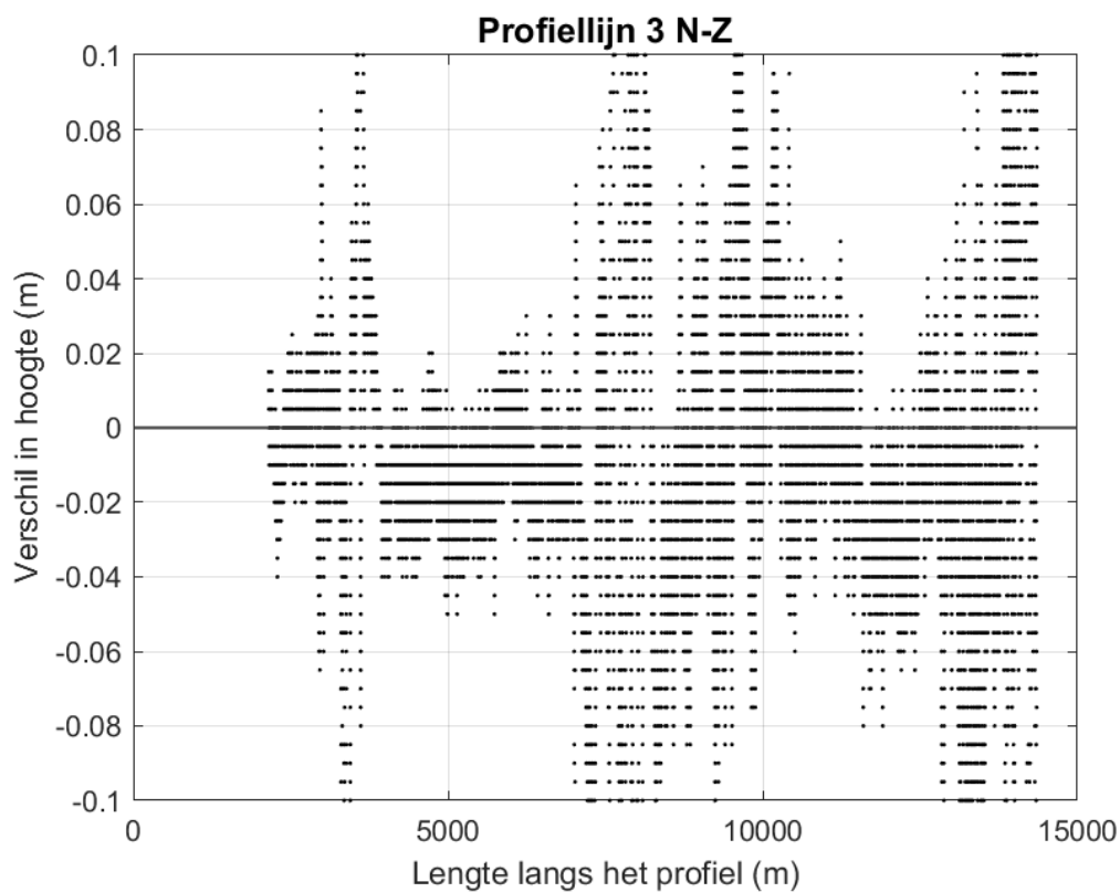
Figuur 9-136 Ingezoomde verschilplot langs profiellijn 3 van noord naar zuid voor de hoogte/diepte raai meetgegevens van 2017 en 2018. Een negatieve waarde betekent dat de hoogte/diepteraai van 2018 lager ligt dan de hoogte/diepteraai van 2017.
