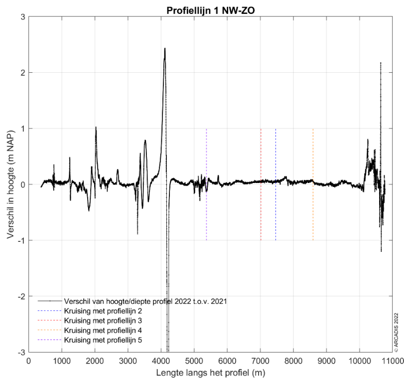
Figuur 9-174 Verschilplot langs profiellijn 1 van noordwest naar zuidoost voor de hoogte/diepte raai meetgegevens van 2021 en 2022. Een positieve waarde betekent dat de hoogte/diepteraai van 2022 hoger ligt dan de hoogte/diepteraai van 2021.
