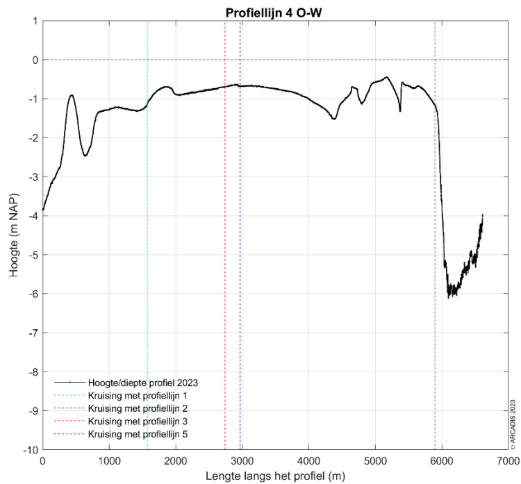
Figuur 9-94 Dwarsdoorsnede langs profiellijn 4 van oost naar west in 2023.
