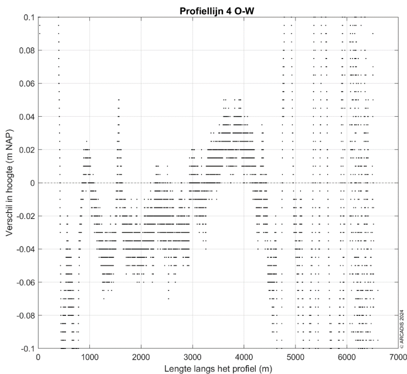
Figuur 3-15: Ingezoomde verschilplot langs profiellijn 4 van oost naar west voor de hoogte/diepte raai meetgegevens van 2023 en 2024. Een positieve waarde betekent dat de hoogte/diepteraai van 2024 hoger ligt dan de hoogte/diepteraai van 2023.
