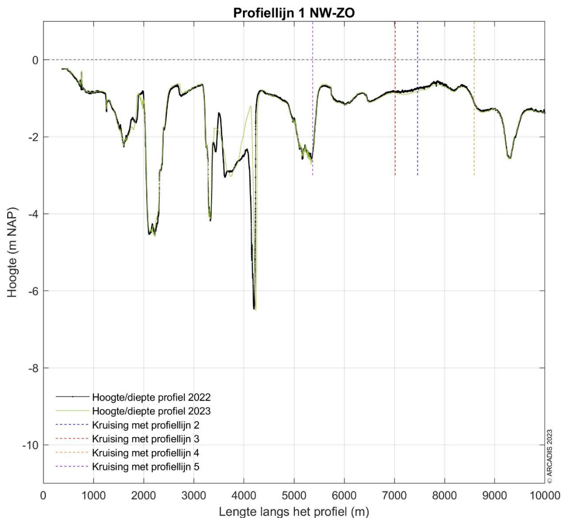
Figuur 9-188 Dwarsdoorsnede langs profiellijn 1 van noordwest naar zuidoost voor de hoogte/diepte raai meetgegevens van 2022 en 2023.
