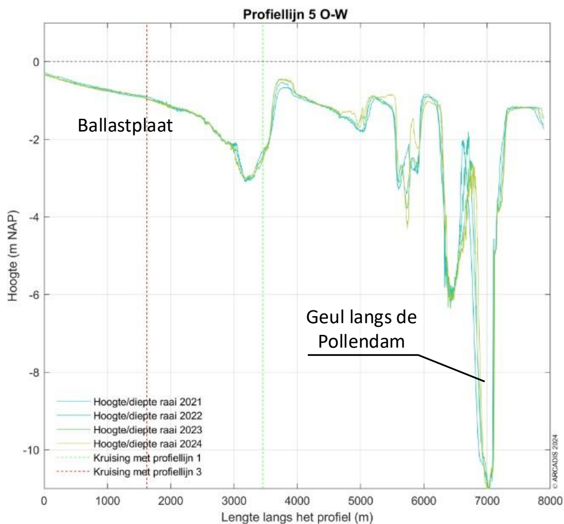
Figuur 4-13 Dwarsprofiel langs profiellijn 5 van oost naar west voor de hoogte/diepte raai meetgegevens van 2016 - 2024.
