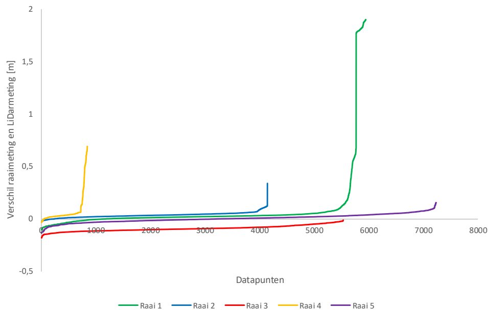
Figuur 9-213: Vergelijking raaimetingen en LiDarmetingen 2022, inclusief extreme waarden.
