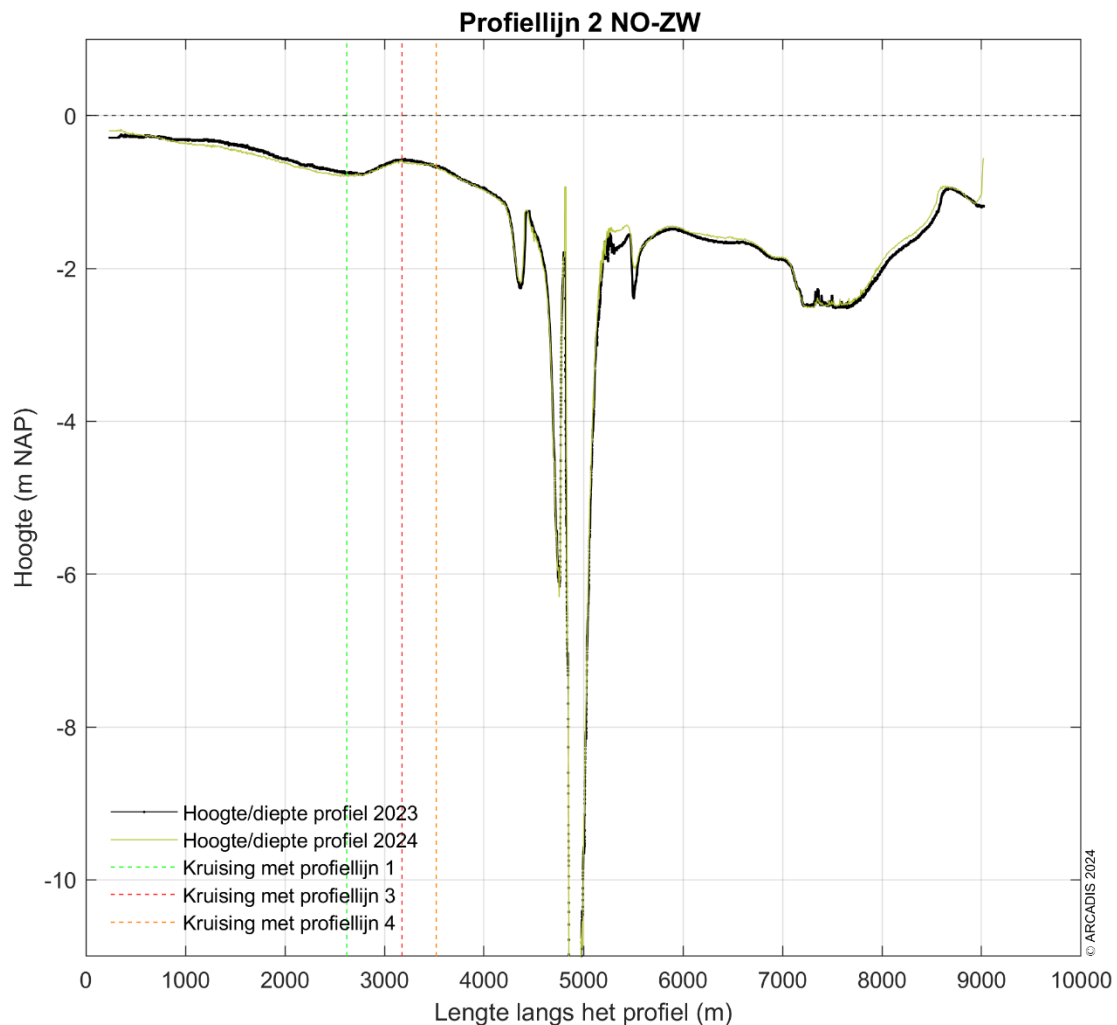
Figuur 3-7 Dwarsdoorsnede langs profiellijn 2 van noordoost naar zuidwest voor de hoogte/diepte raai meetgegevens van 2023 en 2024.
