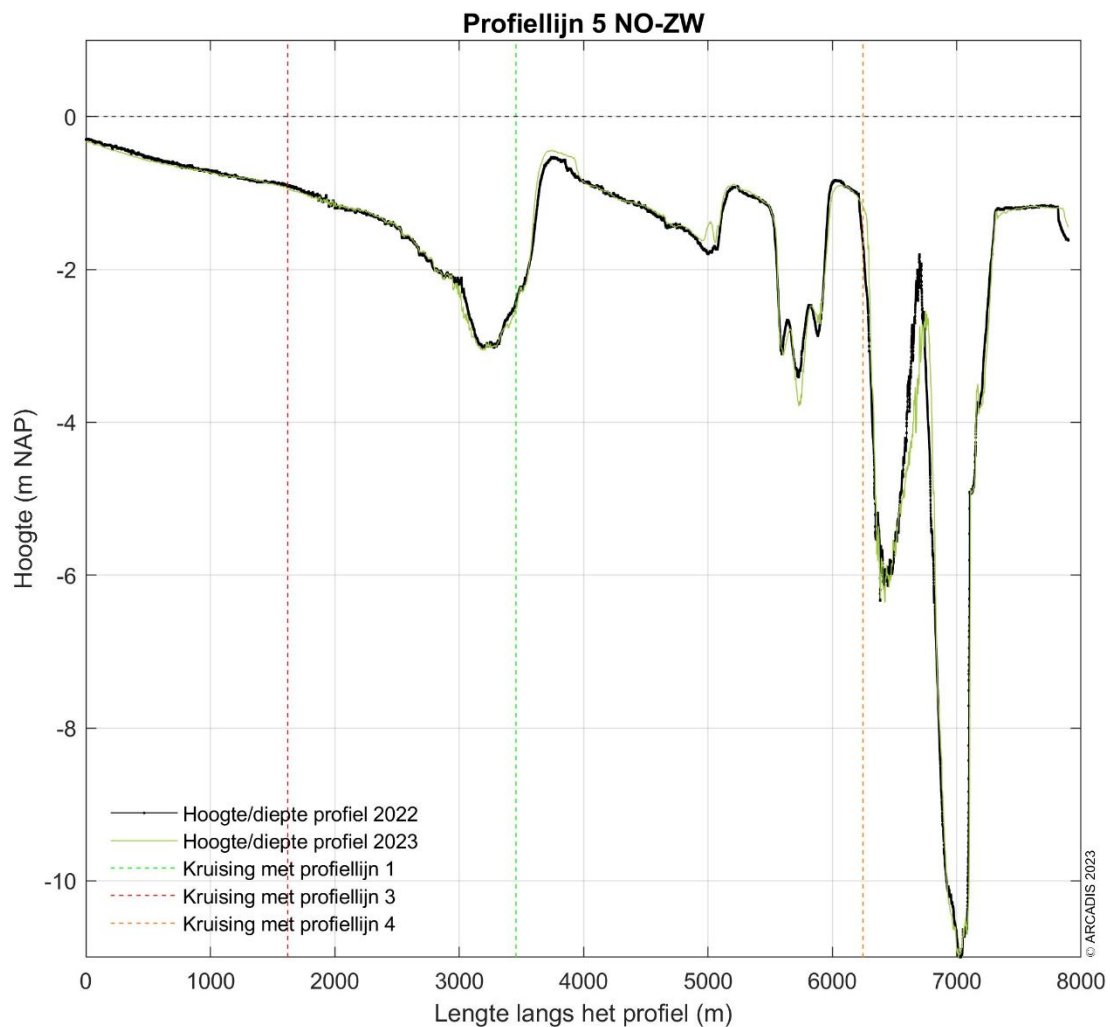
Figuur 9-200 Dwarsprofiel langs profiellijn 5 van noordoost naar zuidwest voor de hoogte/diepte raai meetgegevens van 2022 en 2023.
