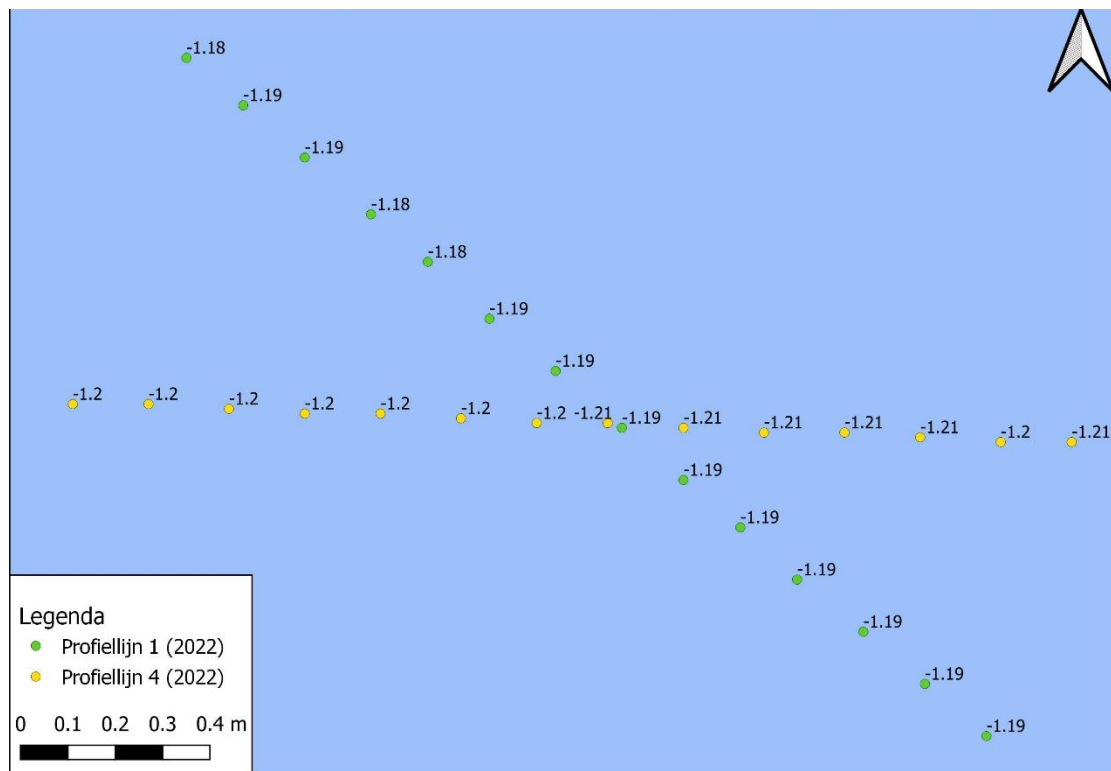
Figuur 9-84 Detailkaart controlepunt tussen profiellijn 1 en profiellijn 4 voor de hoogte/diepte raaien 2022, hoogtemetingen zijn weergegeven in m NAP.
