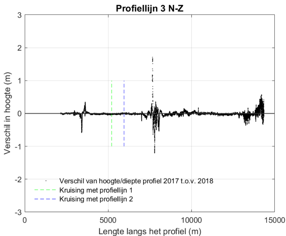
Figuur 9-135 Verschilplot langs profiellijn 3 van noord naar zuid voor de hoogte/diepte raai meetgegevens van 2017 en 2018. Een negatieve waarde betekent dat de hoogte/diepteraai van 2018 lager ligt dan de hoogte/diepteraai van 2017.
