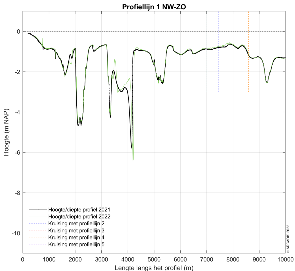
Figuur 9-173 Dwarsdoorsnede langs profiellijn 1 van noordwest naar zuidoost voor de hoogte/diepte raai meetgegevens van 2021 en 2022.
