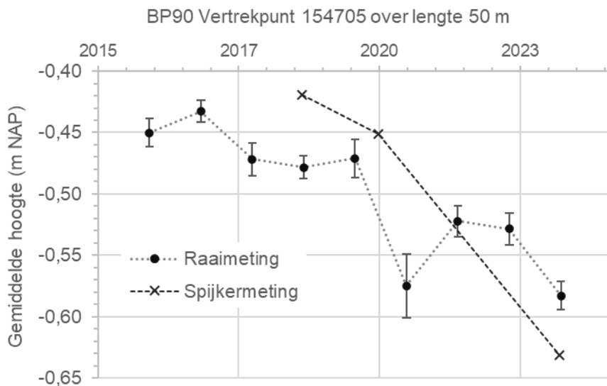
Figuur 6-9 Hoogte van de raaimetingen en de Spijkermetingen bij BP90.
