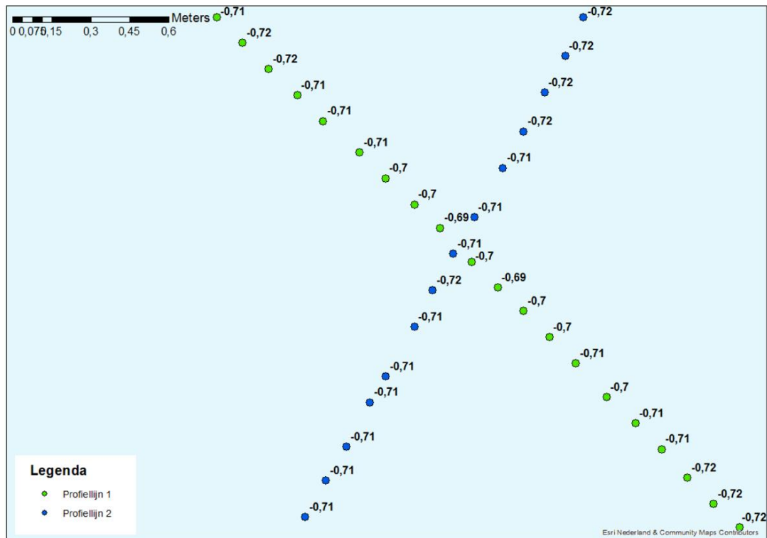
Figuur 9-36 Detailkaart controlepunt tussen profiellijn 1 en profiellijn 2 voor de hoogte/diepte raaien 2017, hoogtemetingen zijn weergegeven in m NAP.
