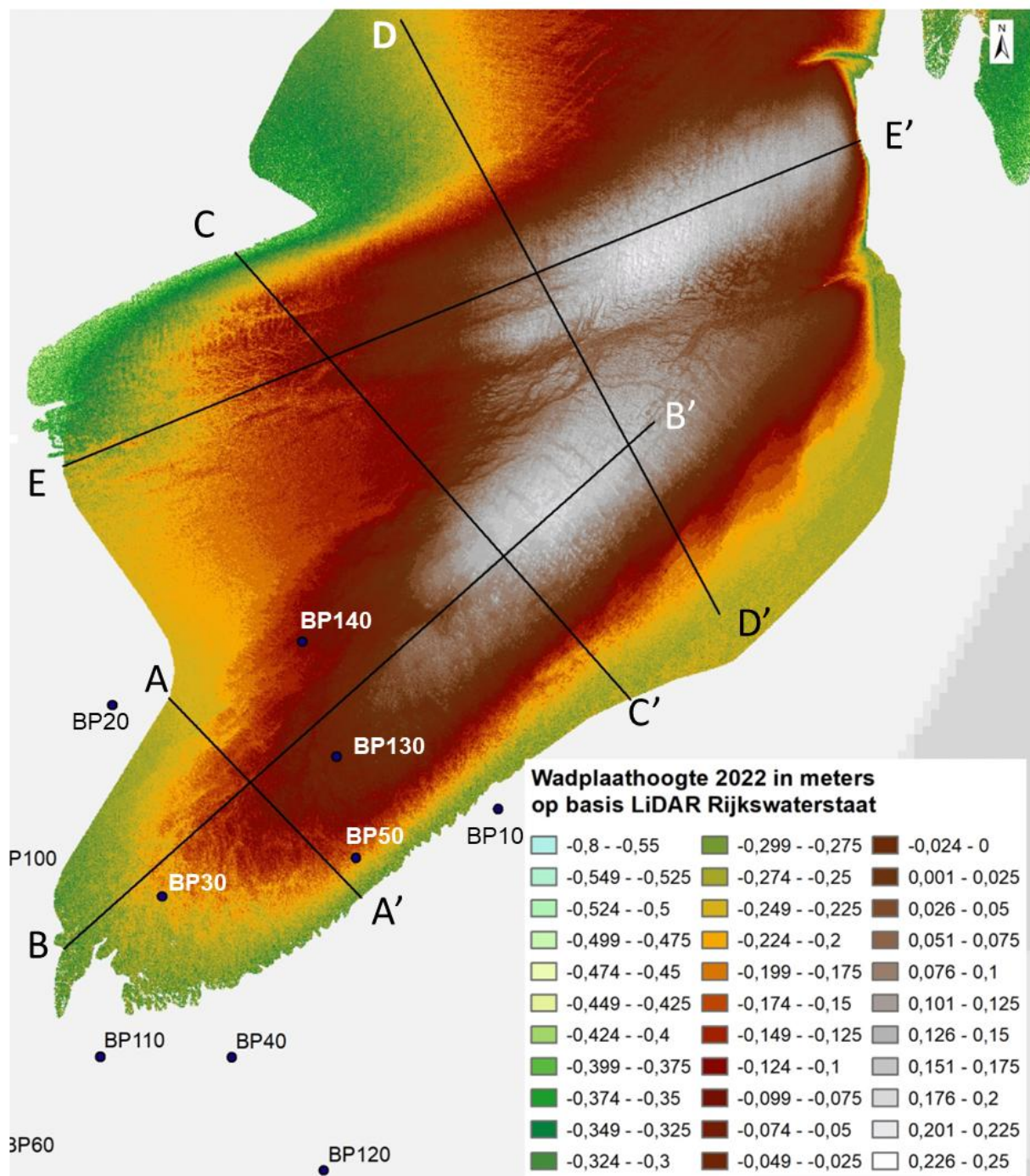
Figuur 9-217 Kaart met de hoogte van de wadplaten, zoals in 2022 ingemeten met LiDAR. De zwarte stippen zijn de locaties van de Spijkermetingen op de Ballastplaat. In de kaart zijn 5 profiellijnen gemarkeerd.
