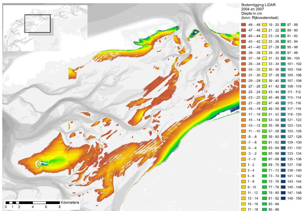
Figuur 9-1 Overzichtskartaal van het kombergingsgebied van het Vlie met de gecombineerde LiDAR opname van 2004 en 2007.
