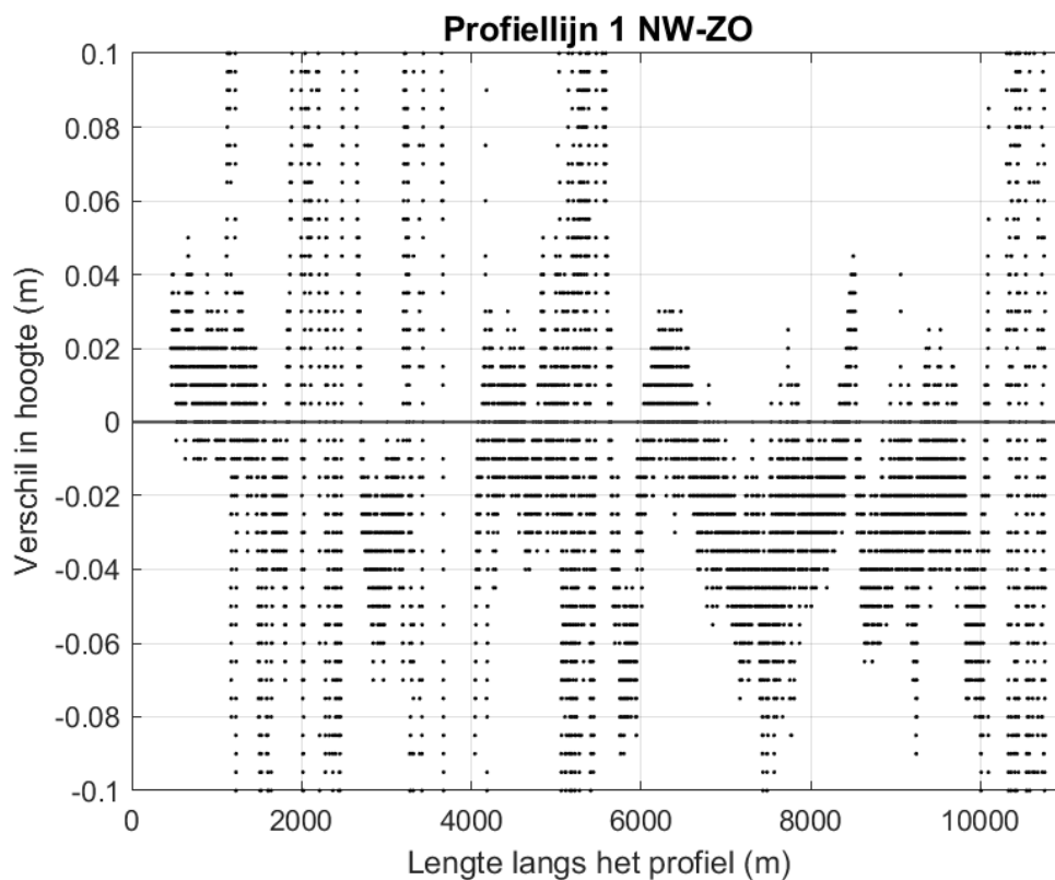
Figuur 9-130 Ingezoomde verschilplot langs profiellijn 1 van noordwest naar zuidoost voor de hoogte/diepte raai meetgegevens van 2017 en 2018. Een negatieve waarde betekent dat de hoogte/diepteraai van 2018 lager ligt dan de hoogte/diepteraai van 2017.
