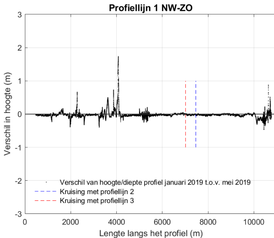
Figuur 9-147 Verschilplot langs profiellijn 1 van noordwest naar zuidoost voor de hoogte/diepte raai meetgegevens van januari 2019 en mei 2019. Een negatieve waarde betekent dat de hoogte/diepteraai van mei 2019 lager ligt dan de hoogte/diepteraai van januari 2019.
