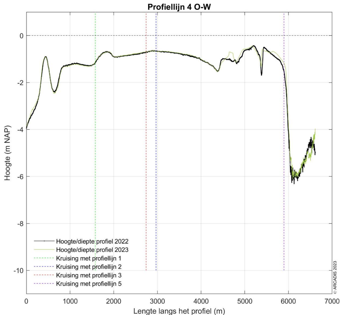
Figuur 9-197 Dwarsprofiel langs profiellijn 4 van oost naar west voor de hoogte/diepte raai meetgegevens van 2022 en 2023.
