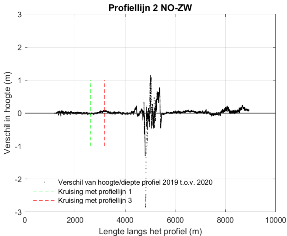
Figuur 9-159 Verschilplot langs profiellijn 2 van noordoost naar zuidwest voor de hoogte/diepte raai meetgegevens van 2019 en 2020. Een positieve waarde betekent dat de hoogte/diepteraai van mei 2020 hoger ligt dan de hoogte/diepteraai van 2019.
