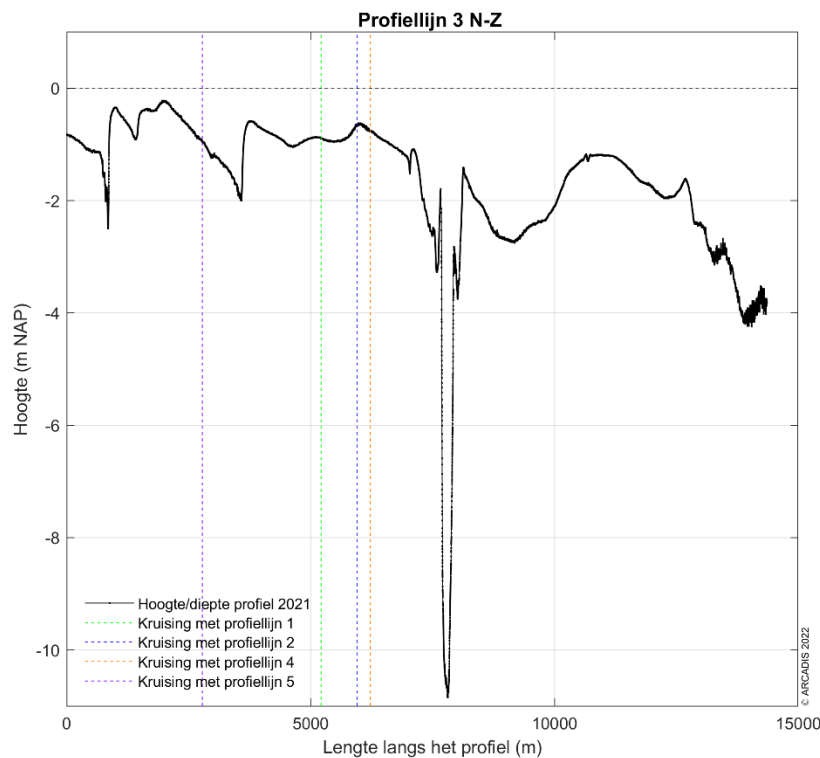
Figuur 9-65 Dwarsdoorsnede langs profiellijn 3 van noord naar zuid in 2021.
