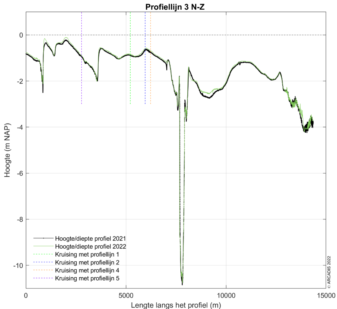
Figuur 9-179 Dwarsprofiel langs profiellijn 3 van noord naar zuid voor de hoogte/diepte raai meetgegevens van 2021 en 2022.
