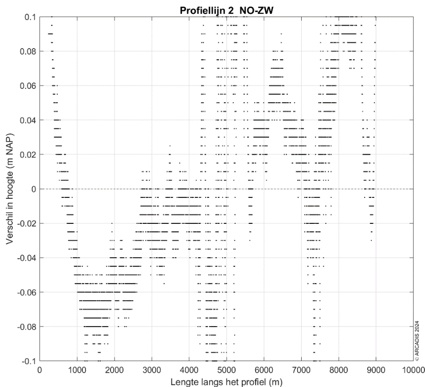
Figuur 3-9 Ingezoomde verschilplot langs profiellijn 2 van noordoost naar zuidwest voor de hoogte/diepte raai meetgegevens van 2023 en 2024. Een positieve waarde betekent dat de hoogte/diepteraai van 2024 hoger ligt dan de hoogte/diepteraai van 2023.
