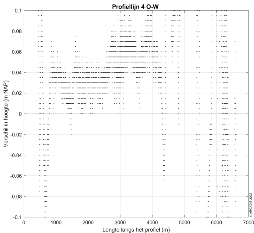
Figuur 9-184: Ingezoomde verschilplot langs profiellijn 4 van oost naar west voor de hoogte/diepte raai meetgegevens van 2021 en 2022. Een positieve waarde betekent dat de hoogte/diepteraai van 2022 hoger ligt dan de hoogte/diepteraai van 2021.
