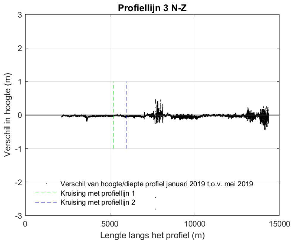
Figuur 9-153 Verschilplot langs profiellijn 3 van noord naar zuid voor de hoogte/diepte raai meetgegevens van januari 2019 en mei 2019. Een negatieve waarde betekent dat de hoogte/diepteraai van mei 2019 lager ligt dan de hoogte/diepteraai van januari 2019.
