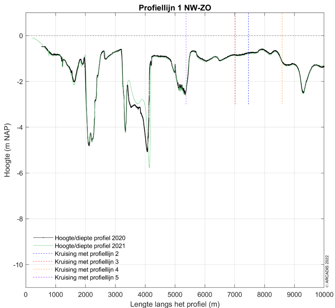
Figuur 9-164 Dwarsdoorsnede langs profiellijn 1 van noordwest naar zuidoost voor de hoogte/diepte raai meetgegevens van 2020 en 2021.
