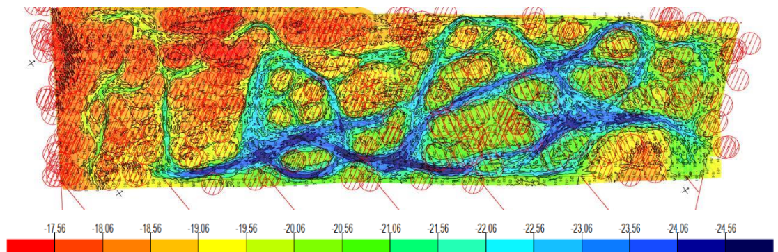
Figuur 3.2 Voorbeeld van een uitpeiling van een zandwingebed na winning, waarbij de blauwere kleuren dieper liggende bodem en rode kleuren ondieper liggende bodem aangeven. De gestreepte cirkels zijn bufferzones om gedetecteerde objecten. Bron: Rijkswaterstaat (pers. com. Suzan van Lieshout, Rijkswaterstaat).
