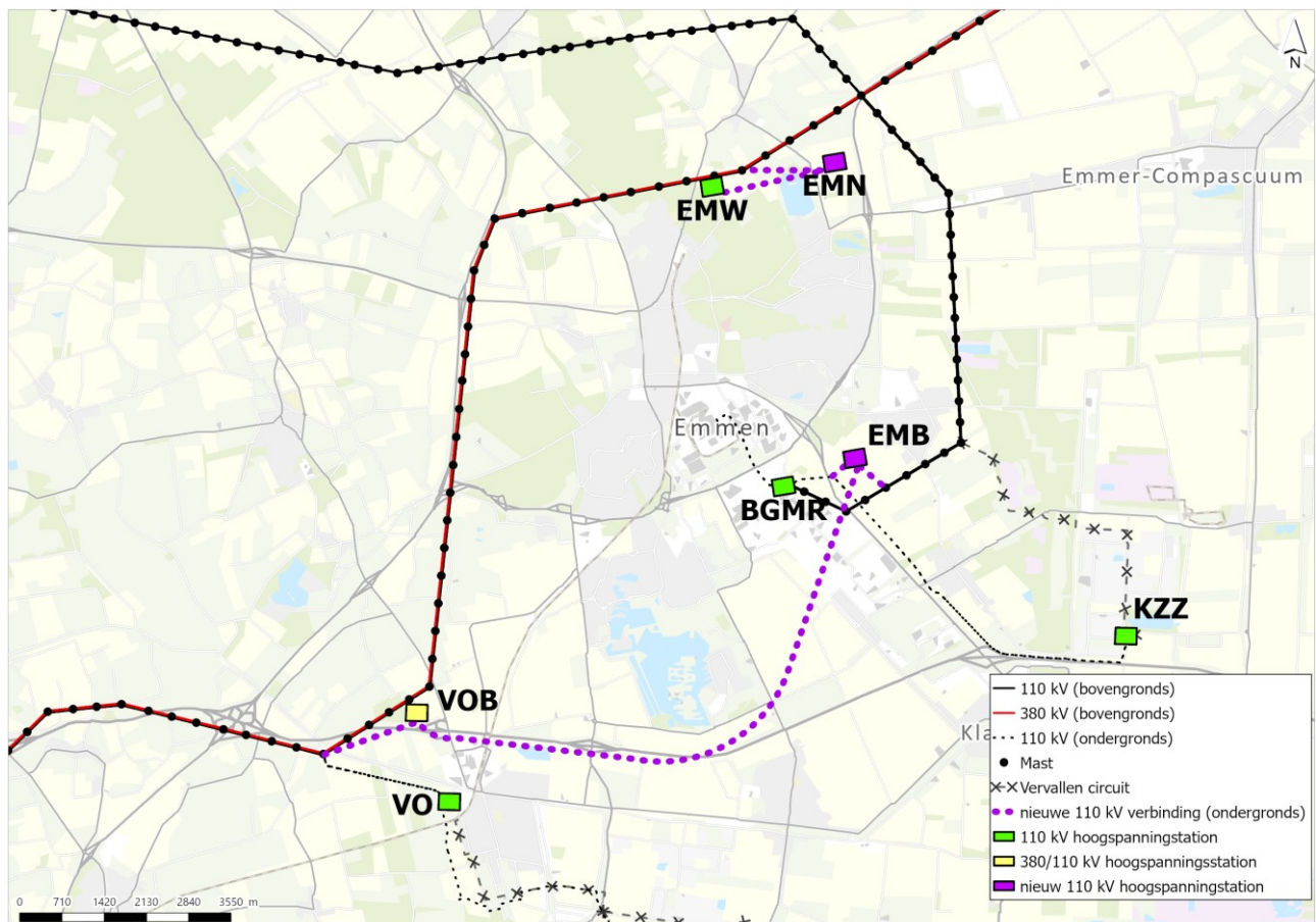
Figuur 2.1 Hoogspanningsnetwerk in omgeving Emmen inclusief de nieuwe projectonderdelen (paars). De ligging van de nieuwe projectonderdelen is indicatief
