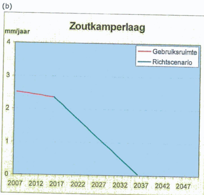
Figuur gebruiksruimte voor inpassen gaswinning voor respectievelijk kombereingsgebied Pinkegat (a) en Zoutkamperlaag (b).
