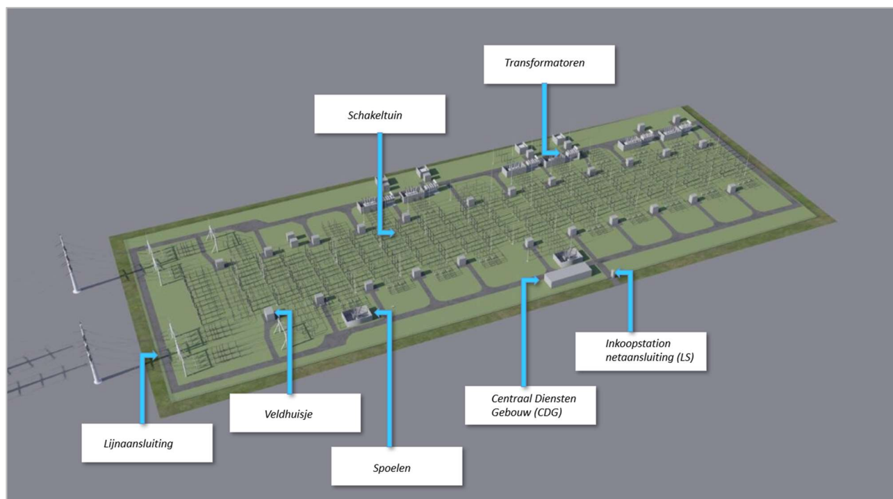
Figuur 1-3 Schematisch weergave 380kV-station
