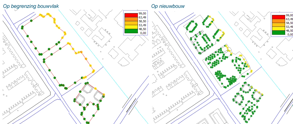
Abbeelding 4-4: Maximale geluidbelasting op grens bouwvlakken t.g.v. Maarssebroeksedijk.
