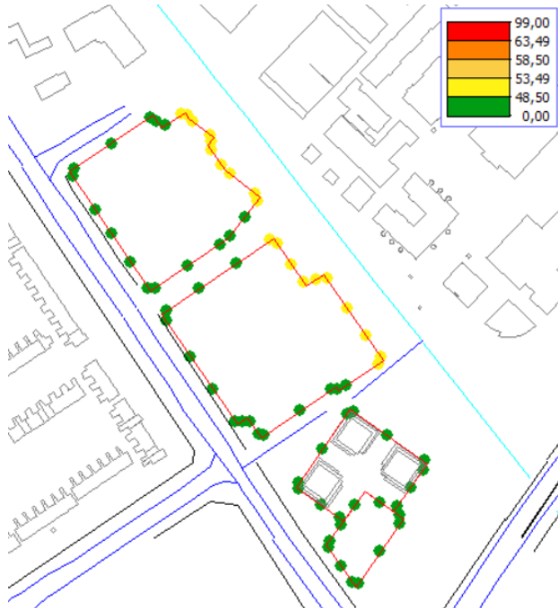
Afbeelding 5-4: Geluidbelasting Maarssebroeksedijk na maatregelen.
