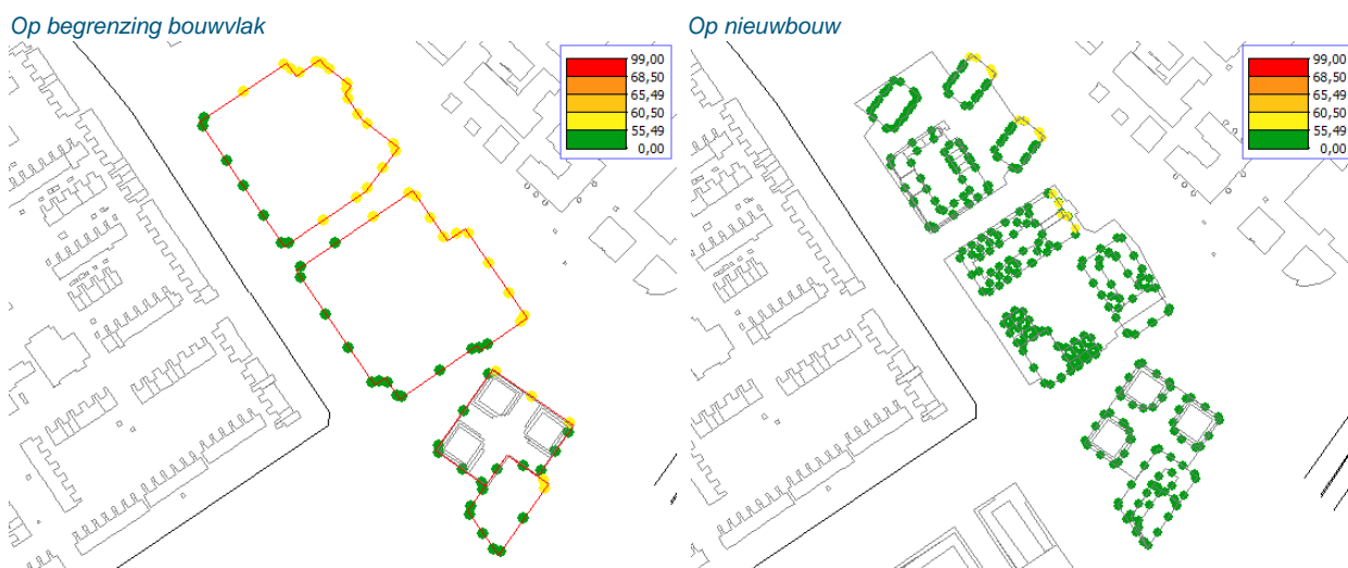
Afbeelding 4-5: Maximale geluidbelasting t.g.v. spoorlijn.
