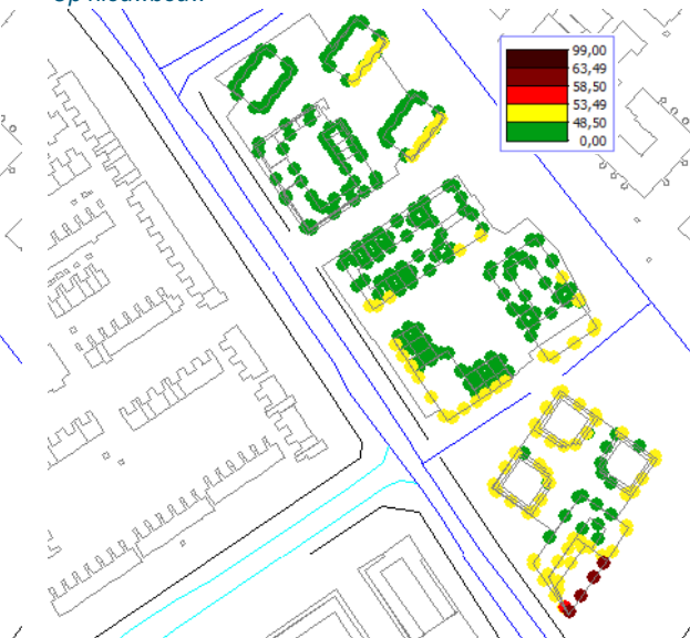
Afbeelding 5-2: Geluidbelasting Zuilense Ring na maatregelen, incl. art. 110g Wgh.
