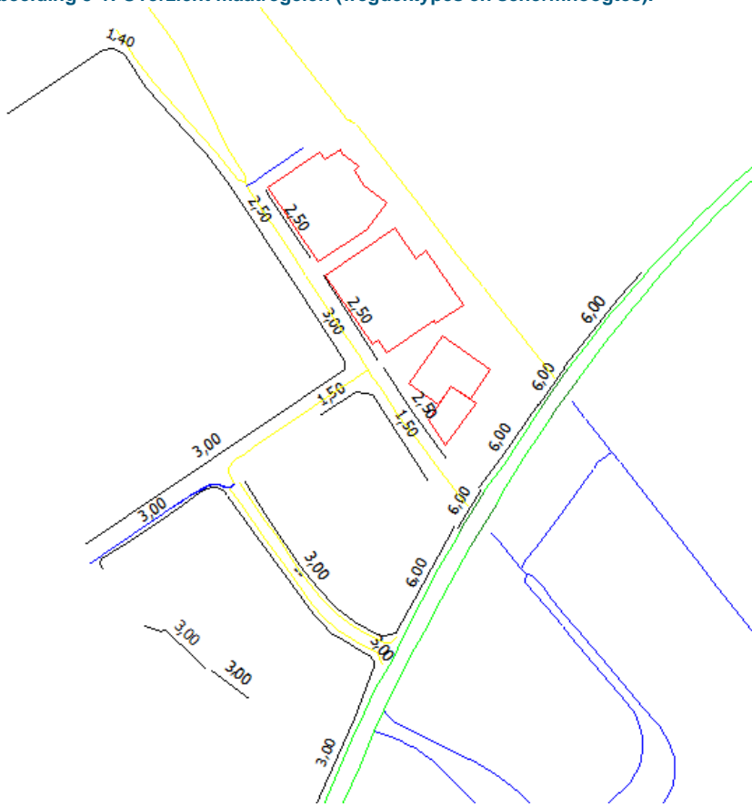
Afbeelding 5-1: Overzicht maatregelen (wegdektypes en schermhoogtes).
