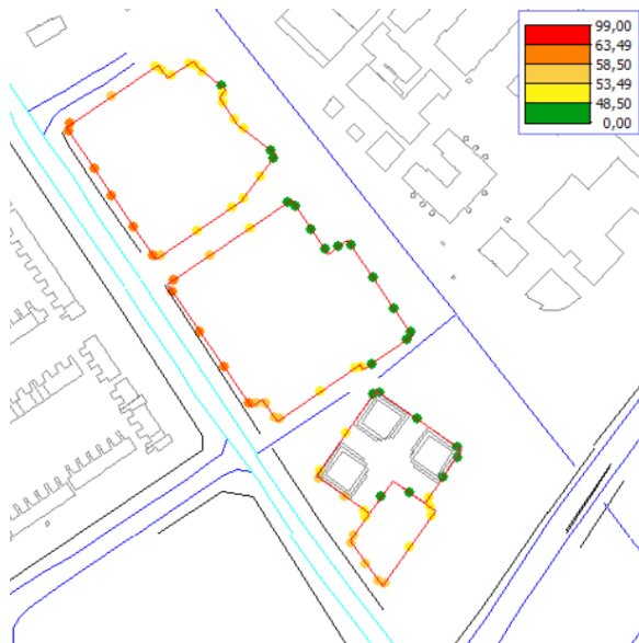
Afbeelding 5-4: Geluidbelasting Maarssebroeksedijk na maatregelen.
