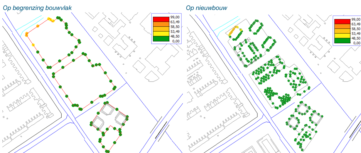
Afbeelding 4-3: Maximale geluidbelasting t.g.v. Kometenweg.
