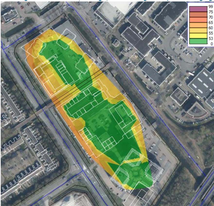
Afbeelding 5-5: Geluidcontour 1,5m hoogte, cumulatief wegverkeer (excl. art. 110g Wgh).
