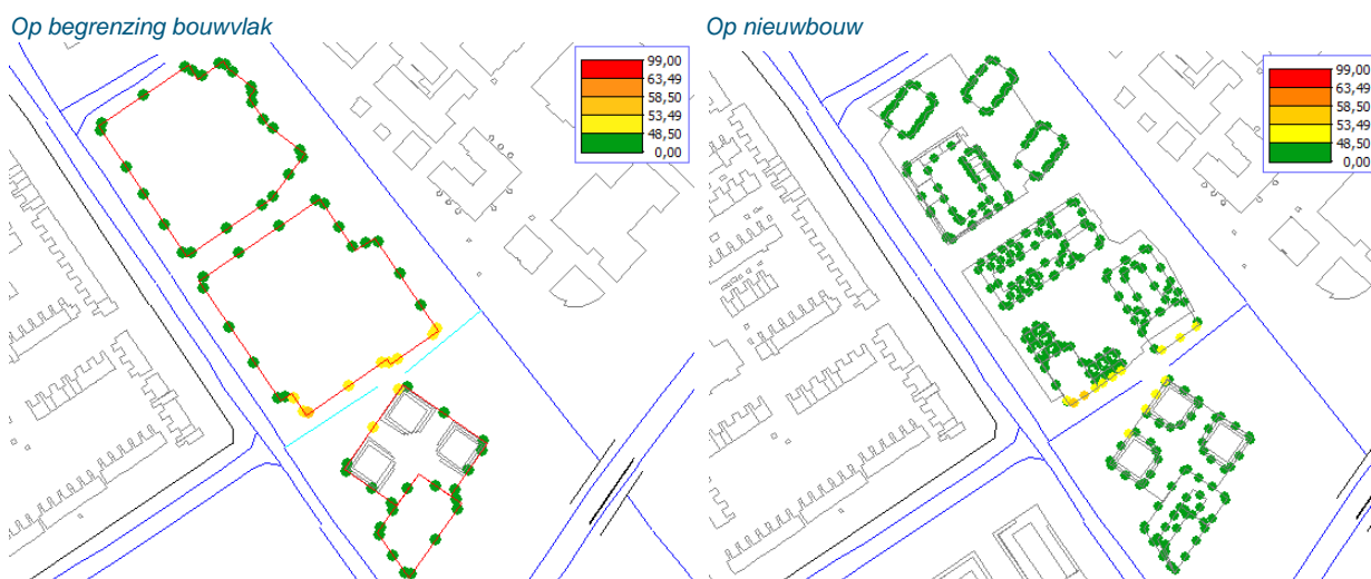
Afbeelding 4-6: Maximale geluidbelasting t.g.v. 30 km/uur wegen.
