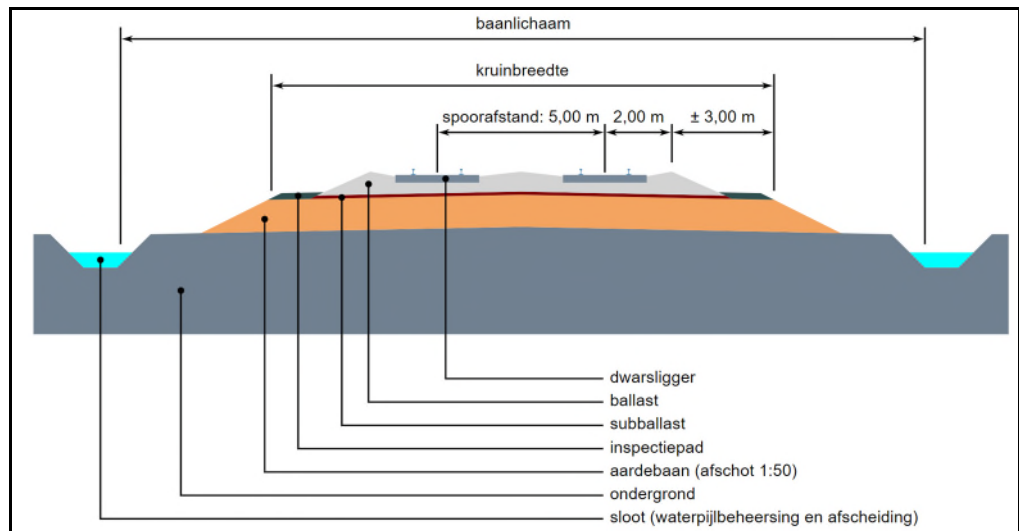
Figuur 3: Dwarsdoorsnede van het baanlichaam.
