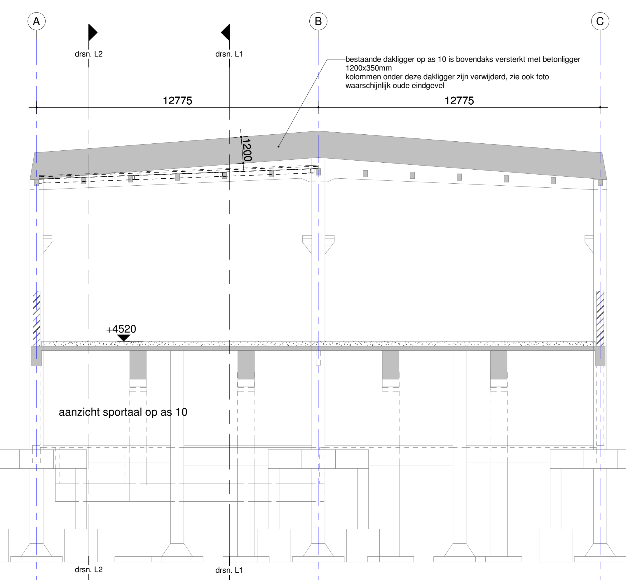
drsn. 9-10 1 : 100
