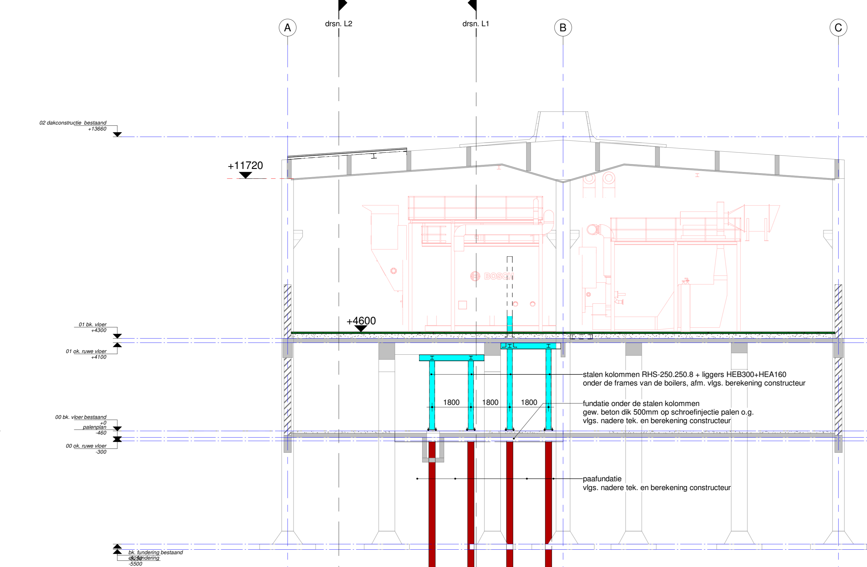
drsn. 11-13 1 : 100
