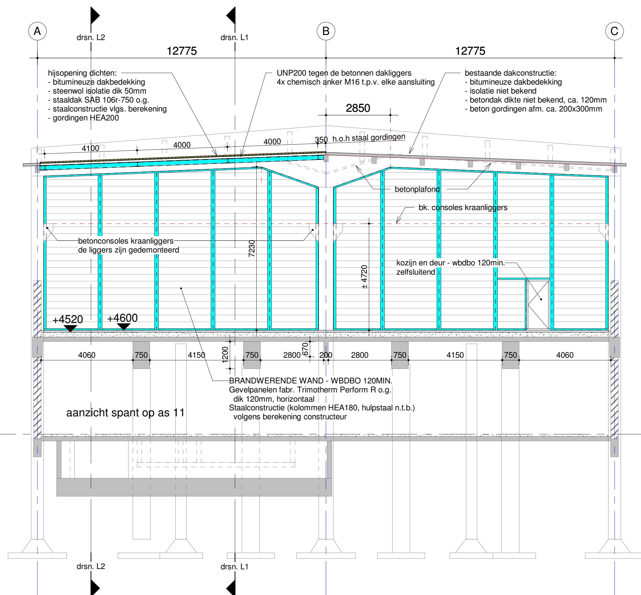
drsn. 10-11 1 : 100
