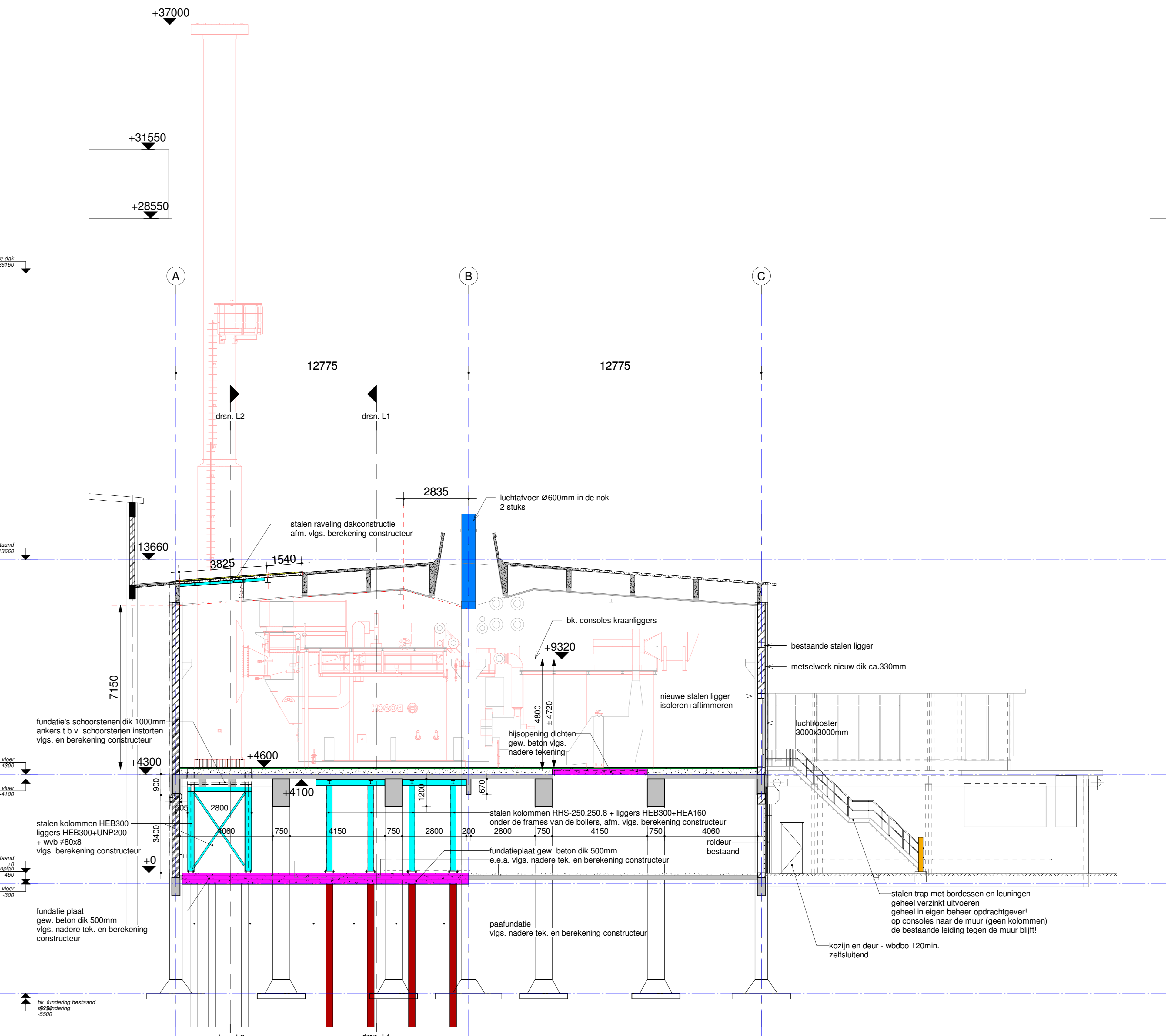
drsn. 14-15 1 : 100
