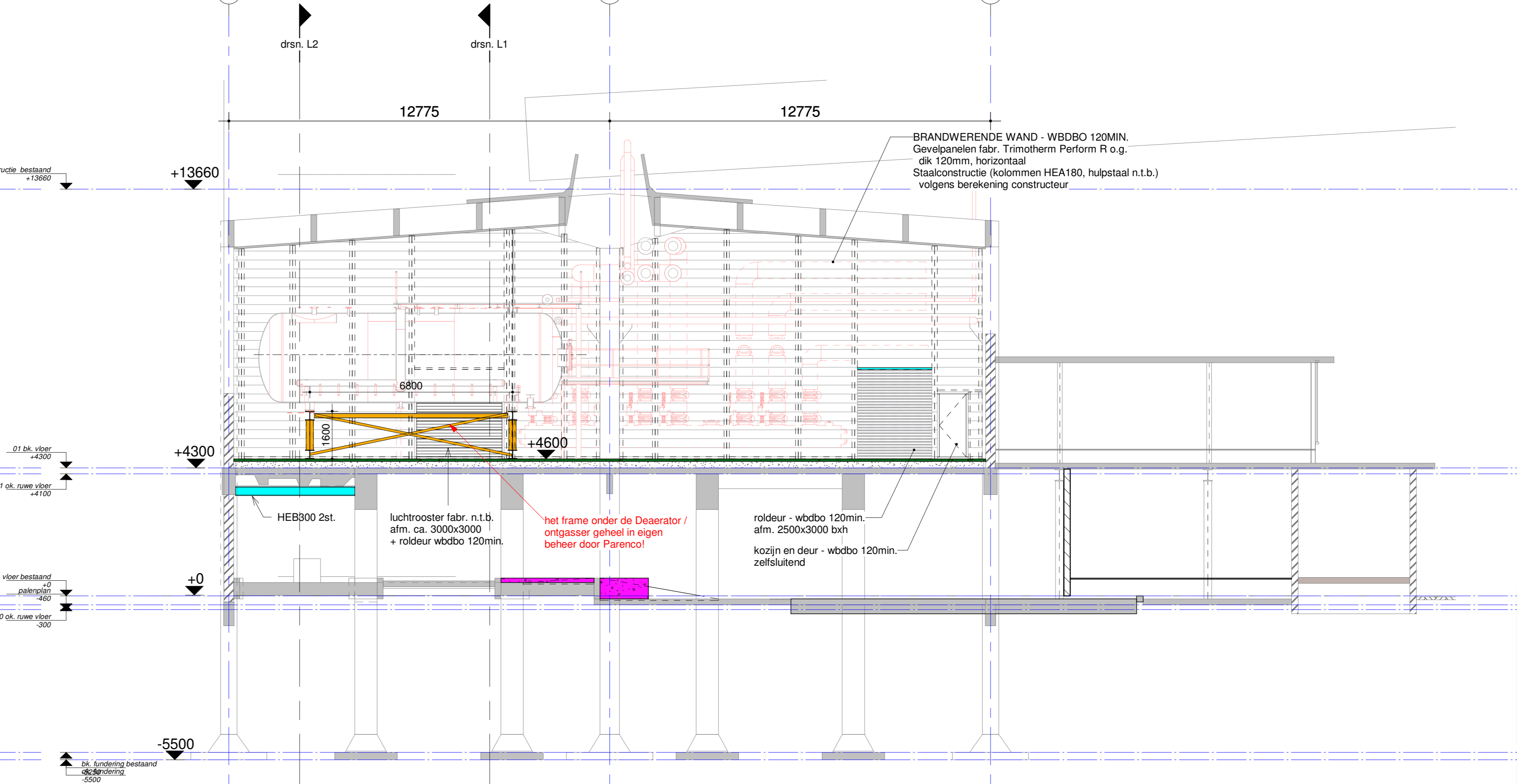
drsn. 15-16 1 : 100
