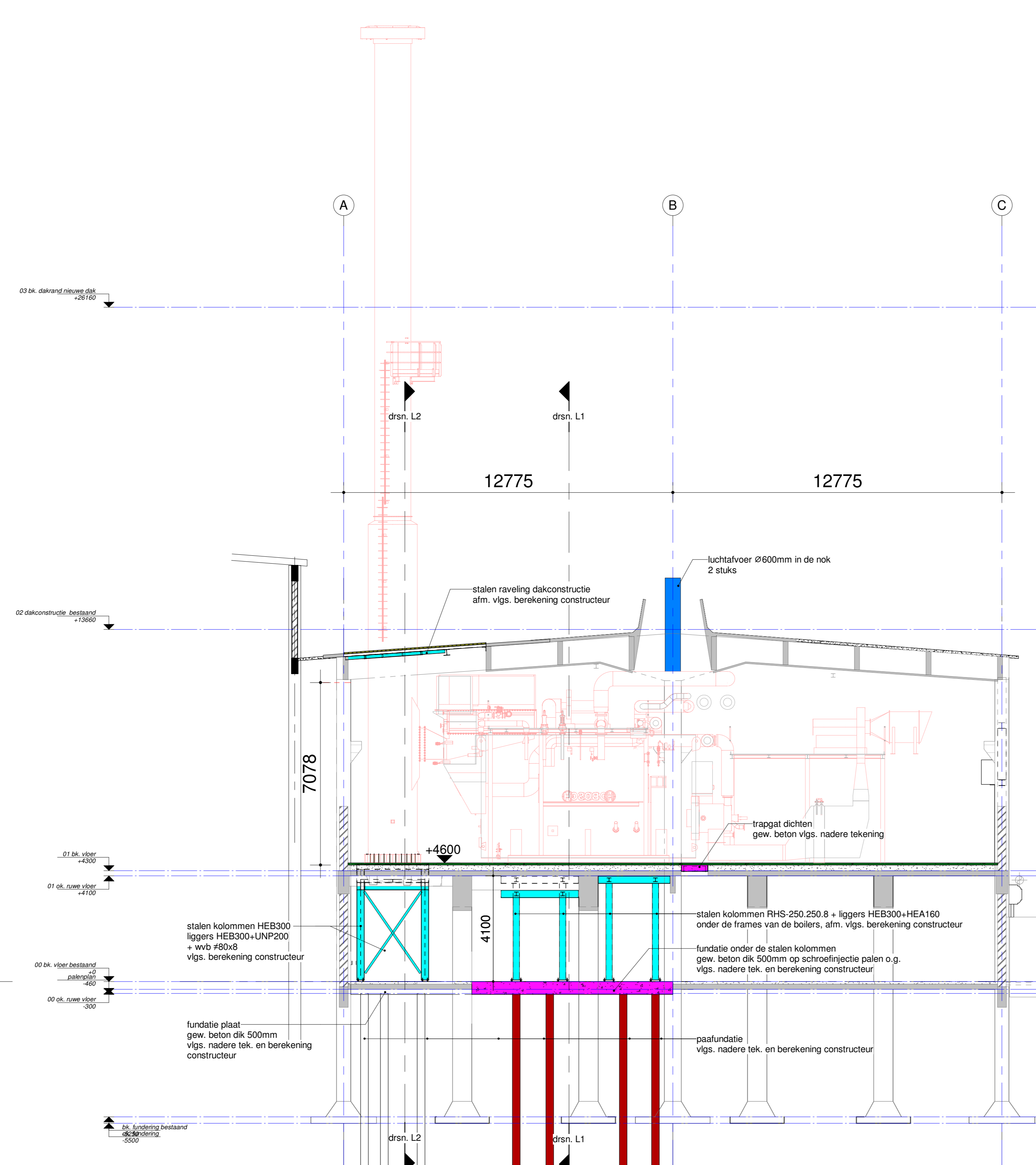
drsn. 13-14 1 : 100
