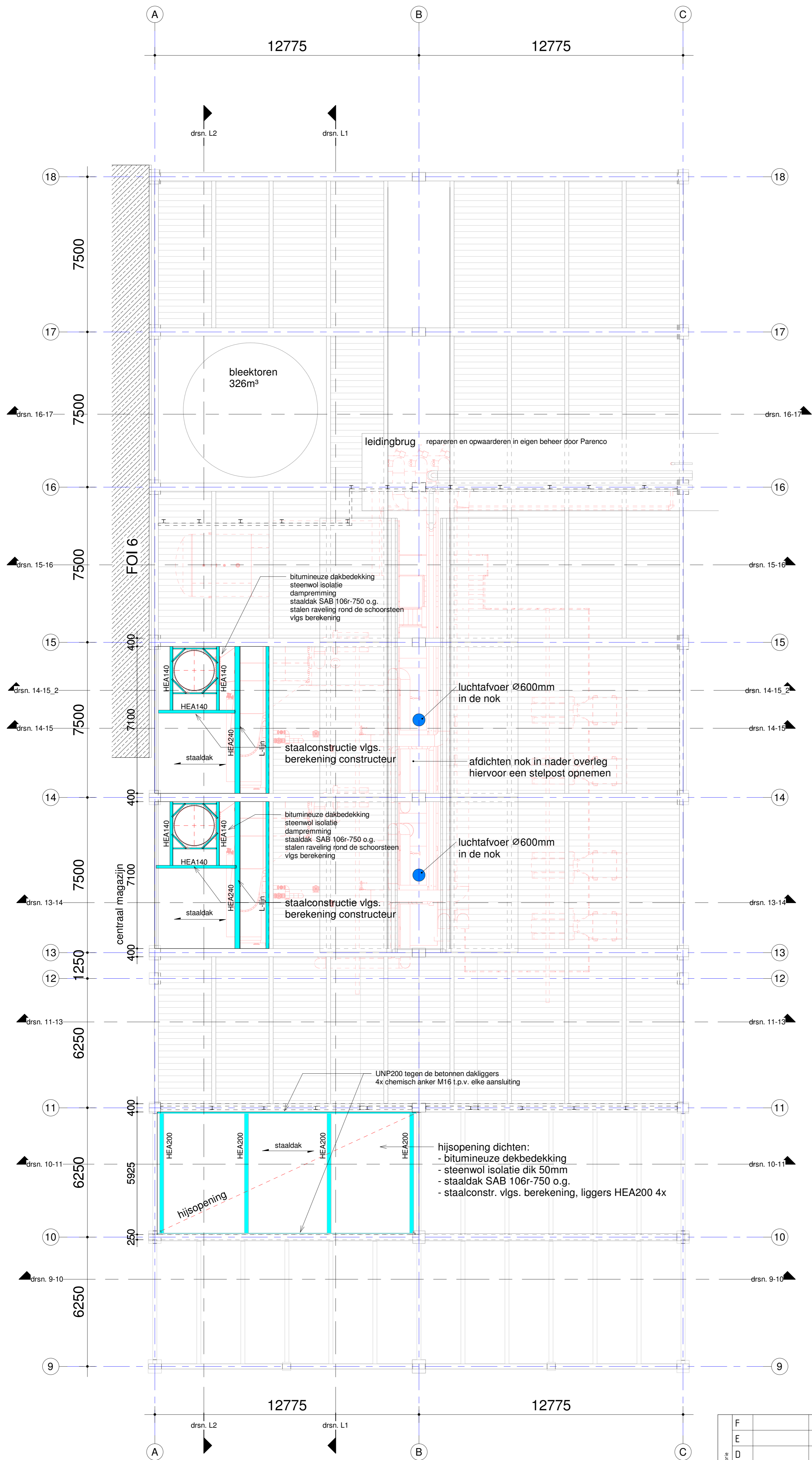
dakconstructie 1 : 100
