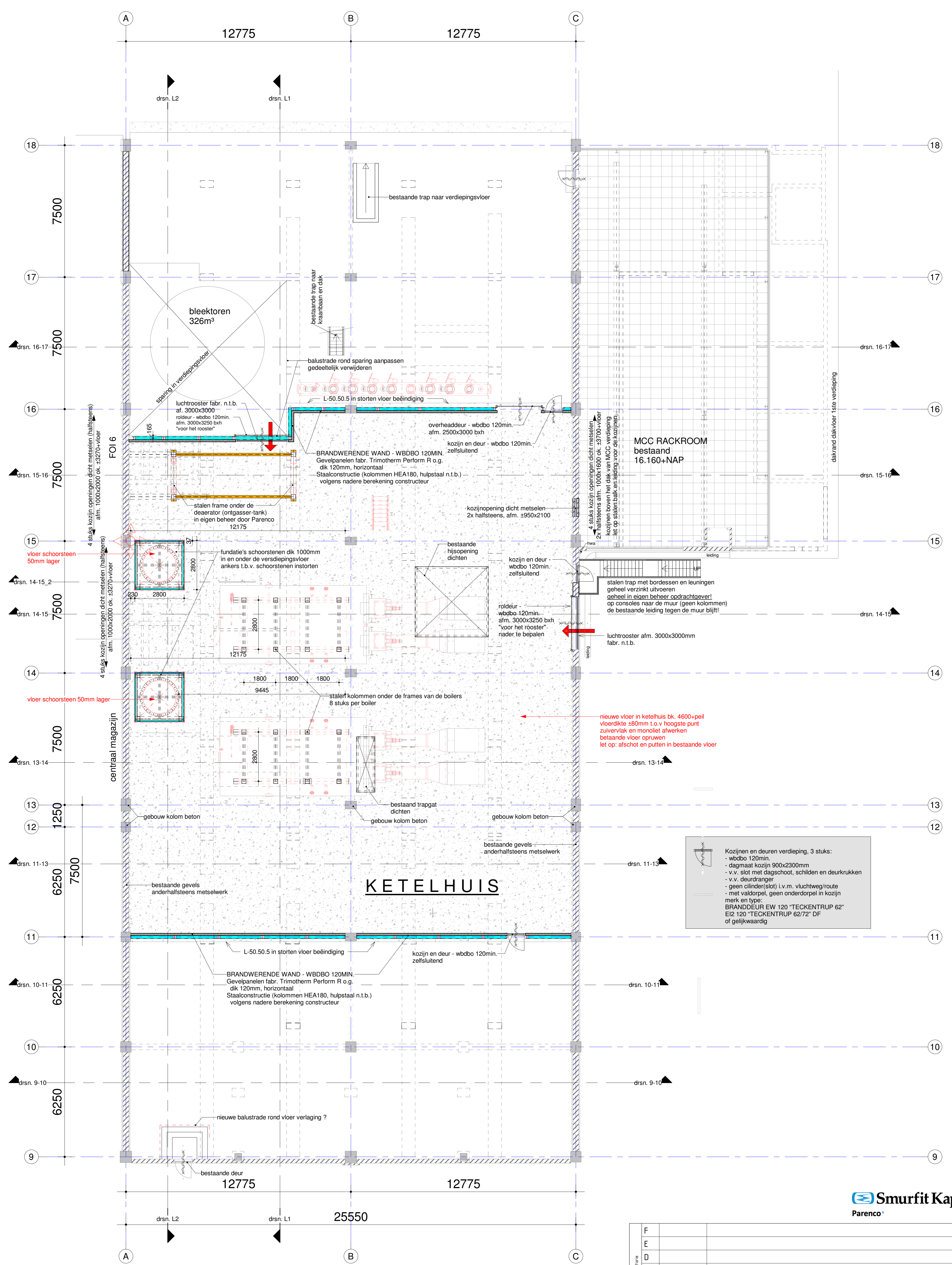
verdieping 15.750+NAP 1 : 100
