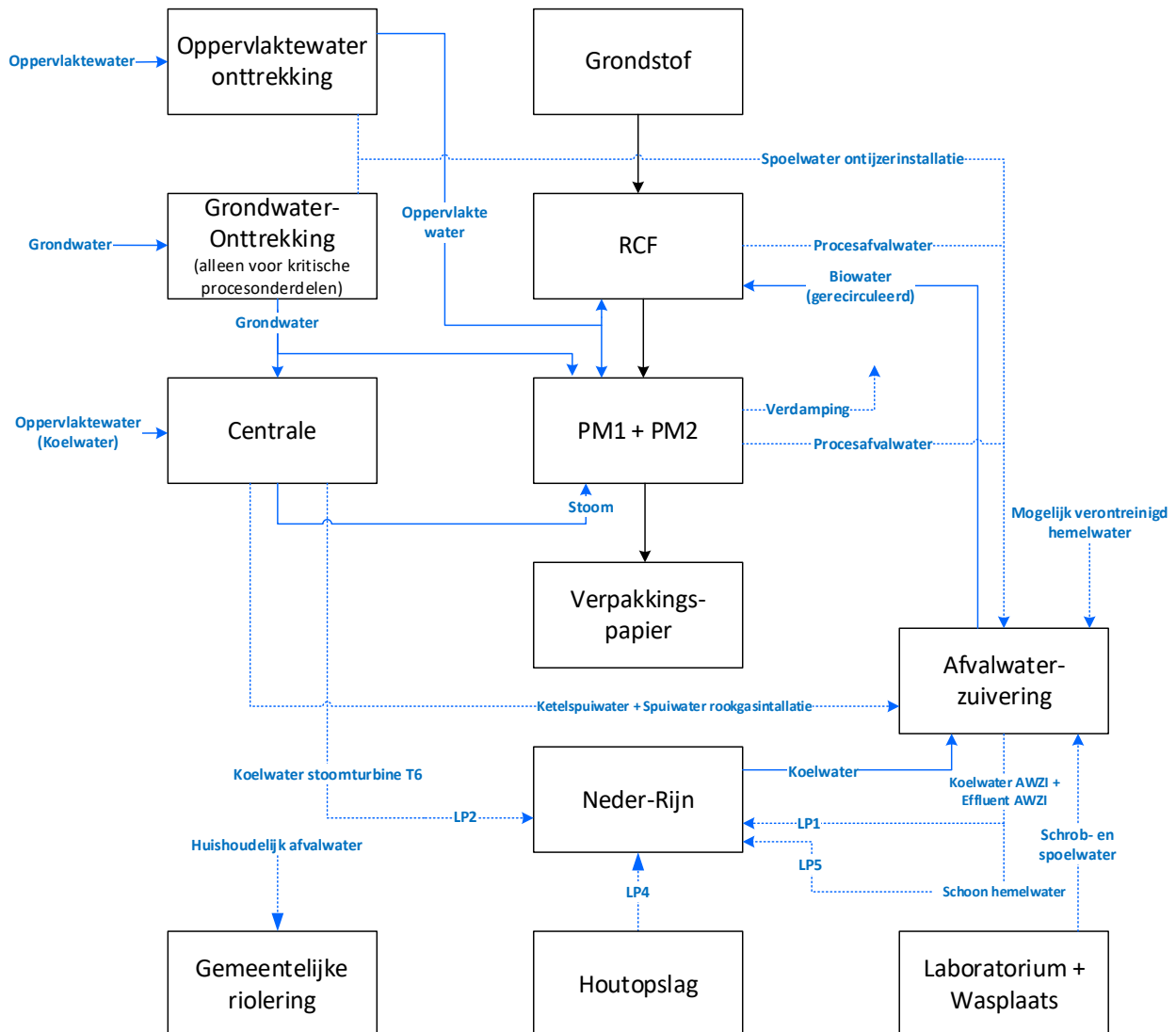
Figuur 3-3: Schematische weergave waterstromen SK Parenco alternatief 2 (100% verpakingspapier).
