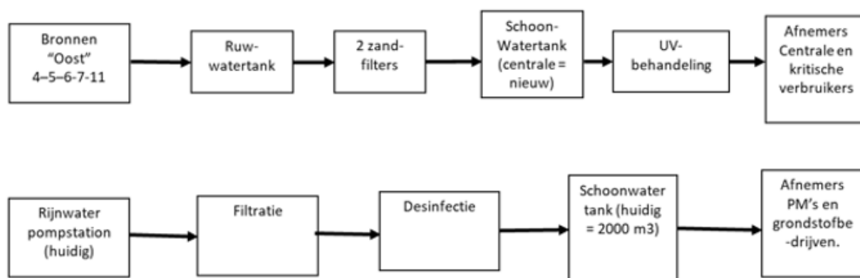
Figuur 3-4: Schema grondwater- en oppervlaktewatervoorziening bij volledige productie verpakkingspapier van SK Pirengo.
