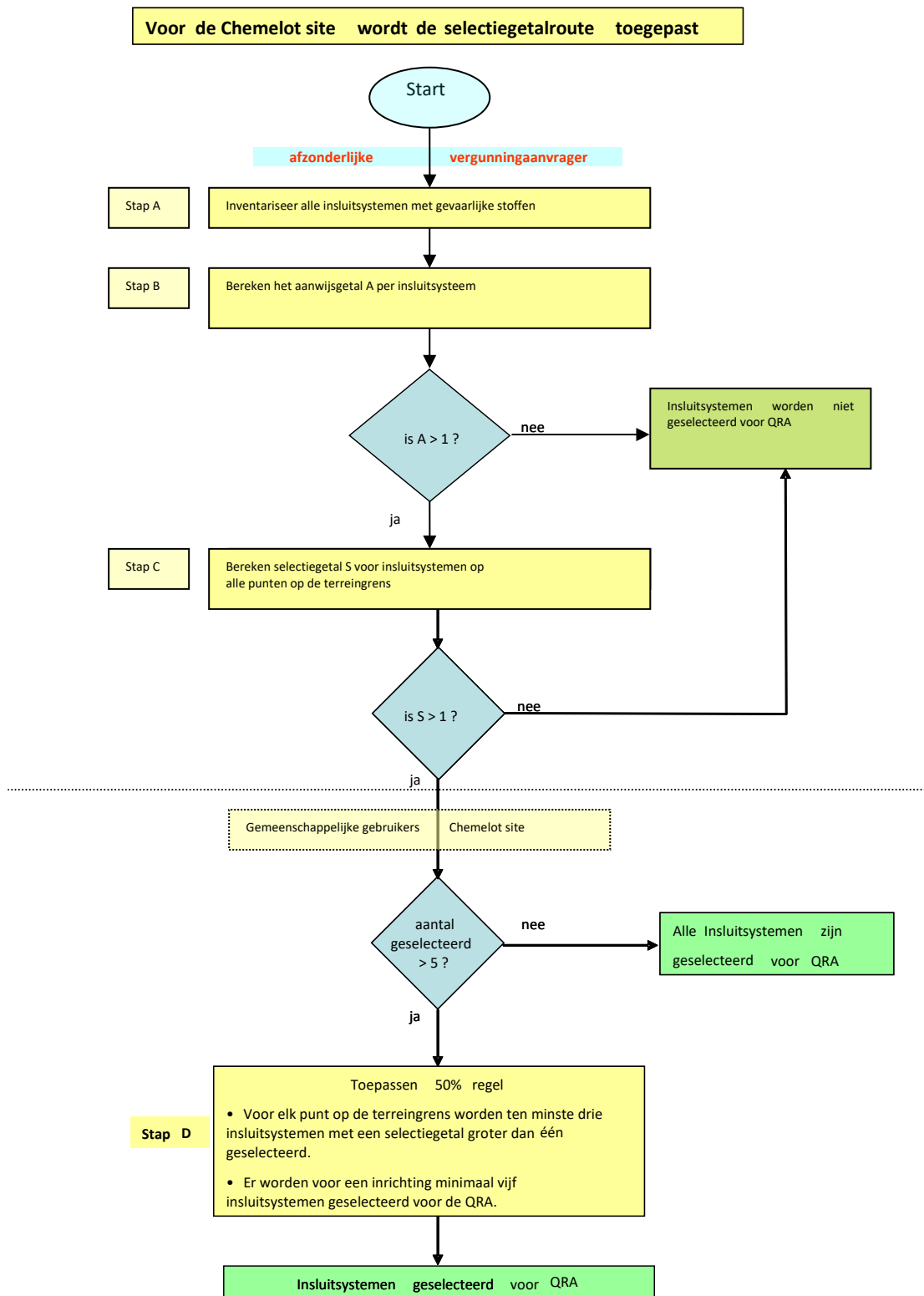
Figuur 2 : Schematische weergave selectieberekeningen site Chemelot
