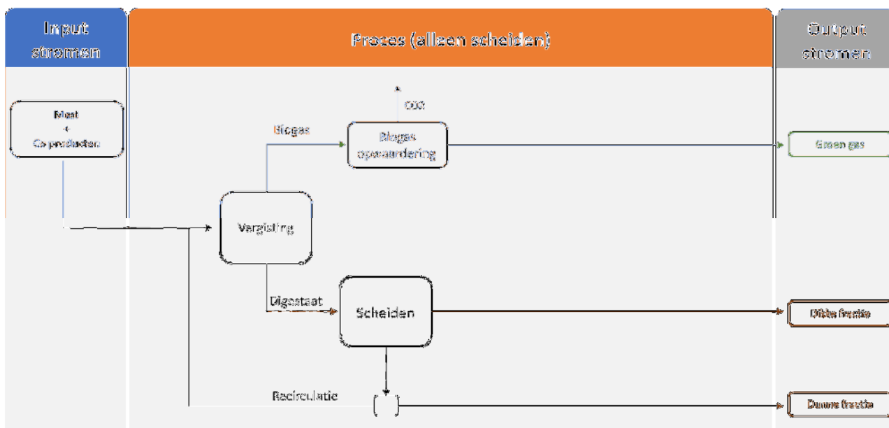
Figuur 18. Digestaat scheiden in dikke en dunne fracties
