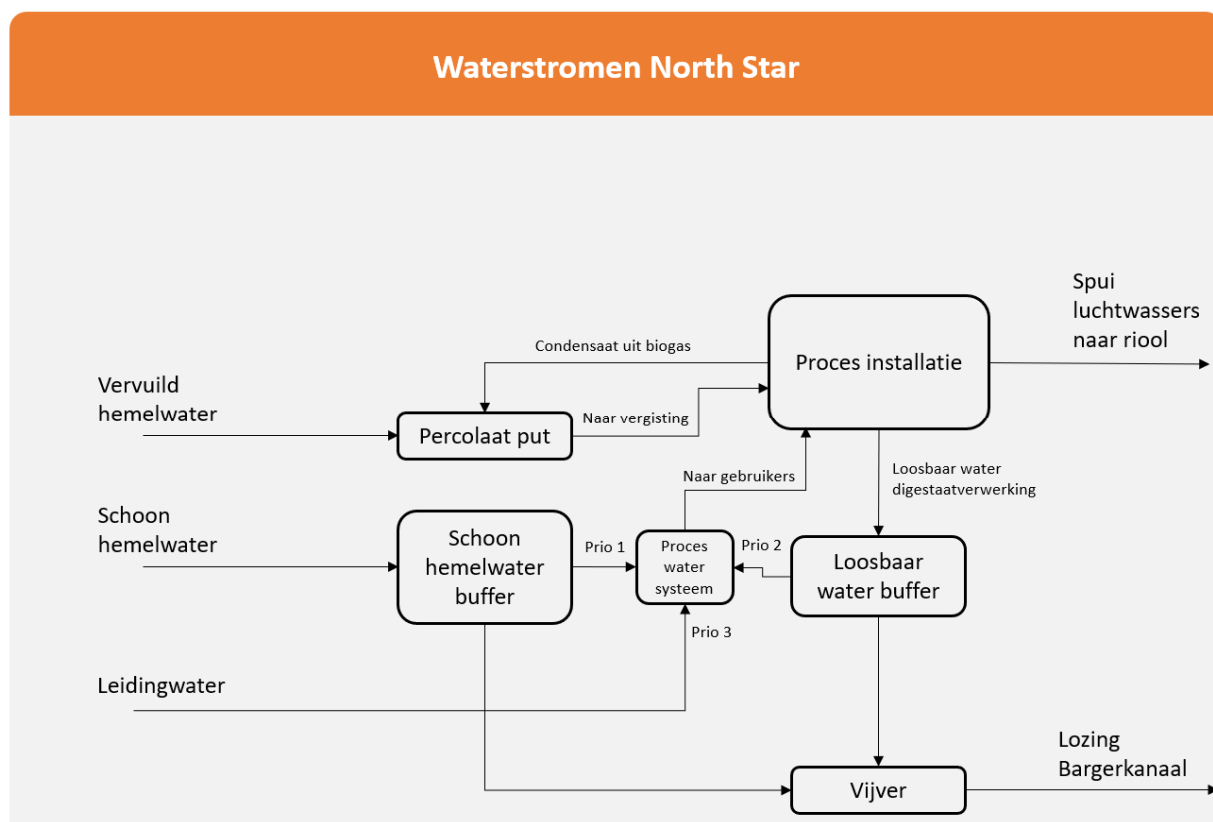
Figuur 27 schematische weergave water hergebruik en lozing
