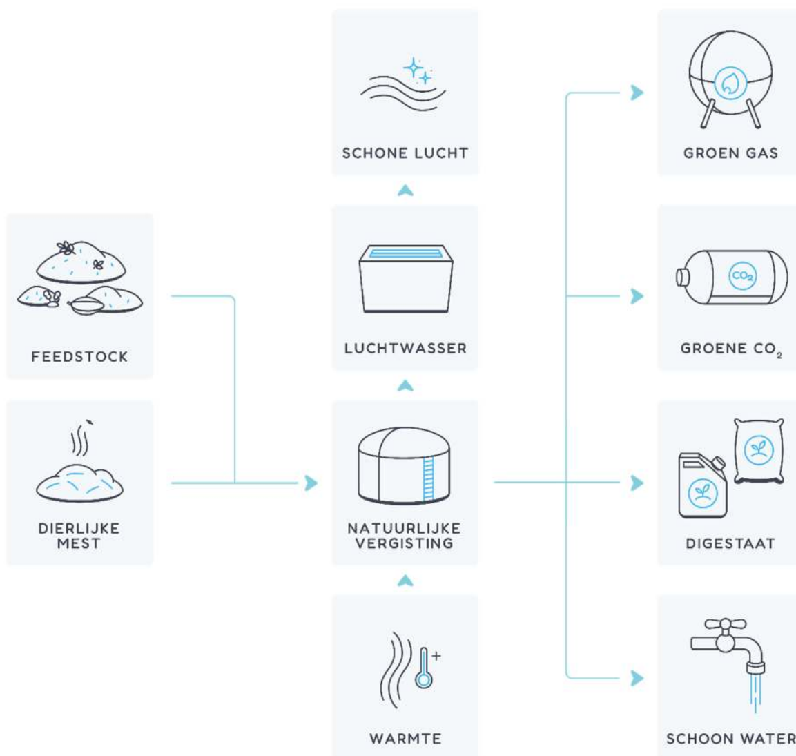
Afbeelding 1. Schematische weergave verwerkingsproces installatie.
