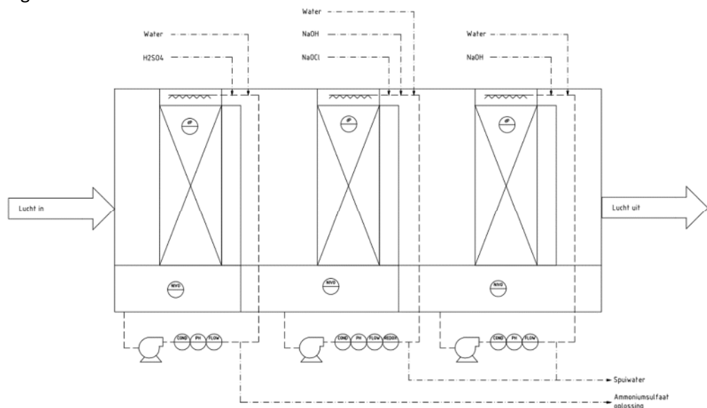
Figuur 12 principeschema 3 traps luchtwasser
