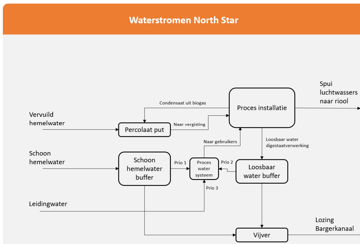
Afbeelding 6 schematische weergave water hergebruik en lozing
