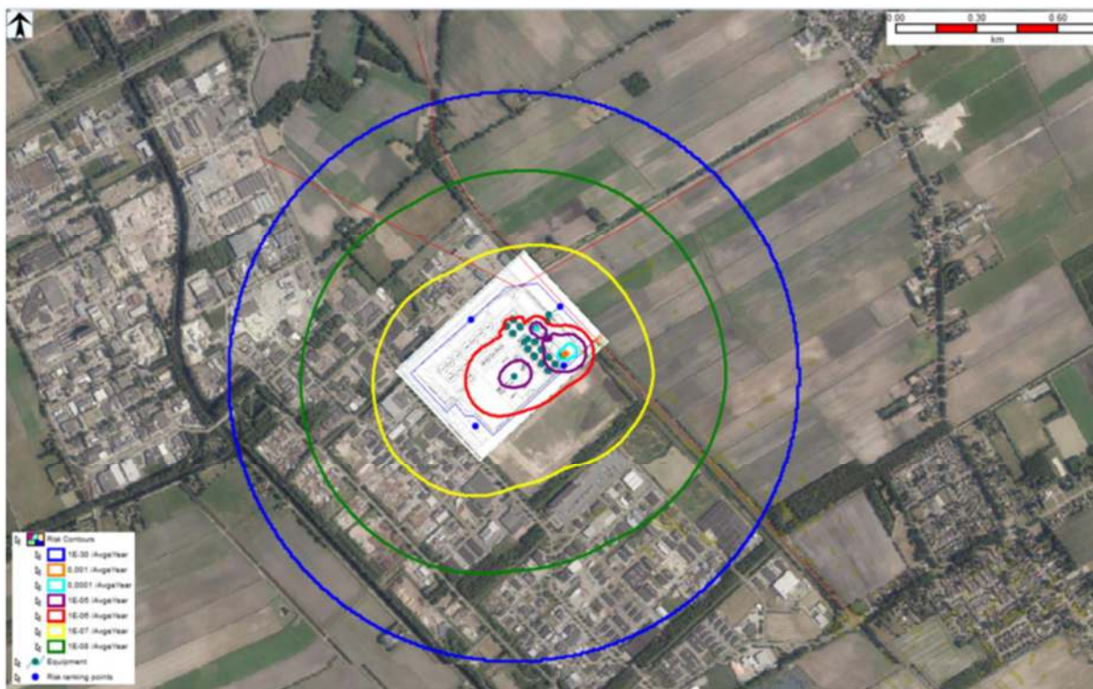
Figuur 24 Plaatsgebonden risicocontouren aangevraagde vergistingsinstallatie North Star in Emmen.
