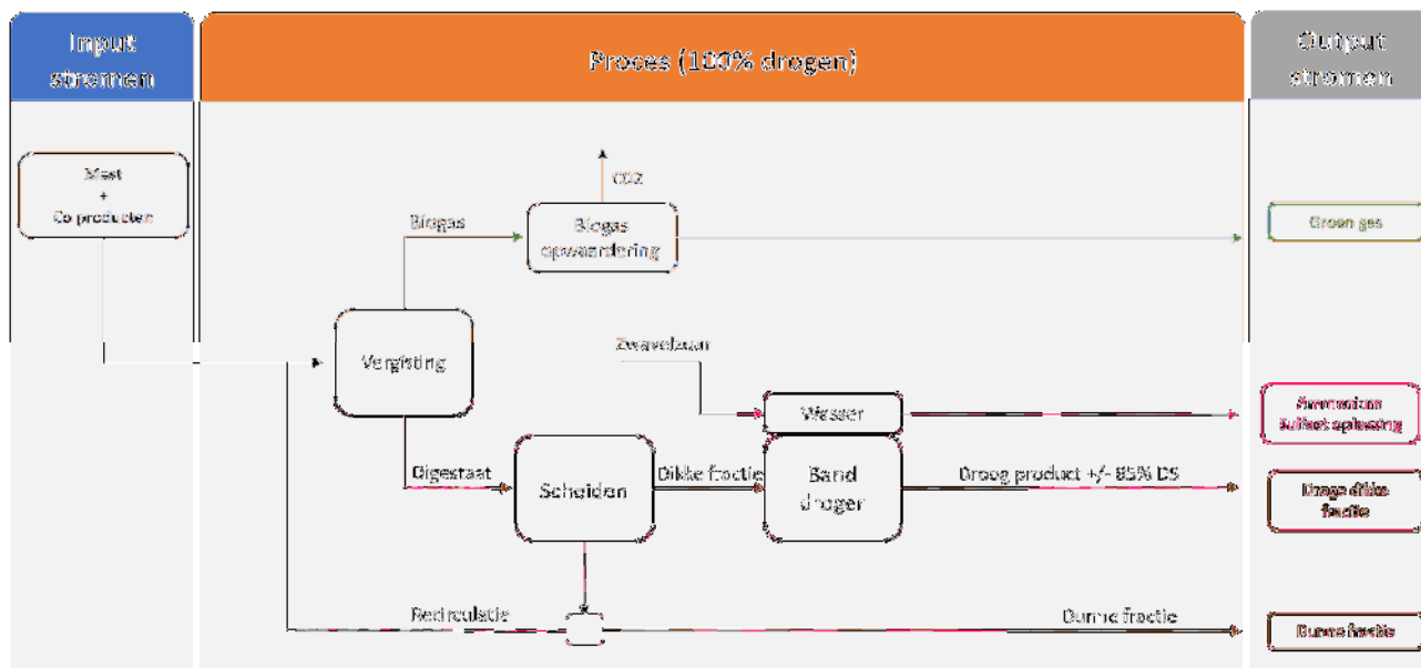
Figuur 19. Mechanisch drogen dikke fractie
