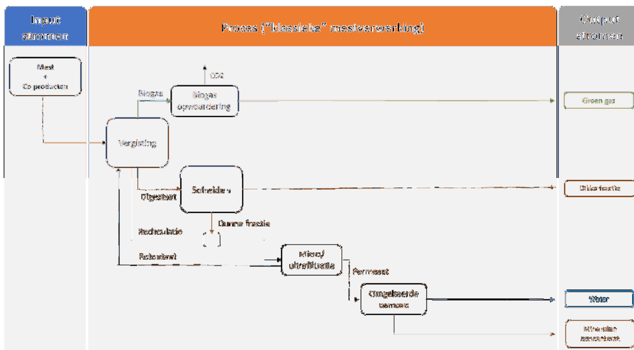
Figuur 23. Klassieke mestverwerking
