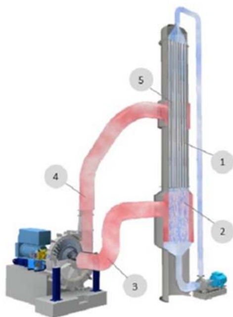
Figuur 11 valfilmverdamper
