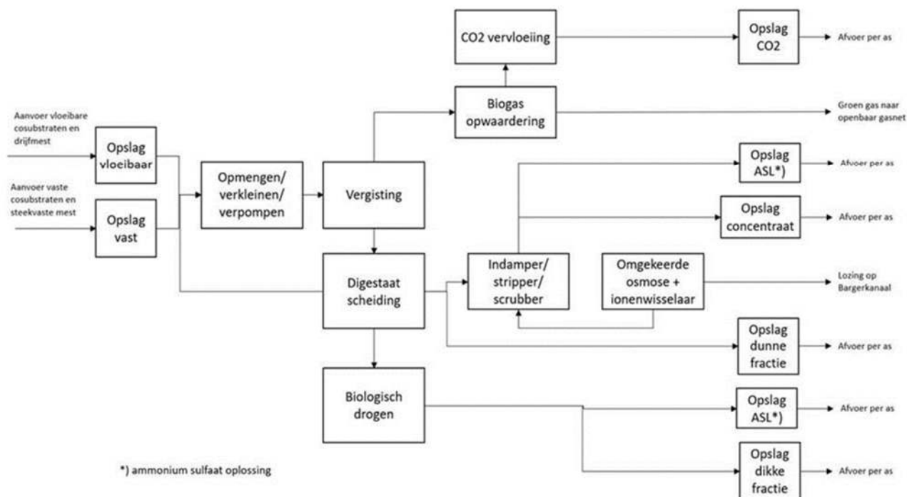
Figuur 25 procesflow installatie
