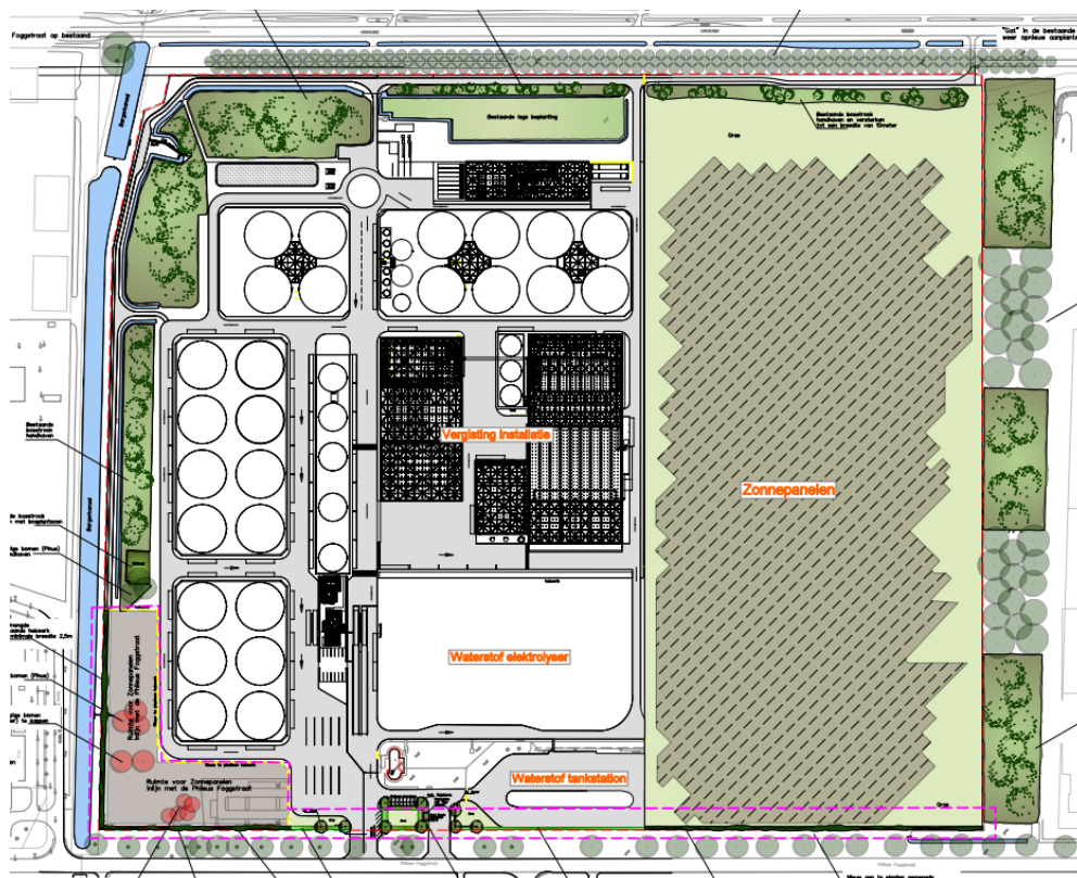
Figuur 2 De nieuwe situatie, waarin de vergistingsinstallatie wordt gebouwd.
