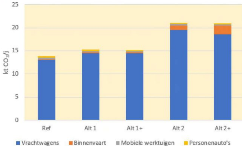
Figuur 5-3: CO 2 -emissie transporten per modaliteit
