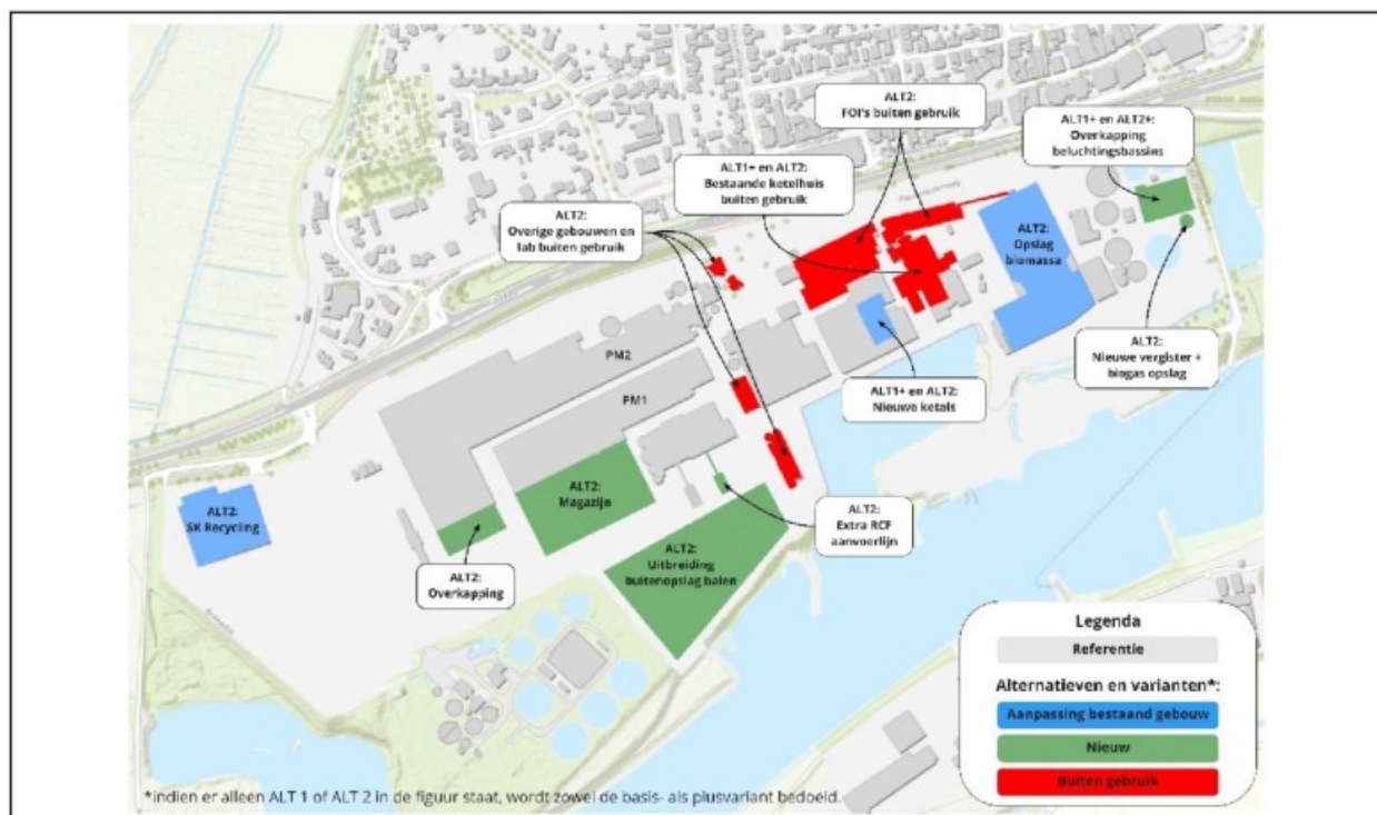
Figuur 2.1: Schematisch overzicht bedrijfsterrein SK Parencó met voor trillingen belangrijke productie-installaties
