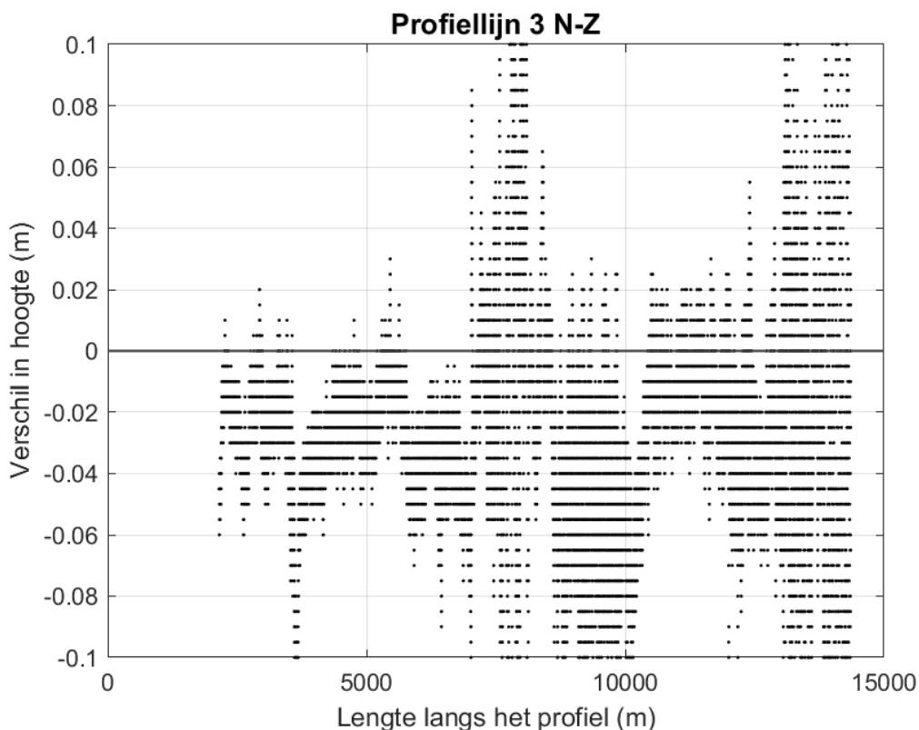
Figuur 4-37 Ingezoomde vershilplot langs profiellijn 3 van noord naar zuid voor de hoogte/diepte raai meetgegevens van januari 2019 en mei 2019. Een negatieve waarde betekent dat de hoogte/diepteraai van mei 2019 lager ligt dan de hoogte/diepteraai van januari 2019.
