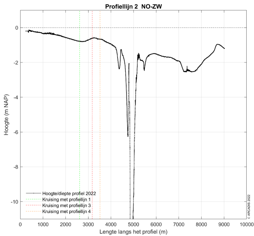
Figuur 3-54 Dwarsdoorsnede langs profiellijn 2 van noordoost naar zuidwest in 2021.
