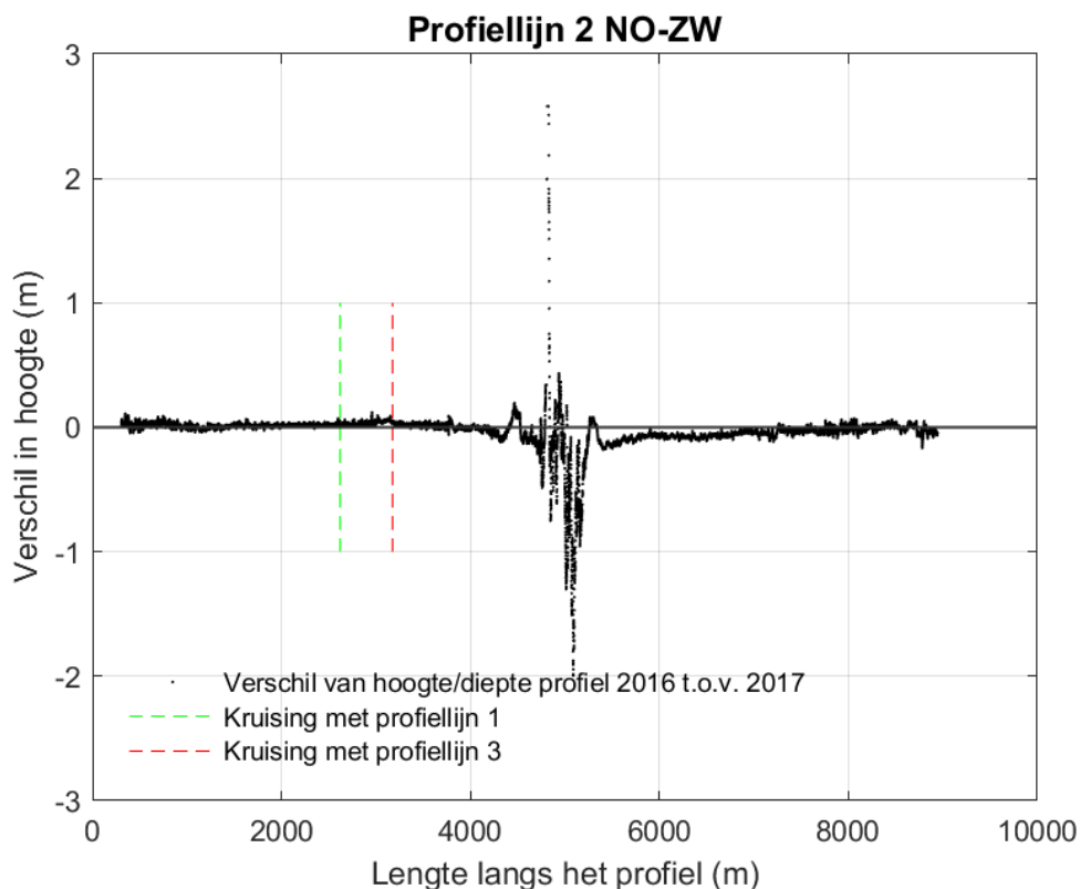
Figuur 4-6 Verschilplot langs profiellijn 2 van noordoost naar zuidwest voor de hoogte/diepte raai meetgegevens van 2016 en 2017. Een positieve waarde betekent dat de hoogte/diepteraai van 2017 hoger ligt dan de hoogte/diepteraai van 2016.
