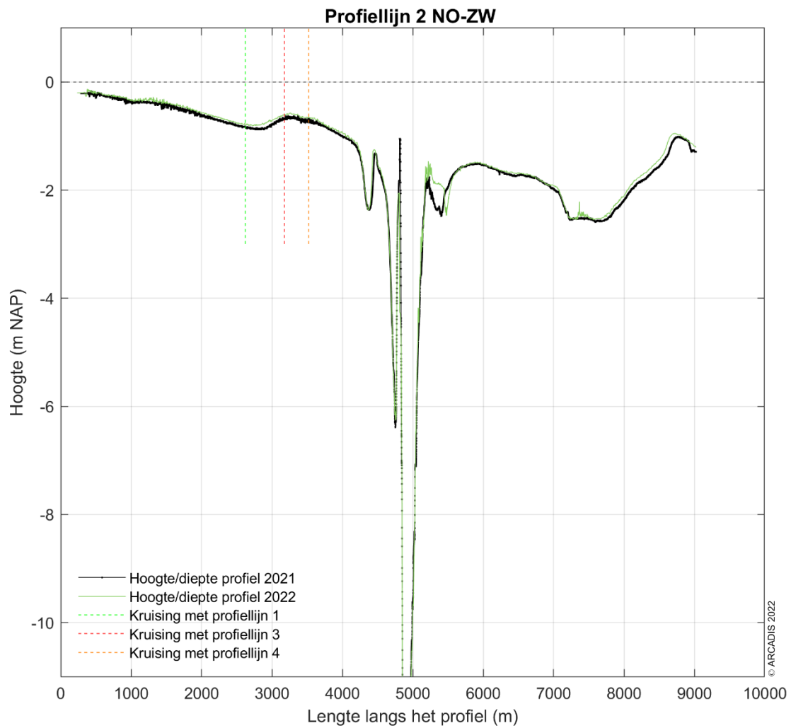
Figuur 4-59 Dwarsdoorsnede langs profiellijn 2 van noordoost naar zuidwest voor de hoogte/diepte raai meetgegevens van 2021 en 2022.
