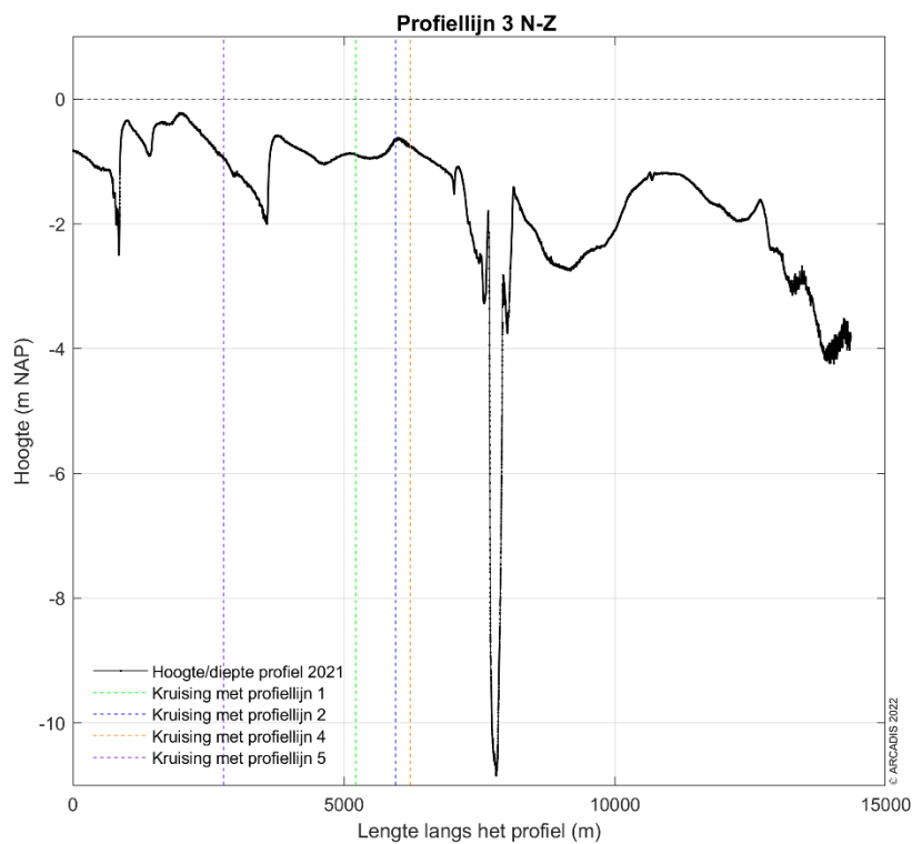
Figuur 3-41 Dwarsdoorsnede langs profiellijn 3 van noord naar zuid in 2021.
