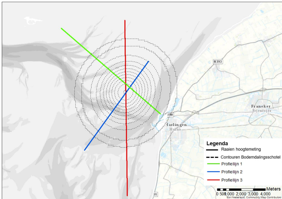
Figuur 2-2 Kaart van de hoogte/diepte raaien die jaarlijks zijn gemeten tussen 2016 - 2020.
