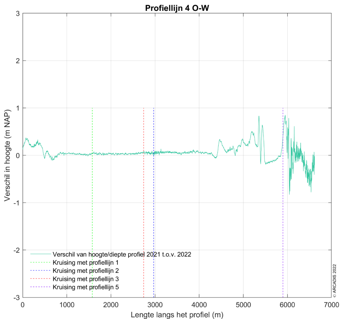
Figuur 5-12 Vershilplot langs profiellijn 4 van noord naar zuid voor de hoogte/diepte raai meetgegevens tussen 2016 t.o.v. 2017, 2017 t.o.v. 2018, 2018 t.o.v. 2019, 2019 t.o.v. 2020, 2020 t.o.v. 2021 en 2021 t.o.v. 2022. Een positieve waarde betekent dat de hoogte/diepteraai van het opvolgende jaar hoger ligt dan de hoogte/diepteraai van het eerdere jaar.
