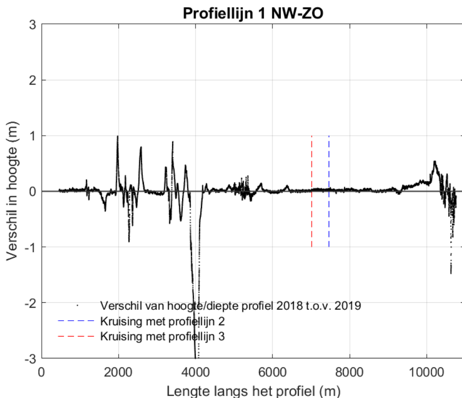
Figuur 4-21 Verschilplot langs profiellijn 1 van noordwest naar zuidoost voor de hoogte/diepte raai meetgegevens van 2018 en mei 2019. Een positieve waarde betekent dat de hoogte/diepteraai van mei 2019 hoger ligt dan de hoogte/diepteraai van 2018.
