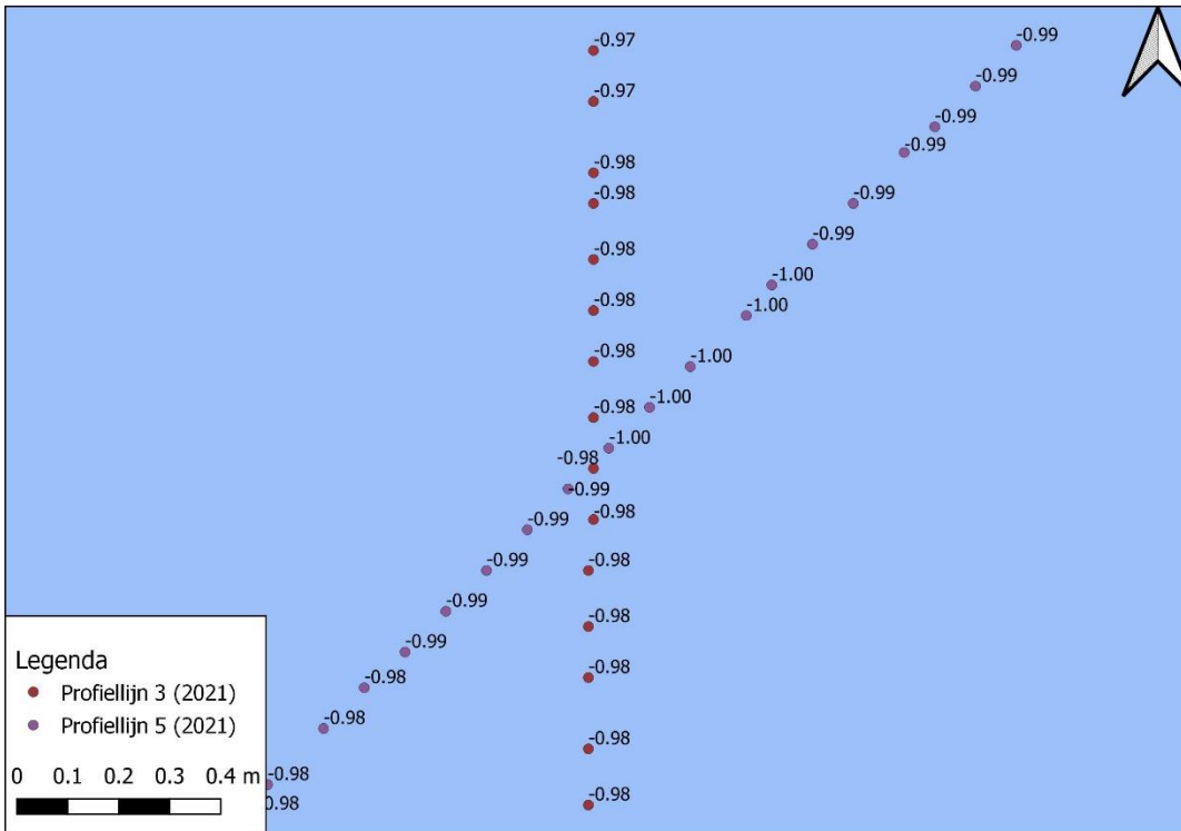
Figuur 3-51 Detailkaart controlepunt tussen profiellijn 3 en profiellijn 5 voor de hoogte/diepte raaien mei 2021, hoogtemetingen zijn weergegeven in m NAP.
