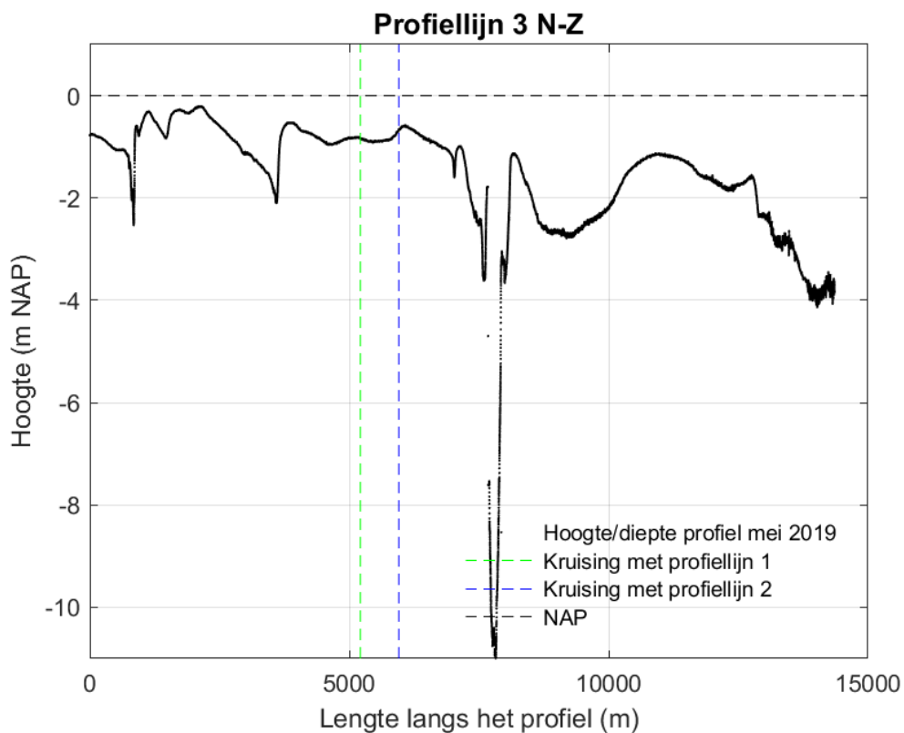
Figuur 3-29 Dwarsdoorsnede langs profiellijn 3 van noord naar zuid in mei 2019.
