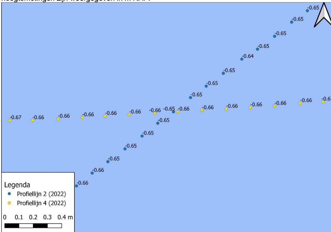
Figuur 3-63 Detailkaart controlepunt tussen profiellijn 2 en profiellijn 4 voor de hoogte/diepte raaien mei 2022, hoogtemetingen zijn weergegeven in m NAP.
