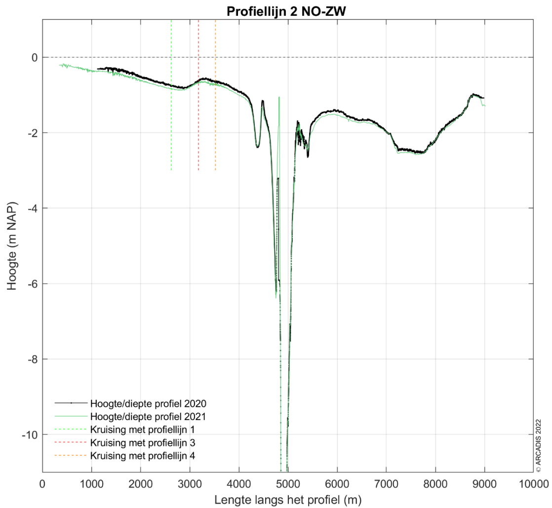
Figuur 4-50 Dwarsdoorsnede langs profiellijn 2 van noordoost naar zuidwest voor de hoogte/diepte raai meetgegevens van 2020 en 2021.
