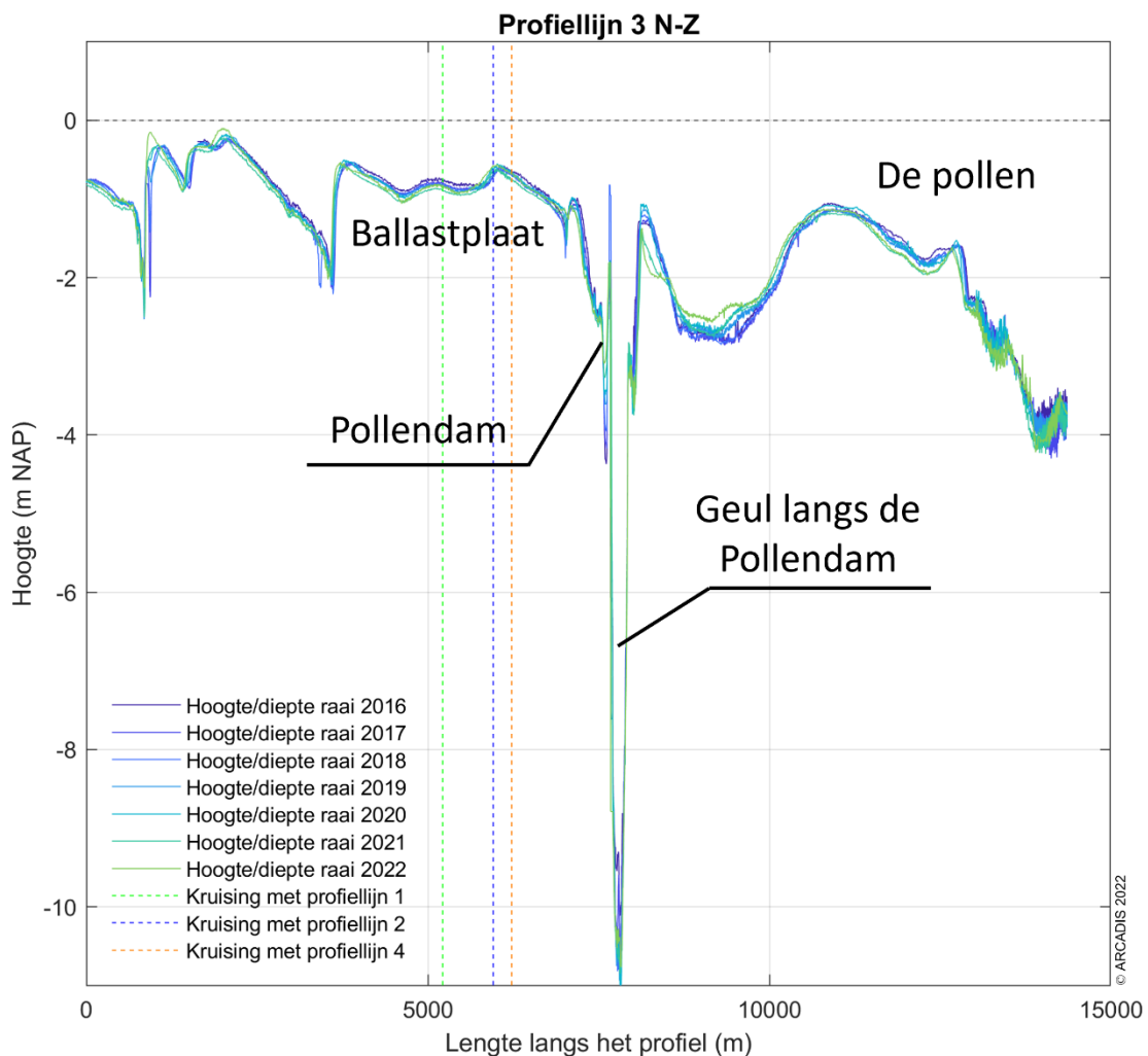
Figuur 5-7 Dwarsprofiel langs profiellijn 3 van noord naar zuid voor de hoogte/diepte raai meetgegevens van 2016 - 2022.
