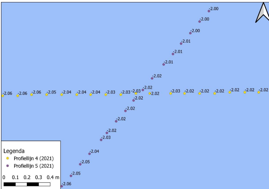
Figuur 3-52 Detailkaart controlepunt tussen profiellijn 4 en profiellijn 5 voor de hoogte/diepte raaien mei 2021, hoogtemetingen zijn weergegeven in m NAP.
