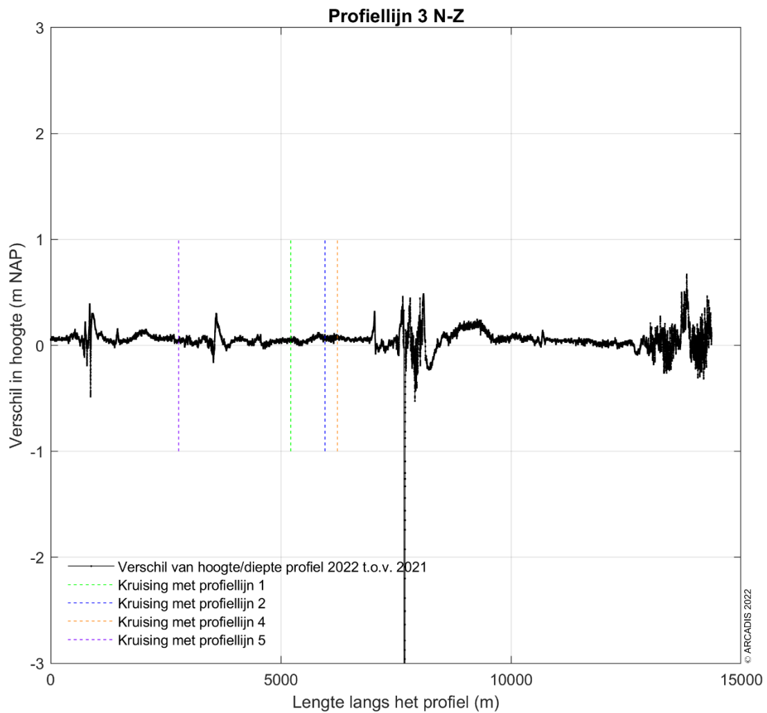
Figuur 4-63 Verschilplot langs profiellijn 3 van noord naar zuid voor de hoogte/diepte raai meetgegevens van 2021 en 2022. Een positieve waarde betekent dat de hoogte/diepteraai van mei 2022 hoger ligt dan de hoogte/diepteraai van 2021.
