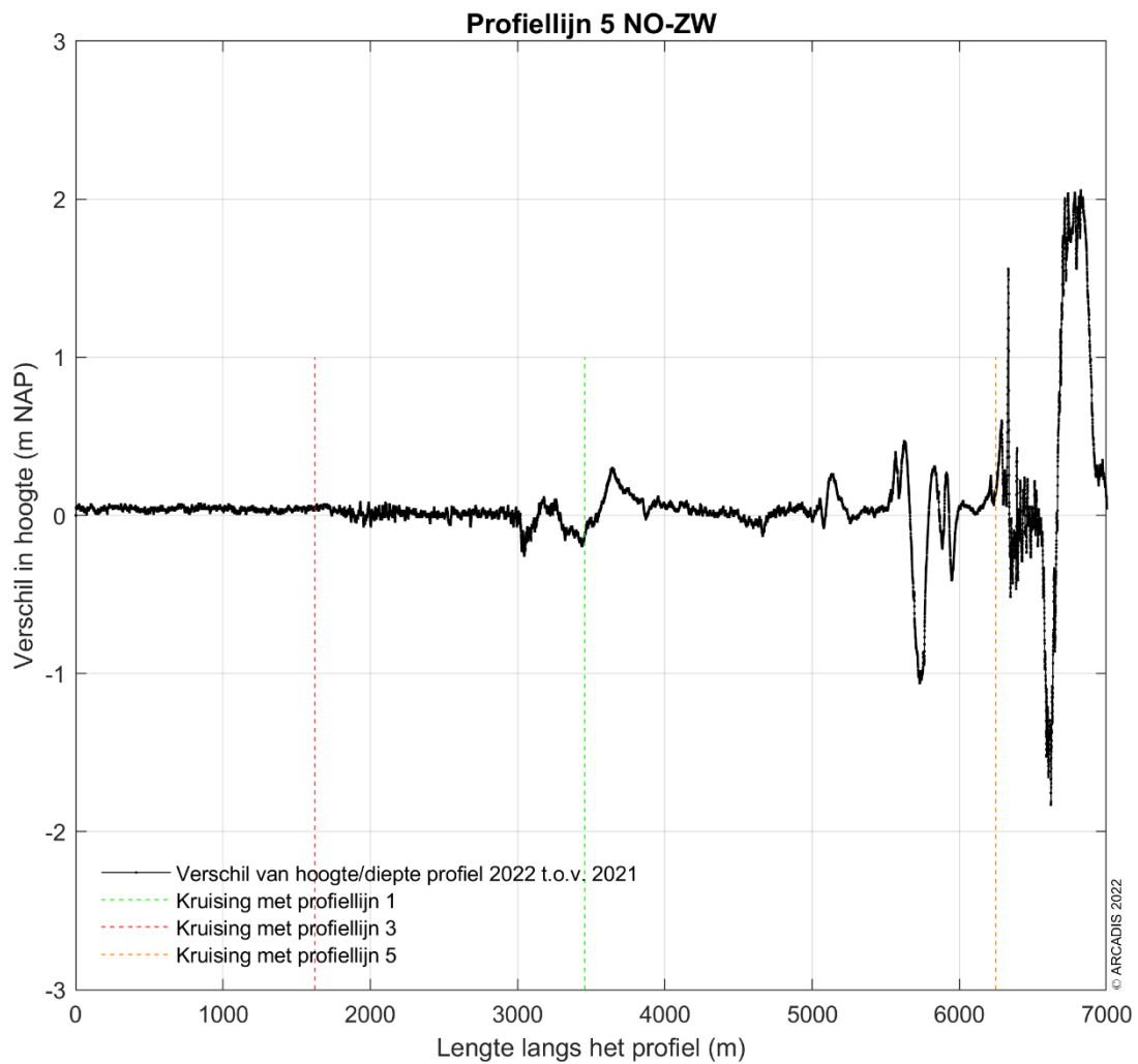
Figuur 4-69 Verschilplot langs profiellijn 5 van noordoost naar zuidwest voor de hoogte/diepte raai meetgegevens van 2021 en 2022. Een positieve waarde betekent dat de hoogte/diepteraai van mei 2022 hoger ligt dan de hoogte/diepteraai van 2021.
