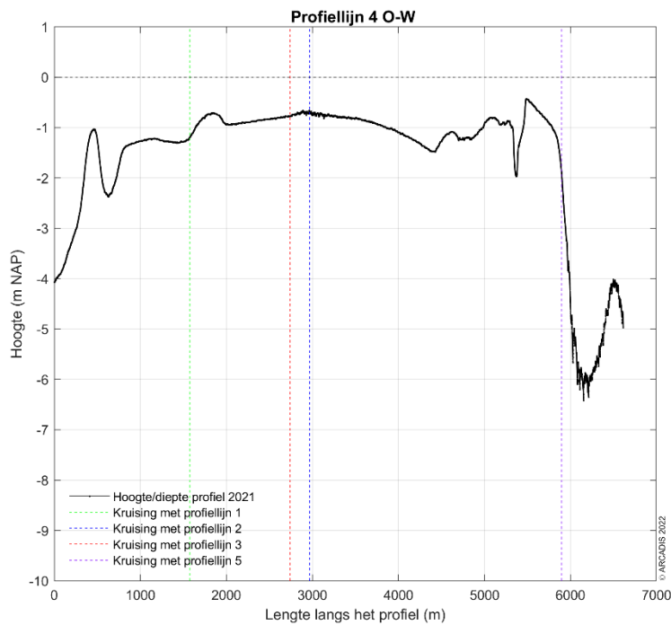
Figuur 3-42 Dwarsdoorsnede langs profiellijn 4 van oost naar west in 2021.
