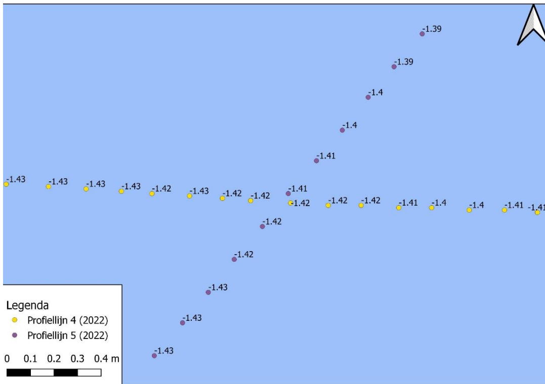
Figuur 3-66 Detailkaart controlepunt tussen profiellijn 4 en profiellijn 5 voor de hoogte/diepte raaien mei 2022, hoogtemetingen zijn weergegeven in m NAP.
