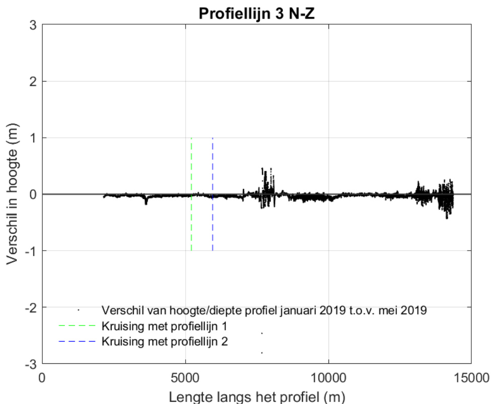
Figuur 4-36 Vershilplot langs profiellijn 3 van noord naar zuid voor de hoogte/diepte raai meetgegevens van januari 2019 en mei 2019. Een negatieve waarde betekent dat de hoogte/diepteraai van mei 2019 lager ligt dan de hoogte/diepteraai van januari 2019.
