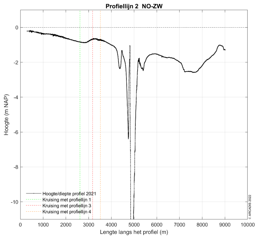
Figuur 3-40 Dwarsdoorsnede langs profiellijn 2 van noordoost naar zuidwest in 2021.
