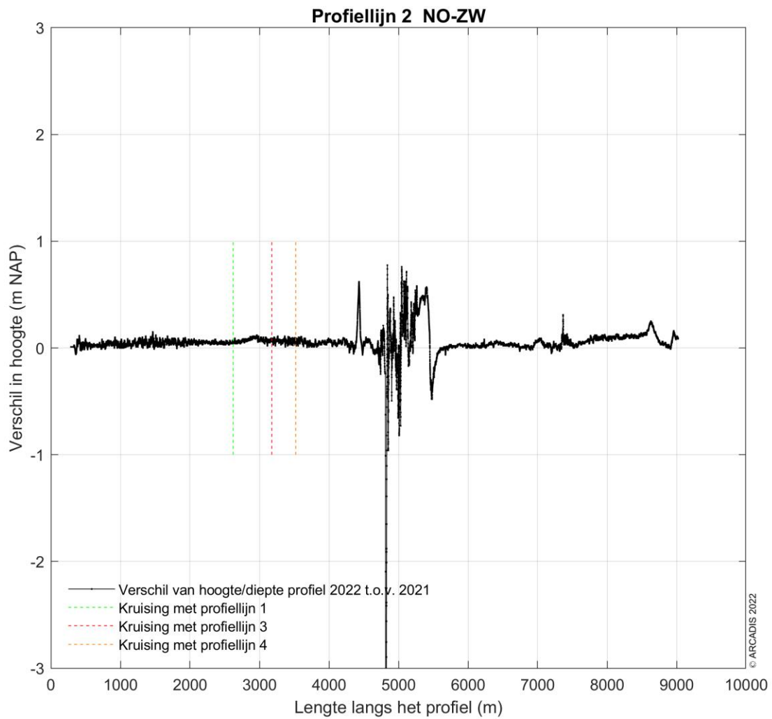
Figuur 4-60 Verschilplot langs profiellijn 2 van noordoost naar zuidwest voor de hoogte/diepte raai meetgegevens van 2021 en 2022. Een positieve waarde betekent dat de hoogte/diepteraai van mei 2022 hoger ligt dan de hoogte/diepteraai van 2021.
