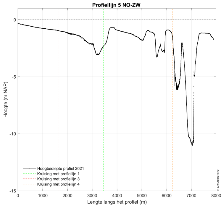
Figuur 3-43 Dwarsdoorsnede langs profiellijn 5 van noordoost naar zuidwest in 2021.
