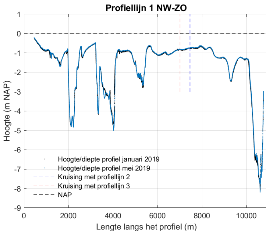
Figuur 4-29 Dwarsdoorsnede langs profiellijn 1 van noordwest naar zuidoost voor de hoogte/diepte raai meetgegevens van januari 2019 en mei 2019.
