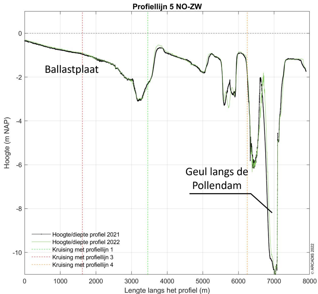
Figuur 5-13 Dwarsprofiel langs profiellijn 5 van noord naar zuid voor de hoogte/diepte raai meetgegevens van 2016 - 2022.
