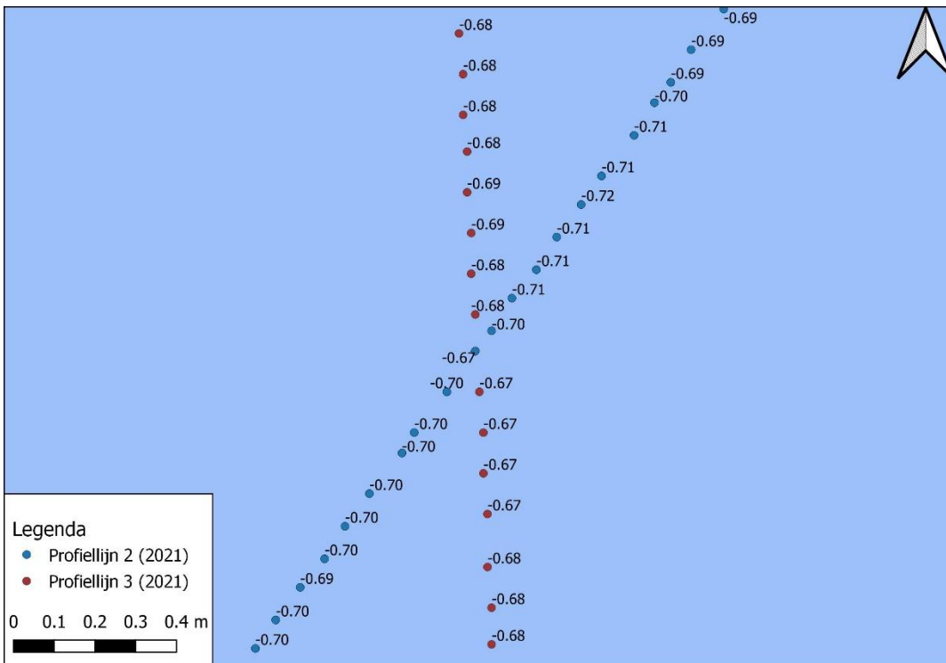
Figuur 3-48 Detailkaart controlepunt tussen profiellijn 2 en profiellijn 3 voor de hoogte/diepte raaien mei 2021, hoogtemetingen zijn weergegeven in m NAP.
