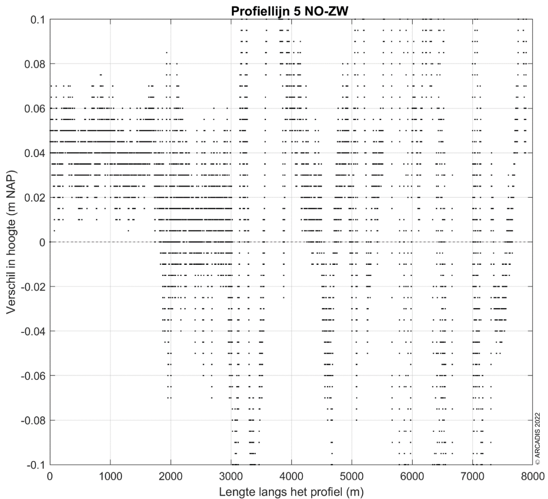
Figuur 4-70: Ingezoomde verschilplot langs profiellijn 5 van noordoost naar zuidwest voor de hoogte/diepte raai meetgegevens van 2021 en 2022. Een positieve waarde betekent dat de hoogte/diepteraai van 2022 hoger ligt dan de hoogte/diepteraai van 2021.
