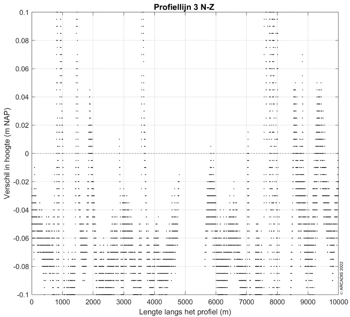
Figuur 4-55: Ingezoomde verschilplot langs profiellijn 3 van noord naar zuid voor de hoogte/diepte raai meetgegevens van 2020 en 2021. Een positieve waarde betekent dat de hoogte/diepteraai van 2021 hoger ligt dan de hoogte/diepteraai van 2020.
