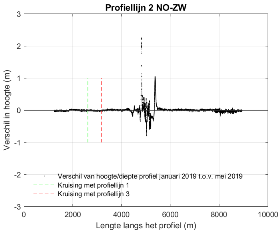
Figuur 4-33 Verschilplot langs profiellijn 2 van noordoost naar zuidwest voor de hoogte/diepte raai meetgegevens van januari 2019 en mei 2019. Een positieve waarde betekent dat de hoogte/diepteraai van mei 2019 hoger ligt dan de hoogte/diepteraai van januari 2019.
