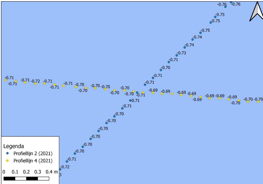
Figuur 3-49 Detailkaart controlepunt tussen profiellijn 2 en profiellijn 4 voor de hoogte/diepte raaien mei 2021, hoogtemetingen zijn weergegeven in m NAP.
