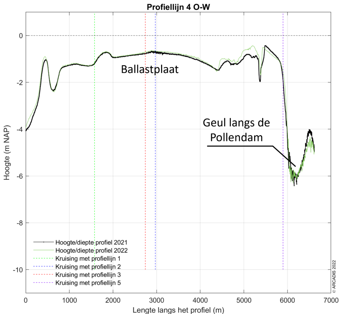
Figuur 5-10 Dwarsprofiel langs profiellijn 4 van noord naar zuid voor de hoogte/diepte raai meetgegevens van 2016 - 2022.
