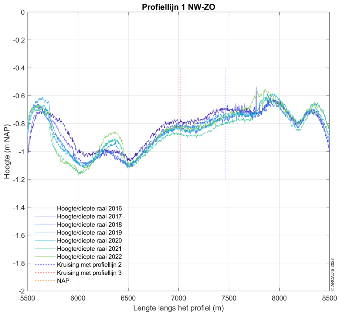
Figuur 5-2 Ingezoomd dwarsprofiel van de Ballastplaat langs profiellijn 2 van noordwest naar zuidoost voor de hoogte/diepte raai meetgegevens van 2016 -2022 (Detail van Figuur 5-1).
