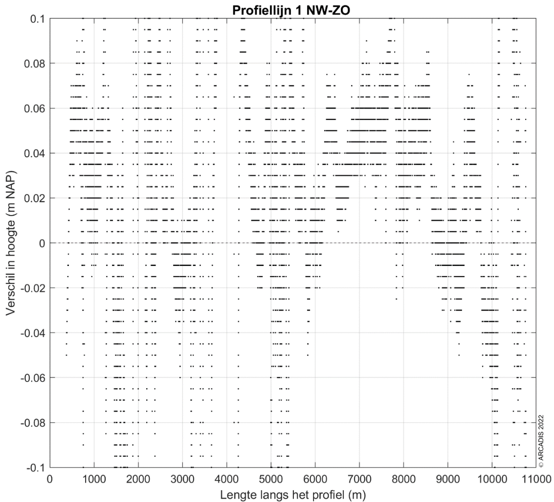
Figuur 4-58 Ingezoomde verschilplot langs profiellijn 1 van noordwest naar zuidoost voor de hoogte/diepte raai meetgegevens van 2021 en 2022. Een positieve waarde betekent dat de hoogte/diepteraai van 2022 hoger ligt dan de hoogte/diepteraai van 2021.
