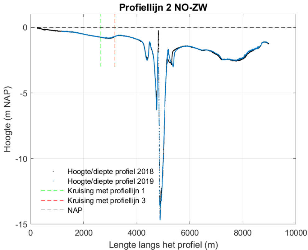
Figuur 4-23 Dwarsdoorsnede langs profiellijn 2 van noordoost naar zuidwest voor de hoogte/diepte raai meetgegevens van 2018 en mei 2019.
