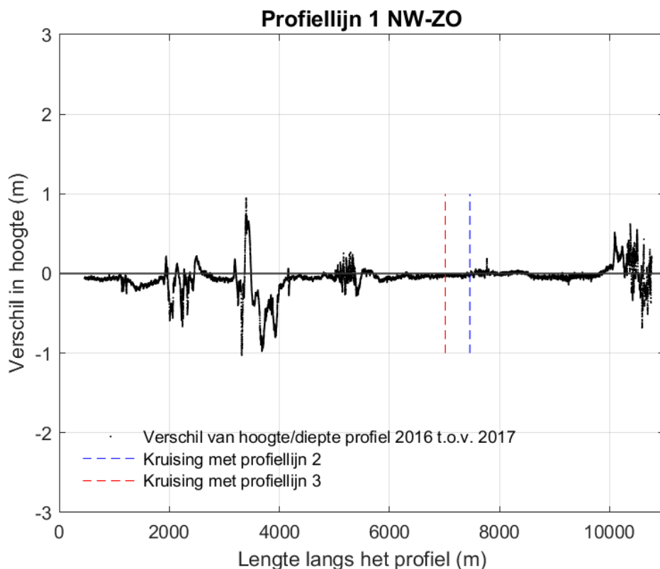
Figuur 4-3 Verschilplot langs profiellijn 1 van noordwest naar zuidoost voor de hoogte/diepte raai meetgegevens van 2016 en 2017. Een negatieve waarde betekent dat de hoogte/diepteraai van 2017 lager ligt dan de hoogte/diepteraai van 2016.
