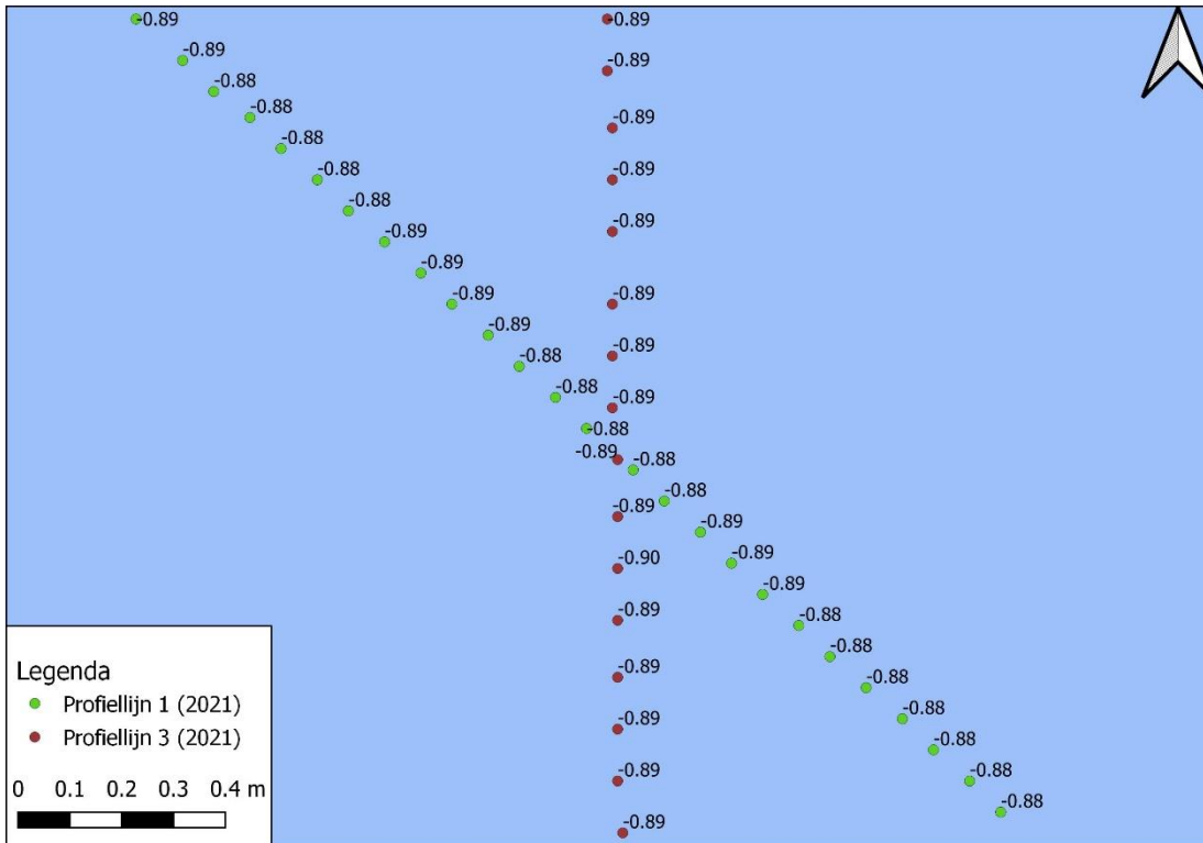
Figuur 3-45 Detailkaart controlepunt tussen profiellijn 1 en profiellijn 3 voor de hoogte/diepte raaien 2021, hoogtemetingen zijn weergegeven in m NAP.
