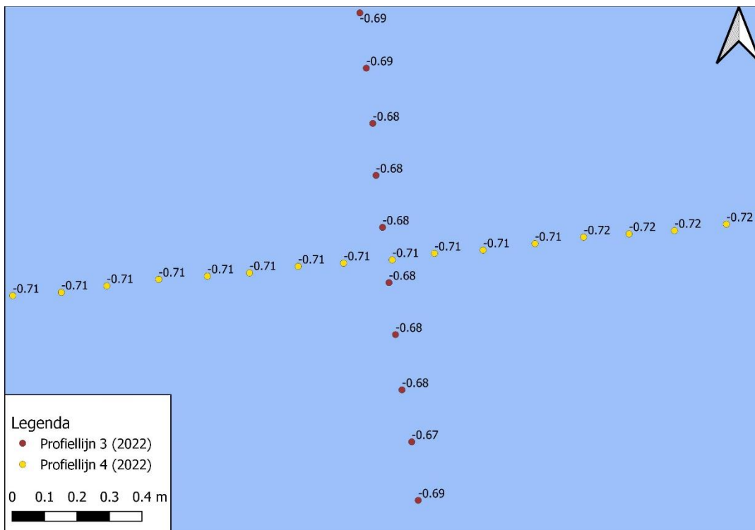
Figuur 3-64 Detailkaart controlepunt tussen profiellijn 3 en profiellijn 4 voor de hoogte/diepte raaien mei 2022, hoogtemetingen zijn weergegeven in m NAP.
