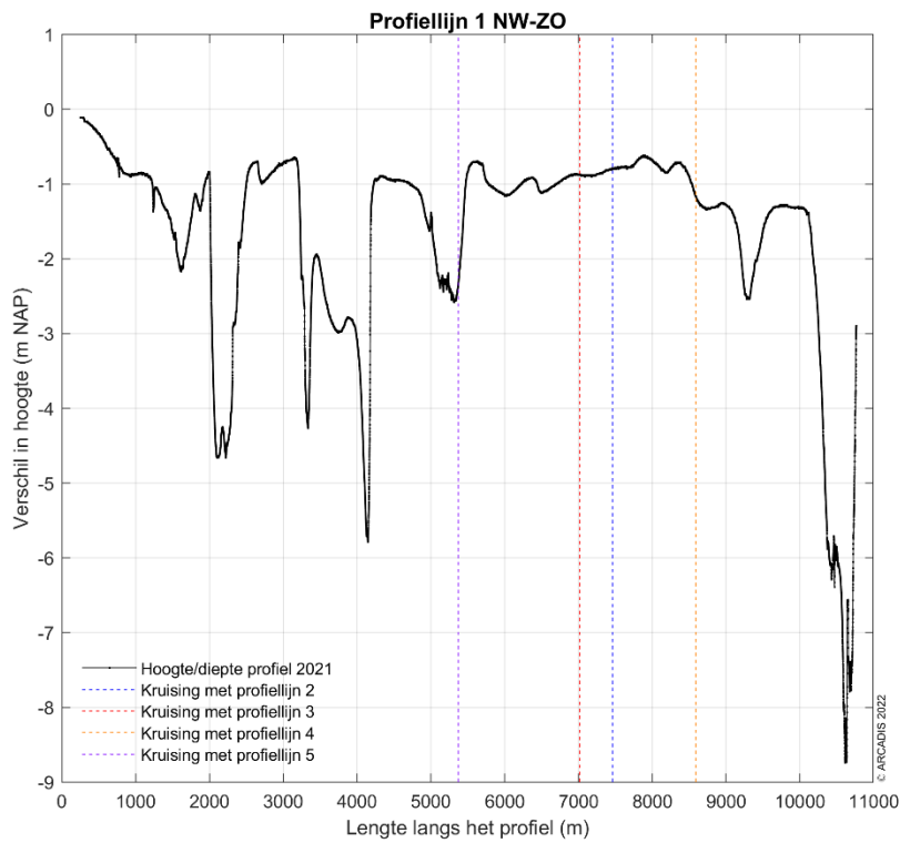
Figuur 3-39 Dwarsdoorsnede langs profiellijn 1 van noordwest naar zuidoost in 2021.
