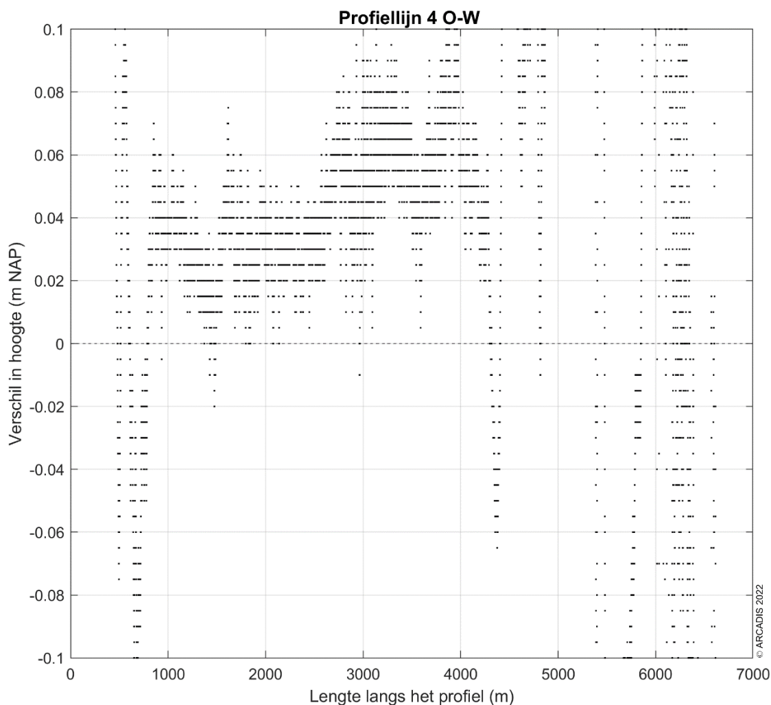
Figuur 4-67: Ingezoomde verschilplot langs profiellijn 4 van oost naar west voor de hoogte/diepte raai meetgegevens van 2021 en 2022. Een positieve waarde betekent dat de hoogte/diepteraai van 2022 hoger ligt dan de hoogte/diepteraai van 2021.
