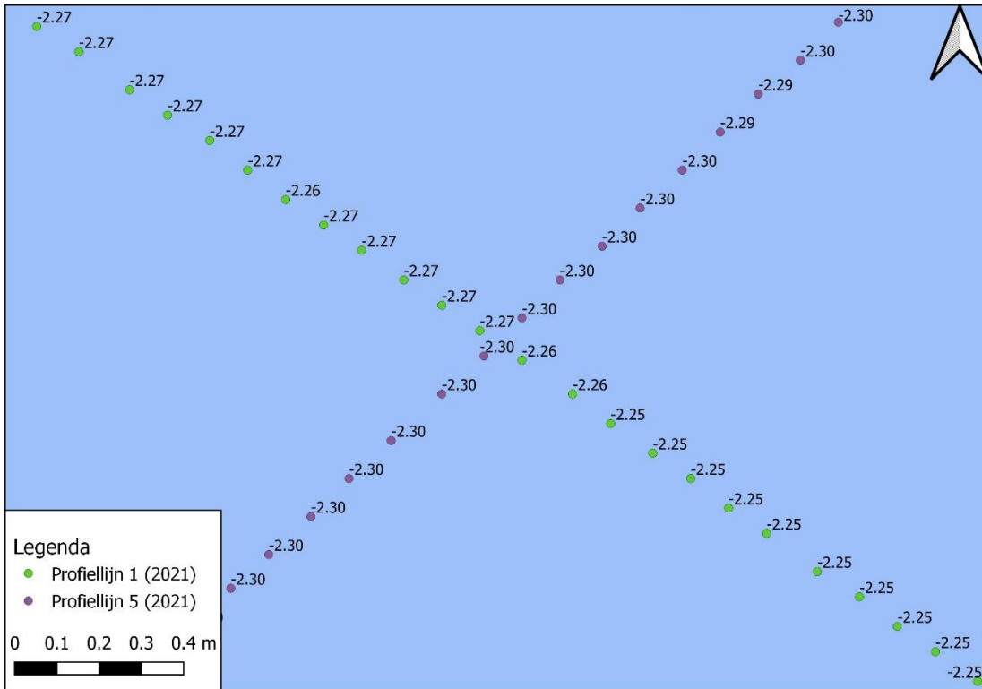
Figuur 3-47 Detailkaart controlepunt tussen profiellijn 1 en profiellijn 5 voor de hoogte/diepte raaien 2021, hoogtemetingen zijn weergegeven in m NAP.
