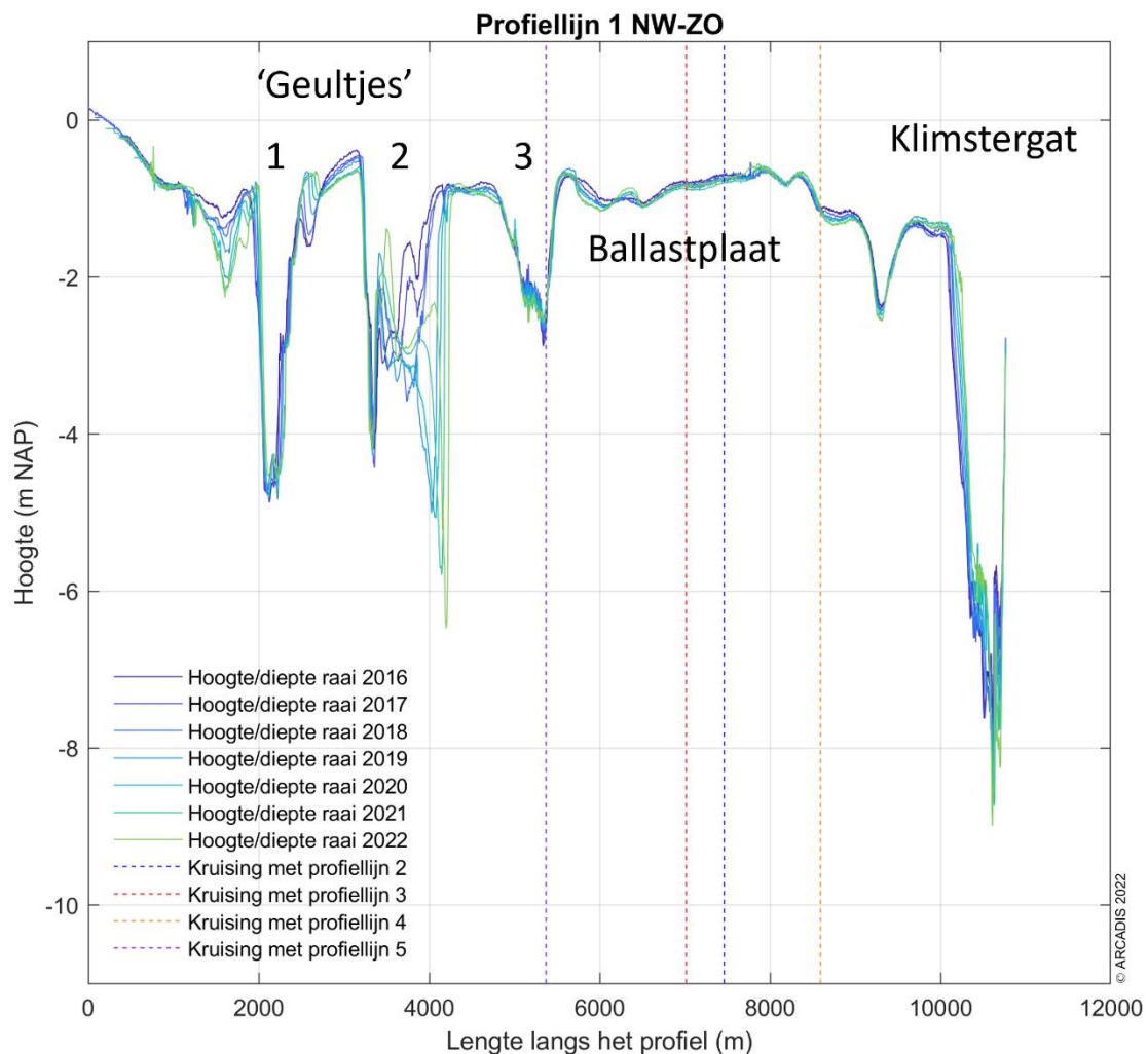
Figuur 5-1 Dwarsprofiel langs profiellijn 1 van noordwest naar zuidoost voor de hoogte/diepte raai meetgegevens van 2016 – 2022.
