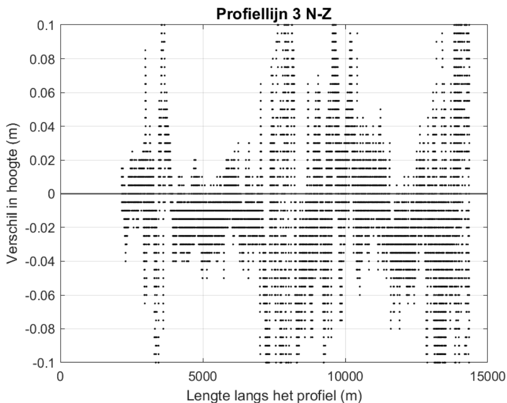
Figuur 4-19 Ingezoomde verschilplot langs profiellijn 3 van noord naar zuid voor de hoogte/diepte raai meetgegevens van 2017 en 2018. Een negatieve waarde betekent dat de hoogte/diepteraai van 2018 lager ligt dan de hoogte/diepteraai van 2017.
