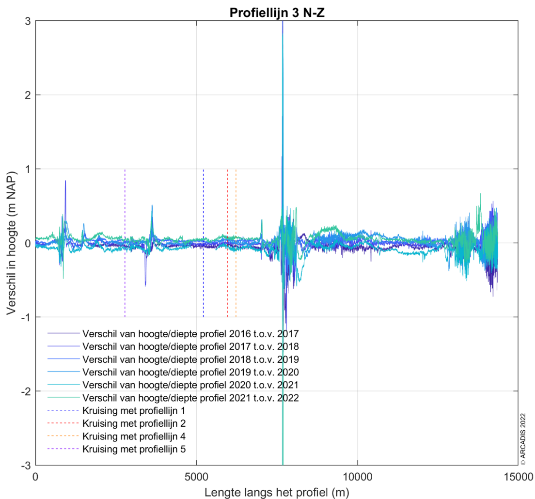
Figuur 5-9 Verschilplot langs profiellijn 3 van noord naar zuid voor de hoogte/diepte raai meetgegevens tussen 2016 t.o.v. 2017, 2017 t.o.v. 2018, 2018 t.o.v. 2019, 2019 t.o.v. 2020, 2020 t.o.v. 2021 en 2021 t.o.v. 2022. Een positieve waarde betekent dat de hoogte/diepteraai van het opvolgende jaar hoger ligt dan de hoogte/diepteraai van het eerdere jaar.
