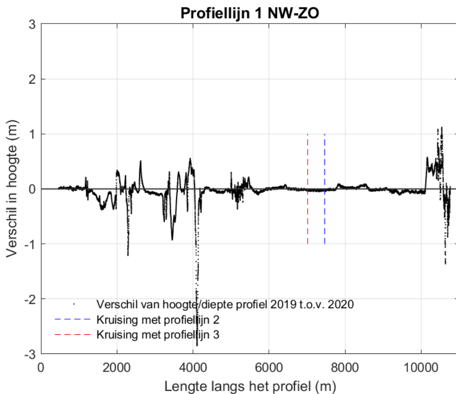
Figuur 4-39 Vershilplot langs profielijn 1 van noordwest naar zuidoost voor de hoogte/diepte raai meetgegevens van 2019 en 2020. Een positieve waarde betekent dat de hoogte/diepteraai van 2020 hoger ligt dan de hoogte/diepteraai van 2019.
