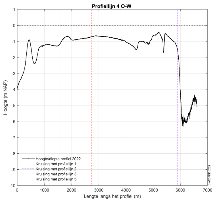
Figuur 3-56 Dwarsdoorsnede langs profiellijn 4 van oost naar west in 2021.
