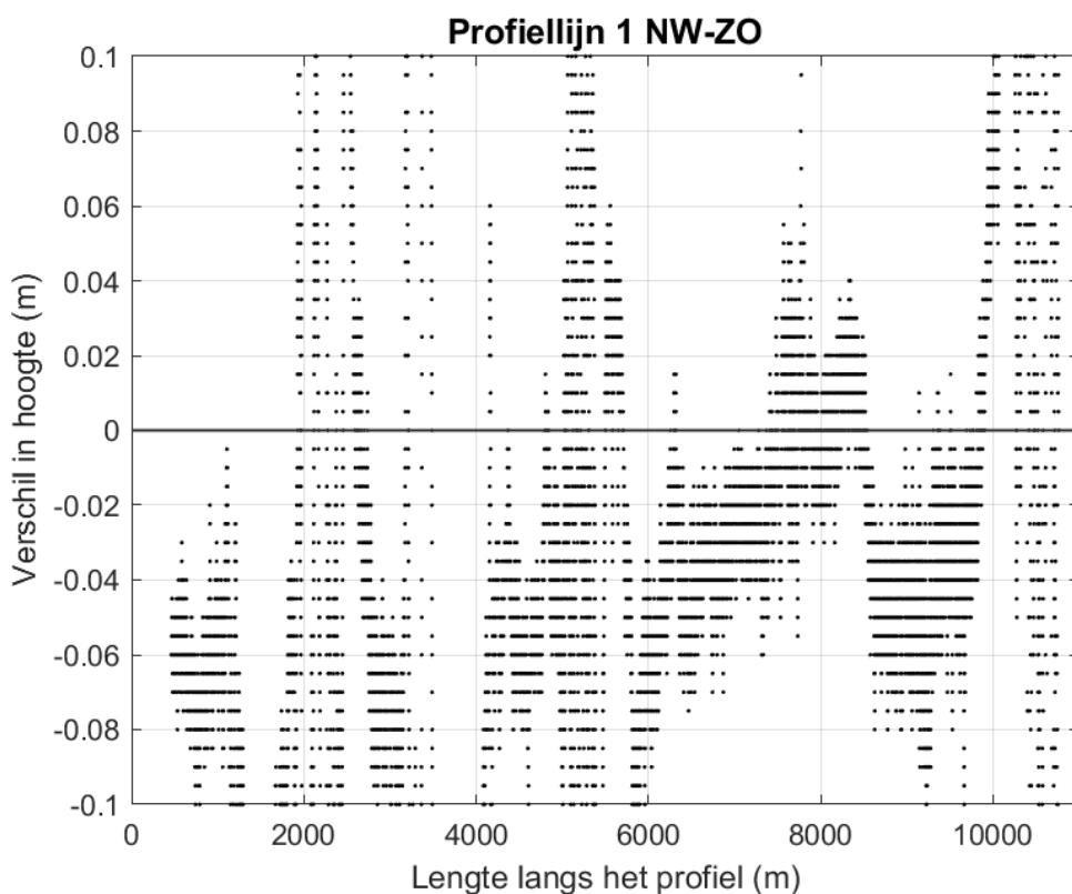
Figuur 4-4 Ingezoomde verschilplot langs profiellijn 1 van noordwest naar zuidoost voor de hoogte/diepte raai meetgegevens van 2016 en 2017. Een negatieve waarde betekent dat de hoogte/diepteraai van 2017 lager ligt dan de hoogte/diepteraai van 2016.
