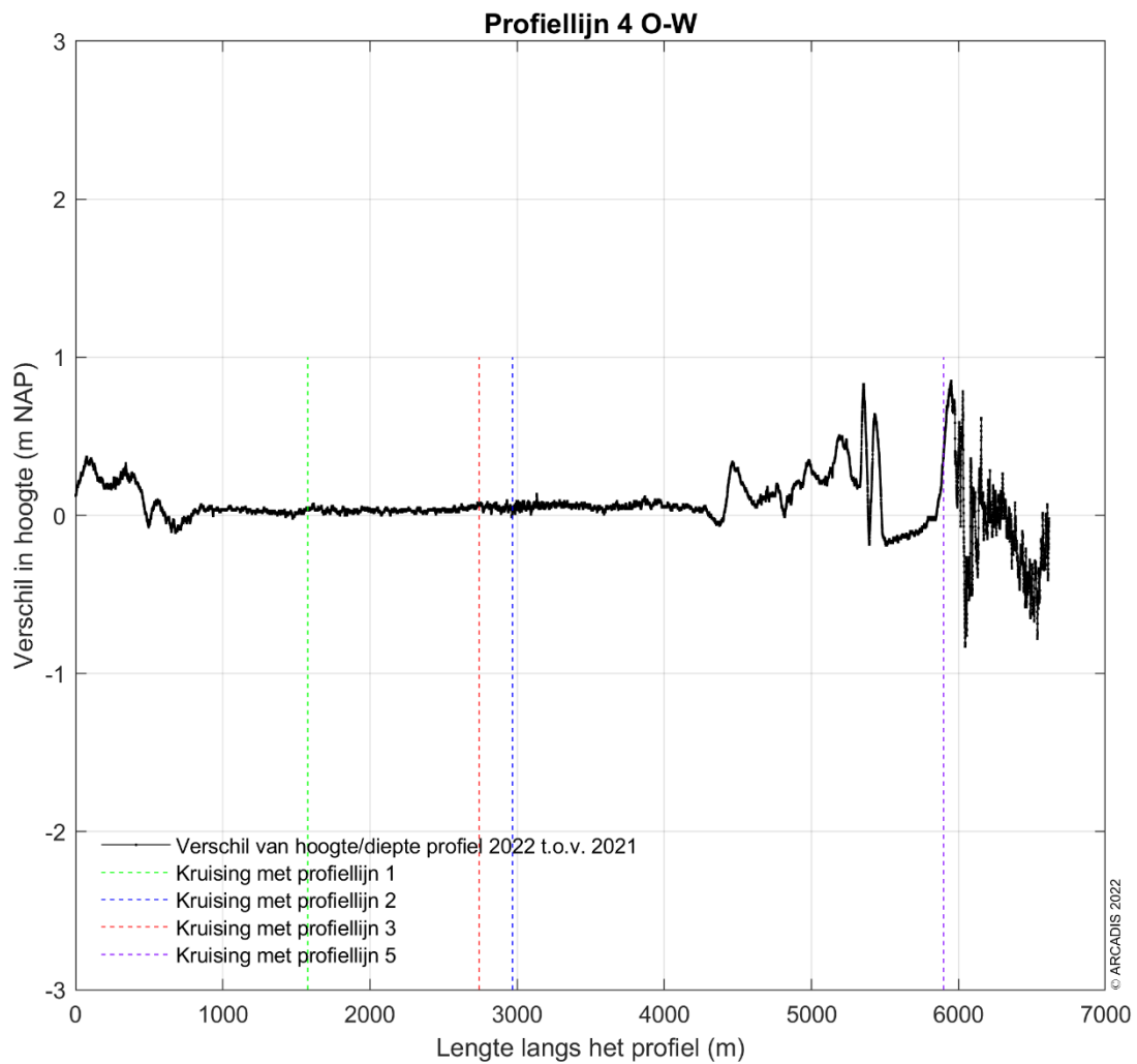
Figuur 4-66 Verschilplot langs profiellijn 4 van oost naar west voor de hoogte/diepte raai meetgegevens van 2021 en 2022. Een positieve waarde betekent dat de hoogte/diepteraai van mei 2022 hoger ligt dan de hoogte/diepteraai van 2021.
