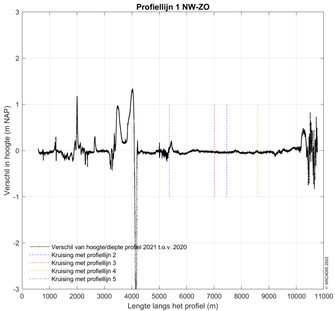
Figuur 4-48 Verschilplot langs profiellijn 1 van noordwest naar zuidoost voor de hoogte/diepte raai meetgegevens van 2020 en 2-21. Een positieve waarde betekent dat de hoogte/diepteraai van 2021 hoger ligt dan de hoogte/diepteraai van 2020.
