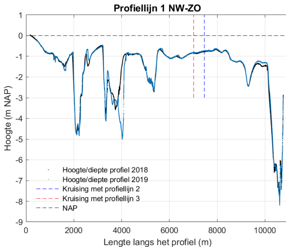
Figuur 4-20 Dwarsdoorsnede langs profiellijn 1 van noordwest naar zuidoost voor de hoogte/diepte raai meetgegevens van 2018 en mei 2019.
