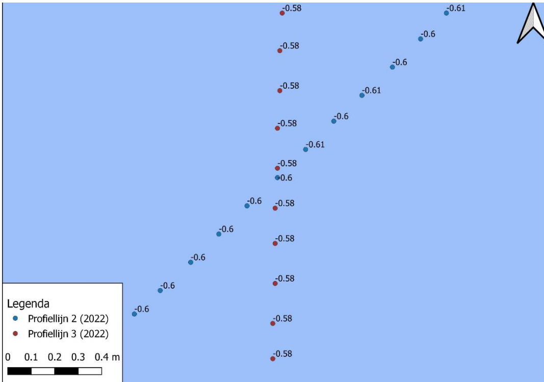
Figuur 3-62 Detailkaart controlepunt tussen profiellijn 2 en profiellijn 3 voor de hoogte/diepte raaien mei 2022, hoogtemetingen zijn weergegeven in m NAP.
