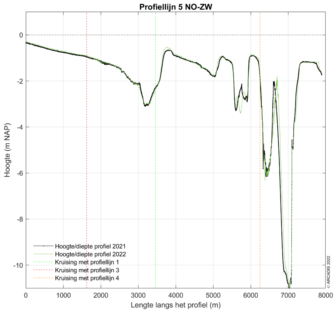
Figuur 4-68 Dwarsprofiel langs profiellijn 5 van noordoost naar zuidwest voor de hoogte/diepte raai meetgegevens van 2021 en 2022.
