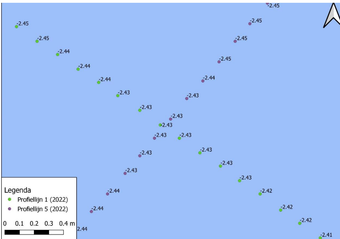
Figuur 3-61 Detailkaart controlepunt tussen profiellijn 1 en profiellijn 5 voor de hoogte/diepte raaien 2022, hoogtemetingen zijn weergegeven in m NAP.
