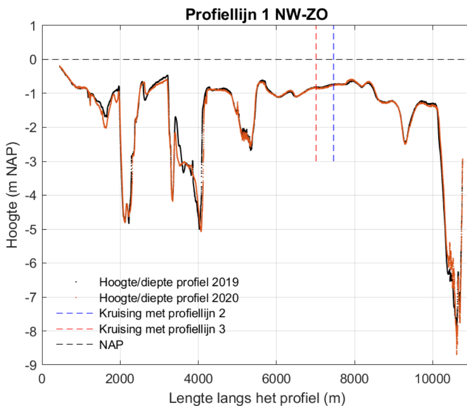
Figuur 4-38 Dwarsdoorsnede langs profiellijn 1 van noordwest naar zuidoost voor de hoogte/diepte raai meetgegevens van 2019 en 2020.
