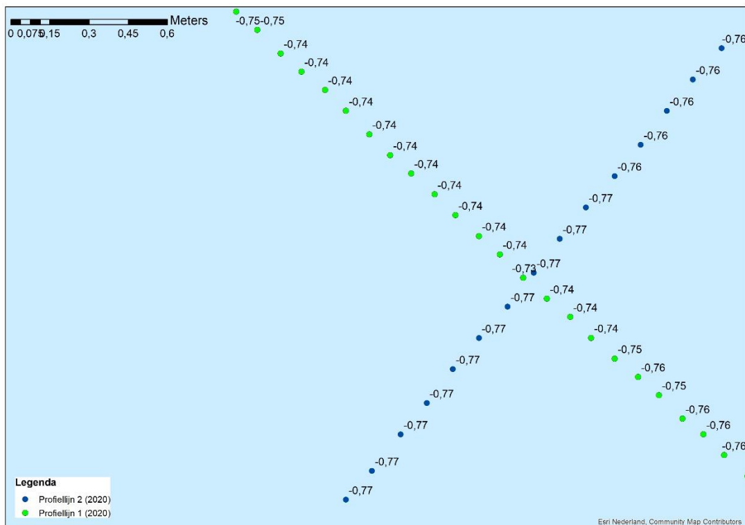
Figuur 3-30 Detailkaart controlepunt tussen profiellijn 1 en profiellijn 2 voor de hoogte/diepte raaien mei 2019, hoogtemetingen zijn weergegeven in m NAP.
