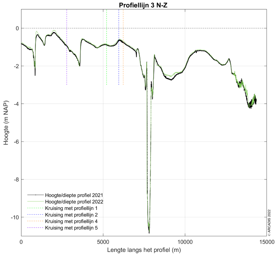
Figuur 4-62 Dwarsprofiel langs profiellijn 3 van noord naar zuid voor de hoogte/diepte raai meetgegevens van 2021 en 2022.
