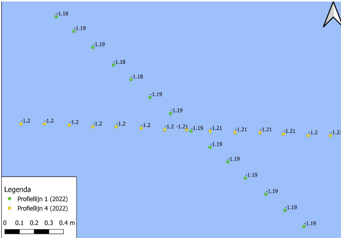
Figuur 3-60 Detailkaart controlepunt tussen profiellijn 1 en profiellijn 4 voor de hoogte/diepte raaien 2022, hoogtemetingen zijn weergegeven in m NAP.
