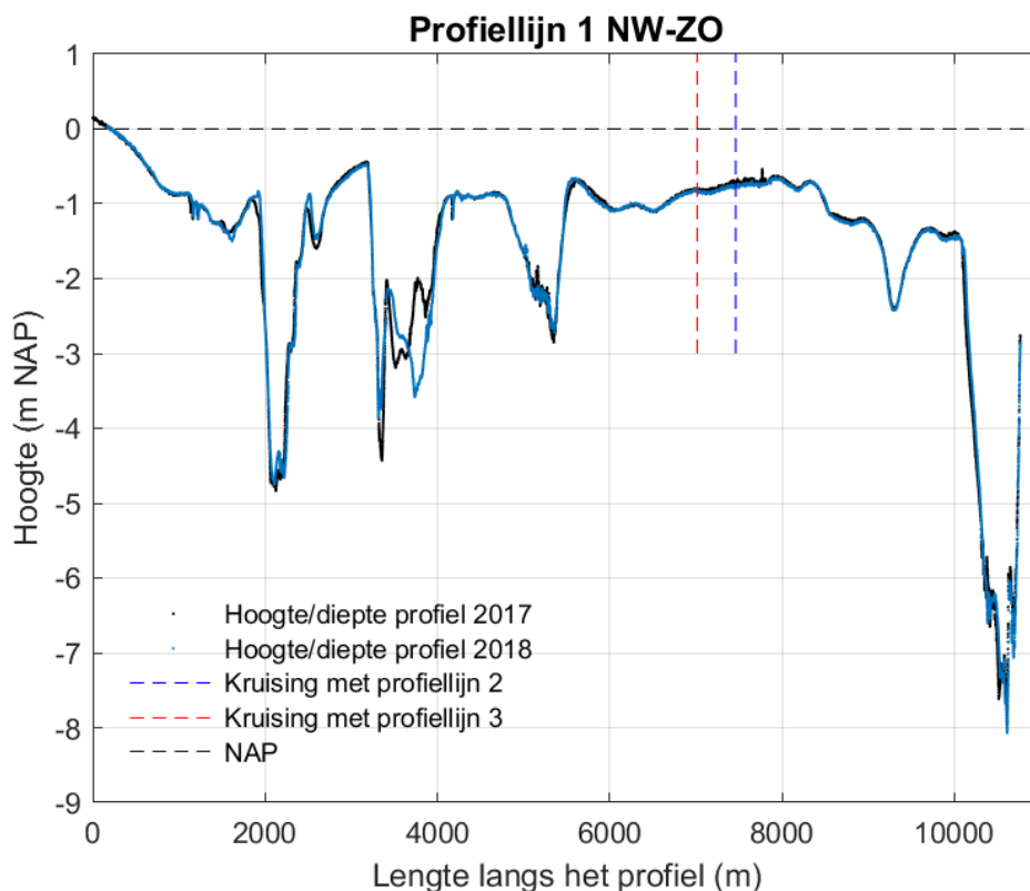
Figuur 4-11 Dwarsdoorsnede langs profiellijn 1 van noordwest naar zuidoost voor de hoogte/diepte raai meetgegevens van 2017 en 2018.
