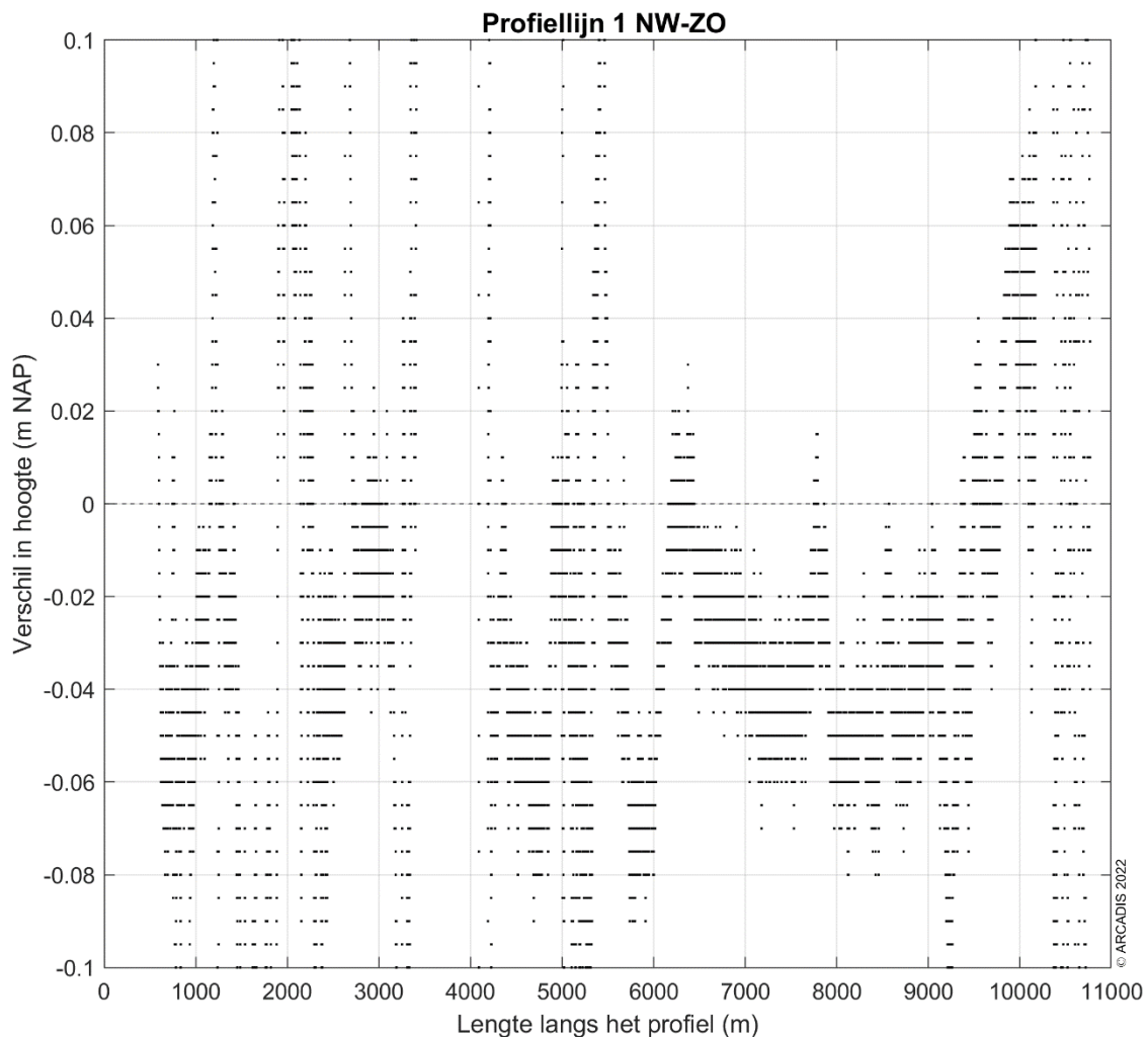
Figuur 4-49 Ingezoomde verschilplot langs profiellijn 1 van noordwest naar zuidoost voor de hoogte/diepte raai meetgegevens van 2020 en 2021. Een positieve waarde betekent dat de hoogte/diepteraai van 2021 hoger ligt dan de hoogte/diepteraai van 2020.
