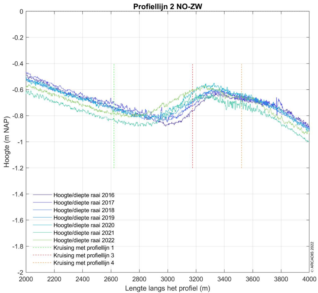
Figuur 5-5 Ingezoomd dwarsprofiel langs profiellijn 2 van noordoost naar zuidwest voor de hoogte/diepte raai meetgegevens van 2016 – 2022 (Detail van Figuur 5-4).
