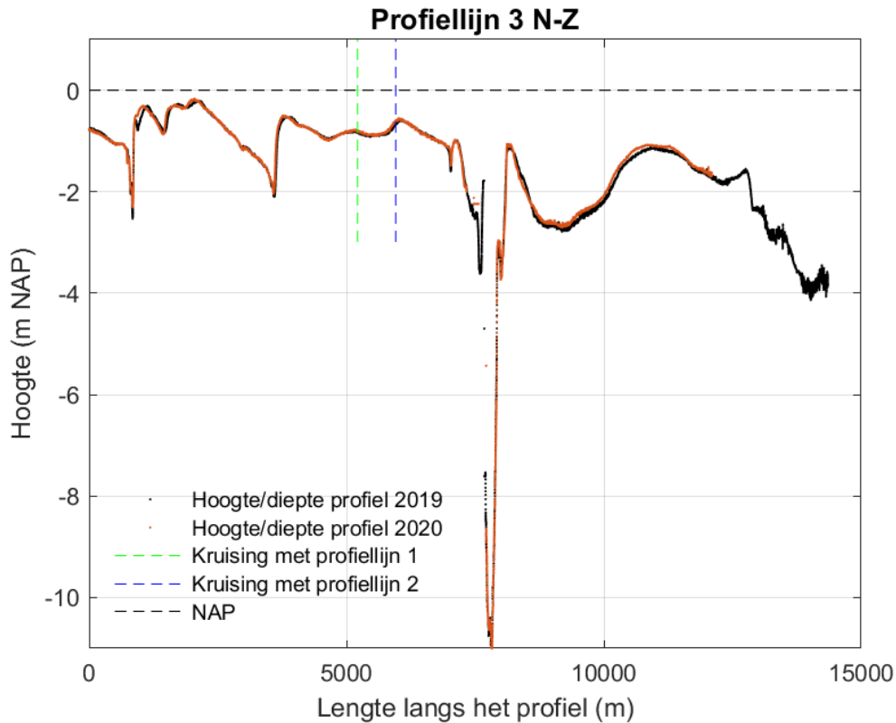
Figuur 4-44 Dwarsprofiel langs profiellijn 3 van noord naar zuid voor de hoogte/diepte raai meetgegevens van 2019 en 2020.
