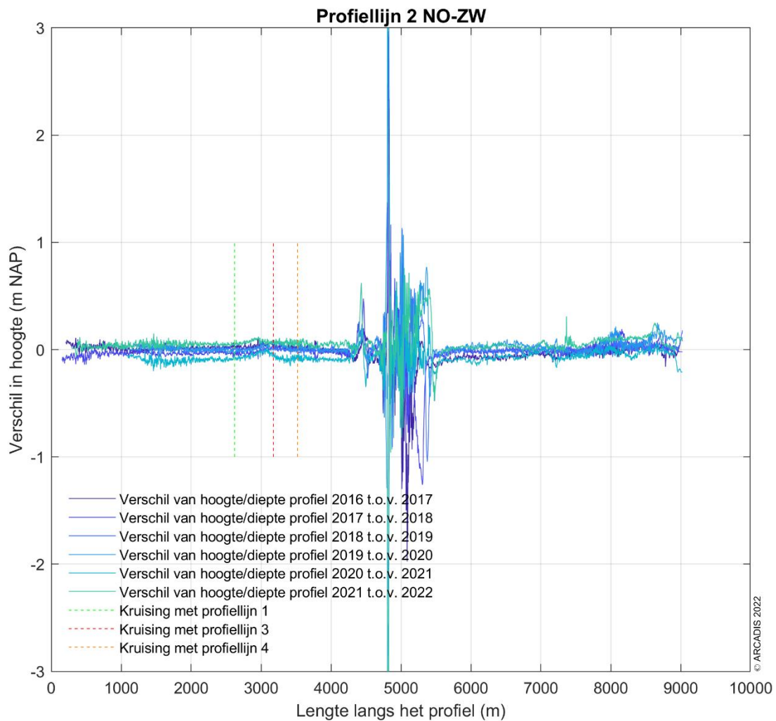
Figuur 5-6 Verschilplot langs profiellijn 2 van noordoost naar zuidwest voor de hoogte/diepte raai meetgegevens tussen 2016 t.o.v. 2017, 2017 t.o.v. 2018, 2018 t.o.v. mei 2019, 2019 t.o.v. 2020, 2020 t.o.v. 2021 en 2021 t.o.v. 2022. Een positieve waarde betekent dat de hoogte/diepteraai van het opvolgende jaar hoger ligt dan de hoogte/diepteraai van het eerdere jaar.
