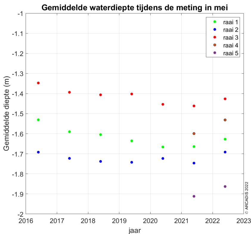
Figuur 4-1 Plot van de gemiddelde waterdiepte per raai langs de verschillende profielen voor alle meetmomenten. Binnen de raai zijn alleen de punten meegenomen waar voor elk jaar een dieptemeting beschikbaar is in de berekening van de gemiddelde diepte.
