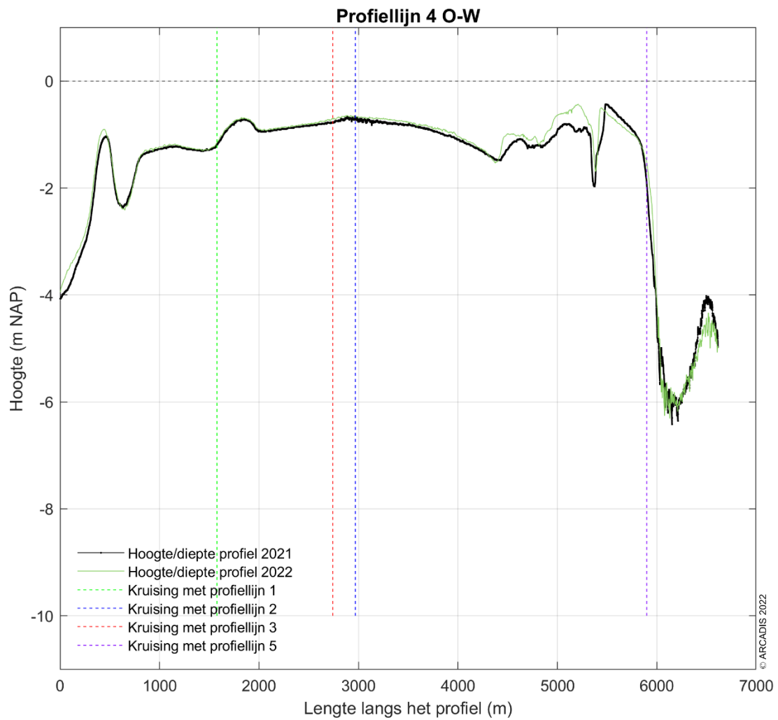
Figuur 4-65 Dwarsprofiel langs profiellijn 4 van oost naar west voor de hoogte/diepte raai meetgegevens van 2021 en 2022.
