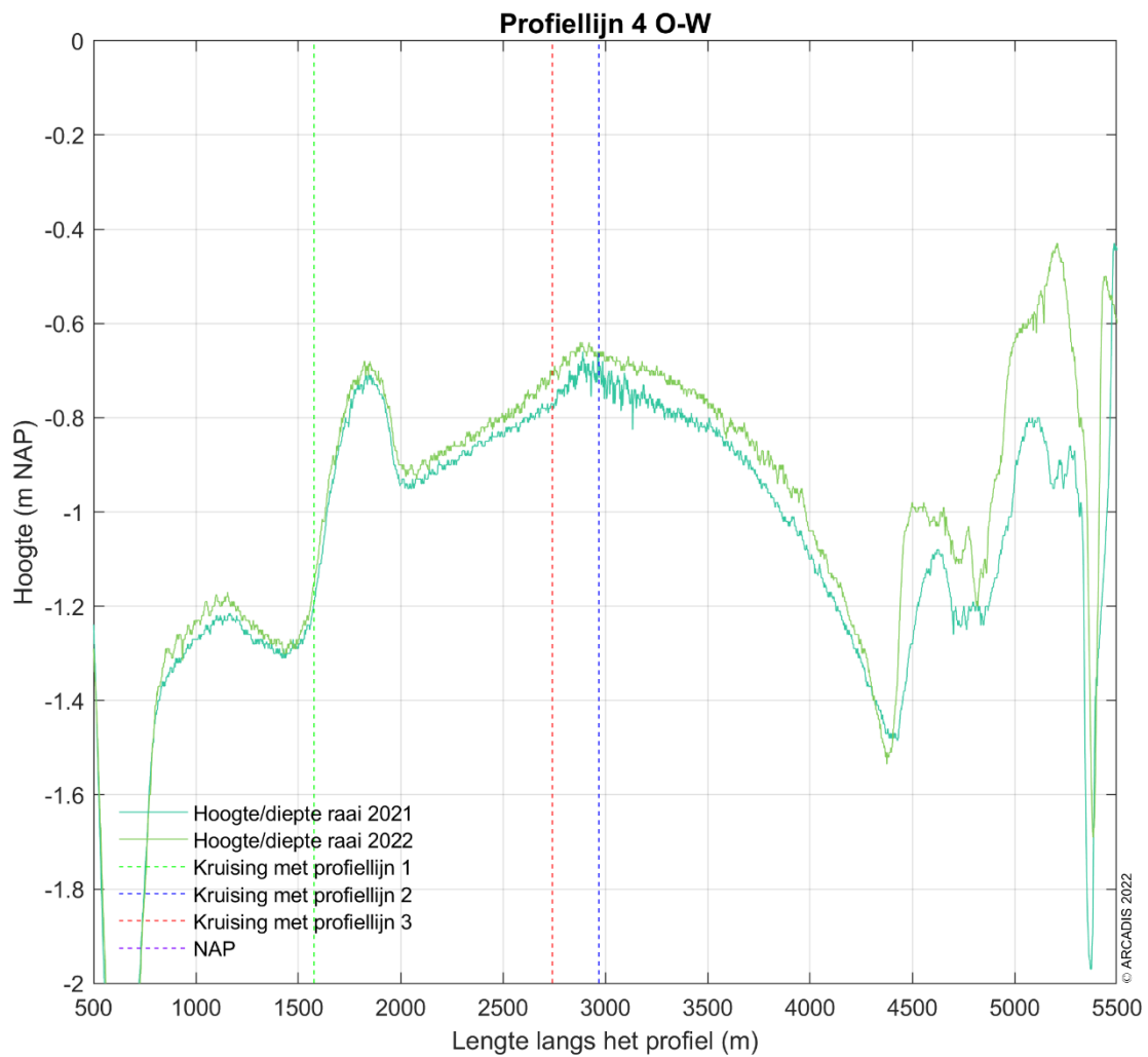
Figuur 5-11 Ingezoomd dwarsprofiel langs profiellijn 4 van noord naar zuid voor de hoogte/diepte raai meetgegevens van 2016 - 2022 (Detail van Figuur 5-10/Figuur 5-7).
