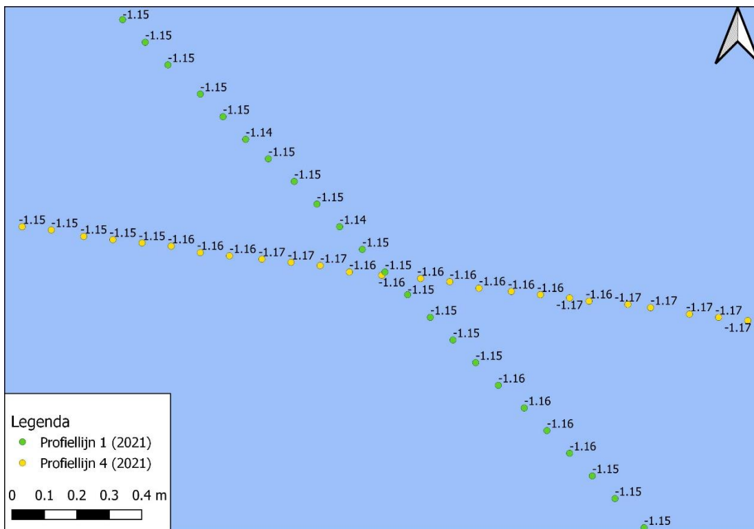
Figuur 3-46 Detailkaart controlepunt tussen profiellijn 1 en profiellijn 4 voor de hoogte/diepte raaien 2021, hoogtemetingen zijn weergegeven in m NAP.
