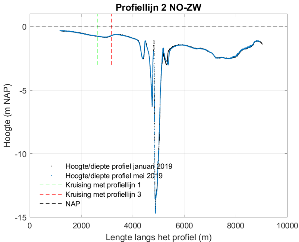
Figuur 4-32 Dwarsdoorsnede langs profiellijn 2 van noordoost naar zuidwest voor de hoogte/diepte raai meetgegevens van januari 2019 en mei 2019.
