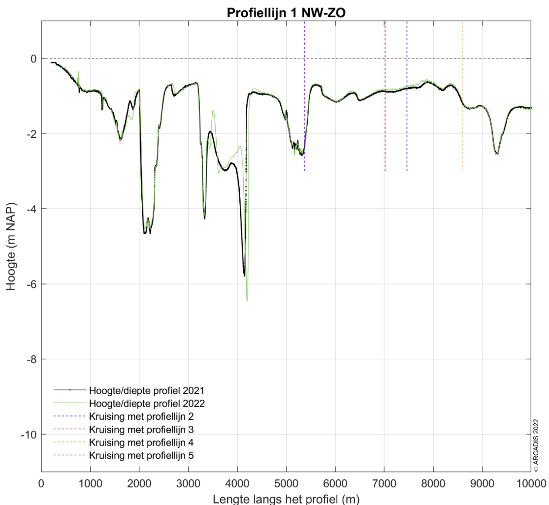
Figuur 4-56 Dwarsdoorsnede langs profiellijn 1 van noordwest naar zuidoost voor de hoogte/diepte raai meetgegevens van 2021 en 2022.
