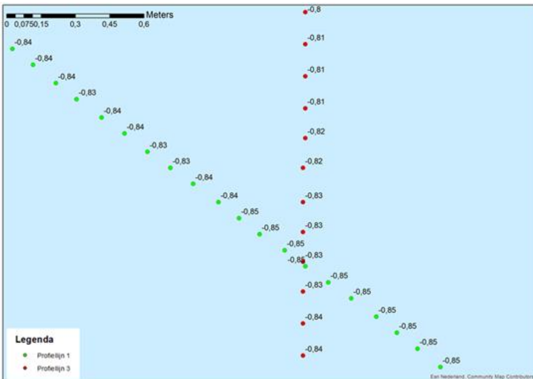
Figuur 3-37 Detailkaart controlepunt tussen profiellijn 1 en profiellijn 3 voor de hoogte/diepte raaien 2020, hoogtemetingen zijn weergegeven in m NAP.
