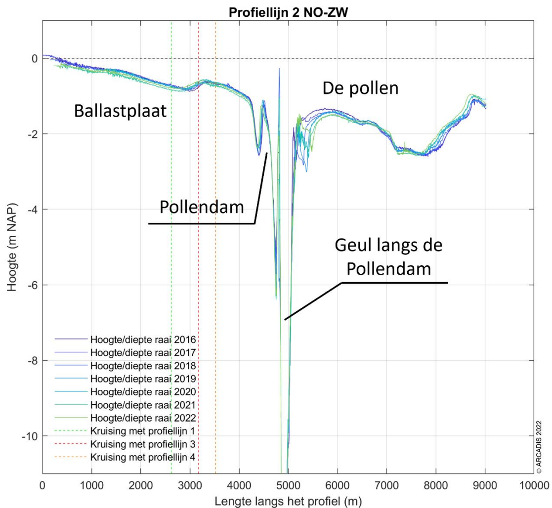
Figuur 5-4 Dwarsprofiel langs profiellijn 2 van noordoost naar zuidwest voor de hoogte/diepte raai meetgegevens van 2016 - 2022.
