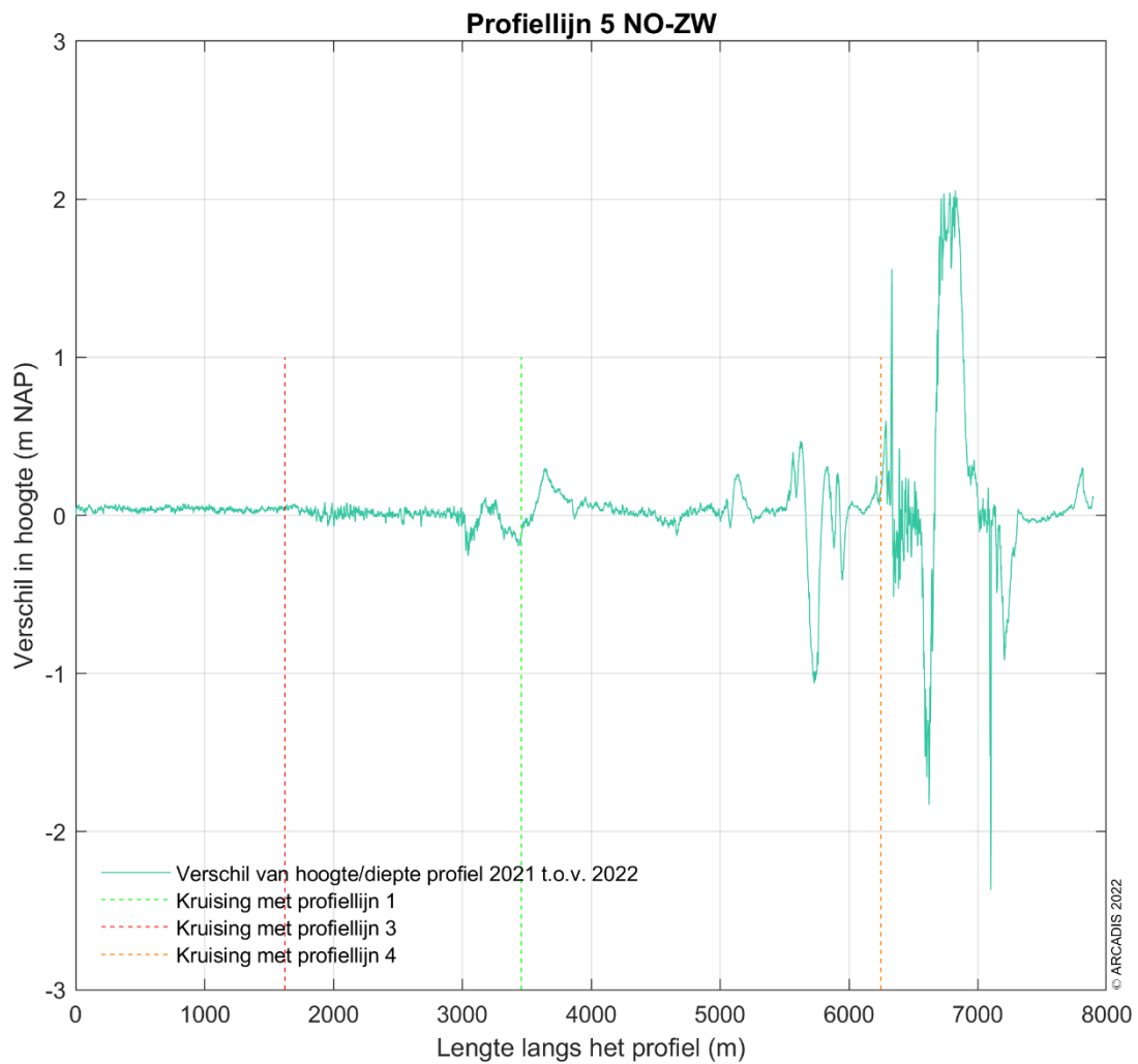
Figuur 5-15 Vershilplot langs profiellijn 5 van noord naar zuid voor de hoogte/diepte raai meetgegevens tussen 2016 t.o.v. 2017, 2017 t.o.v. 2018, 2018 t.o.v. 2019, 2019 t.o.v. 2020, 2020 t.o.v. 2021 en 2021 t.o.v. 2022. Een positieve waarde betekent dat de hoogte/diepteraai van het opvolgende jaar hoger ligt dan de hoogte/diepteraai van het eerdere jaar.
