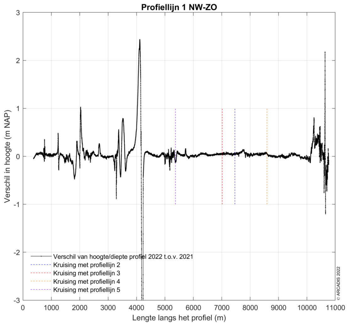
Figuur 4-57 Vershilplot langs profiellijn 1 van noordwest naar zuidoost voor de hoogte/diepte raai meetgegevens van 2021 en 2022. Een positieve waarde betekent dat de hoogte/diepteraai van 2022 hoger ligt dan de hoogte/diepteraai van 2021.
