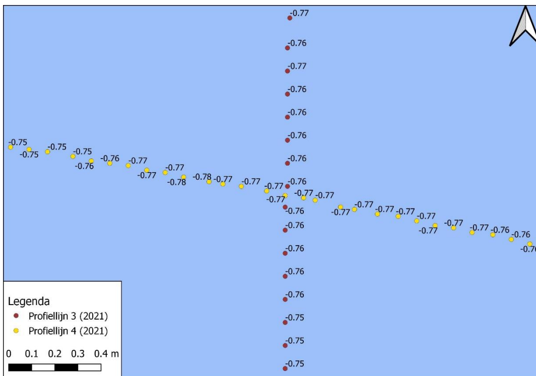
Figuur 3-50 Detailkaart controlepunt tussen profiellijn 3 en profiellijn 4 voor de hoogte/diepte raaien mei 2021, hoogtemetingen zijn weergegeven in m NAP.
