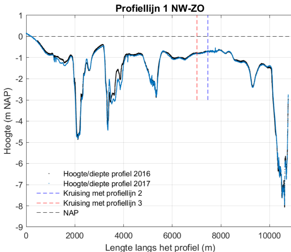
Figuur 4-2 Dwarsdoorsnede langs profiellijn 1 van noordwest naar zuidoost voor de hoogte/diepte raai meetgegevens van 2016 en 2017.
