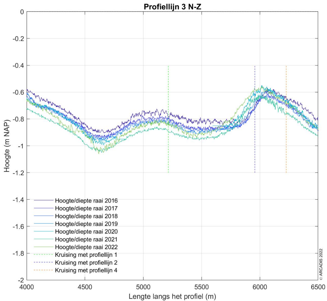
Figuur 5-8 Ingezoomd dwarsprofiel van de Ballastplaat langs profiellijn 3 van noord naar zuid voor de hoogte/diepte raai meetgegevens van 2016 - 2022 (Detail van Figuur 5-7).
