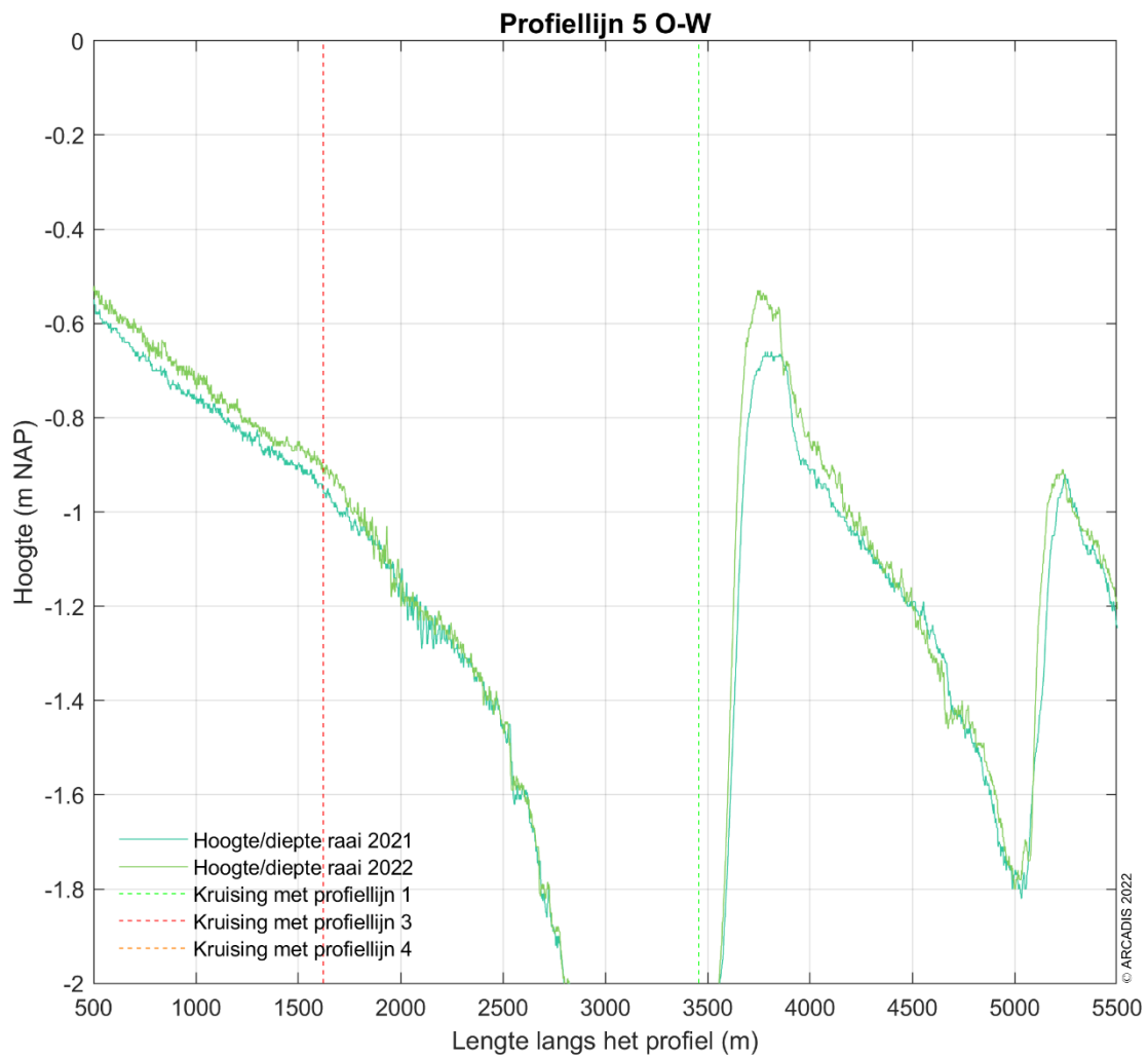
Figuur 5-14 Ingezoomd dwarsprofiel langs profiellijn 5 van noord naar zuid voor de hoogte/diepte raai meetgegevens van 2016 - 2022 (Detail van Figuur 5-13).
