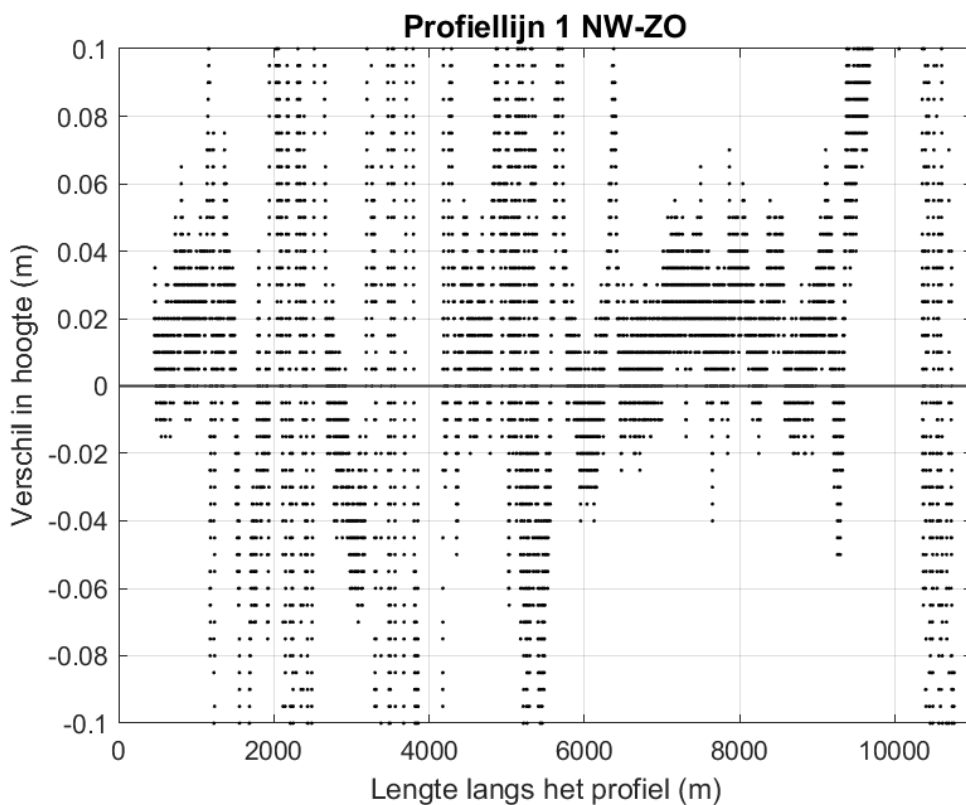
Figuur 4-22 Ingezoomde verschilplot langs profiellijn 1 van noordwest naar zuidoost voor de hoogte/diepte raai meetgegevens van 2018 en mei 2019. Een positieve waarde betekent dat de hoogte/diepteraai van mei 2019 hoger ligt dan de hoogte/diepteraai van 2018.
