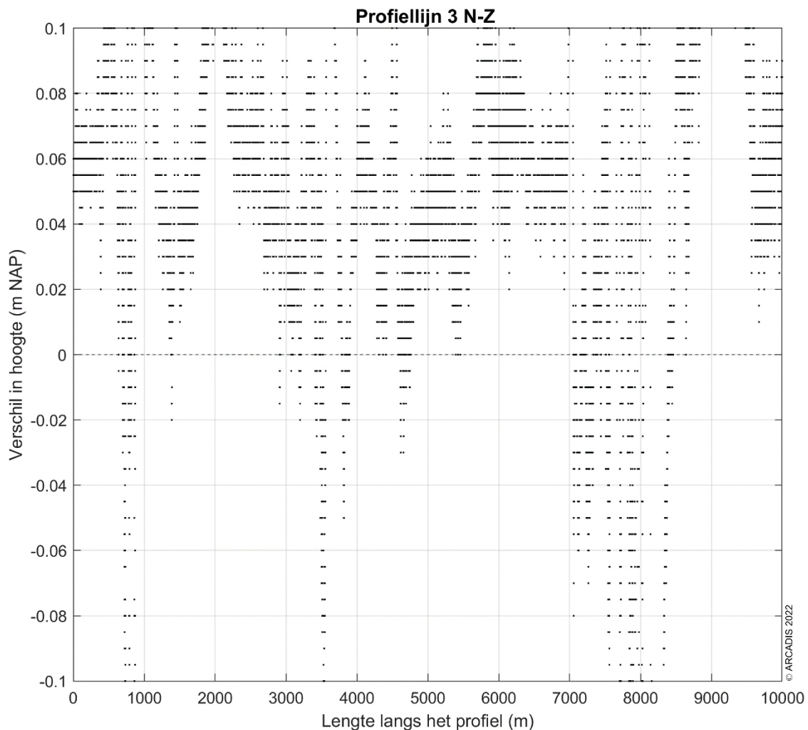
Figuur 4-64: Ingezoomde verschilplot langs profiellijn 3 van noord naar zuid voor de hoogte/diepte raai meetgegevens van 2021 en 2022. Een positieve waarde betekent dat de hoogte/diepteraai van 2022 hoger ligt dan de hoogte/diepteraai van 2021.
