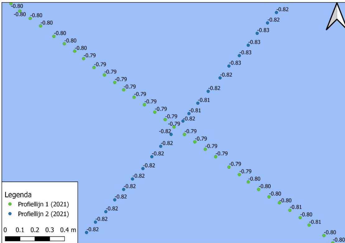
Figuur 3-44 Detailkaart controlepunt tussen profiellijn 1 en profiellijn 2 voor de hoogte/diepte raaien 2021, hoogtemetingen zijn weergegeven in m NAP.
