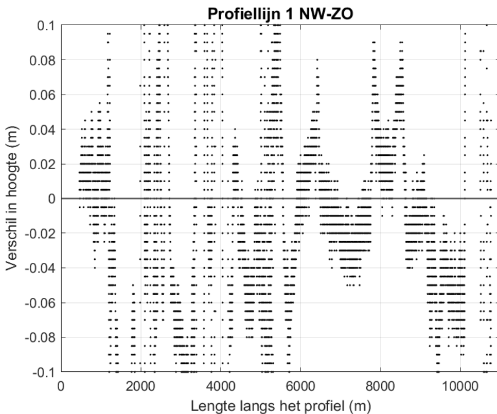
Figuur 4-40 Ingezoomde vershilplot langs profielijn 1 van noordwest naar zuidoost voor de hoogte/diepte raai meetgegevens van 2019 en 2020. Een positieve waarde betekent dat de hoogte/diepteraai van 2020 hoger ligt dan de hoogte/diepteraai van 2019.
