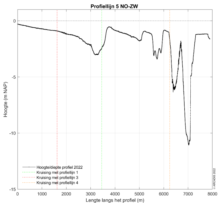
Figuur 3-57 Dwarsdoorsnede langs profiellijn 5 van noordoost naar zuidwest in 2021.
