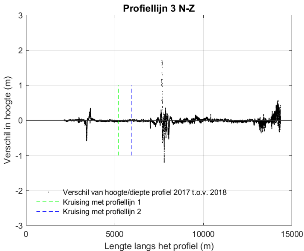
Figuur 4-18 Verschilplot langs profiellijn 3 van noord naar zuid voor de hoogte/diepte raai meetgegevens van 2017 en 2018. Een negatieve waarde betekent dat de hoogte/diepteraai van 2018 lager ligt dan de hoogte/diepteraai van 2017.
