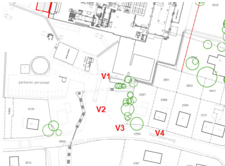
Figuur 1.8 Opstellocaties wachtende vrachtwagens voor poort en op Volmolenweg in referentiesituatie (wachtende vrachtwagens staan voor 7 uur voor de poort op positie V1 en V2)
