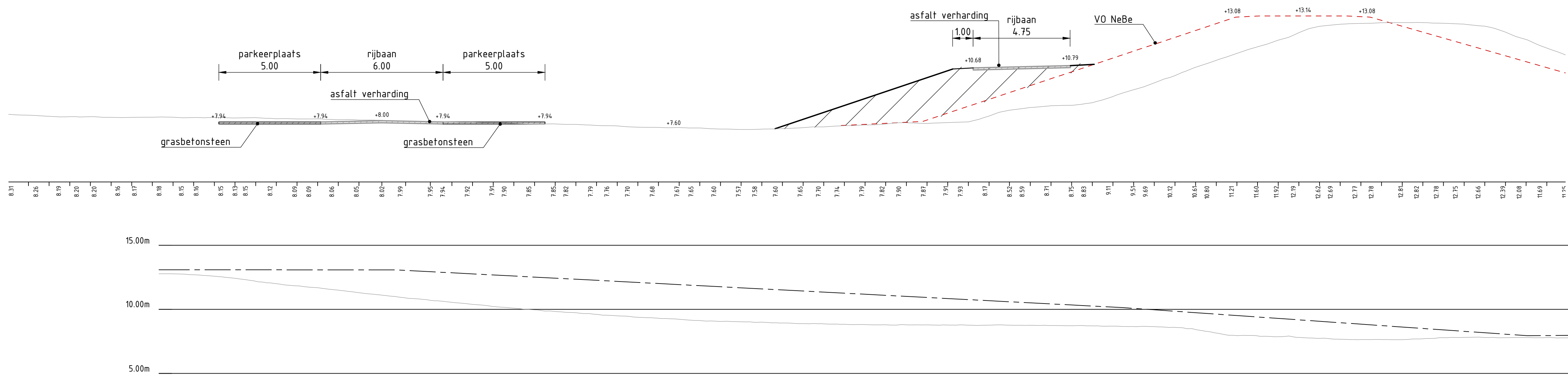
ALM-toegangsweg-parkeerplaats 1 Lengteprofiel as ALM-toegangsweg-parkeerplaats Metrering 0.000 tot 114.617
