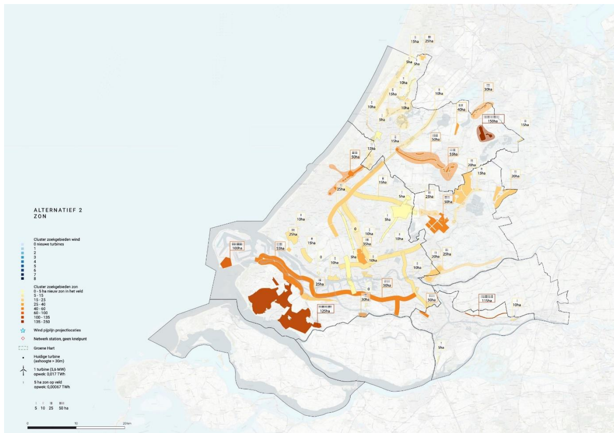
Kaart alternatief 2: RES 1.0 – na besluitvorming (zonne-energie)
