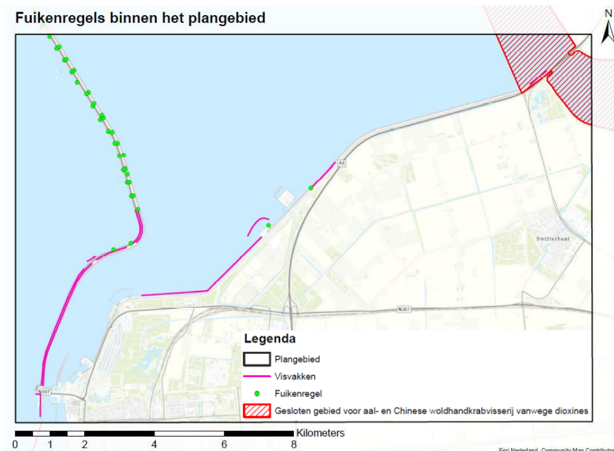
Figuur 6-17: Fuikenregels en vakken aan de IJsselmeerdijk.
