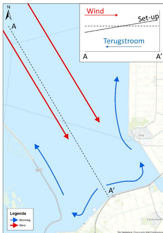
Figuur 6-15: Verwachte stroming langs de IJsselmeerdijk tijdens aanlandige wind (links).
