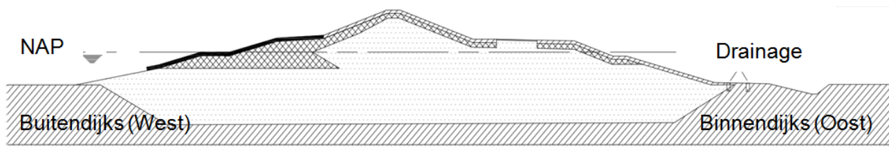
Figuur 6-3: Kenmerkende dijkopbouw IJsselmeerdijk
