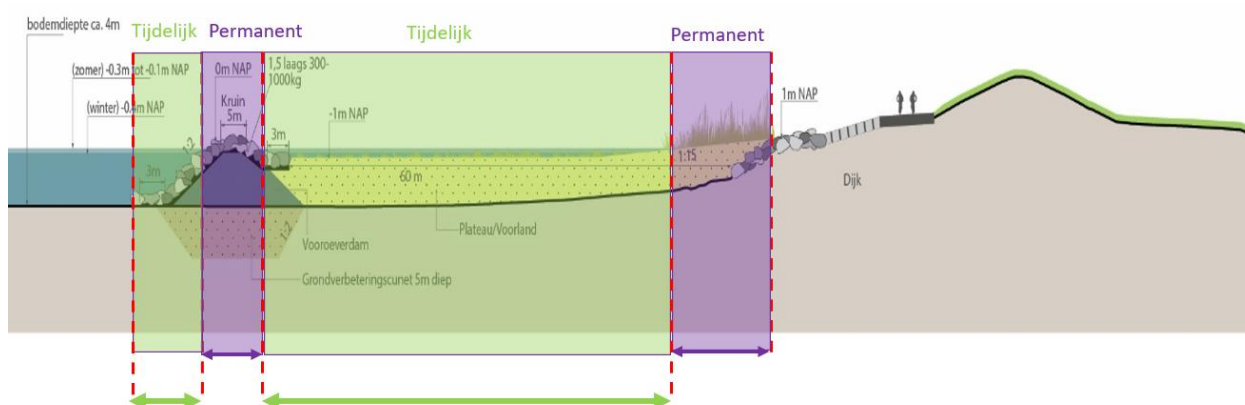
Figuur 5-1 Overzicht van tijdelijk en permanent ruimtebeslag tijdens en na de realisatie van de vooroever
