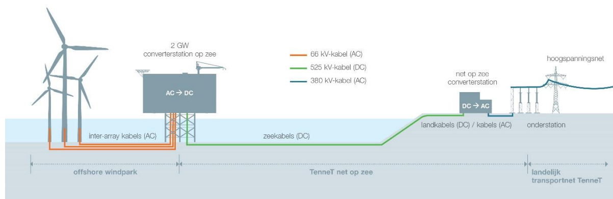
Figuur 1-1 Onderdelen project Net op Zee IJmuiden Ver Alpha
