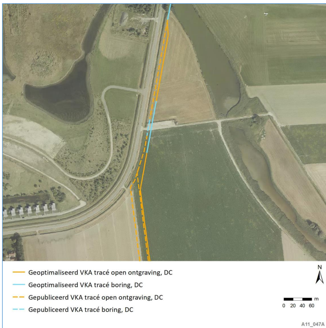
Figuur 4-17 Zuidwaartse verplaatsing parallel aan Muidenweg ten zuiden van vliegveld
