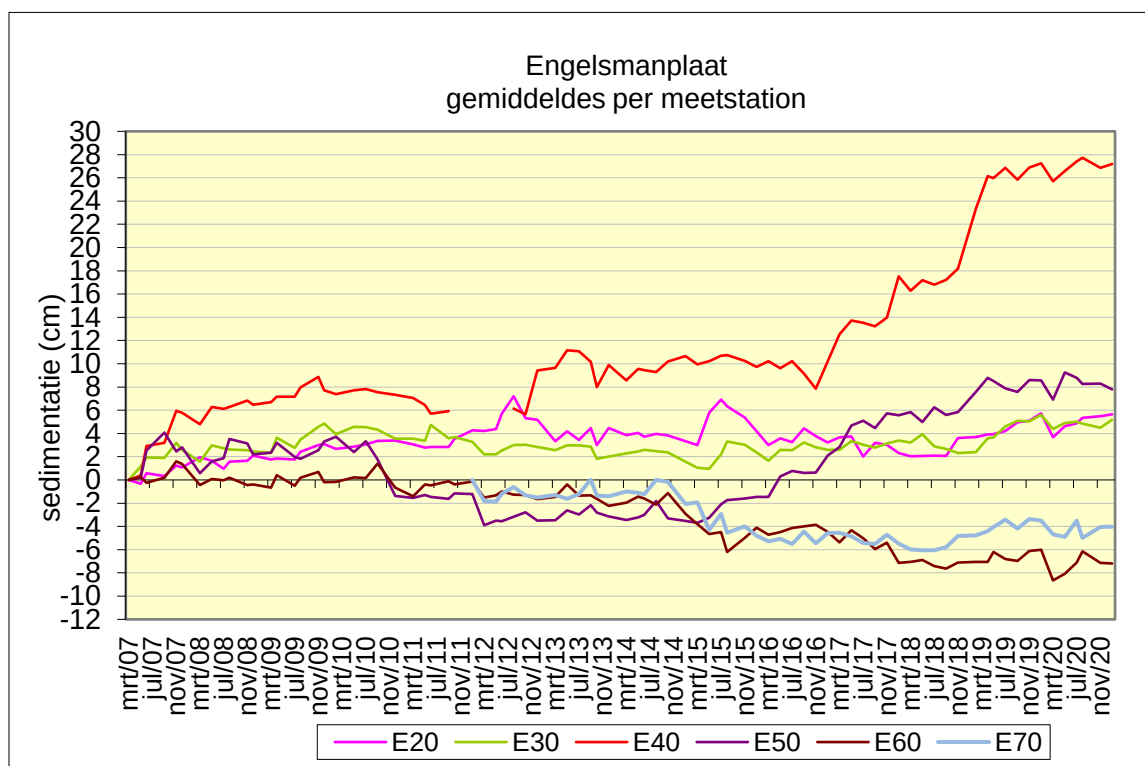
Figuur 17. Gemiddelde meetlijnen van de meetstations E20 tm E70 in het onderzoeksgebied Engelsmanplaat.
