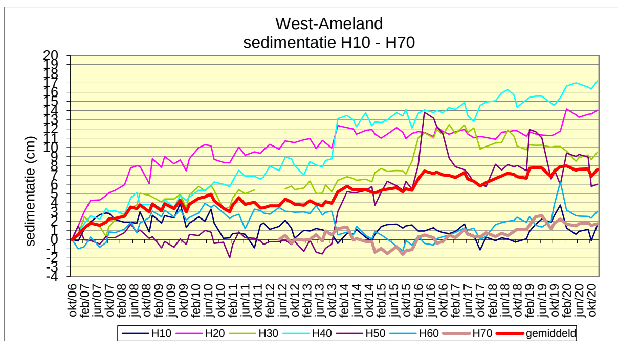
Figuur 23. Gemiddelde meetlijnen van de meetstations H10 tm H70 in het onderzoeksgebied West-Ameland.
