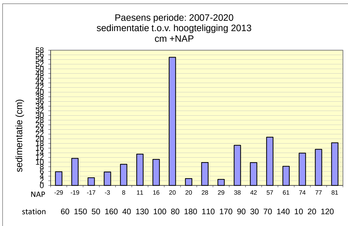
Figuur 31. Sedimentatie P10 – P180 in relatie tot de hoogteligging in 2013.
