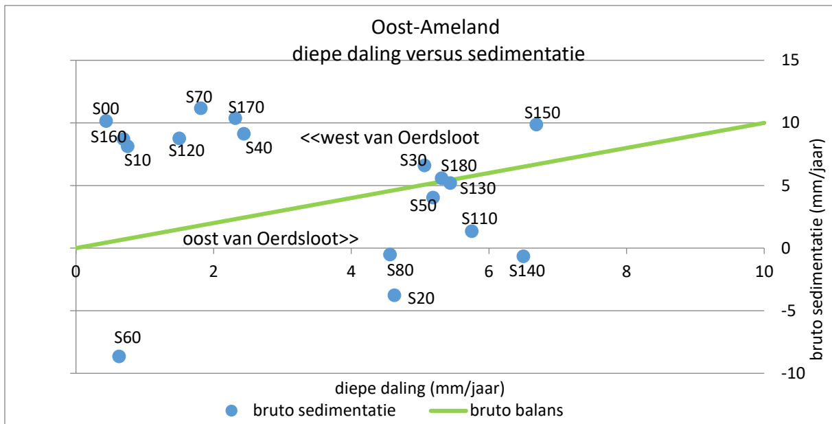
Figuur 34. Sedimentatie of erosie aan het oppervlak uitgezet tegen de diepe daling. Op de balanslijn blijft een station op dezelfde hoogte door gelijke sedimentatie en diepe daling.
