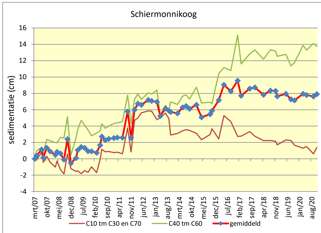
Figuur 20. Gemiddelde van de gebieden C10 – C30 en C70 (oost) en C40 – C60 (west) en het overall gemiddelde van de meetstations C10 tm C70 in het onderzoeksgebied Schiermonnikoog. Er is een duidelijk verschil tussen de twee deelgebieden.
