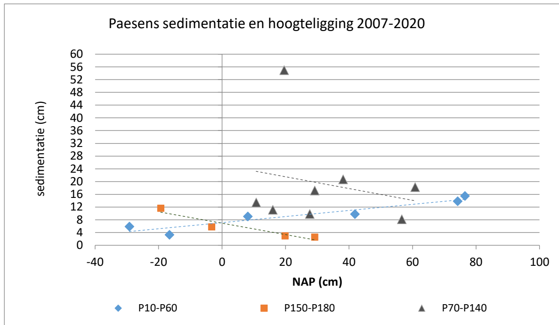
Figuur 32. Hoogteligging (2013) en sedimentatie van meetstations bij Paesens in de periode 2007-2020.
