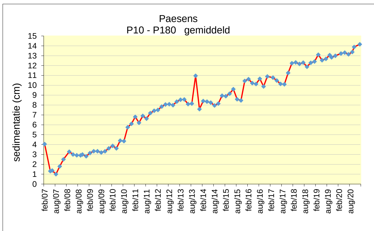
Figuur 16. Gemiddelde verschilmeting van de meetstations P10 tm P180 in het onderzoeksgebied bij Paesens.
