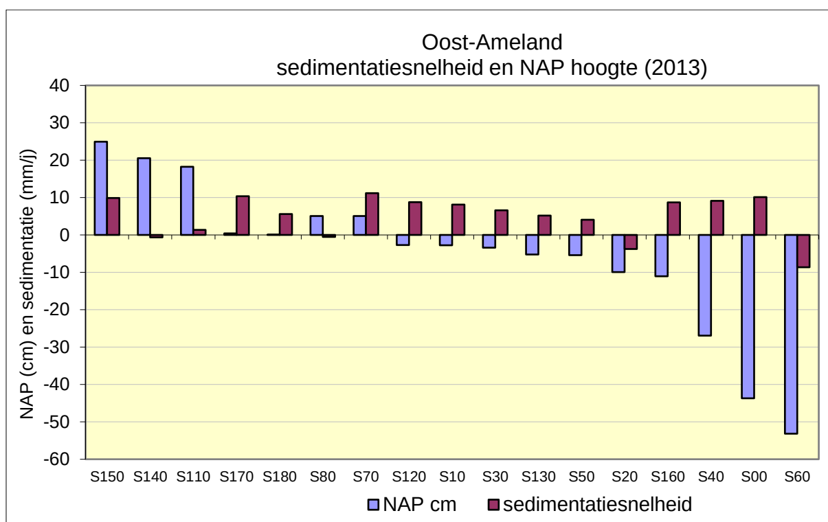
Figuur 29. Wadsedimentatie ten opzichte van hoogteligging van de meetstations bij Oost-Ameland. Sedimentatiesnelheid in mm per jaar over de totale meetperiode tm december 2020. Meetperiode van de meetstations varieert van 13 tot 19 jaar tussen 2000 en 2020 (zie tabel 7).
