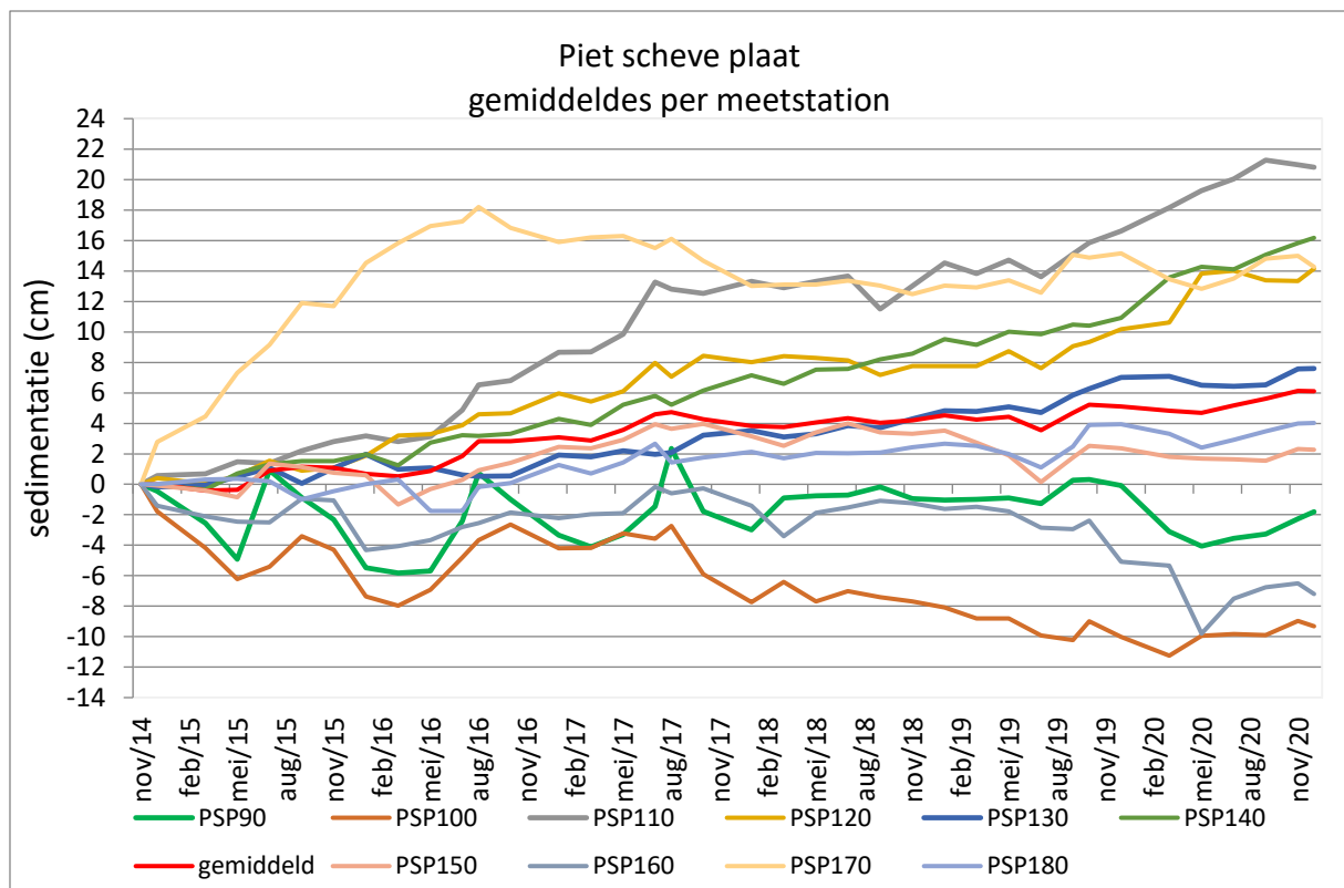
Figuur 24. Gemiddelde meetlijnen van de meetstations PSP90 tm PSP180 in het onderzoeksgebied Piet scheve plaat. Tevens is het gemiddelde van deze 10 meetlijnen genomen als weergave van de sedimentatie van het gebied waarin de meetstations liggen.
