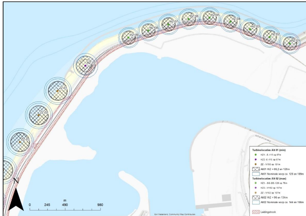
Figuur 8.8 Weergave buisleidingstroom i.r.t. windpark deelgebied Noord
