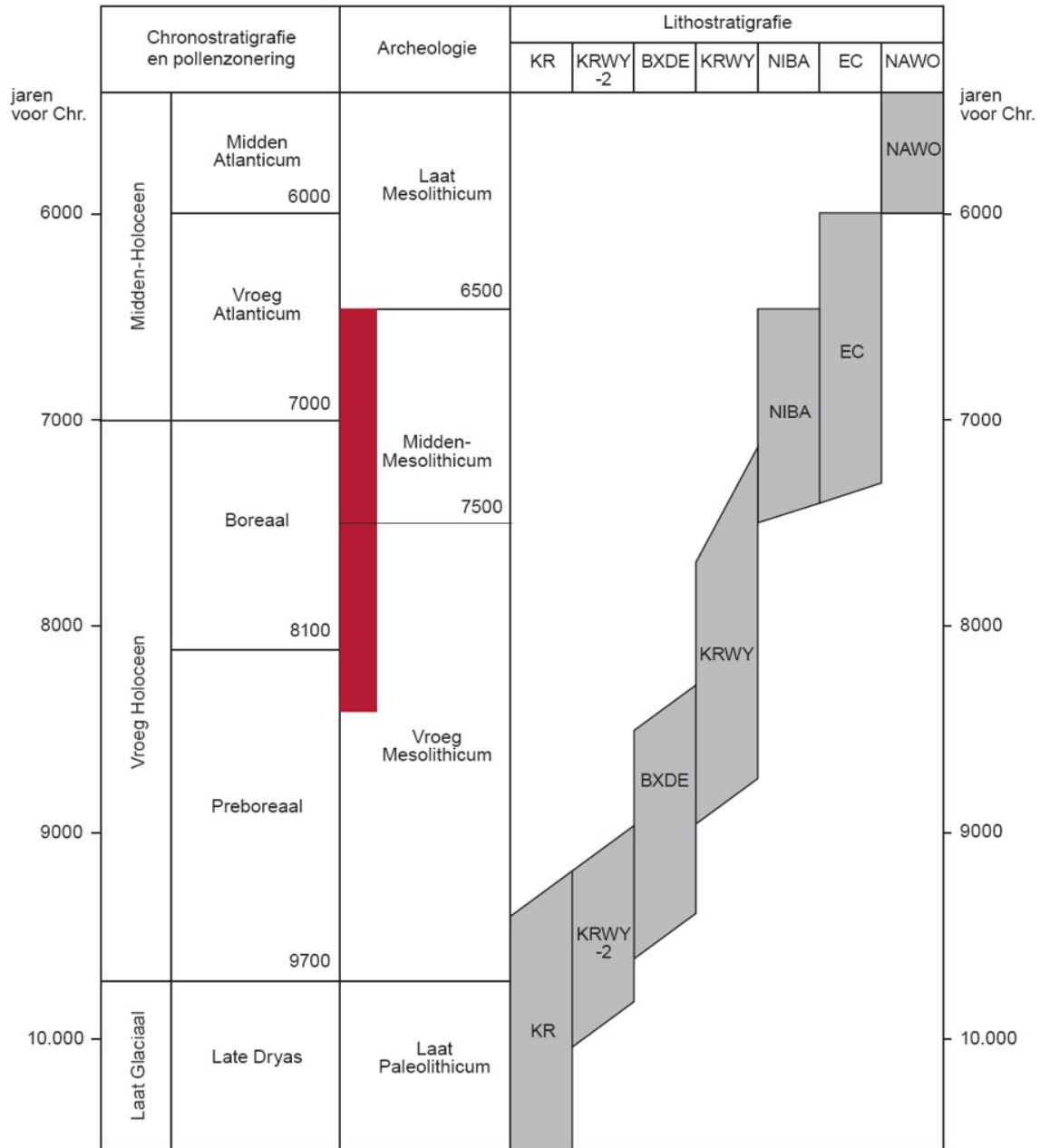
Afbeelding 10. Stratigrafische tabel met tijdindelingen, archeologische perioden, laageenheden en hun chronologie in de Yangtzehaven. Met de rode balk wordt de periode van menselijk gebruik van het rivierduincomplex (bepaald aan de hand van 14C-dateringen) aangegeven (uit: Vos en Cohen, 2015).
