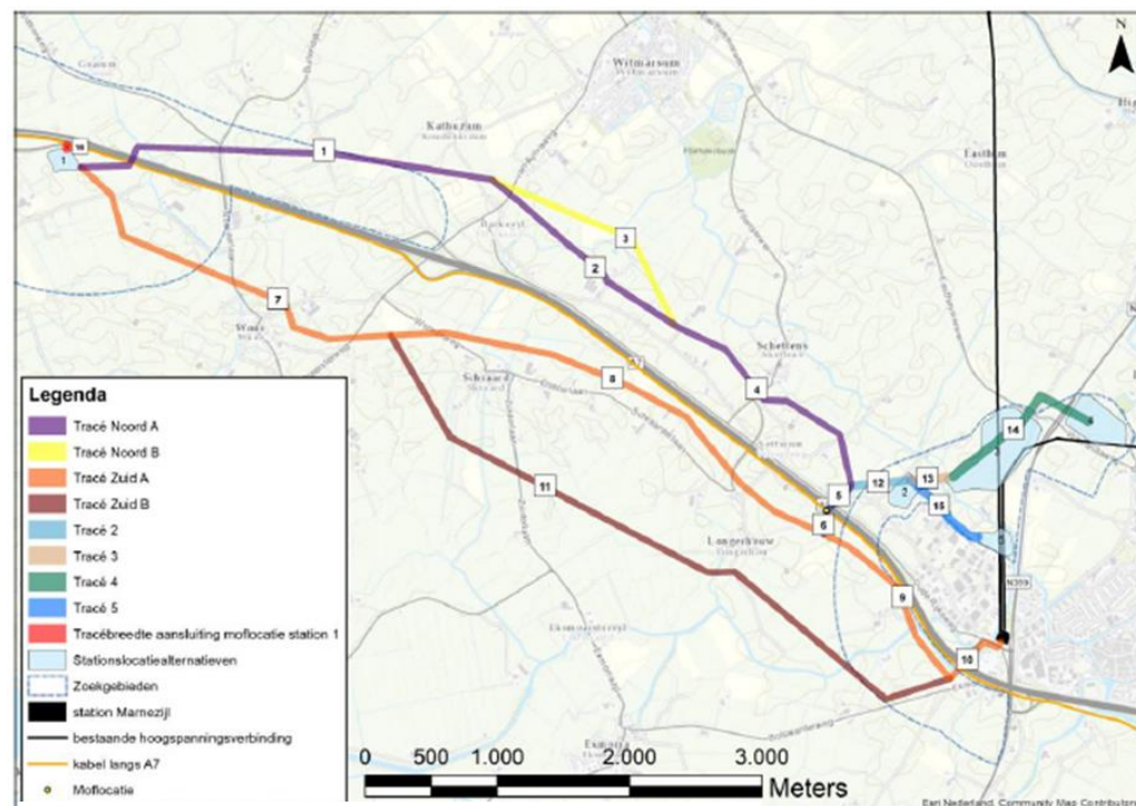
Afbeelding 4.5 Kabeltracéalternatieven
