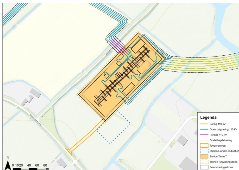
Afbeelding 2.3 Stationslocatie met bijbehorende voorzieningen
