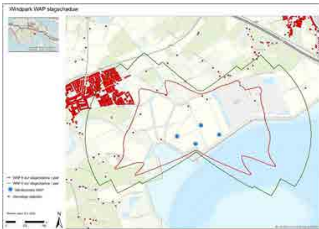
Figuur 17.2 Slagschaduwcontouren VKA
