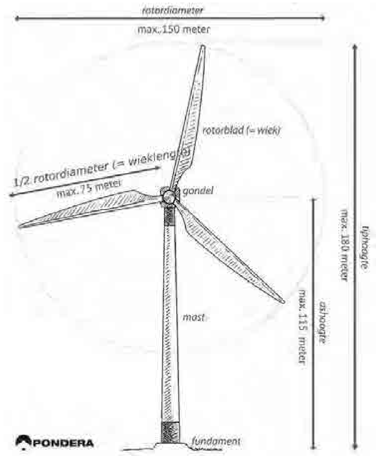
Figuur 4.2 Illustratie afmetingen en begrippen windturbine
