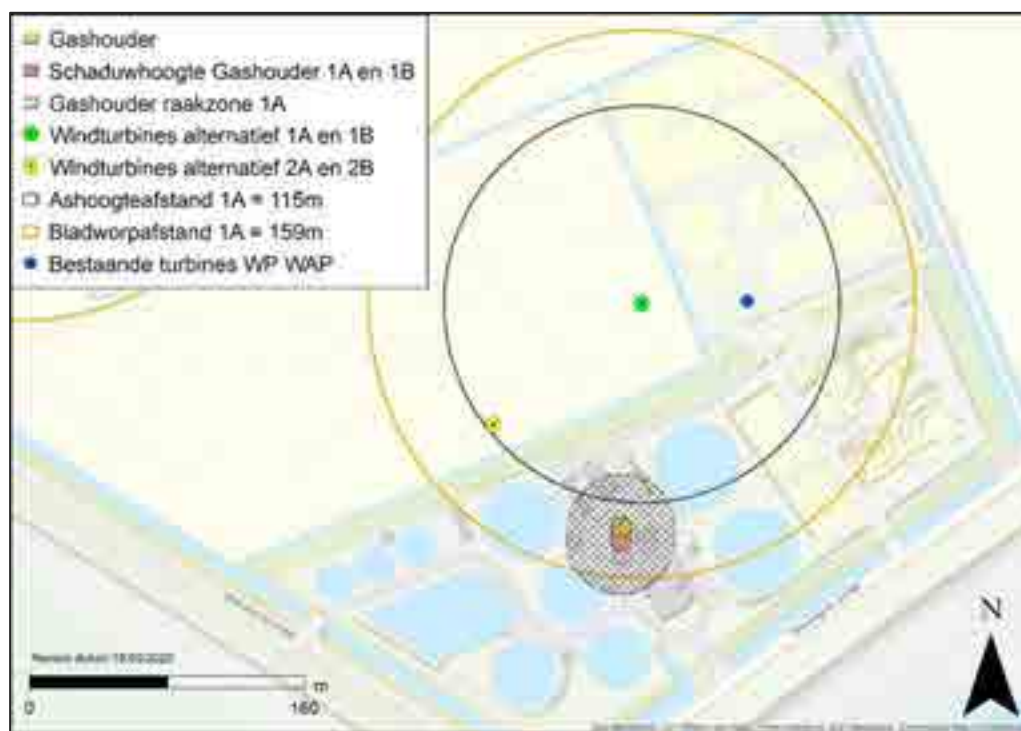
Figuur 4.1 Voorbeeldweergave trefzones gashouder alternatief 1A
