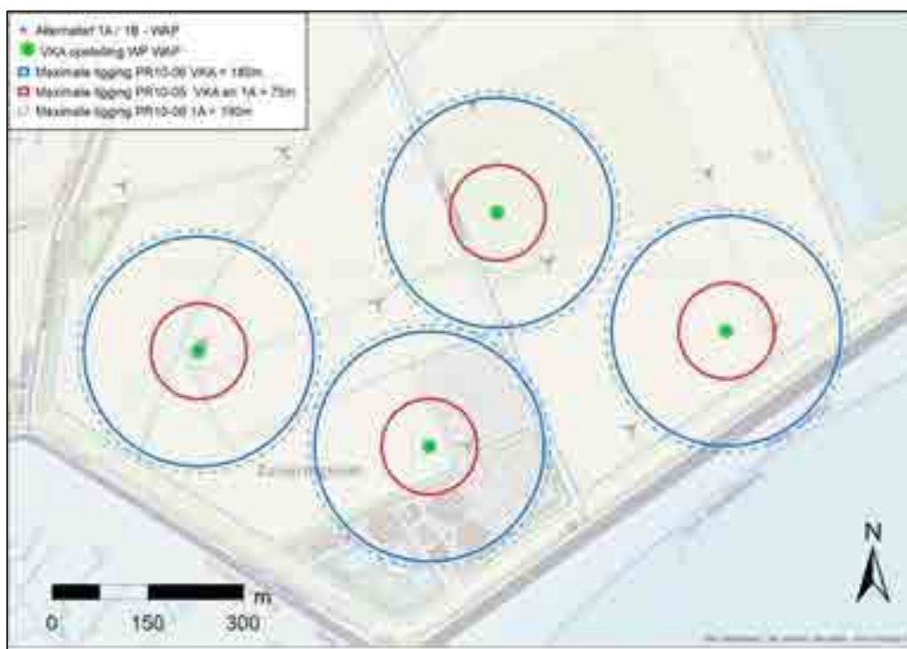
Figuur 17.6 Maximale ligging PR-contouren VKA
