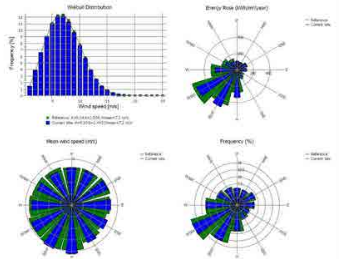
Figuur 2 Karakteristieken lokaal windklimaat op hoogte 100 meter
