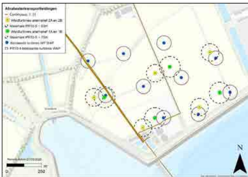
Figuur 1.1 Weergave afvalwaterleidingen i.r.t. bestaand windpark en beoogde windturbines
