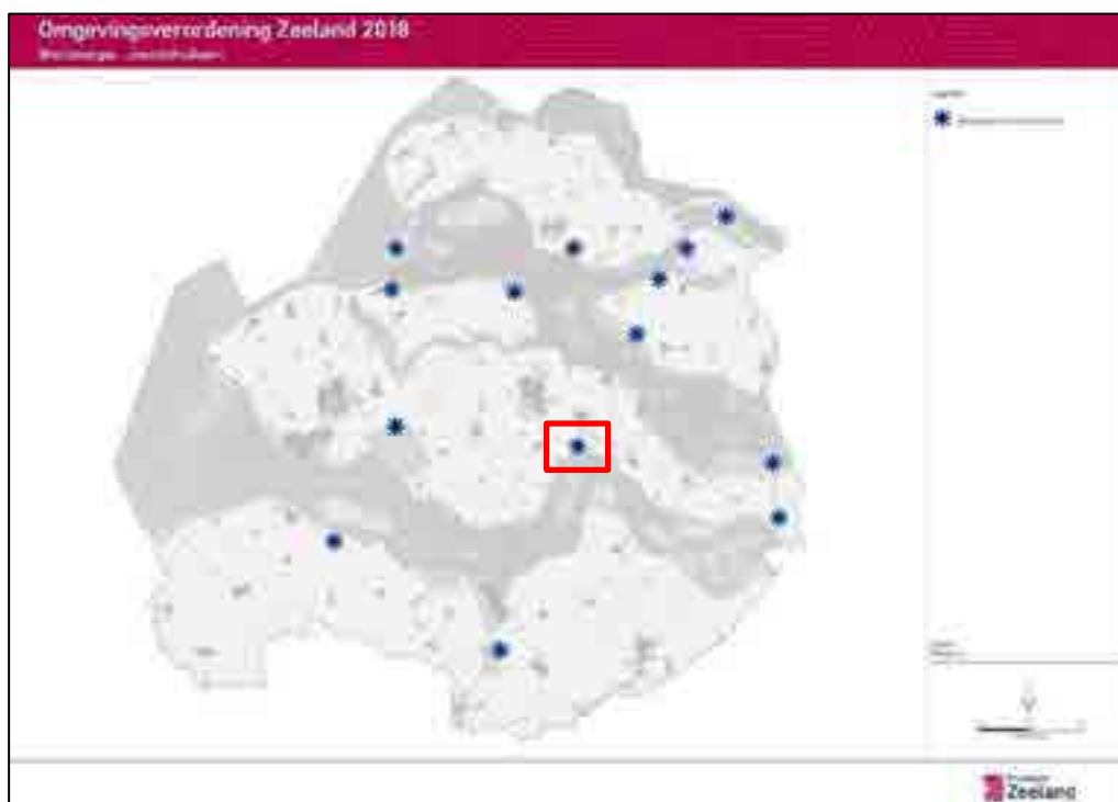
Figuur 3.5 Concentratieplaatsen windenergie (rood = locaties Kapelle)
