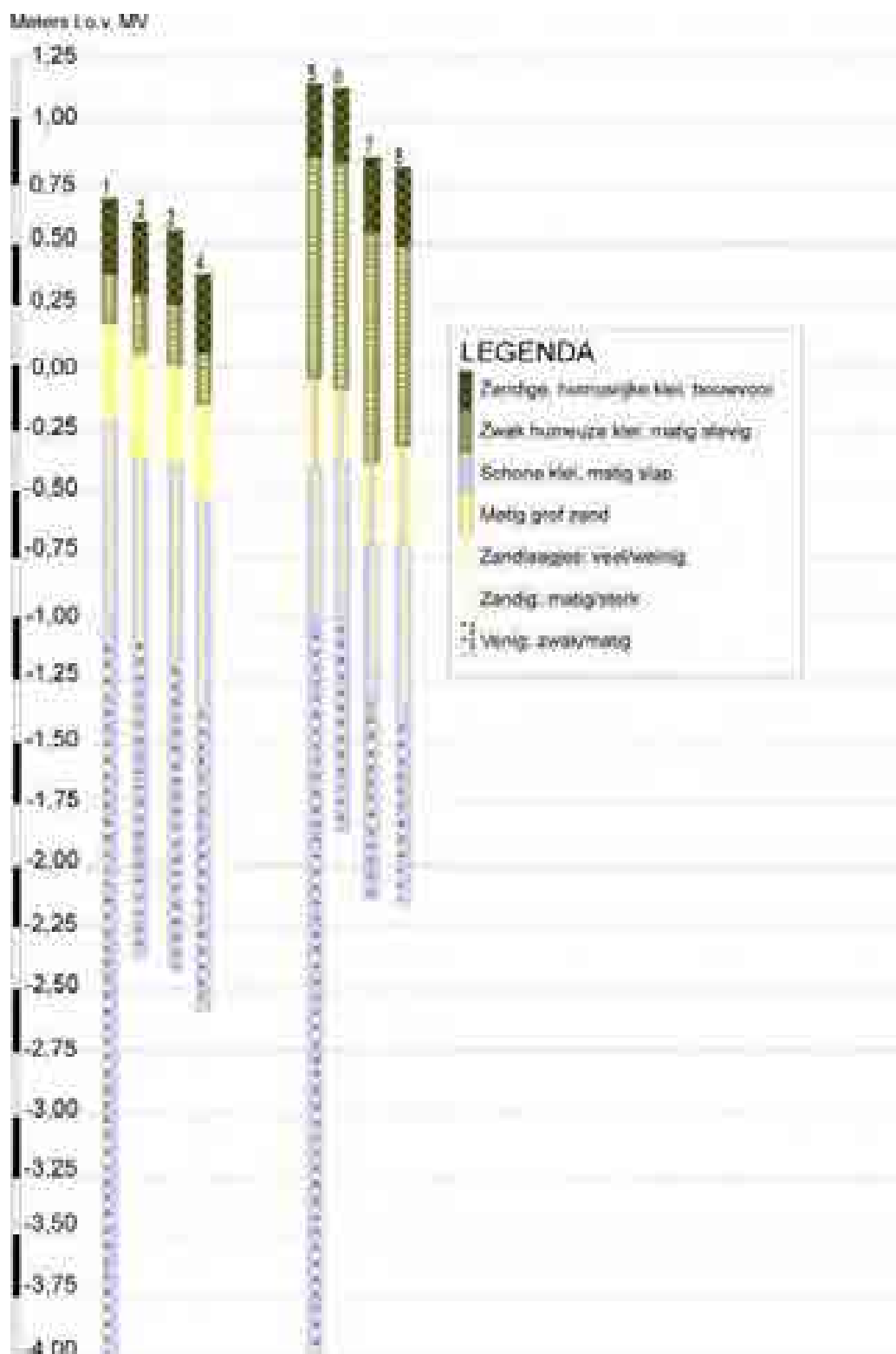
Figuur 28: Boorprofielen
