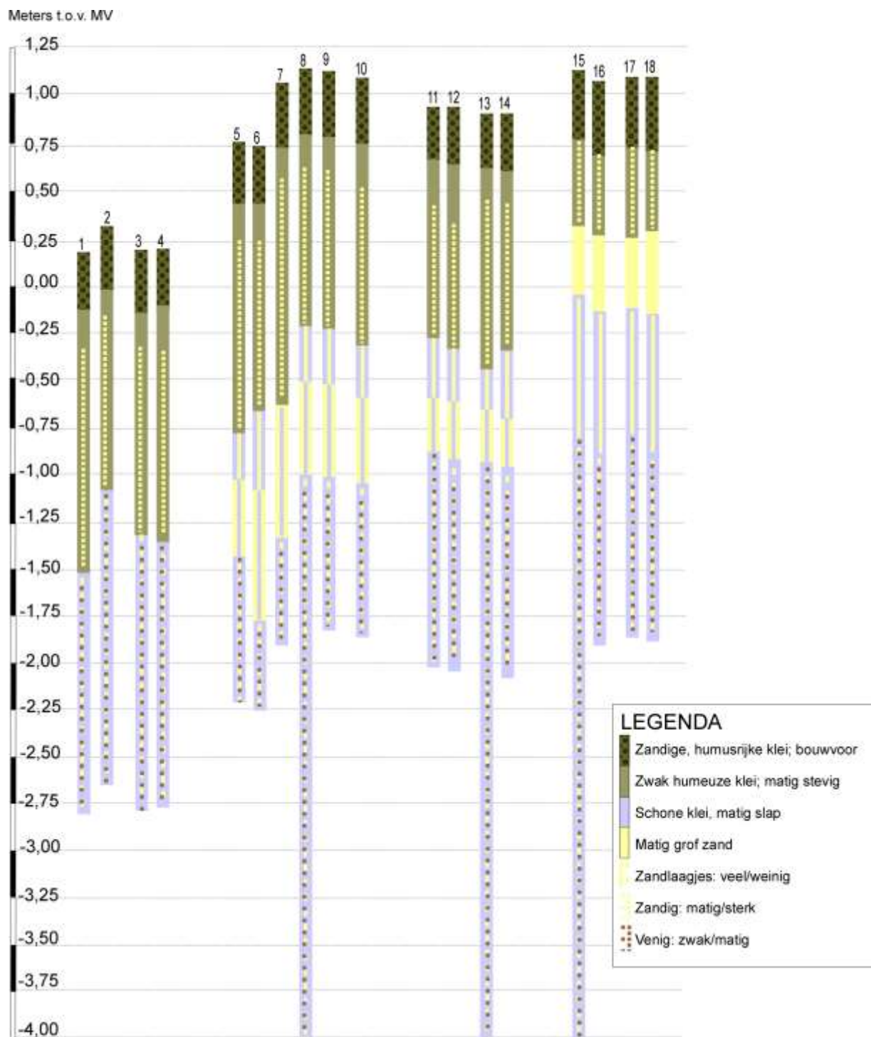
Figuur 27: Boorprofielen
