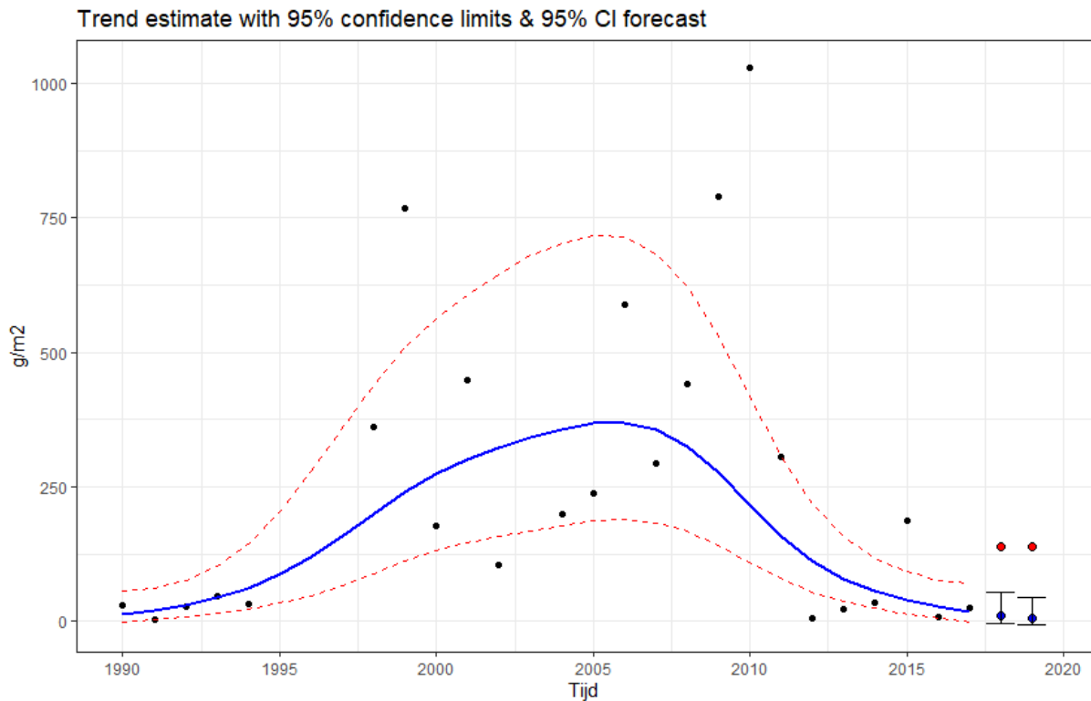
Figuur 4-12 Grafiek met de waarnemingen en de trend van de biomassa van kokkels in referentiegebied Vlie. Het 95% betrouwbaarheidsinterval rond de metingen is met rode stippellijnen weergegeven. De rode punten staan voor de gemeten waarden in 2018 en 2019 en de blauwe punten voor de trend met in de balk het 95% betrouwbaarheidsinterval.
