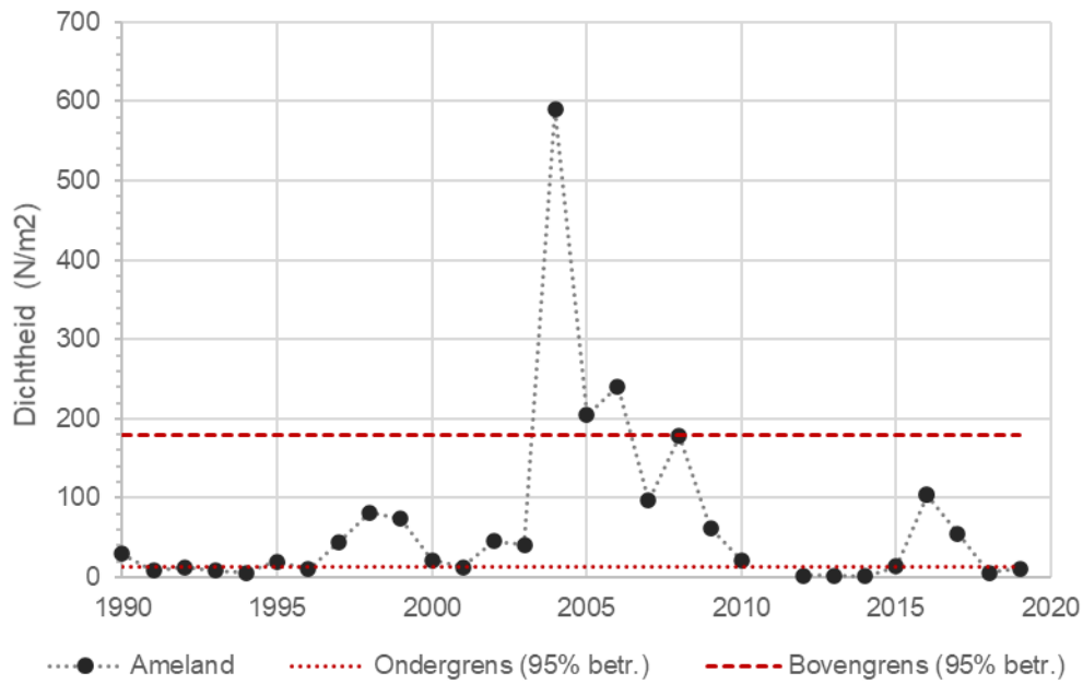
Figuur 4-6 Grafiek met de waarnemingen van de dichtheid van kokkels in referentiegebied Richel. Het 95% betrouwbaarheidsinterval rond het gemiddelde de metingen is met rode stippellijnen weergegeven.
