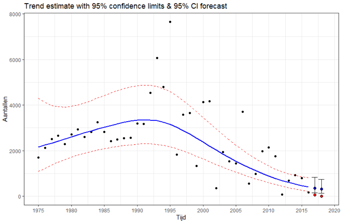
Figuur 5-30 Grafiek met de waarnemingen en de Trendspotter-trends van de aantallen Scholeksters op WG27 Friese kust (nabij het invloedsgebied). Het 95% betrouwbaarheidsinterval rond de metingen is met rode stippellijnen weergegeven. De rode punten staan voor de gemeten waarden in 2017 en 2018 en de blauwe punten voor de trend met in de balk het 95% betrouwbaarheidsinterval.
