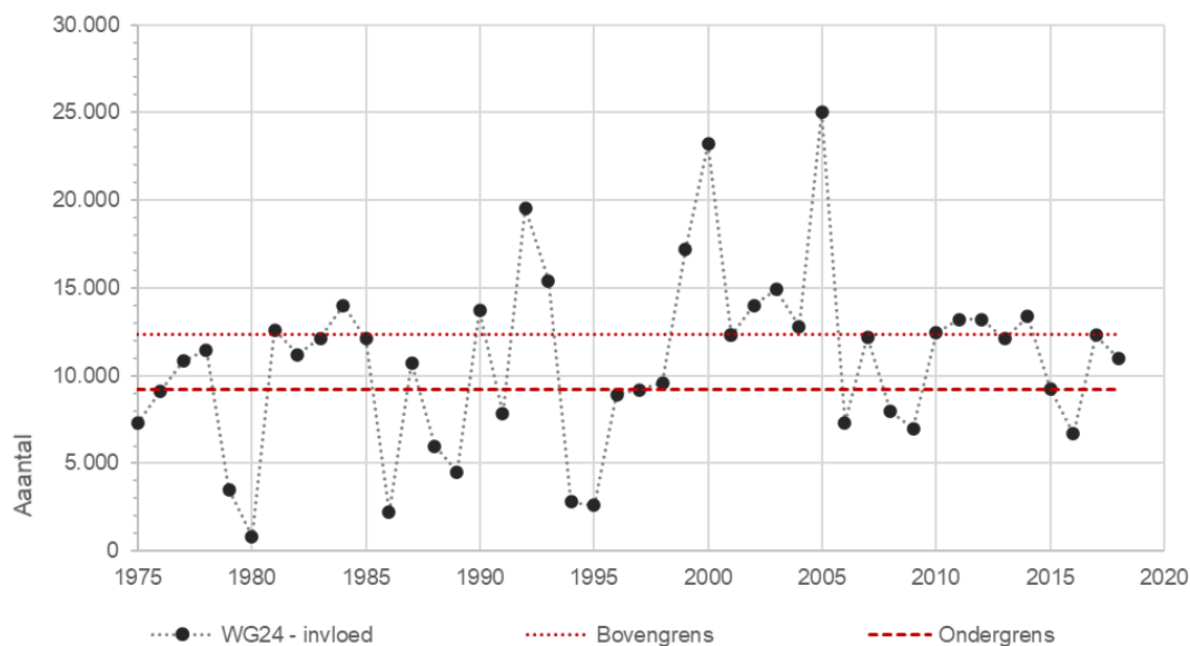
Figuur 5-29 Grafiek met de waarnemingen van de aantallen Scholeksters op WG24 Griend (nabij het invloedsgebied). Het 95% betrouwbaarheidsinterval rond het gemiddelde van de metingen is met rode stippellijnen weergegeven.
