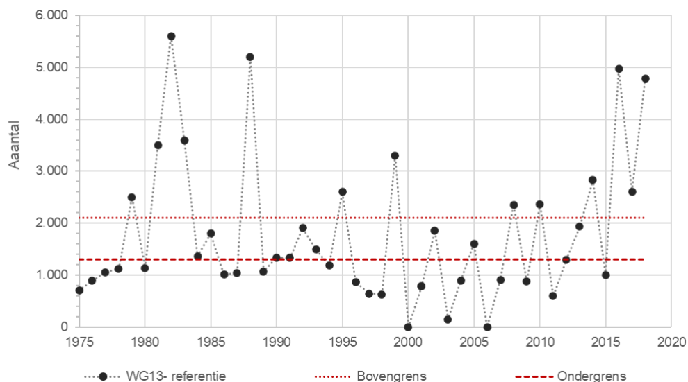
Figuur 5-33 Grafiek met de waarnemingen van de aantallen Scholeksters op WG13 Richel (nabij het invloedsgebied). Het 95% betrouwbaarheidsinterval rond het gemiddelde van de metingen is met rode stippellijnen weergegeven.
