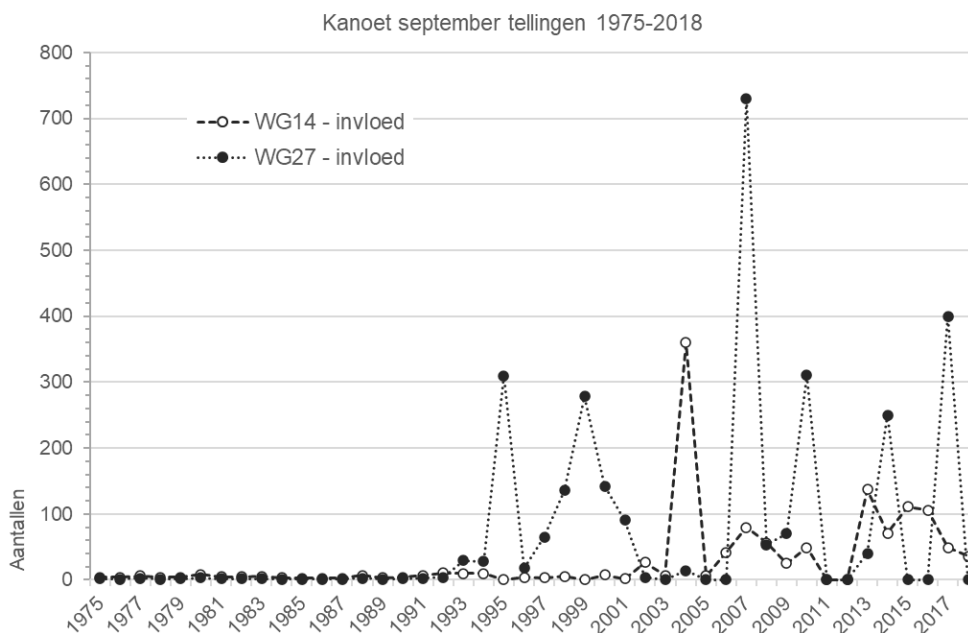
Figuur 5-25 Grafiek met de aantallen Kanoetstrandlopers in de maand september op de twee HVP's nabij het invloedsgebied langs de Friese vastelandskust.
