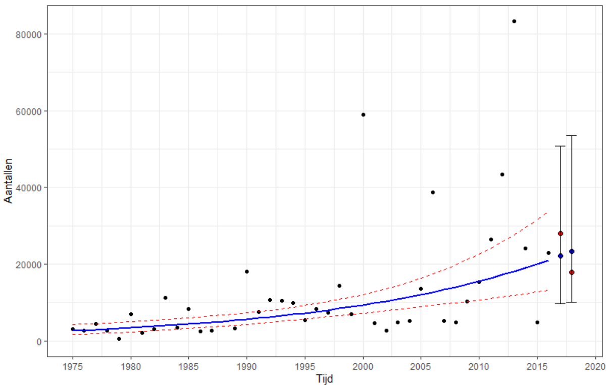
Figuur 5-19 Grafiek met de waarnemingen en de Trendspotter-trends van de aantallen Kanoetstrandlopers op WG12 Vlieland (referentiegebied). Het 95% betrouwbaarheidsinterval rond de metingen is met rode stippellijnen weergegeven. De rode punten staan voor de gemeten waarden in 2017 en 2018 en de blauwe punten voor de trend met in de balk het 95% betrouwbaarheidsinterval.
