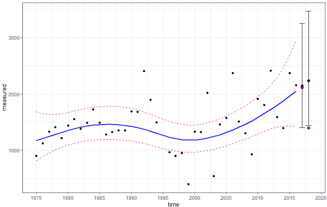
Figuur 5-28 Grafiek met de waarnemingen en de Trendspotter-trends van de aantallen Scholeksters op WG14 Harlingen (nabij het invloedsgebied). Het 95% betrouwbaarheidsinterval rond de metingen is met rode stippellijnen weergegeven. De rode punten staan voor de gemeten waarden in 2017 en 2018 en de blauwe punten voor de trend met in de balk het 95% betrouwbaarheidsinterval.
