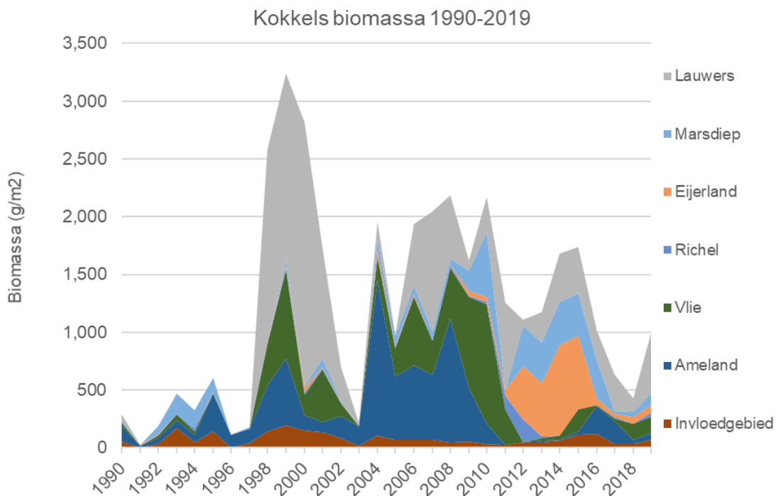
Figuur 4-2 Weergave van de biomassa van kokkels in de referentiegebieden en het invloedsgebied in de periode 1990-2019.
