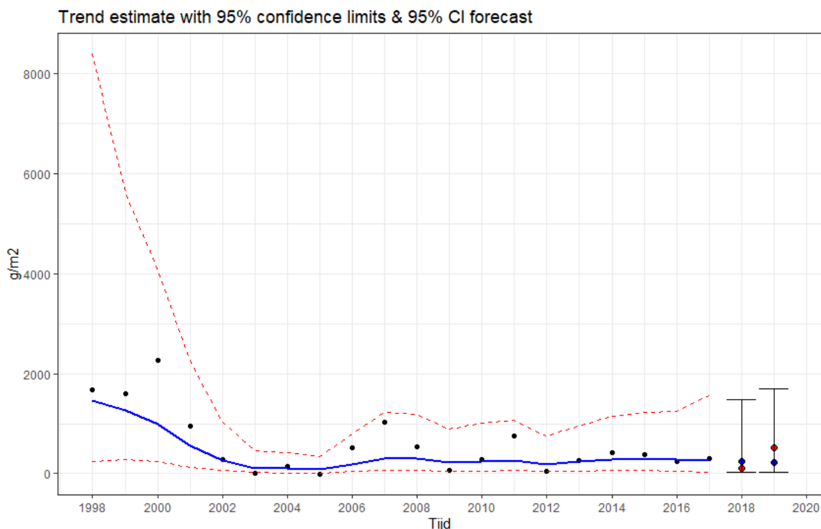
Figuur 4-16 Grafiek met de waarnemingen en de trend van de biomassa van kokkels in referentiegebied Lauwers. Het 95% betrouwbaarheidsinterval rond de metingen is met rode stippellijnen weergegeven. De rode punten staan voor de gemeten waarden in 2018 en 2019 en de blauwe punten voor de trend met in de balk het 95% betrouwbaarheidsinterval.
