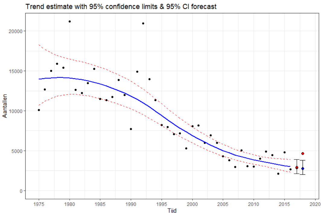
Figuur 5-31 Grafiek met de waarnemingen en de Trendspotter-trends van de aantallen Scholeksters op referentiegebied WG11 Texel. Het 95% betrouwbaarheidsinterval rond de metingen is met rode stippellijnen weergegeven. De rode punten staan voor de gemeten waarden in 2017 en 2018 en de blauwe punten voor de trend met in de balk het 95% betrouwbaarheidsinterval.
