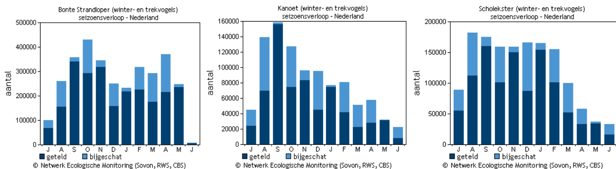
Figuur 5-2. Seizoensvoorkomen (juli t/m juni) per maand in Nederland, totaal aantallen per maand is uitgesplitst in geteld en bijschat (sovon.nl)
