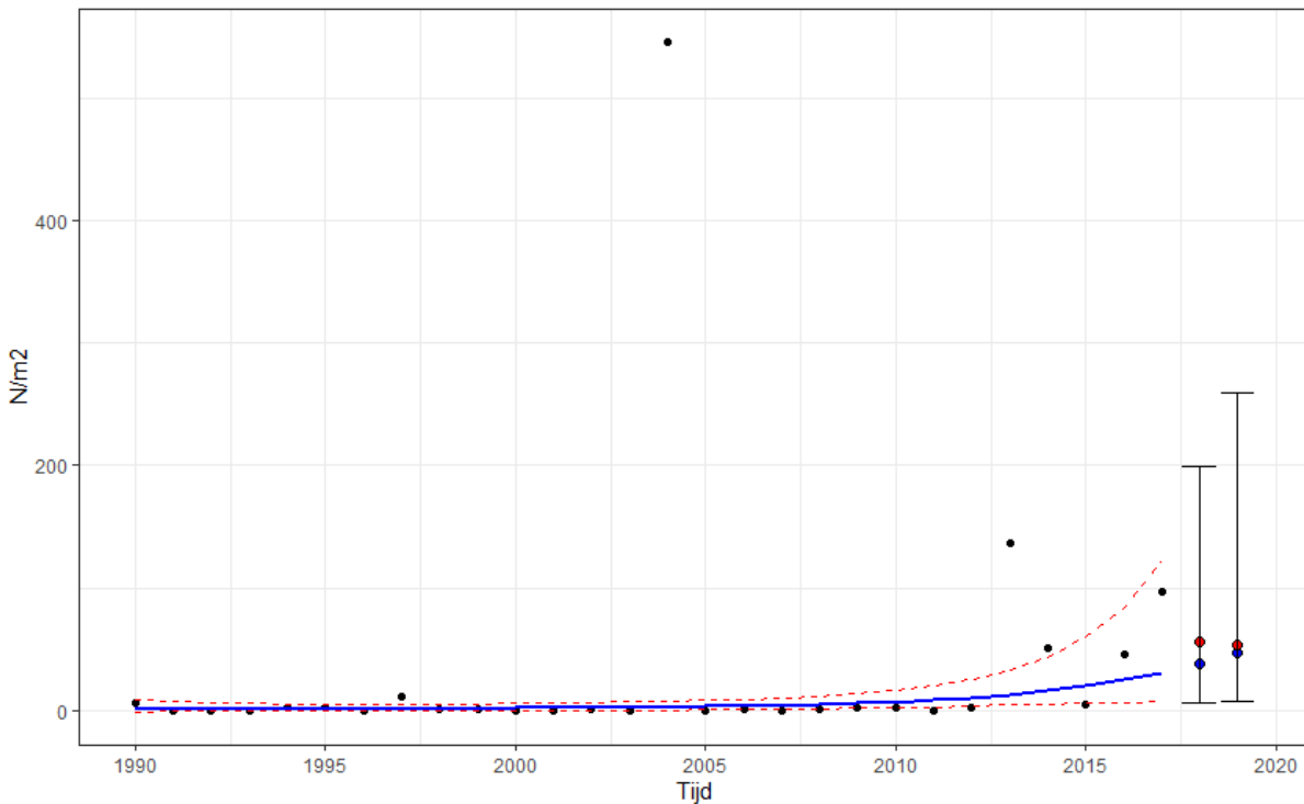
Figuur 4-22 Grafiek met de waarnemingen en de trend van de dichtheid van mosselen in referentiegebied Marsdiep. Het 95% betrouwbaarheidsinterval rond de metingen is met rode stippellijnen weergegeven. De rode punten staan voor de gemeten waarden in 2018 en 2019 en de blauwe punten voor de trend met in de balk het 95% betrouwbaarheidsinterval.
