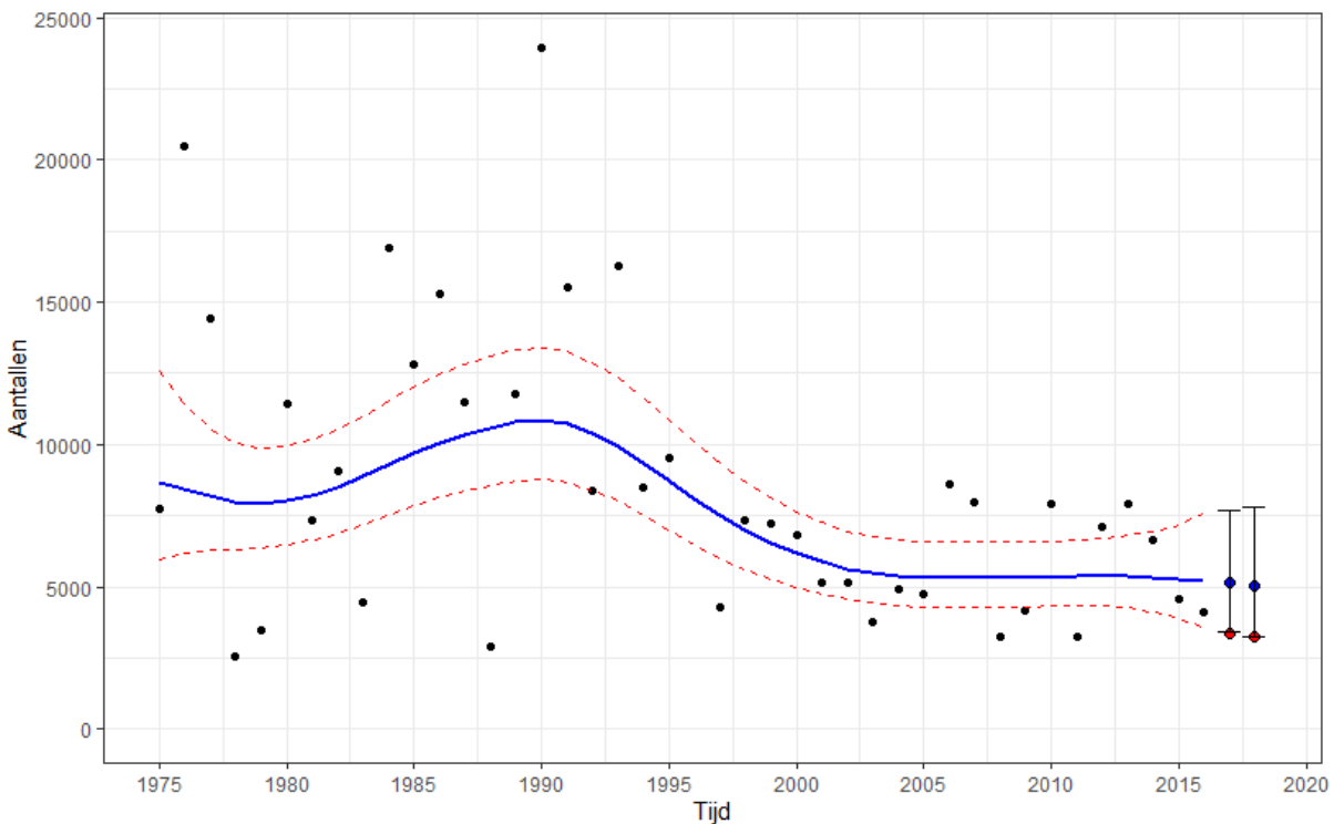
Figuur 5-35 Grafiek met de waarnemingen en de Trendspotter-trends van de aantallen Scholeksters op referentiegebied WG17 Balgzand. Het 95% betrouwbaarheidsinterval rond de metingen is met rode stippellijnen weergegeven. De rode punten staan voor de gemeten waarden in 2017 en 2018 en de blauwe punten voor de trend met in de balk het 95% betrouwbaarheidsinterval.
