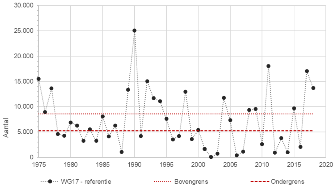
Figuur 5-11 Grafiek met de waarnemingen van de aantallen Bonte strandlopers op referentiegebied WG17 Balgzand. Het 95% betrouwbaarheidsinterval rond het gemiddelde van de metingen is met rode stippellijnen weergegeven.
