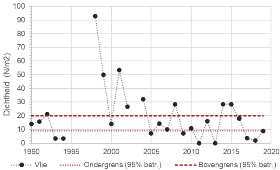
Figuur 4-33 Grafiek met de waarnemingen van de dichtheid van nonnetjes in referentiegebied Ameland. Het 95% betrouwbaarheidsinterval rond het gemiddelde de metingen is met rode stippellijnen weergegeven.
