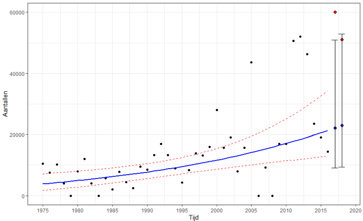
Figuur 5-9 Grafiek met de waarnemingen en de Trendspotter-trends van de aantallen Bonte strandlopers op WG13 Richel (referentiegebied). Het 95% betrouwbaarheidsinterval rond de metingen is met rode stippellijnen weergegeven. De rode punten staan voor de gemeten waarden in 2017 en 2018 en de blauwe punten voor de trend met in de balk het 95% betrouwbaarheidsinterval.
