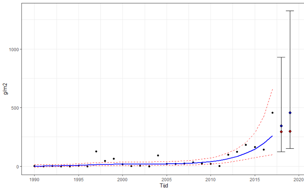
Figuur 4-24 Grafiek met de waarnemingen en de trend van de biomassa van mosselen in het invloedsgebied. Het 95% betrouwbaarheidsinterval rond de metingen is met rode stippellijnen weergegeven. De rode punten staan voor de gemeten waarden in 2018 en 2019 en de blauwe punten voor de trend met in de balk het 95% betrouwbaarheidsinterval.
