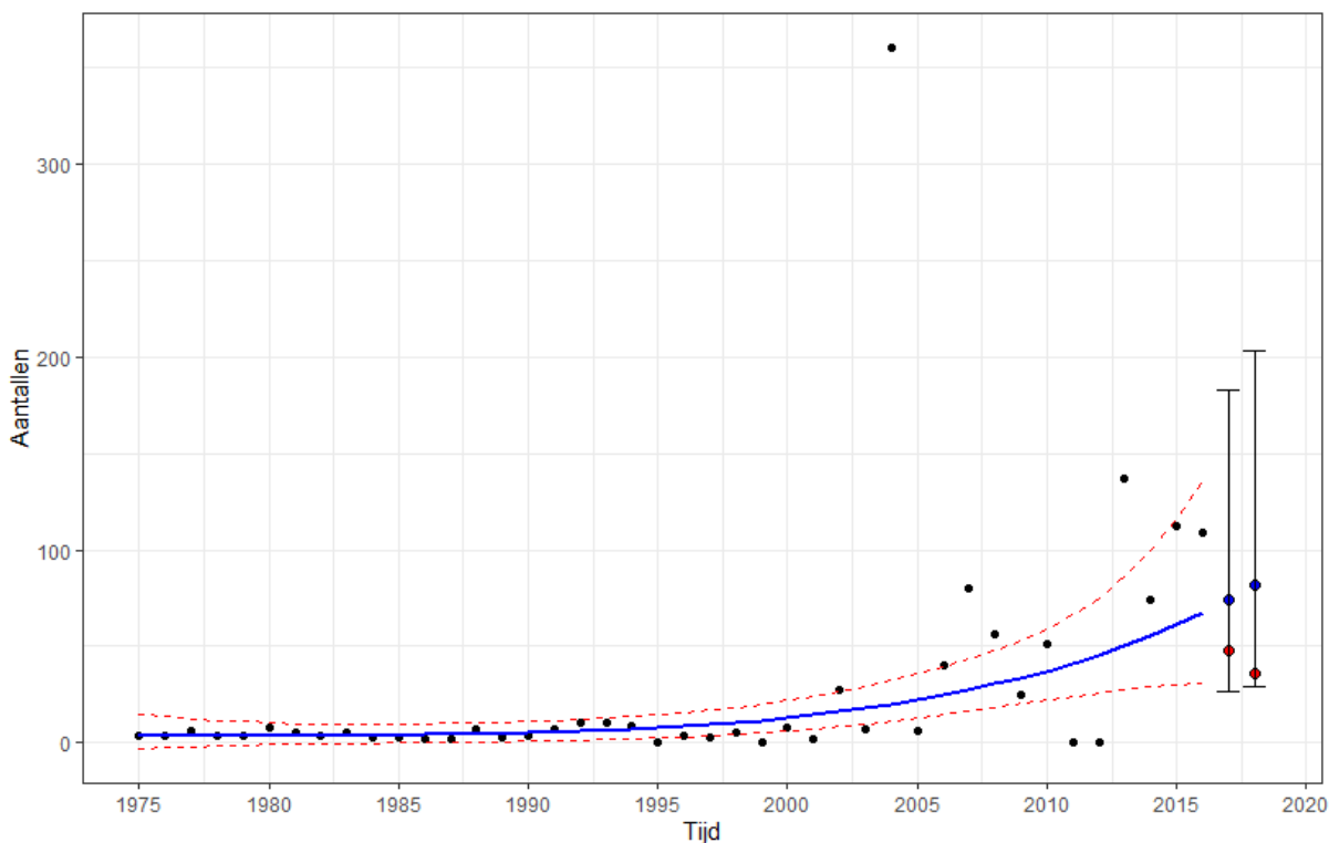
Figuur 5-15 Grafiek met de waarnemingen en de Trendspotter-trends van de aantallen Kanoetstrandlopers op WG14 Harlingen (nabij het invloedsgebied). Het 95% betrouwbaarheidsinterval rond de metingen is met rode stippellijnen weergegeven. De rode punten staan voor de gemeten waarden in 2017 en 2018 en de blauwe punten voor de trend met in de balk het 95% betrouwbaarheidsinterval.
