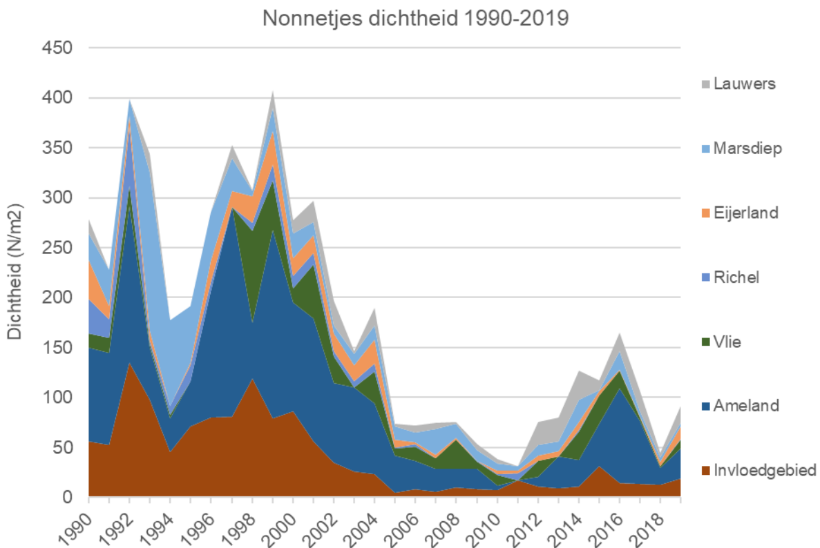
Figuur 4-29. Weergave van de dichtheid van nonnetjes in de referentiegebieden en het invloedsgebied in de periode 1990-2019.
