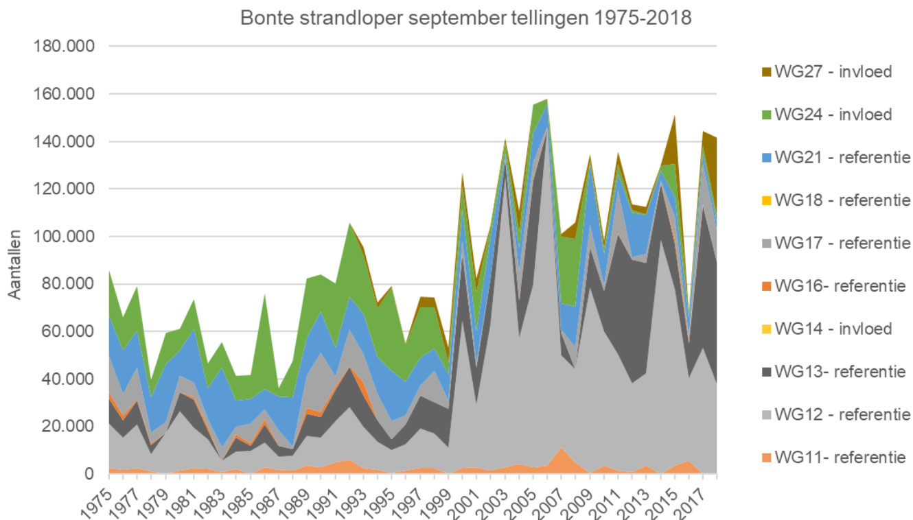
Figuur 5-3 Grafiek van het aantal bonte strandlopers in de maand september in de verschillende referentie HVP's en de HVP's bij het invloedsgebied.
