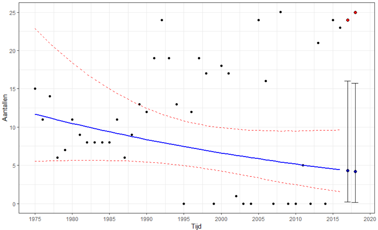
Figuur 5-12 Grafiek met de waarnemingen en de Trendspotter-trends van de aantallen Bonte strandlopers op WG18 Den Helder (referentiegebied). Het 95% betrouwbaarheidsinterval rond de metingen is met rode stippellijnen weergegeven. De rode punten staan voor de gemeten waarden in 2017 en 2018 en de blauwe punten voor de trend met in de balk het 95% betrouwbaarheidsinterval.
