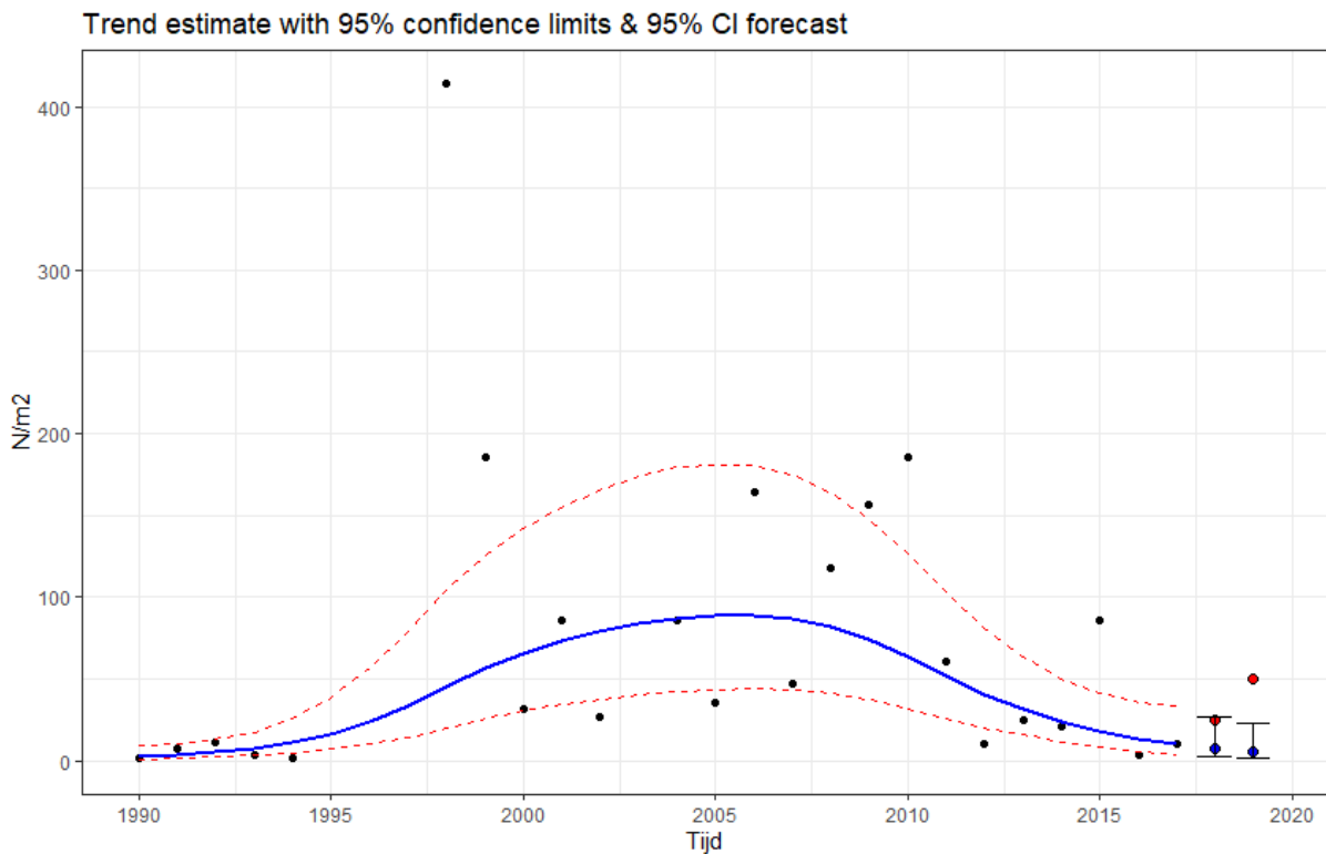
Figuur 4-5 Grafiek met de waarnemingen en de trend van de dichtheid van kokkels in referentiegebied Vlie. Het 95% betrouwbaarheidsinterval rond de metingen is met rode stippellijnen weergegeven. De rode punten staan voor de gemeten waarden in 2018 en 2019 en de blauwe punten voor de trend met in de balk het 95% betrouwbaarheidsinterval.
