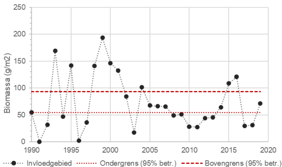
Figuur 4-10 Grafiek met de waarnemingen van de biomassa van kokkels in het Invloedsgebied. Het 95% betrouwbaarheidsinterval rond het gemiddelde de metingen is met rode stippellijnen weergegeven.
