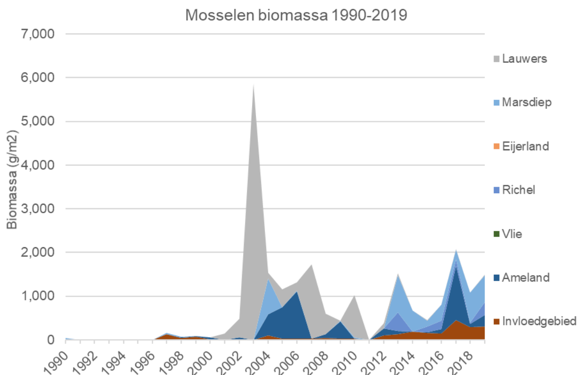
Figuur 4-18 Weergave van de biomassa van mosselen in de referentiegebieden en het invloedsgebied in de periode 1990-2019.
