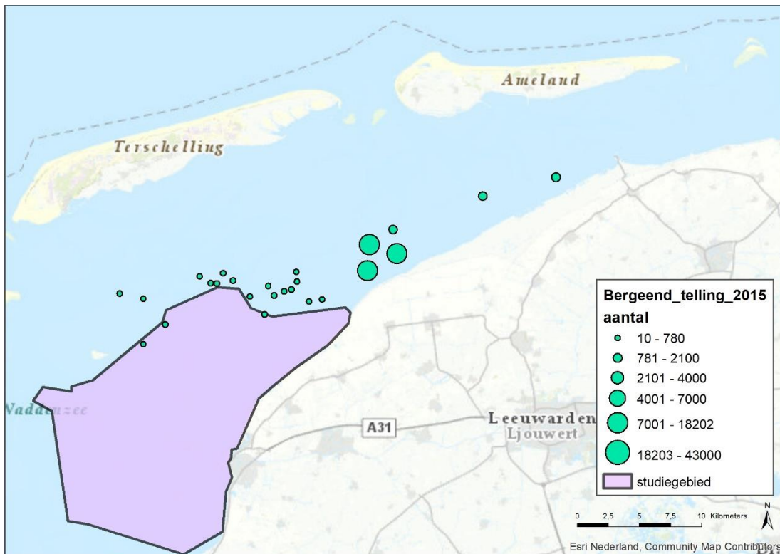
Figuur 6-4 Aantallen ruiende bergeenden in en rondom het studiegebied in 2015.
