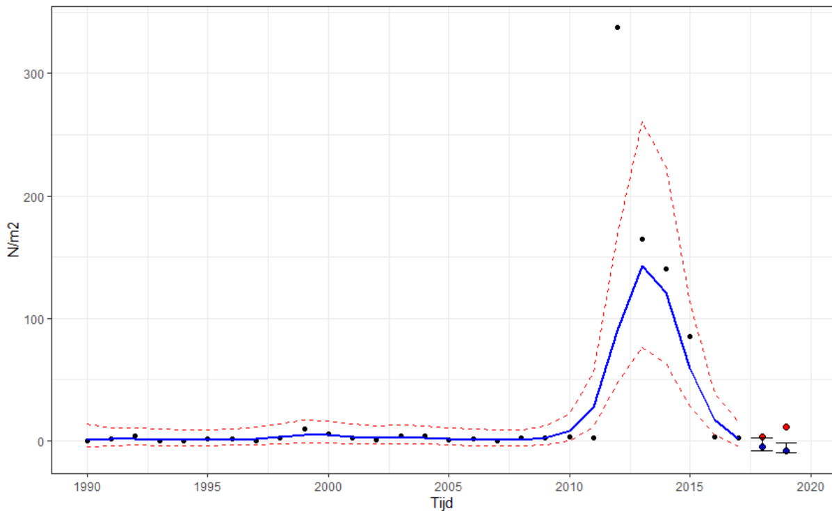
Figuur 4-7 Grafiek met de waarnemingen en de trend van de dichtheid van kokkels in referentiegebied Eierland. Het 95% betrouwbaarheidsinterval rond de metingen is met rode stippellijnen weergegeven. De rode punten staan voor de gemeten waarden in 2018 en 2019 en de blauwe punten voor de trend met in de balk het 95% betrouwbaarheidsinterval.
