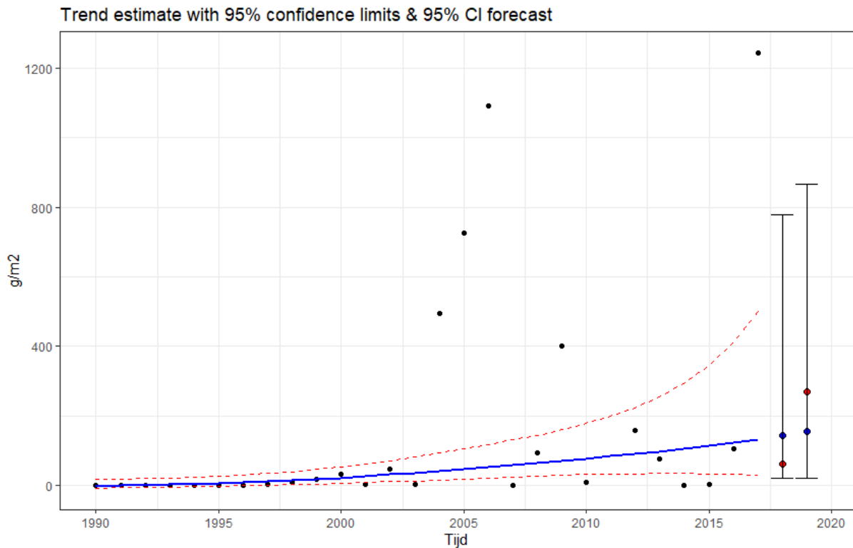
Figuur 4-25 Grafiek met de waarnemingen en de trend van de biomassa van mosselen in referentiegebied Ameland. Het 95% betrouwbaarheidsinterval rond de metingen is met rode stippellijnen weergegeven. De rode punten staan voor de gemeten waarden in 2018 en 2019 en de blauwe punten voor de trend met in de balk het 95% betrouwbaarheidsinterval.
