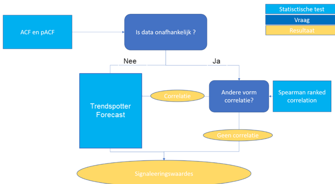
Figuur 3-2: Beslisschema, geeft aan welk statistische pad er doorlopen moet worden om tot signaleringswaardes te komen.
