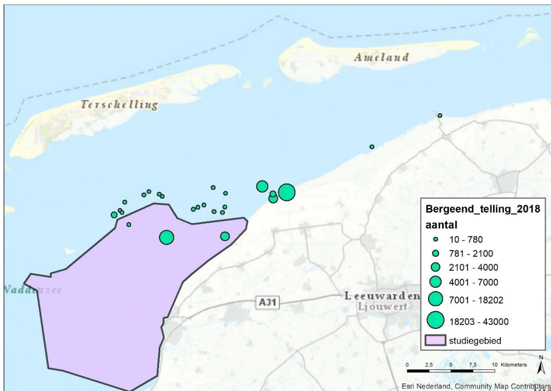
Figuur 6-7 Aantallen ruiende bergeenden in en rondom het studiegebied in 2018.
