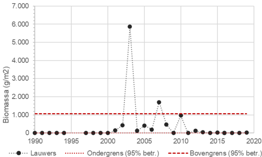
Figuur 4-28 Grafiek met de waarnemingen van de biomassa van mosselen in referentiegebied Lauwers. Het 95% betrouwbaarheidsinterval rond het gemiddelde de metingen is met rode stippellijnen weergegeven.
