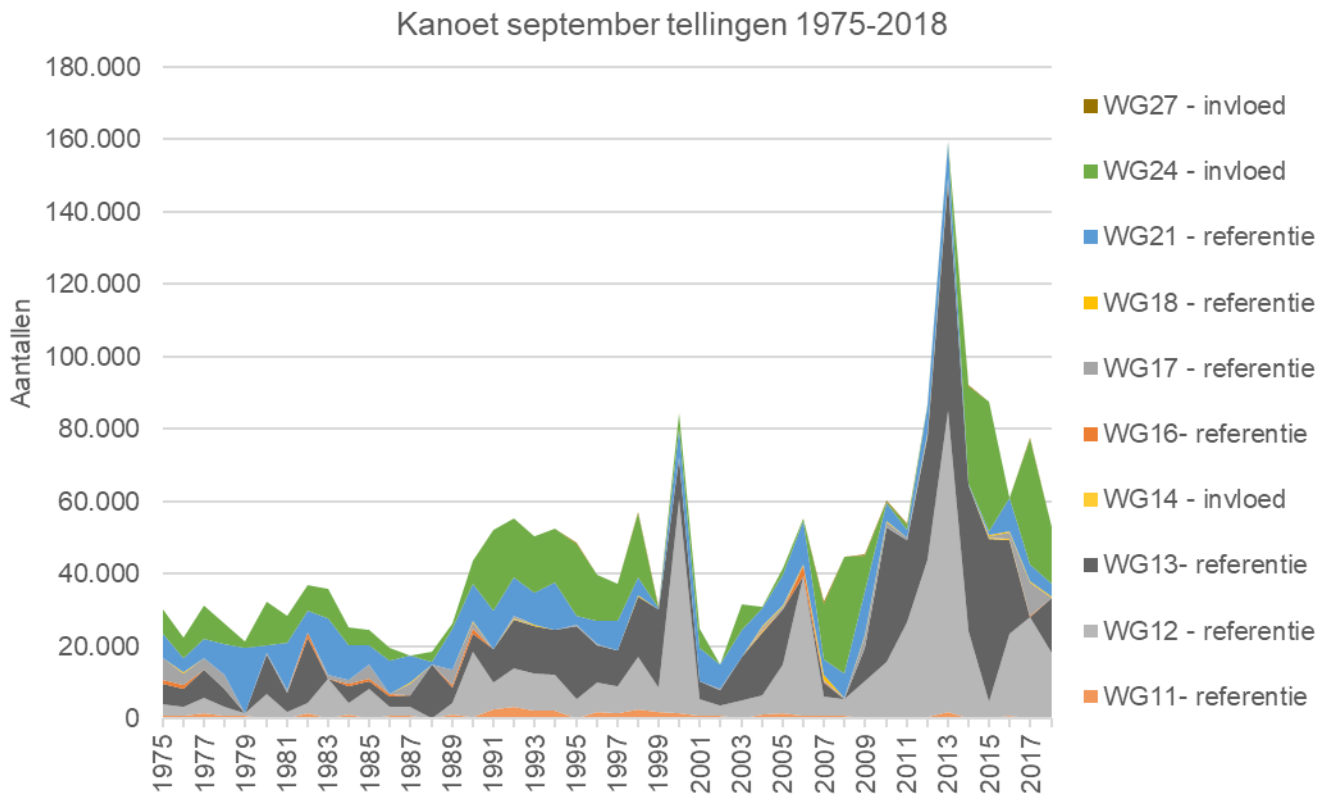
Figuur 5-14 Grafiek van het aantal Kanoetstrandlopers in de maand september in de verschillende referentie HVP's en de HVP's bij het invloedsgebied.
