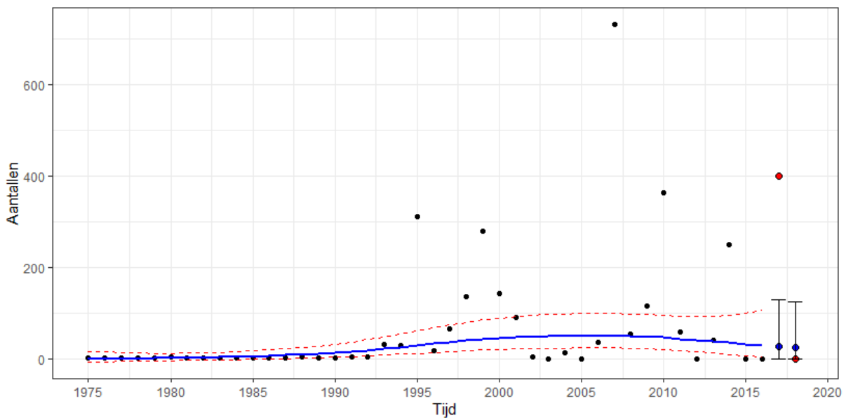
Figuur 5-17 Grafiek met de waarnemingen en de Trendspotter-trends van de aantallen Kanoetstrandlopers op WG27 Friese kust (nabij het invloedsgebied). Het 95% betrouwbaarheidsinterval rond de metingen is met rode stippellijnen weergegeven. De rode punten staan voor de gemeten waarden in 2017 en 2018 en de blauwe punten voor de trend met in de balk het 95% betrouwbaarheidsinterval.
