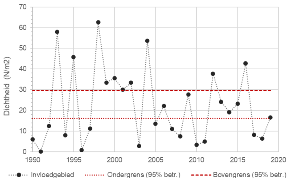
Figuur 4-3 Grafiek met de waarnemingen van de dichtheid van kokkels in het Invloedsgebied. Het 95% betrouwbaarheidsinterval rond het gemiddelde de metingen is met rode stippellijnen weergegeven.
