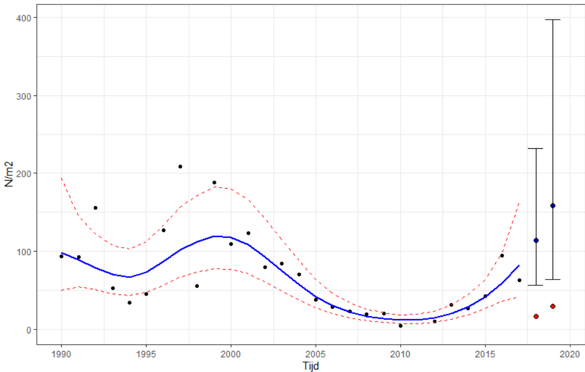
Figuur 4-32 Grafiek met de waarnemingen en de trend van de dichtheid van nonnetjes in referentiegebied Ameland. Het 95% betrouwbaarheidsinterval rond de metingen is met rode stippellijnen weergegeven. De rode punten staan voor de gemeten waarden in 2018 en 2019 en de blauwe punten voor de trend met in de balk het 95% betrouwbaarheidsinterval.
