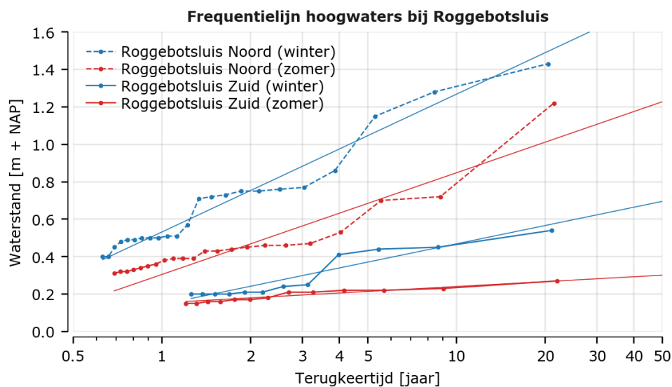
Abbeelding 5.5 Overschrijdingsfrequentielijnen van hoogwaters aan beide zijden van de Roggebotsluis op basis van metingen van de afgelopen decennia
