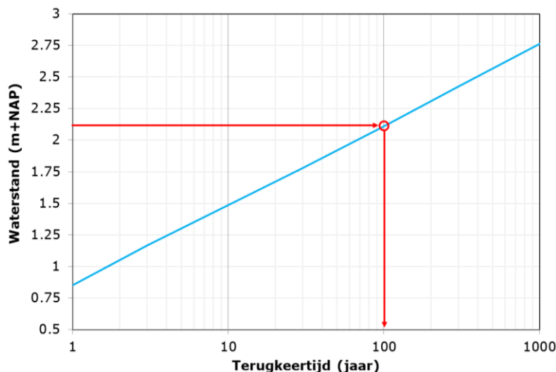
Afbeelding 5.4 Frequentieline van de waterstand voor de representatieve locatie uit afbeelding 5.3
