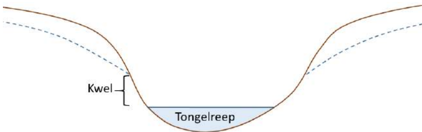
Figuur 5-3 Schematische dwarsdoorsnede Tongelreep
