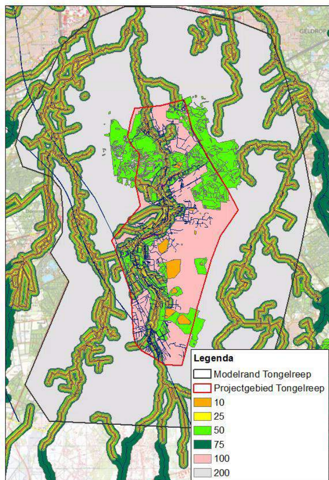
Figuur 4-3 Verfijningspolygoenen met maximale afstand tussen twee rekenpunten per zone.
