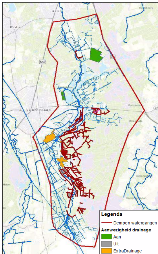
Figuur 7-10 Maatregelen inzichtscenario 4 – minimaal dempen
