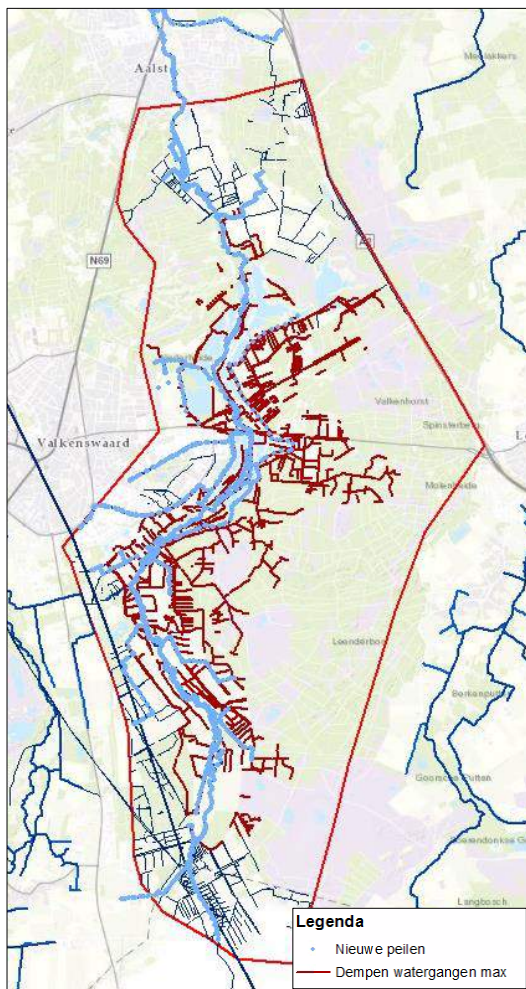
Figuur 7-1 Maatregelen in het maximaal scenario.
