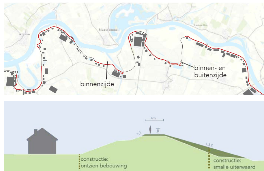
Afbeelding 3.9 Belemmeringen binnen- en/of buitenzijde, dus constructies
