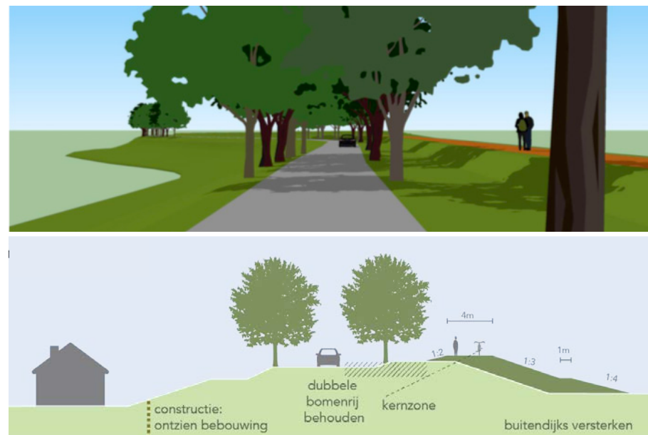
Afbeelding 3.14 Verbrede tuimelkade met behouden bomen
