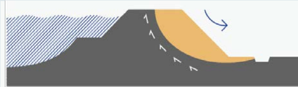
2 Stabiliteit: als er langdurig water tegen de dijk staat, vult deze zich met water en kan de dijk 'slap' worden. Hierdoor wordt deze instabiel en kan bezwijken. Dit gebeurt meestal aan de binnendijkse kant, door de waterdruk vanuit de rivier.
