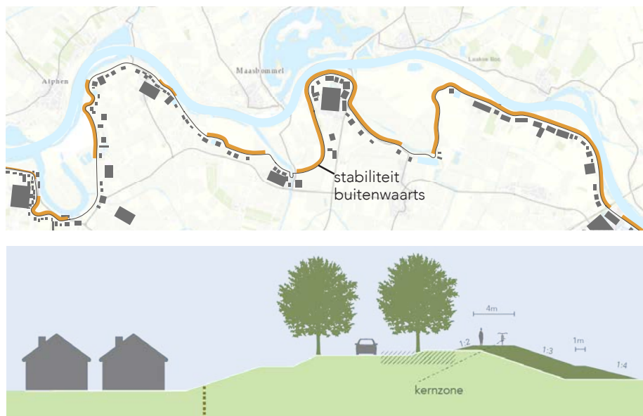
Afbeelding 3.8 Ruimte aan de buitenzijde voor benodigde buitenwaartse stabiliteit
