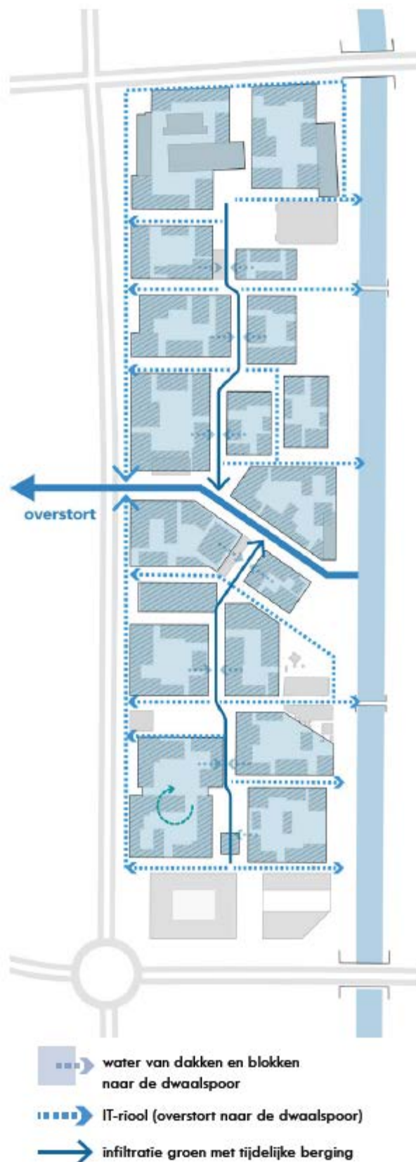
Figuur 14. Voorgesteld systeem waterberging deelgebied 5 (bron: VOSP)
