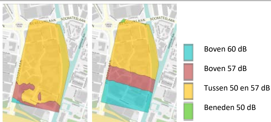
Figuur 25. Wegverkeerslawaaï vanwege de A12 op 10 meter (links) en 40 meter hoogte (rechts)
