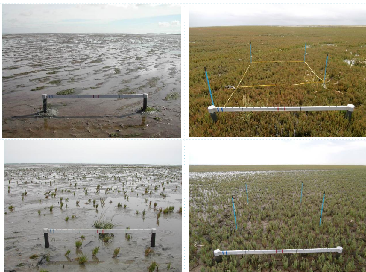
Figuur 3.4. Ontwikkeling (pre-)pionierzone met voornamelijk Zeekraal en (sporadisch) Engels slijkgras bij pq 38 (boven) en pq 44 (onder). Links situatie in 2007 en rechts die in 2018.
