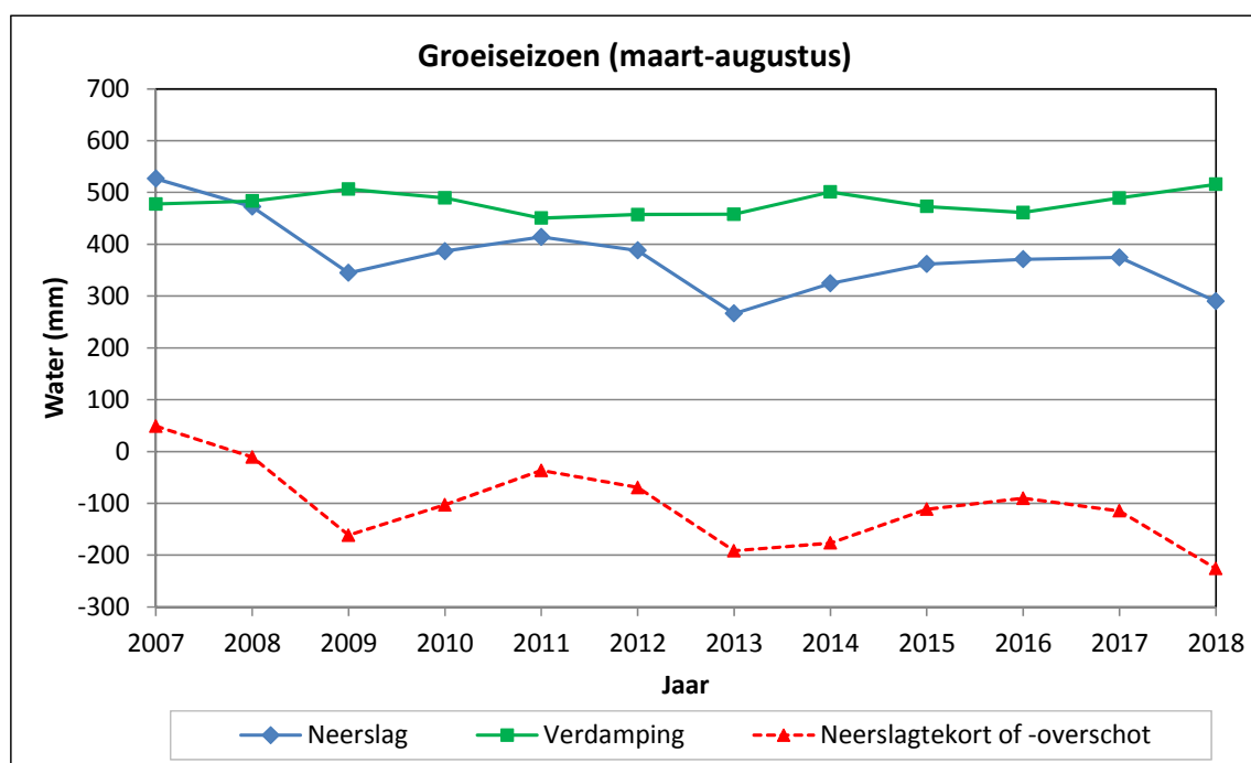
Figuur 3.15 Neerslag, verdamping en neerslagtekort in het groeiseizoen (maart t/m augustus) voor Lauwersoog (station 277) op basis van KNMI-gegevens.
