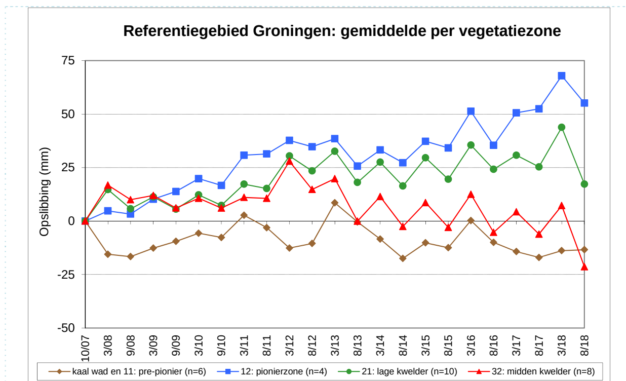
Figuur 3.6 Gemiddelde cumulatieve netto-opslibbing (mm) per vegetatiezone (met SALT97 code) op basis van de SEB-metingen in het referentiegebied West-Groningen vanaf 2007-augustus 2018.
