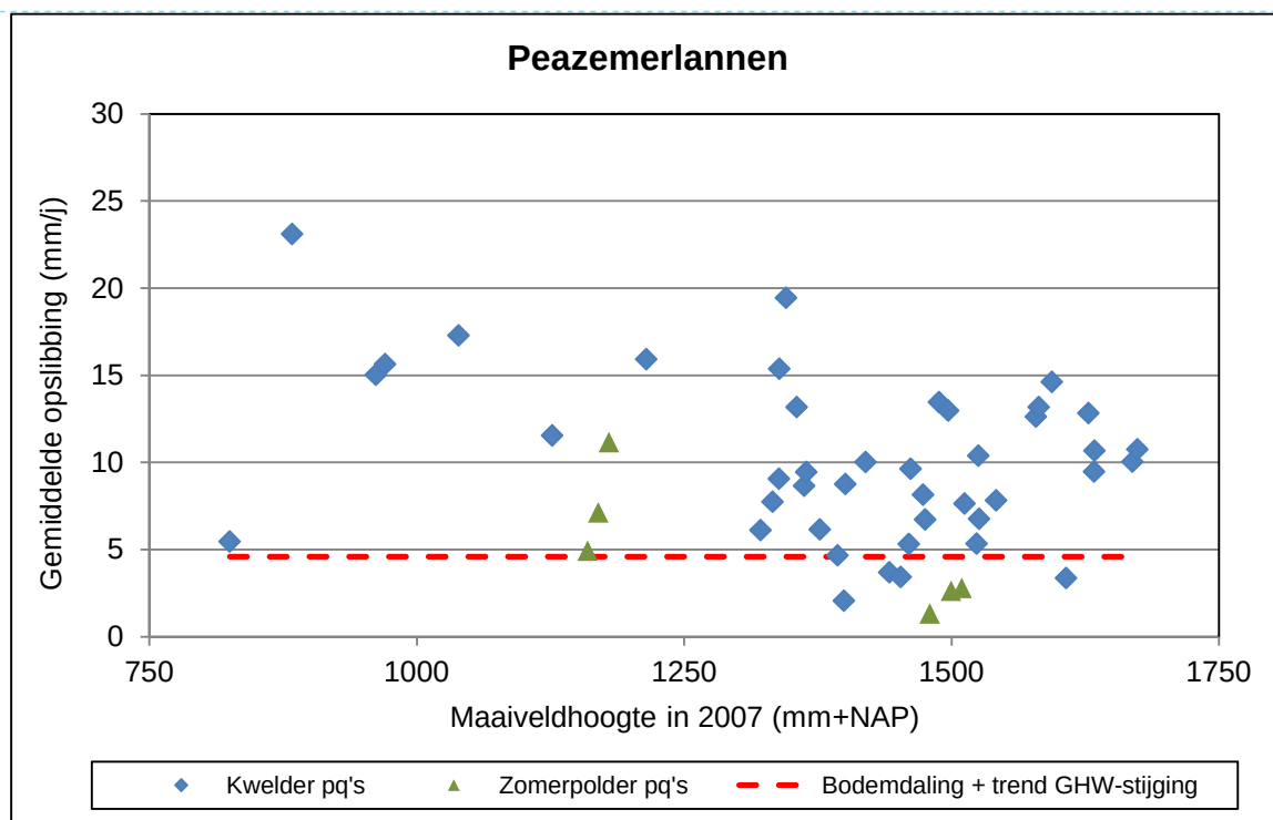
Figuur 3.2 Gemiddelde netto-opslibbing in mm/j per pq over de periode 2007-2018 in de Peazemerlannen. De rode stippellijn geeft de gemiddelde jaarlijkse bodemdaling over de periode 2007 t/m 2018 van 3,6 mm/j (NAM, 2018; zie ook Figuur 1.3) + de trend in GHW-stijging van 1 mm berekend voor Lauwersoog over de periode 1988 t/m 2018 (zie Figuur 3.13).
