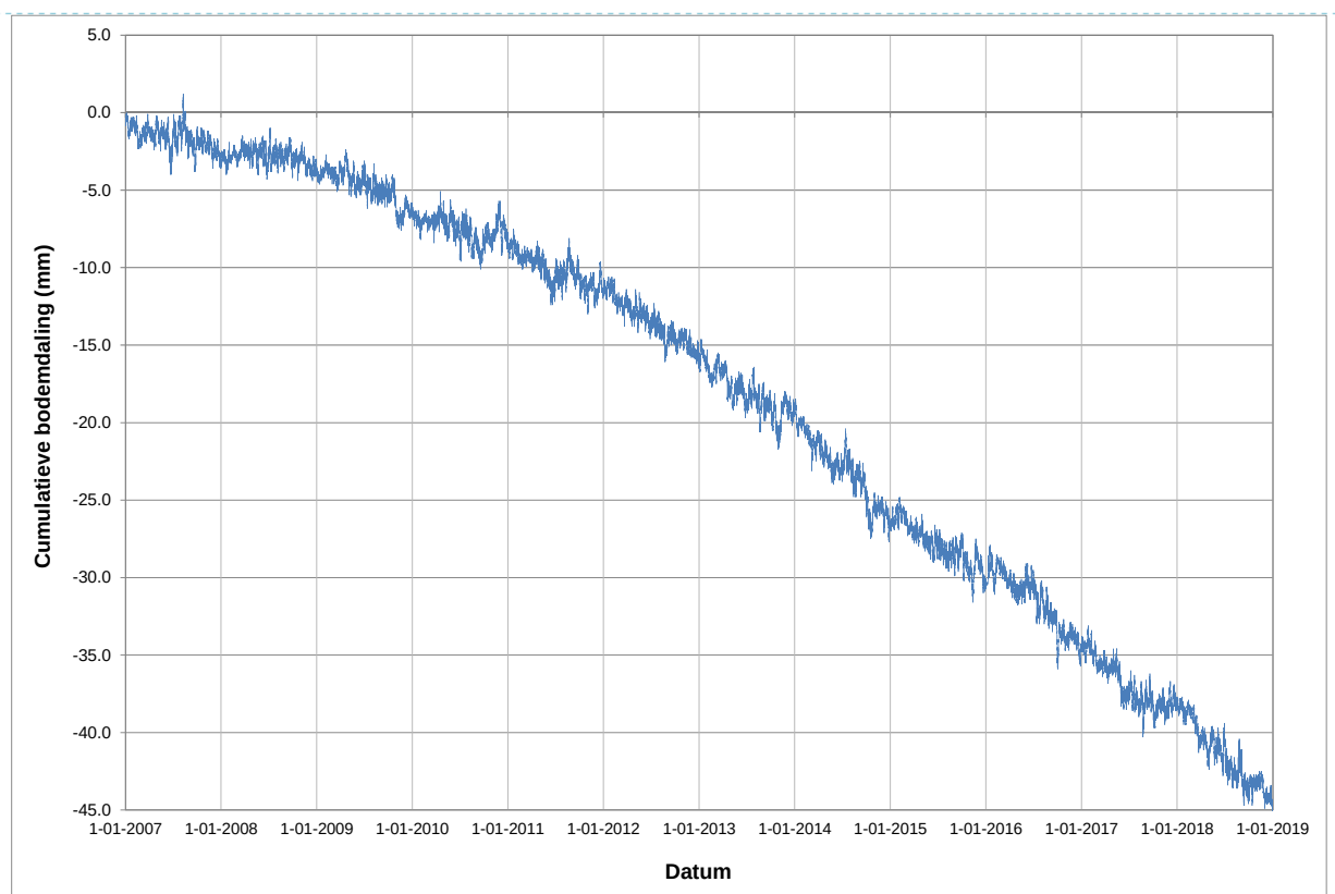
Figuur 1.3 De door gaswinning veroorzaakte diepe bodemdaling (mm) gemeten met behulp van de continue GPS-logger van de locatie Moddergat (NAM, 2019). Op basis van deze metingen is in dit rapport over de monitoringperiode van 2007-2018 een gemiddelde daling van 3,6 mm/j aangehouden.
