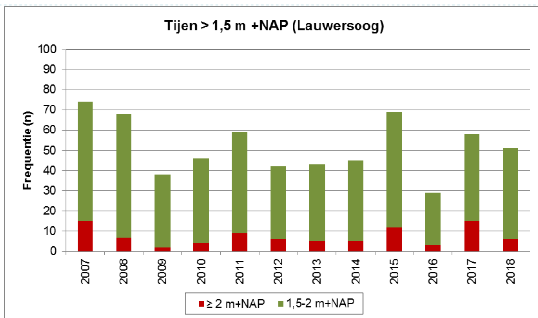
Figuur 3.14 Aantal tijen >1,5 m +NAP voor Lauwersoog van 2007-2018 op basis van RWS-data.
