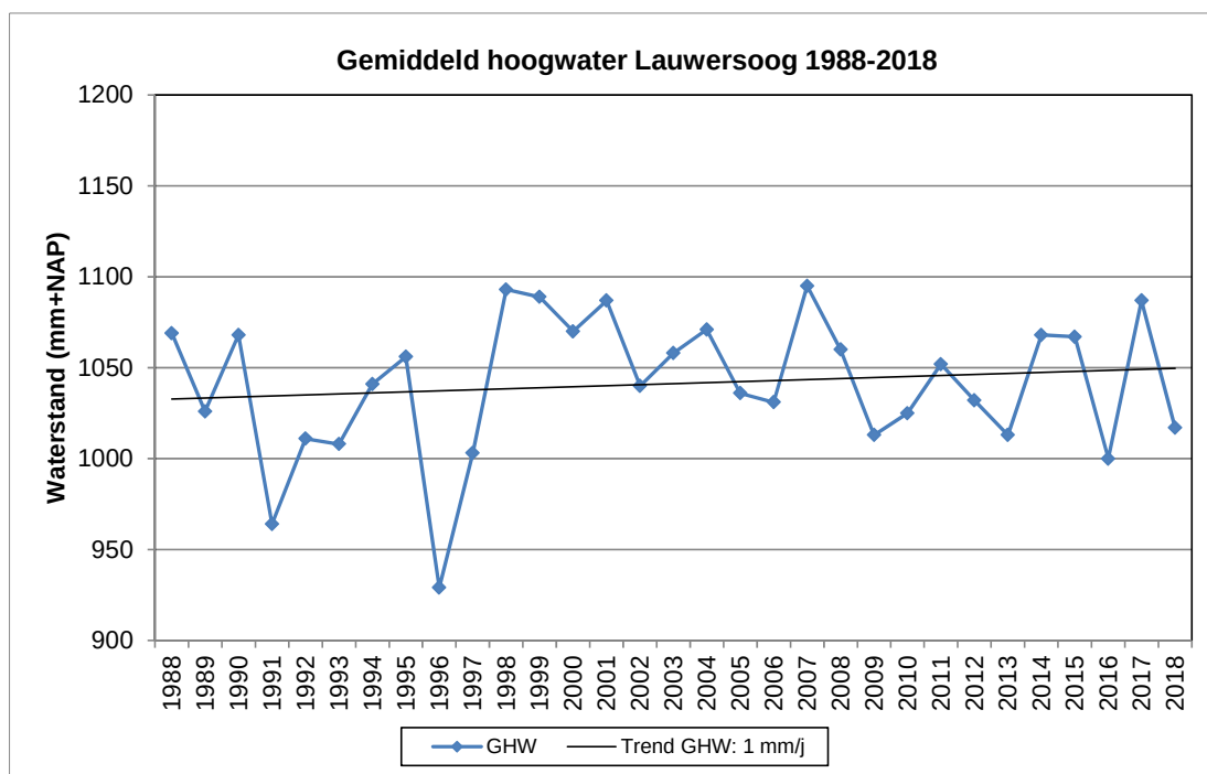
Figuur 3.13 Jaargemiddelde hoogwater van 1988-2018 op basis van hoogwater-data van Rijkswaterstaat voor Lauwersoog.
