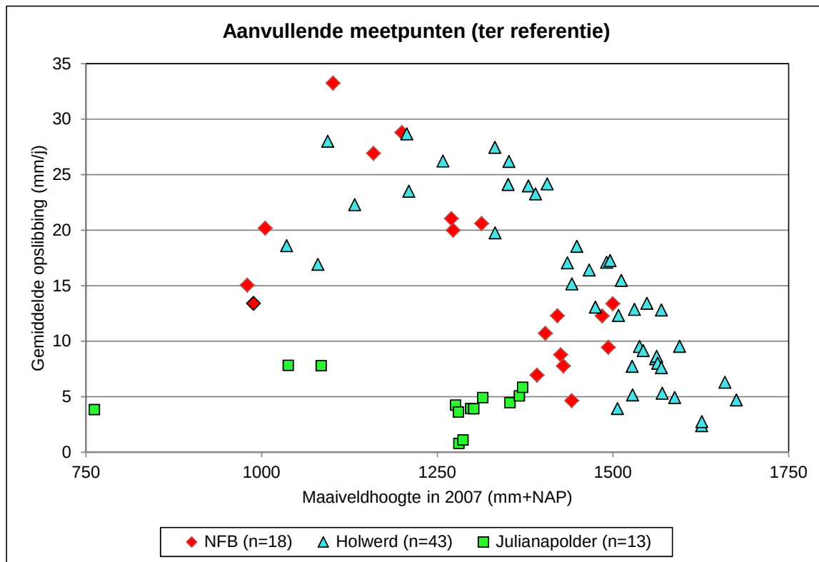
Figuur 3.8 Gemiddelde netto-opslibbing in mm/j per kwelder-pq (inclusief pq's in de pionierzone) over de periode 2007-2018 in de aanvullende meetpunten ter referentie in de deelgebieden Noord-Friesland Buitendijks (NFB), Holwerd (Fr.) en Julianapolder (Gr.).
