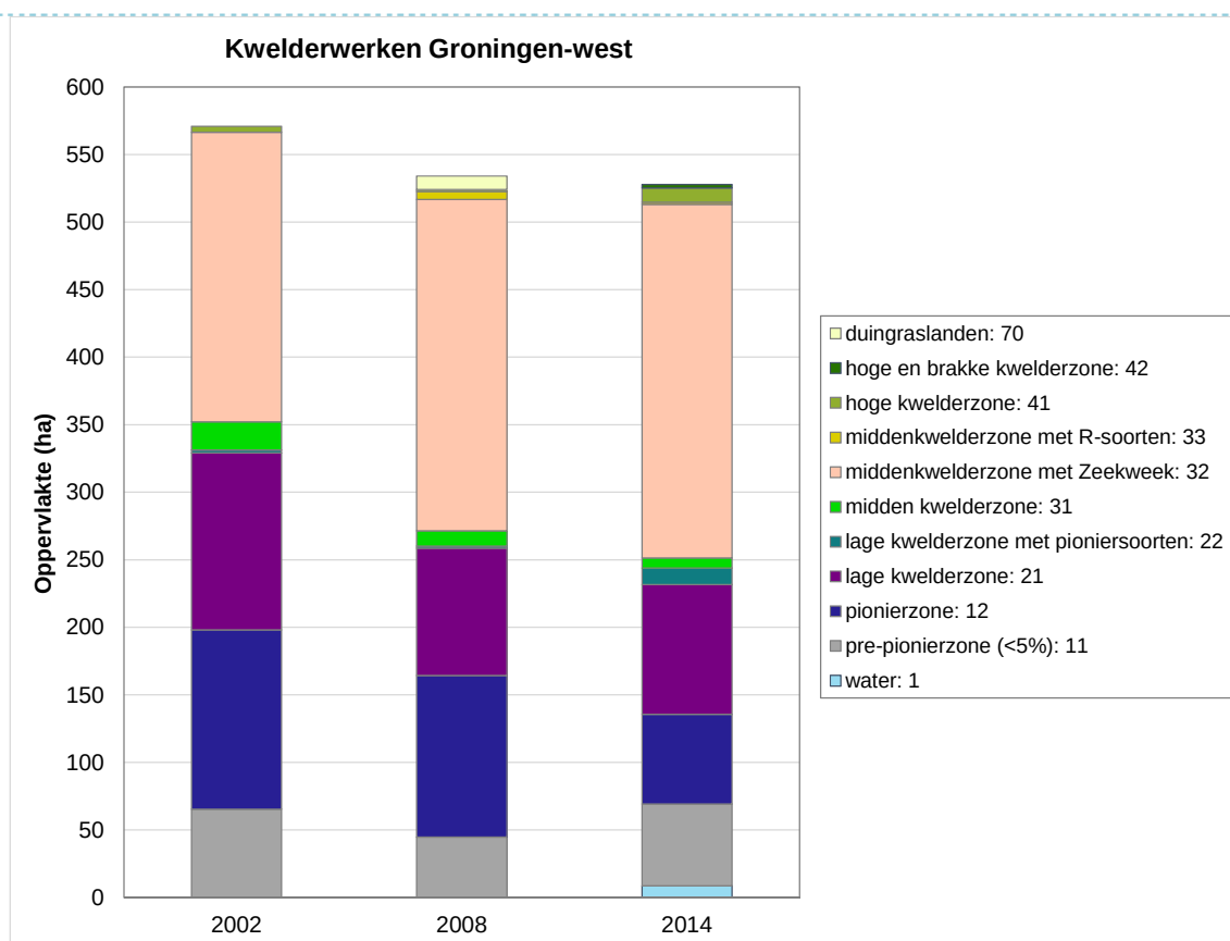
Figuur 3.11 Ontwikkeling vegetatiezones in de de kwelderwerken van Groningen-west van 2002-2014. Gebaseerd op gegevens van Wageningen Marine Research berekend uit de VEGWAD-vegetatiekarteringen door RWS.
