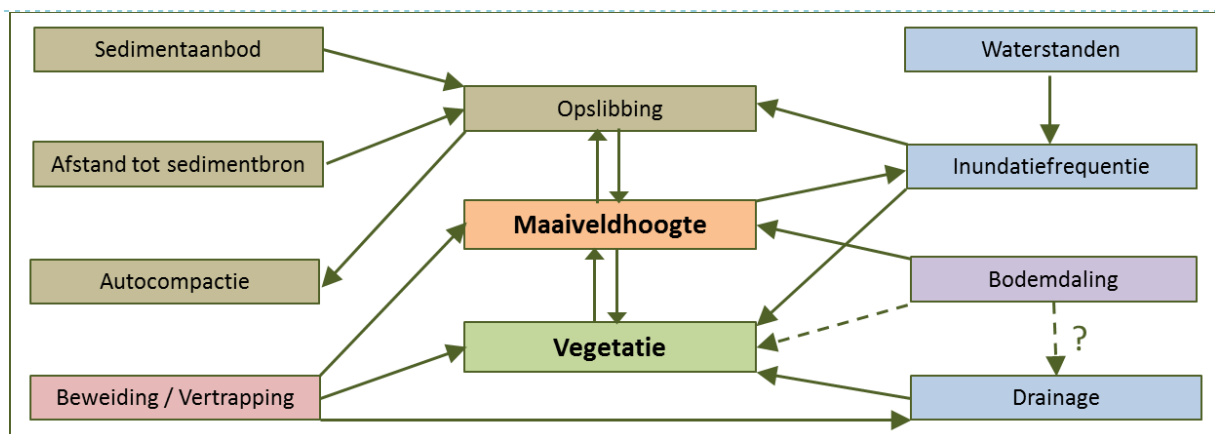
Figuur 1.5 Factoren die een rol spelen bij de maaiveldhoogte- en vegetatie-ontwikkeling op vastelandskwelders.
