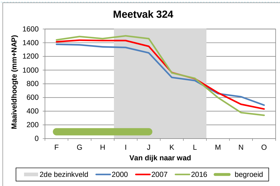
Figuur 3.12 Maaiveldhoogte referentie-meetvak 324 in 2000, 2007 en 2016. Gebaseerd op gegevens van RWS.
