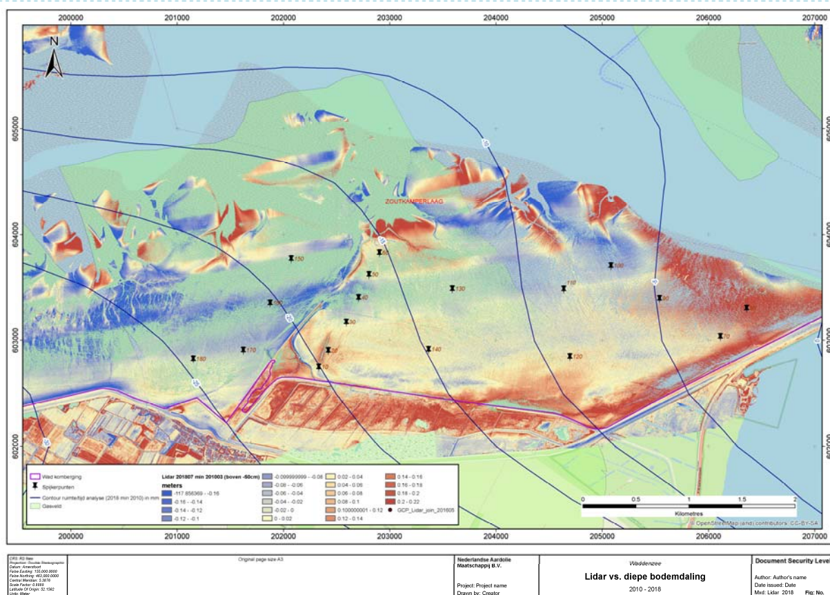
Figuur 1.4 Kleurenkaart met het verschil van de Lidaropnamen van zomer 2018 min voorjaar 2010 (in meters) en de contouren van de gemeten bodemdaling (blauwe lijnen), verwerkt in een ruimte/tijd analyse (in mm), tussen 2010 en 2018. De gasvelden zijn in groen aangegeven. Data en kaart: H. Piening (NAM).
