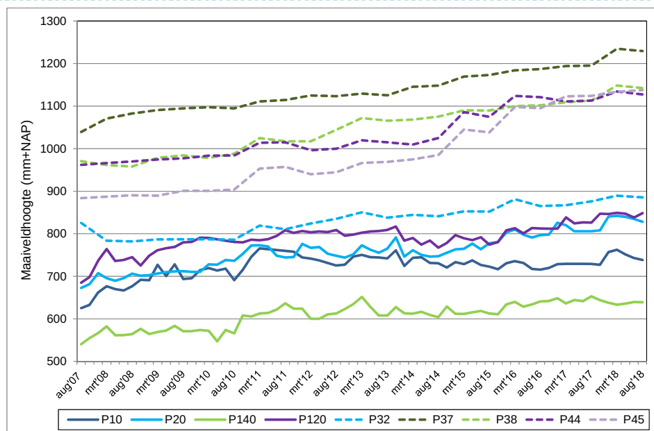
Figuur 3.5a. Vergelijking van de opslibbingsmetingen van NCA en Artemisia op de overgang van wad naar kwelder bij de Peazemerlannen over periode aug 2007- aug 2018. De P met nummer betreft het meetpunt en het getal achter de stip de opslibbing in mm/j (Kaart gemaakt door Johan Krol; zie ook Krol, 2019); b. De ontwikkeling van de maaiveldhoogte (mm+NAP) bij de meetpunten van aug 2007-aug 2018. De doorgetrokken lijnen betreffen de NCA-meetpunten en de gestippelde lijnen de Artemisia-meetpunten. De meetpunten die bij elkaar in de buurt liggen hebben vergelijkbare kleuren.
