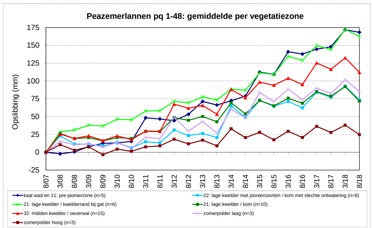
Figuur 3.1 Gemiddelde cumulatieve netto-opslibbing (mm) per vegetatiezone (met SALT97 code) in de kwelder en deelgebied in de zomerpolder op basis van SEB-metingen in de Peazemerlannen van augustus 2007-augustus 2018.
