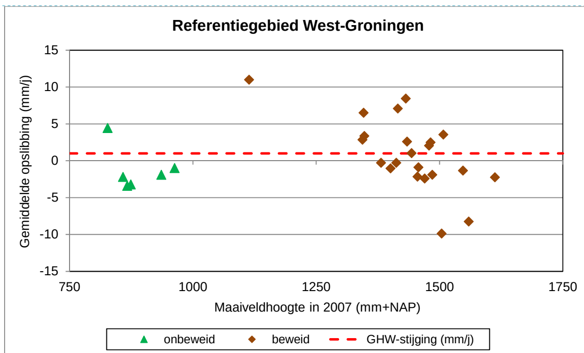
Figuur 3.7 Gemiddelde netto-opslibbing in mm/j per kwelder-pq (inclusief pq's in de pionierzone) over de periode 2007-2018 in het referentiegebied West-Groningen. De rode stippellijn geeft de gemiddelde trend in GHW-stijging van 1 mm berekend voor Lauwersoog over de periode 1988 t/m 2018 (zie Figuur 3.13). In 2018 waren alleen de onbegroeide pq's op het wad nog onbeweid, want ook de laatste vijf vanaf 2007 permanent onbeweide kwelder-pq's in meetvak 286 waren in 2018 beweid.
