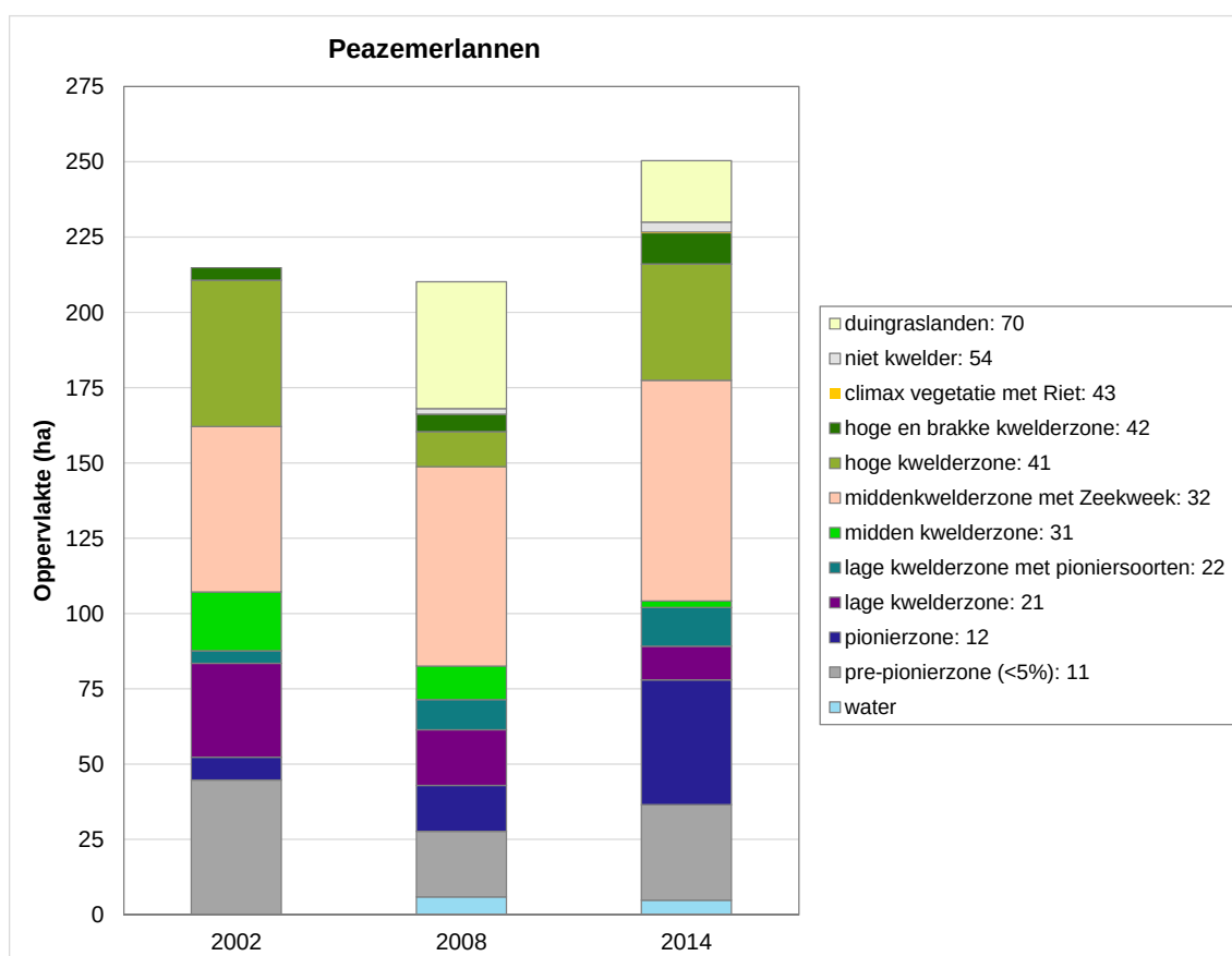
Figuur 3.9 Ontwikkeling vegetatiezones in de Peazemerlanden van 2002-2014. Gebaseerd op gegevens van Wageningen Marine Research berekend uit de VEGWAD-vegetatiekarteringen door RWS.
