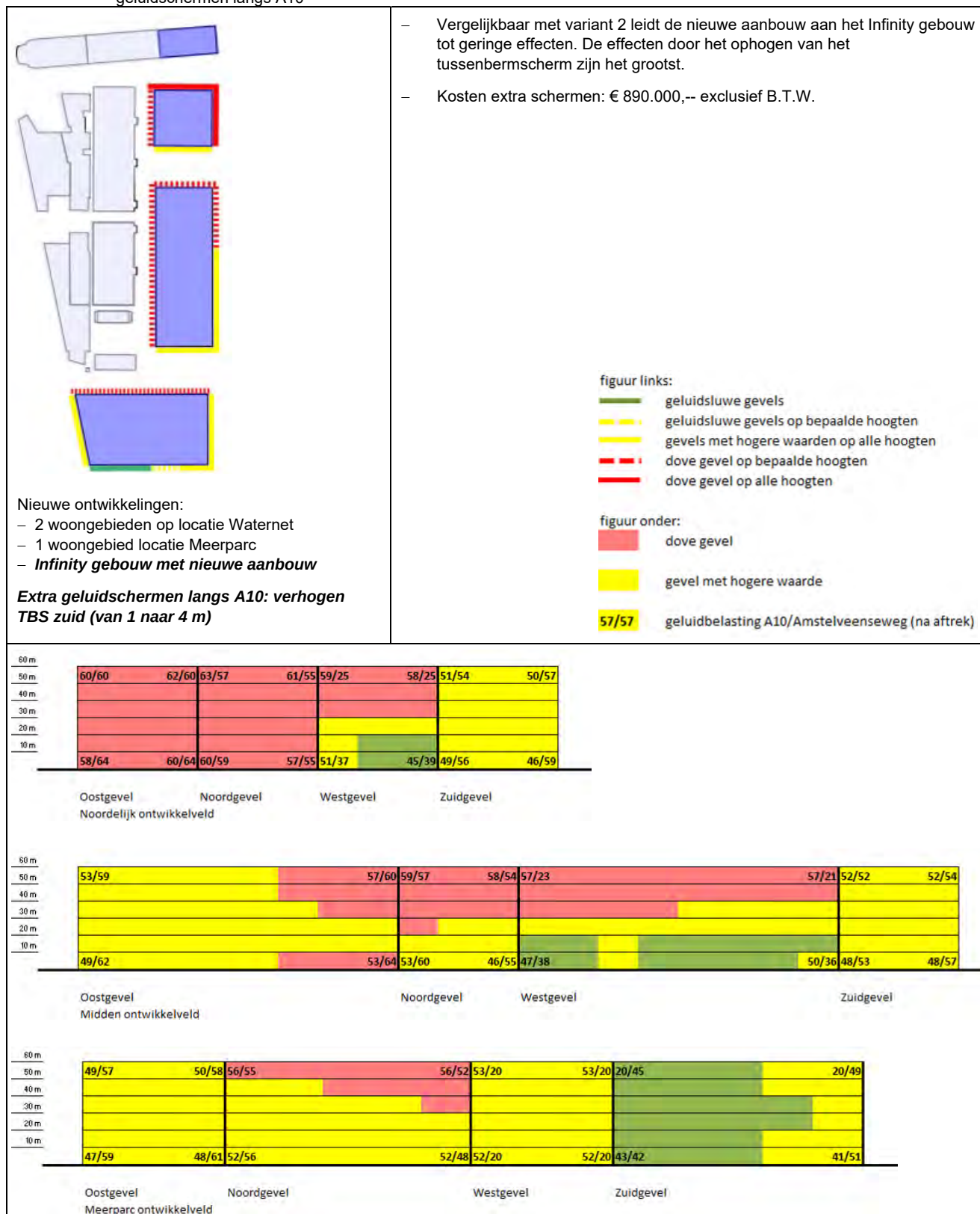
Figuur 6.22: Variant 5, subvariant 1 - Nieuwe ontwikkelingen locatie Waternet/Meerparc, Infinity gebouw met nieuwe aanbouw, extra geluidschermen langs A10
