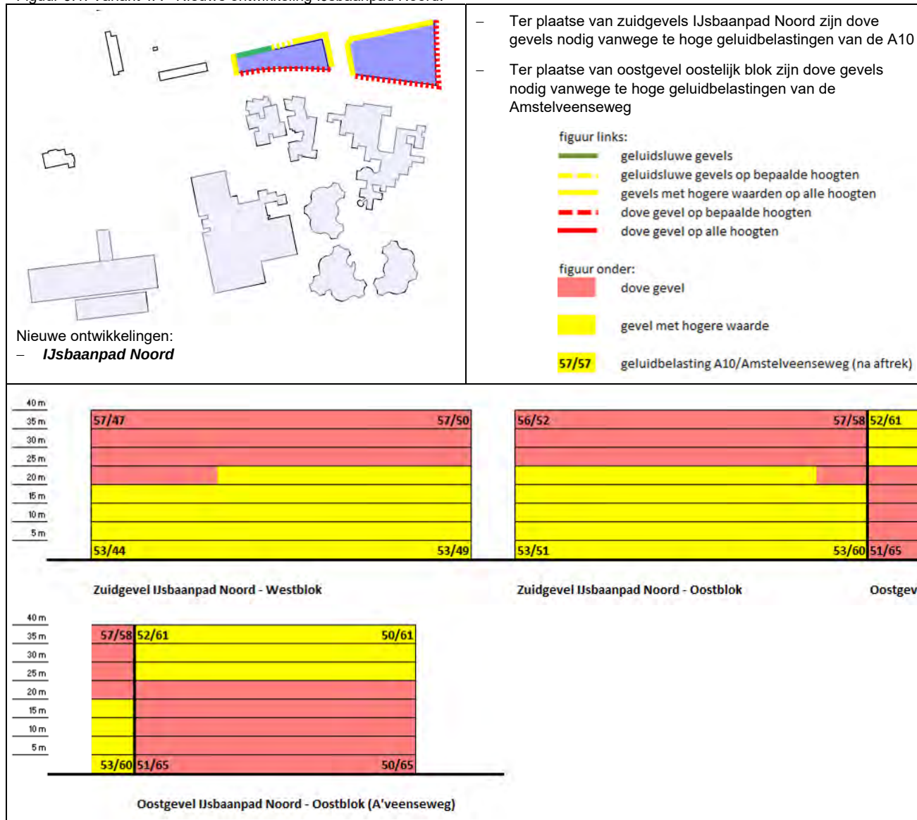
Figuur 6.1: Variant 1A - Nieuwe ontwikkeling IJsbaanpad Noord.
