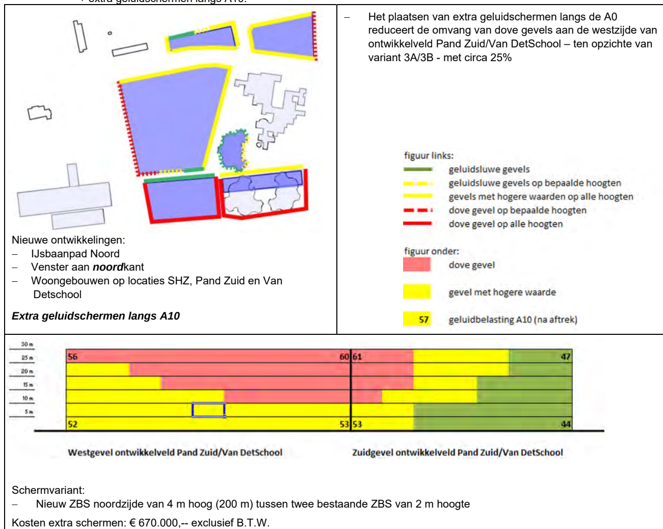
Figuur 6.15: Variant 3G, subvariant 1 - Nieuw: IJsbaanpad Noord, en Venster noordkant, nieuwbouw SHZ, Pand Zuid/Van DetSchool + extra geluidschermen langs A10.
