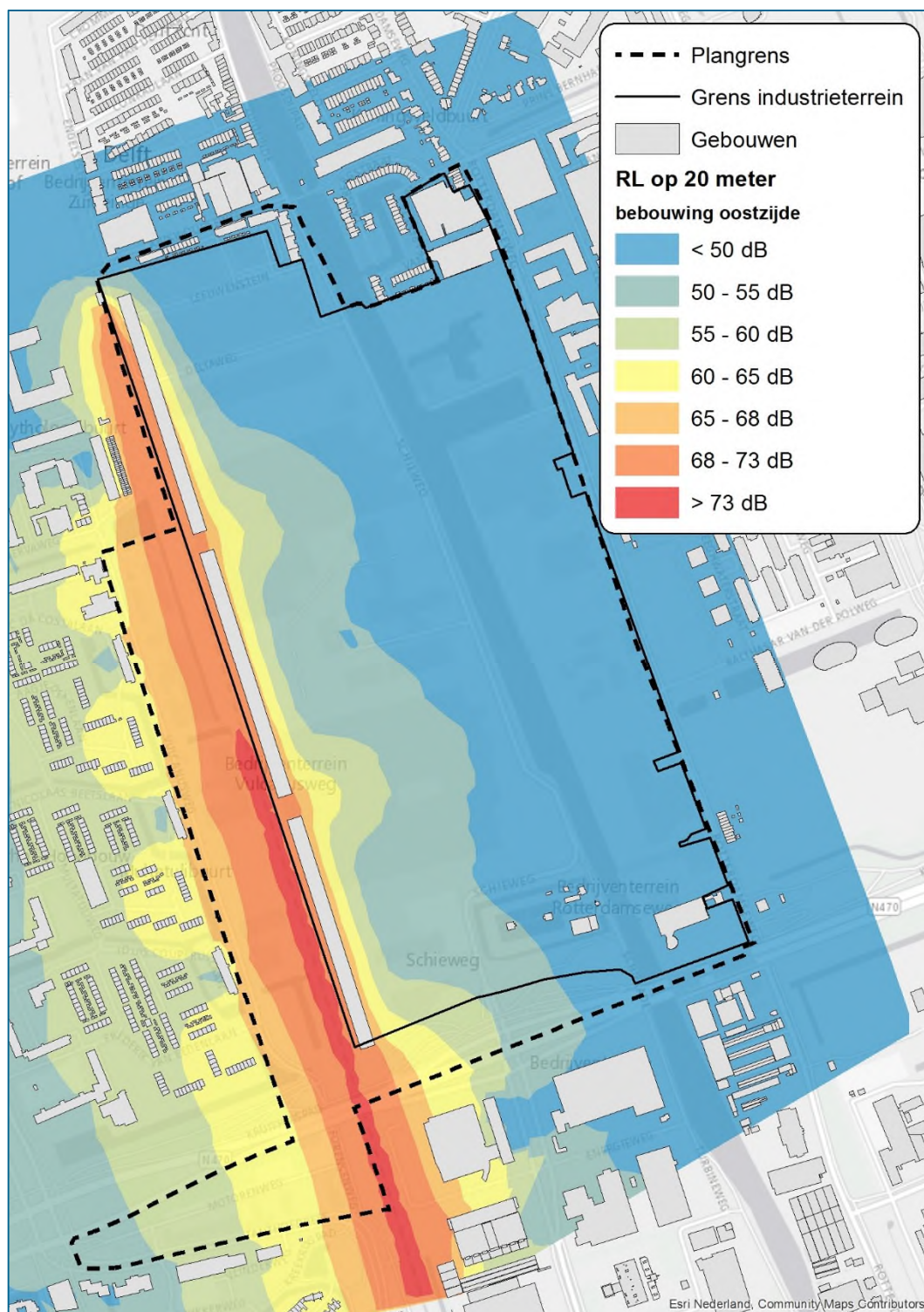
Afbeelding 3.4 Geluidbelasting tgv railverkeerslawaaï in dB op 20 meter hoogte (bebouwing oostzijde)
