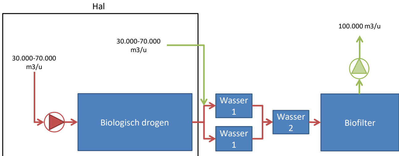
Figuur 1 – schets luchthuishouding hygiënisatie (biologisch drogen)
