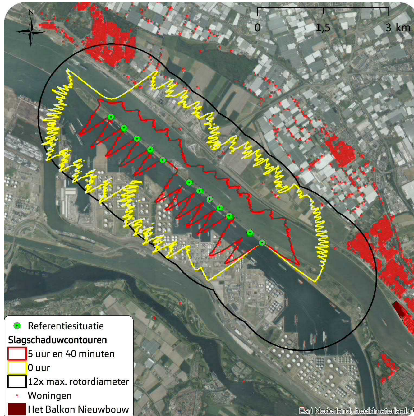
Slagschaduwcontouren Referentiesituatie
