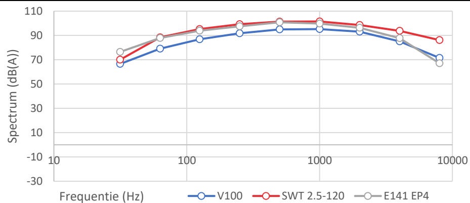
Figuur 7 Spectraalverdeling van de windturbines uit het MER.
