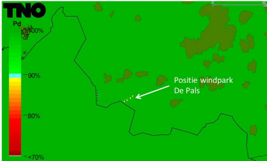
Figuur 6 Detectiekans van het primaire verkeersleidingsradarnetwerk op 1000 voet boven het bouwplan nadat deze is gerealiseerd. De locatie van de verwijderde windturbines is aangegeven met rode kruizen en de nieuwe windturbines met gele stippen.
