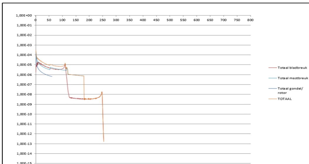
Figuur 2.2: Resultaat risicoberekening Vestas V126
