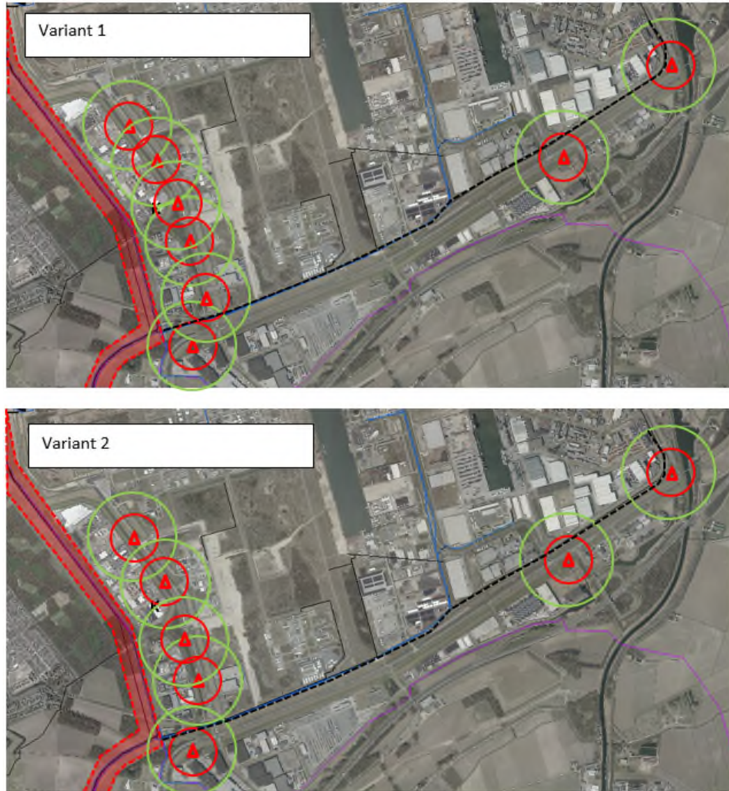
Figuur 5.1: Buisleidingen nabij windpark
