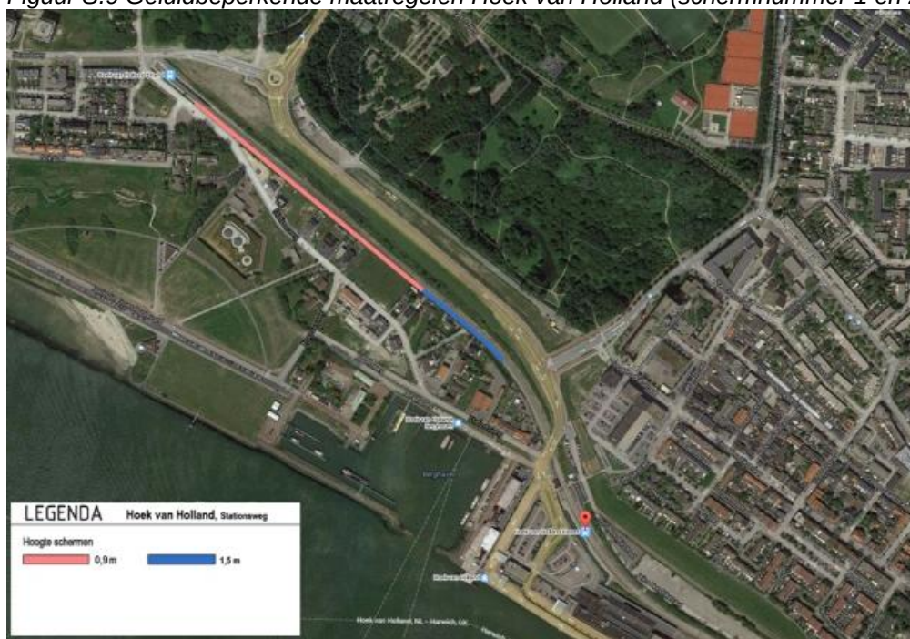
Figuur S.9 Geluidbeperkende maatregelen Hoek van Holland (schermnummer 1 en 2)
