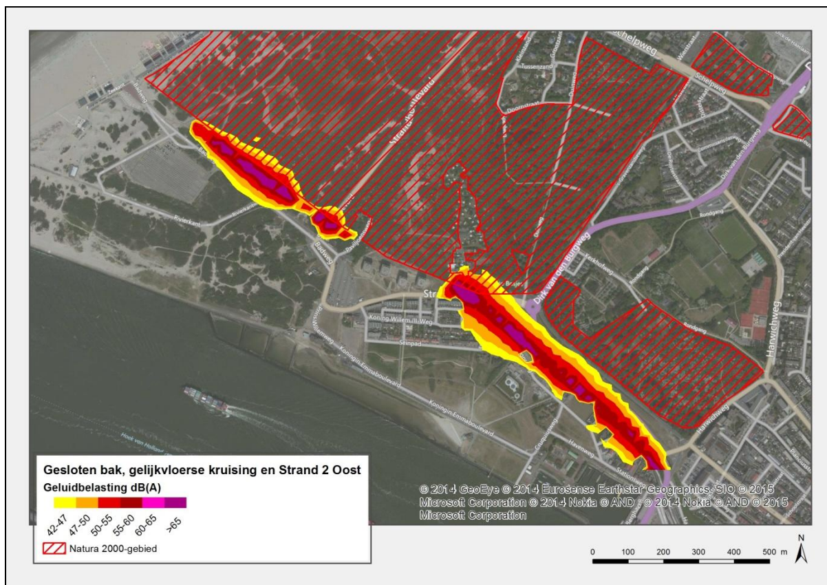
Figuur 6.6 Geluidbelasting als gevolg van alternatief Ombouw + Verlenging.
