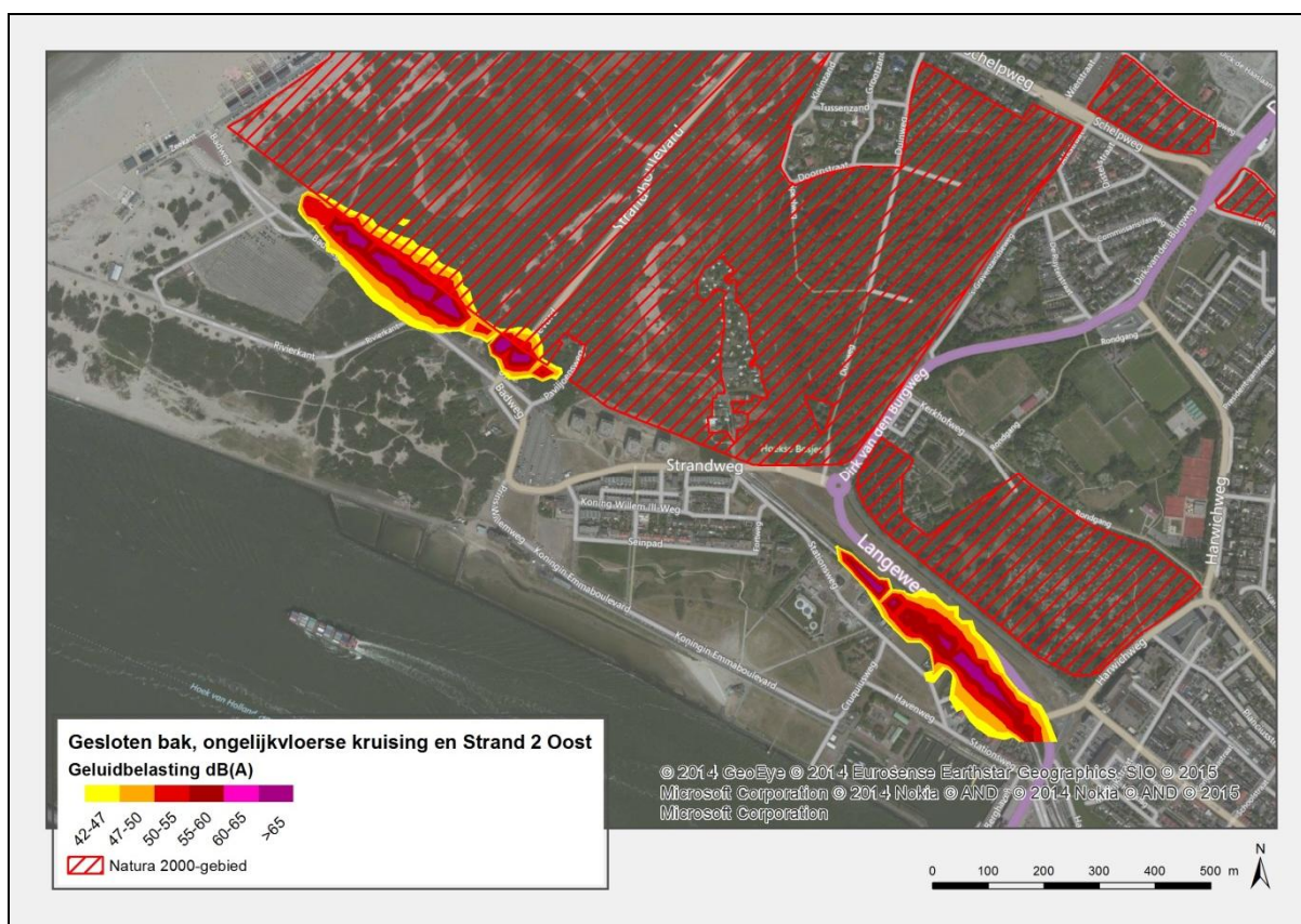
Figuur 6.9 Geluidbelasting in de variant Verdiepte kruising Strandweg
