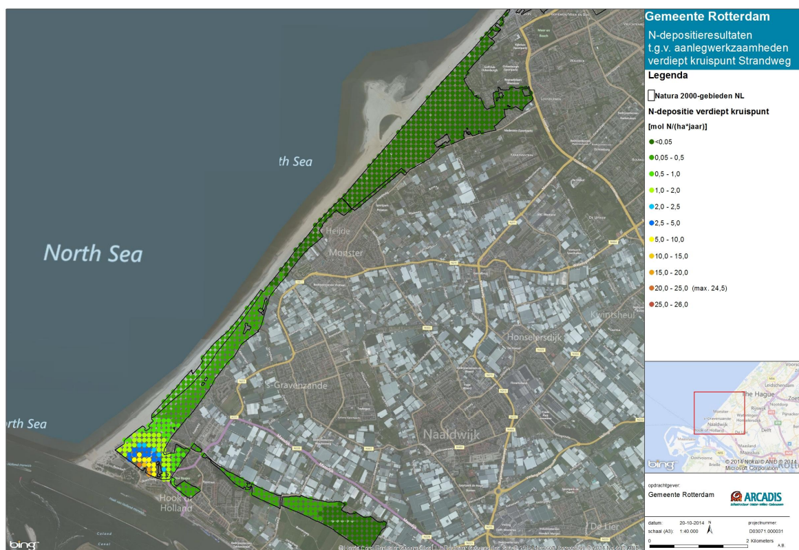
Figuur 6.2 Stikstofdepositie t.g.v. verdiepte aanleg van de kruising van metro met wegverkeer
