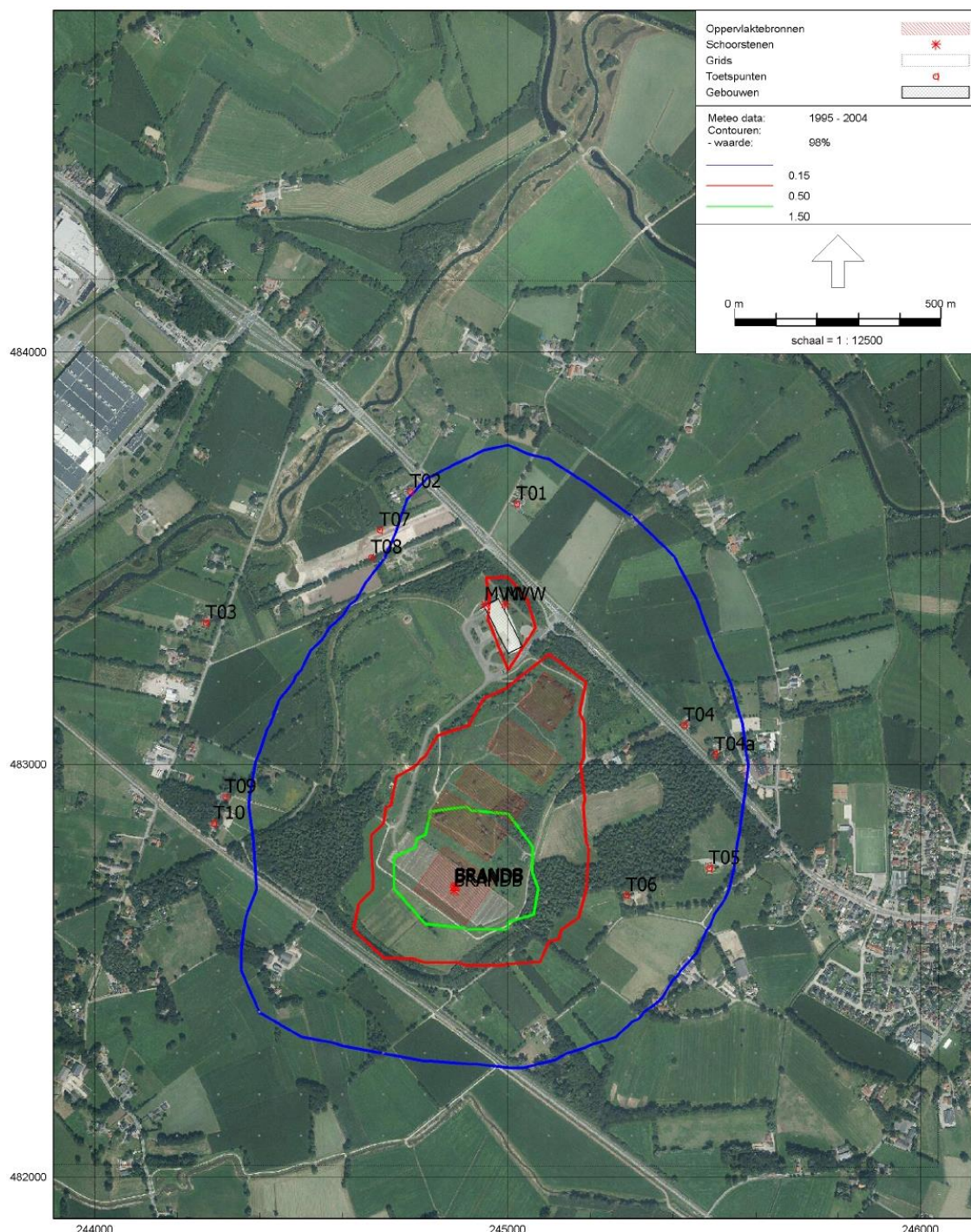
Figuur e Toekomstige situatie: depot brandbaar afval (optie 1) in compartiment 4b+5a inclusief mestverwerkingsinstallatie
