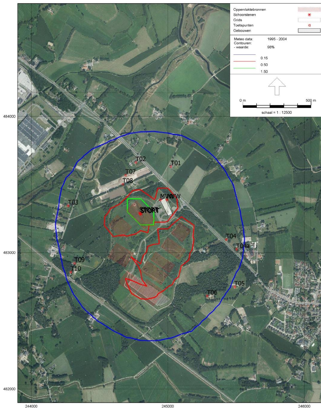
Figuur g Toekomstige situatie: storten in compartiment 8 inclusief mestverwerkingsinstallatie
