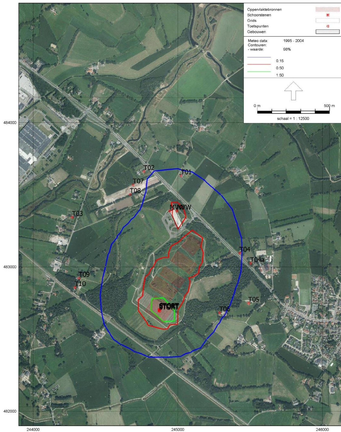
Figuur c Toekomstige situatie: storten in compartiment 4b+5a inclusief mestverwerkingsinstallatie
