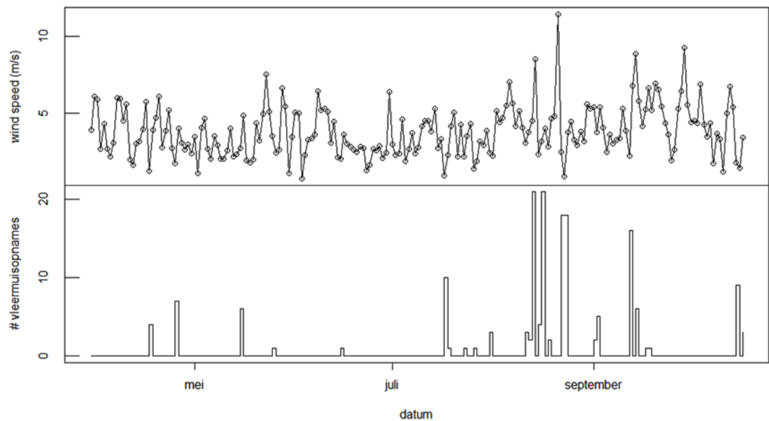
Figuur 7.4 Gemiddelde windsnelheid per nacht voor Irene Vorrink (boven) en aantal vleermuisopnames op gondelhoogte (onder, n = 167 ). De naam van de maand staat aan het begin van de betreffende maand op x-as.
