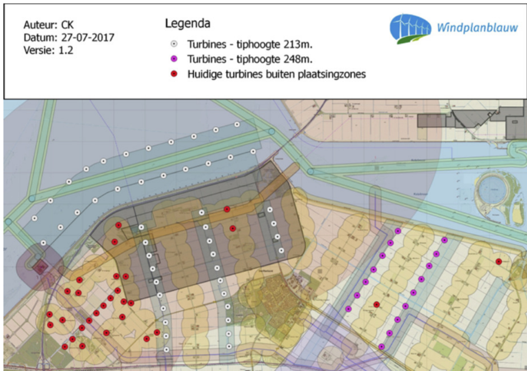
Figuur 2.3 Turbinelocaties van Variant 1A van Windplan Blauw. De rode turbines zijn de zogenaamde dubbeldraaiturbines (§ 2.2.2). De coördinaten van de turbineposities zijn opgenomen in de technische uitgangspuntennotitie in het hoofddocument van het MER.
