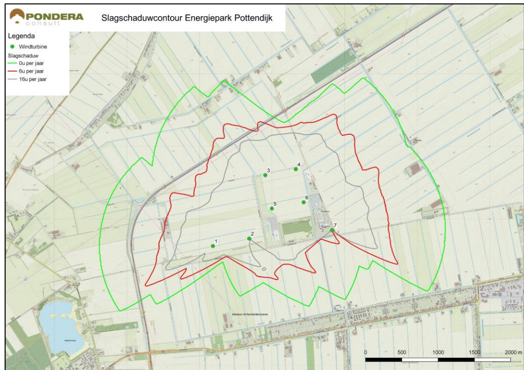
Figuur 16.4 Slagschaduwcontouren Energiepark Pottendijk B.V.
