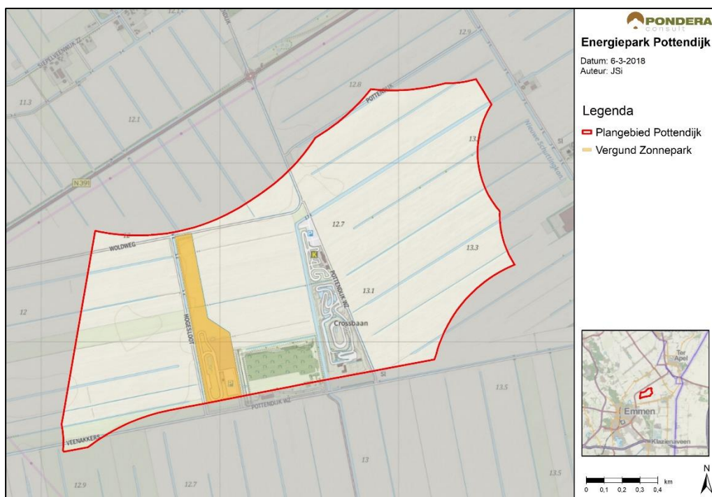
Figuur 4.13 Ligging zonneakker Veenakkers binnen windlocatie Pottendijk
