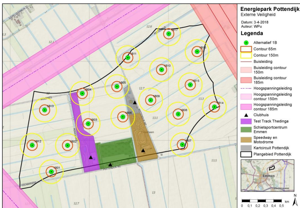
Figuur 12.2 Maximale ligging plaatsgebonden risicocontouren van alternatief 1B
