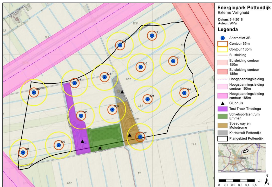
Figuur 12.5 Maximale ligging plaatsgebonden risicocontouren van alternatief 3B
