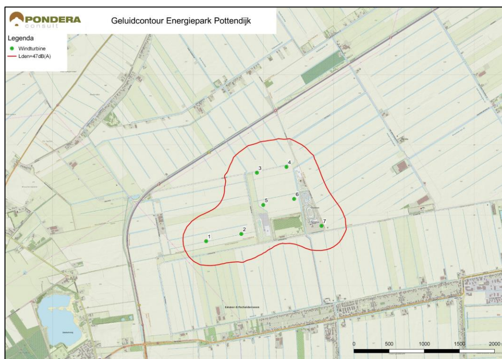
Figuur 16.3 Geluidcontour L_{den} 47 Energiepark Pottendijk
