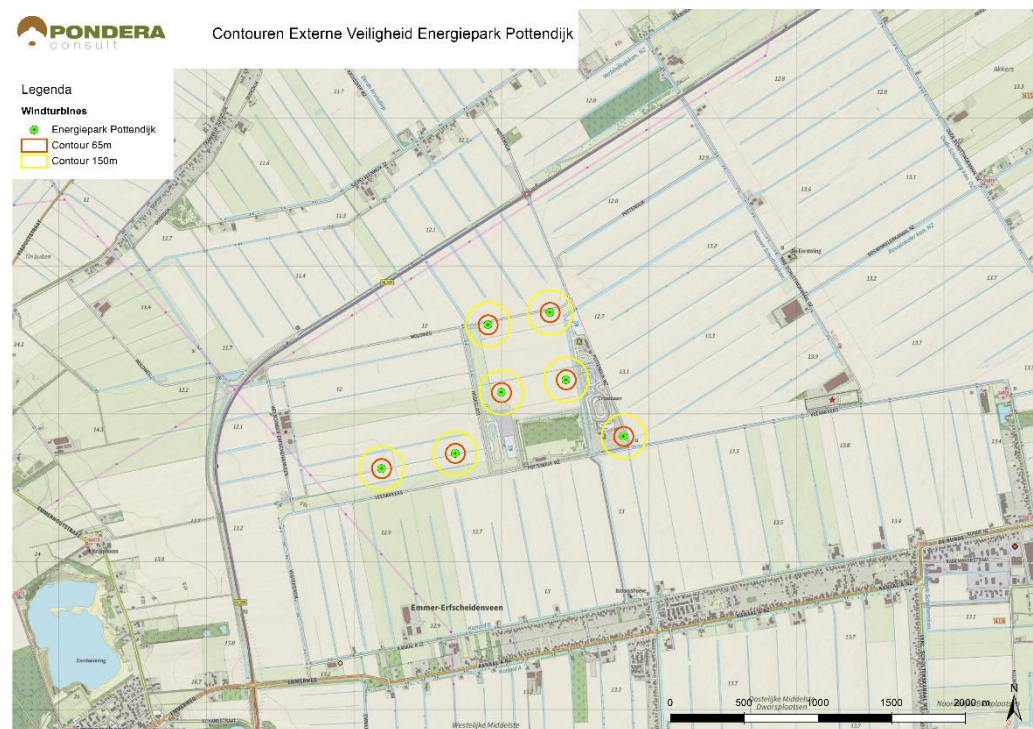
Figuur S10 Veiligheidscontouren Energiepark Pottendijk
