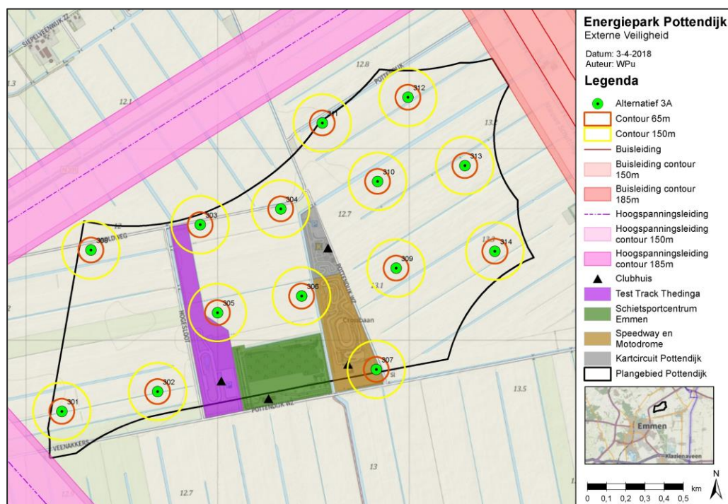
Figuur 12.4 Maximale ligging plaatsgebonden risicocontouren van alternatief 3A
