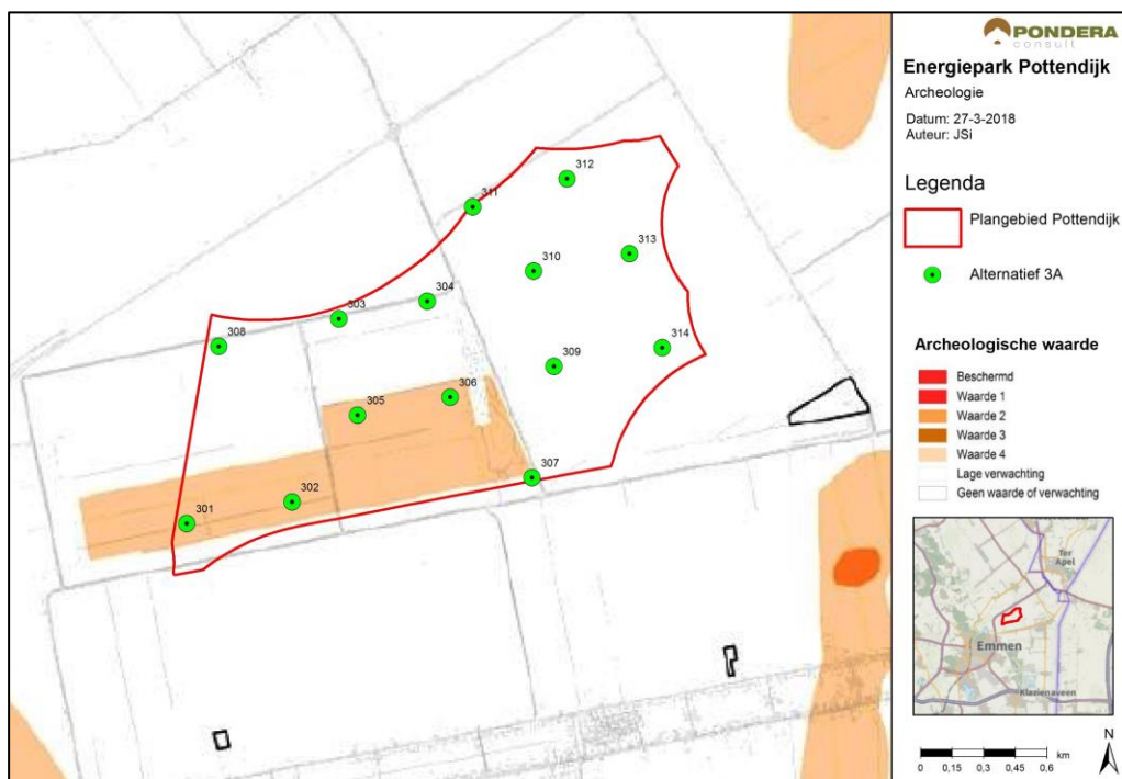
Figuur 10.5 Alternatief 3A, de posities voor alternatief 3B zijn identiek en niet apart weergegeven
