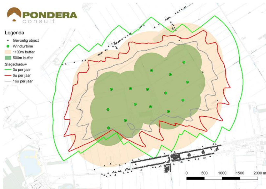
Figuur 7.10 Slagschaduwcontouren Alternatief 4B
