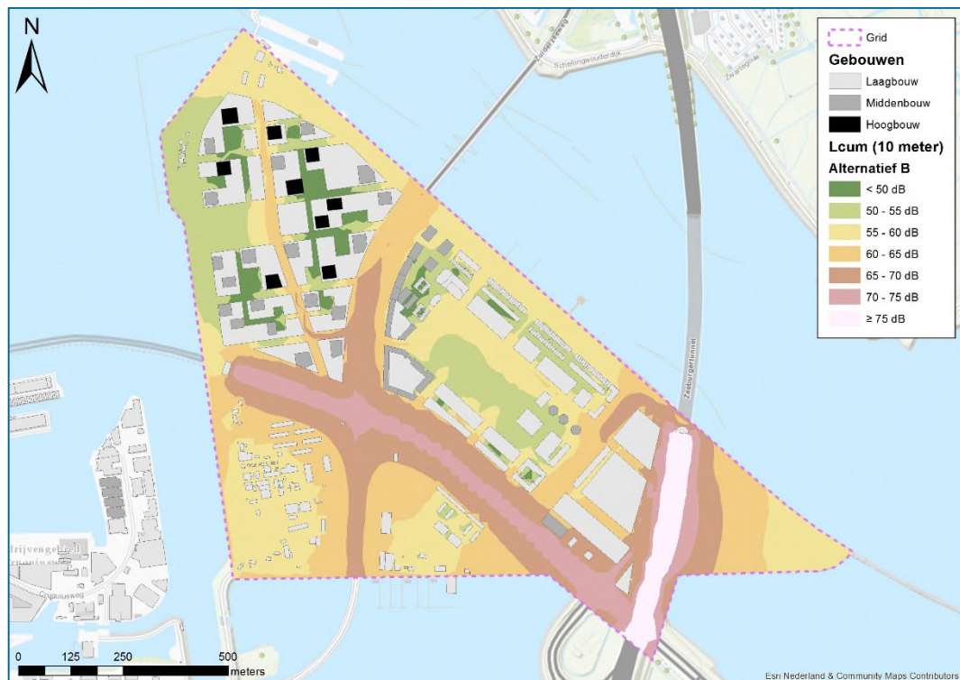
figuur 6.8: Gecumuleerde geluidbelasting (Lcum) alternatief B
