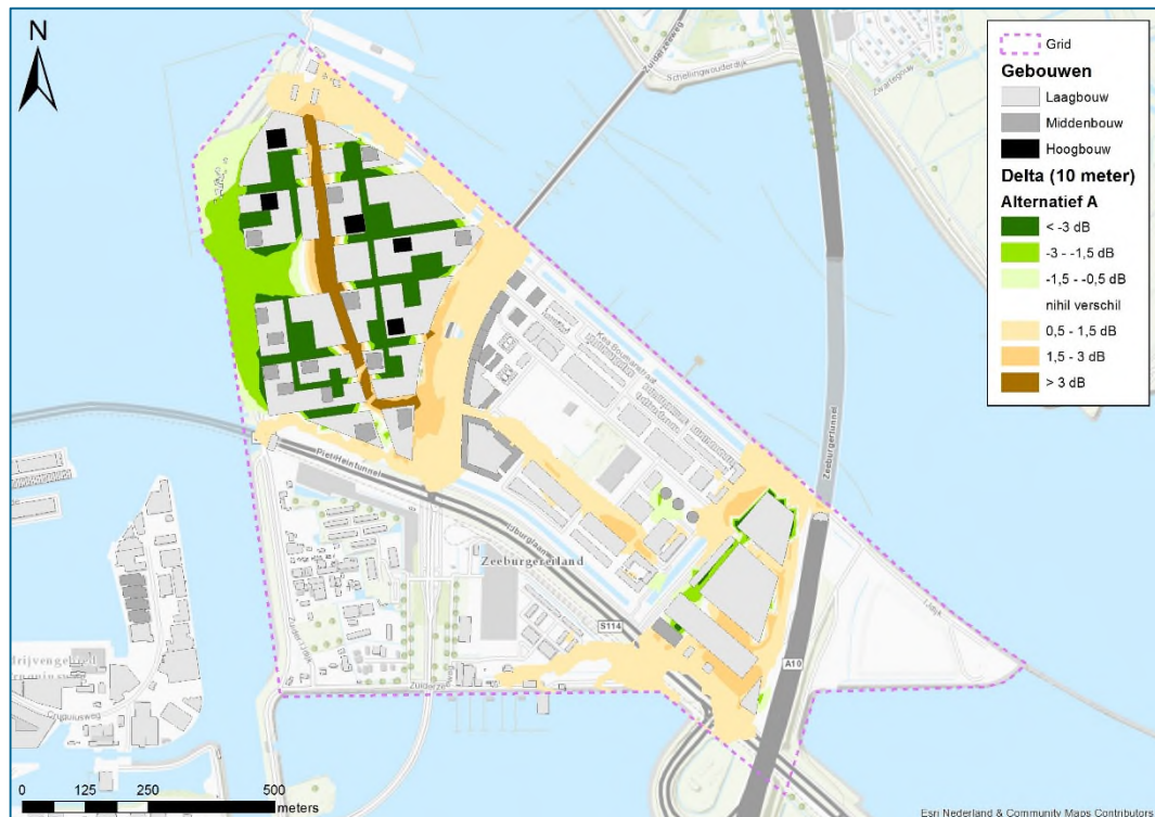
figuur 6.5: Verschilcontour alternatief A ten opzichte van referentiesituatie op 10 m hoogte
