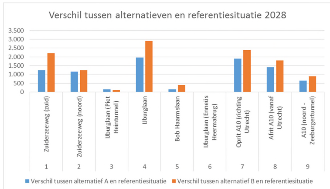
figuur 5.8 Verschil alternatieven in etmaalintensiteiten met de referentiesituatie
