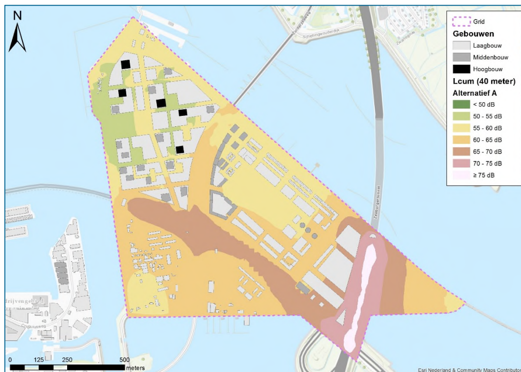
figuur 6.6: Gecumuleerde geluidbelasting ( L_{cum} ) alternatief A op 40 m boven maaiveld.
