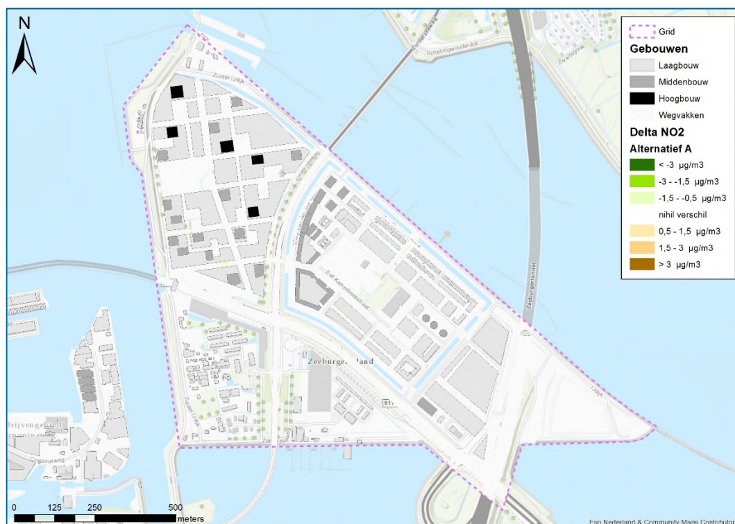
figuur 7.3 Vershilcontour \text{NO}_2 alternatief A ten opzichte van referentie
