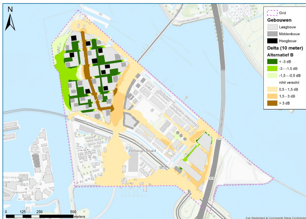
figuur 6.9: Verschilcontour alternatief B ten opzichte van de referentiesituatie op 10 m boven maaiveld.
