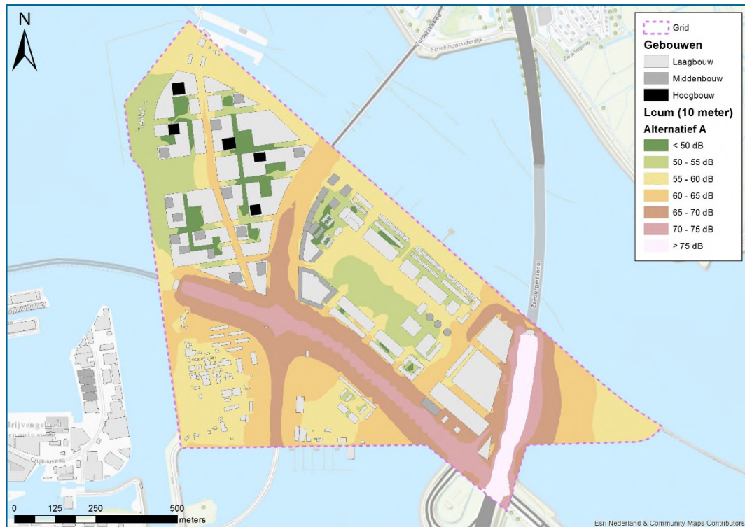
figuur 6.4: Gecumuleerde geluidbelasting (L cum ) alternatief A op 10 m boven maaiveld
