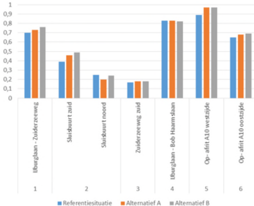
figuur 5.10 Gemiddelde kruispuntbelasting referentiesituatie en alternatieven
