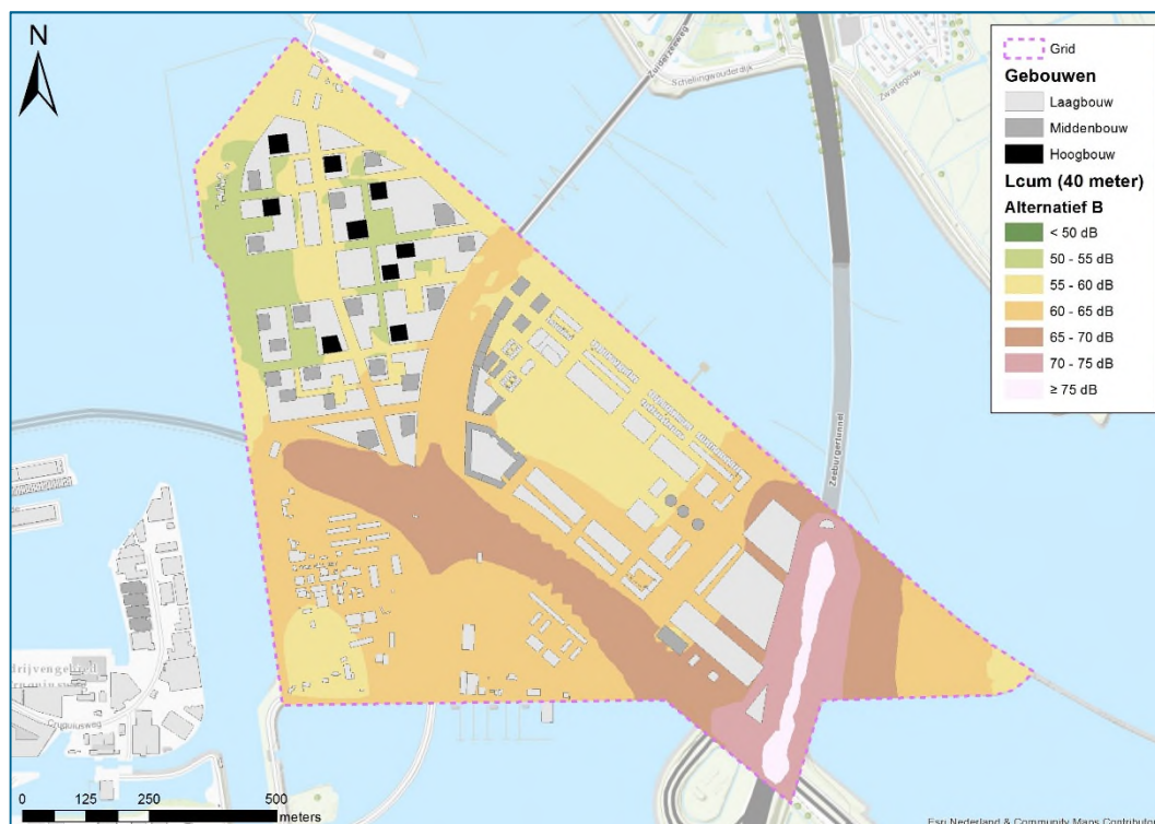
figuur 6.10: Gecumuleerde geluidbelasting ( L_{cum} ) alternatief B op 40 m boven maaiveld
