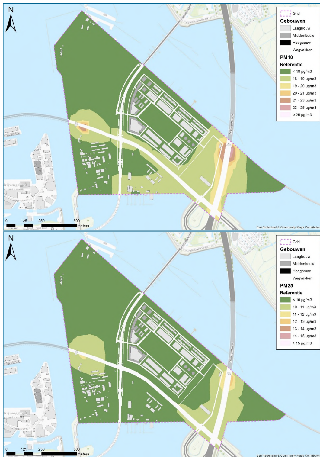
figuur 7.2 Jaargemiddelde concentraties \text{PM}_{10} (boven) en \text{PM}_{2.5} (onder)
