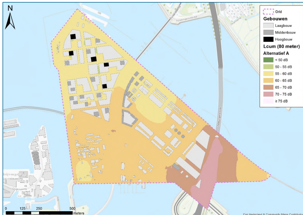
figuur 6.7: Gecumuleerde geluidbelasting ( L_{cum} ) alternatief A op 80 m boven maaiveld.
