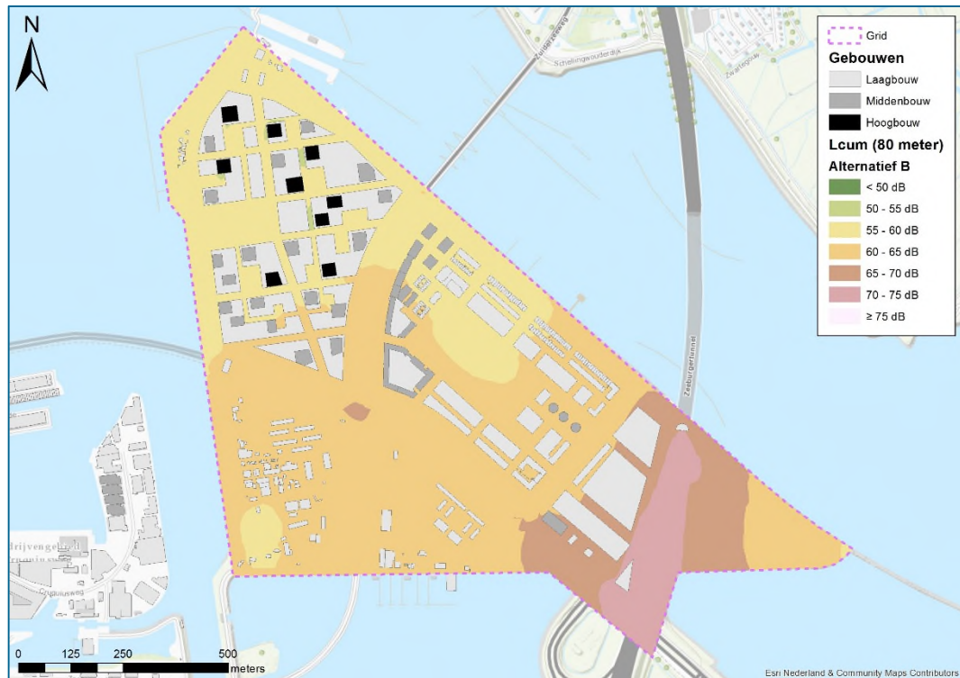
figuur 6.11: Gecumuleerde geluidbelasting ( L_{cum} ) alternatief B op 80 m boven maaiveld
