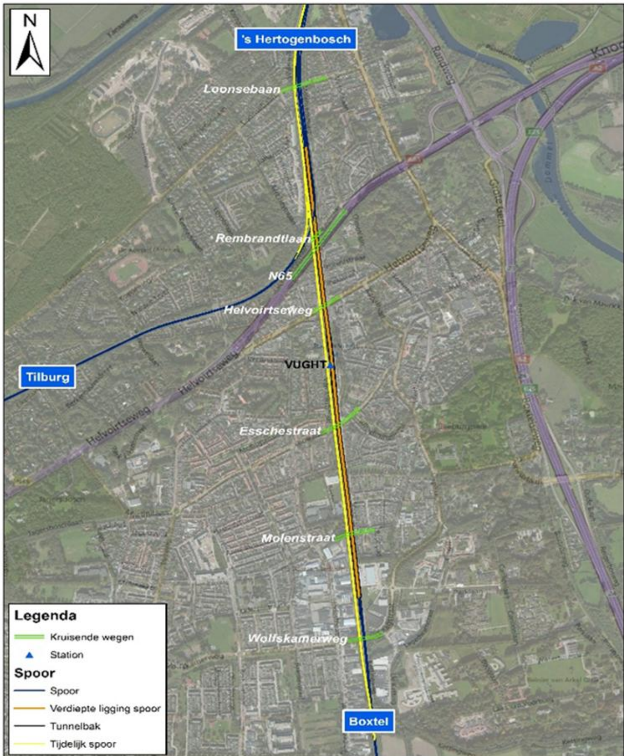
Figuur 3 | Situatieschets van de verdiepte ligging in Vught
