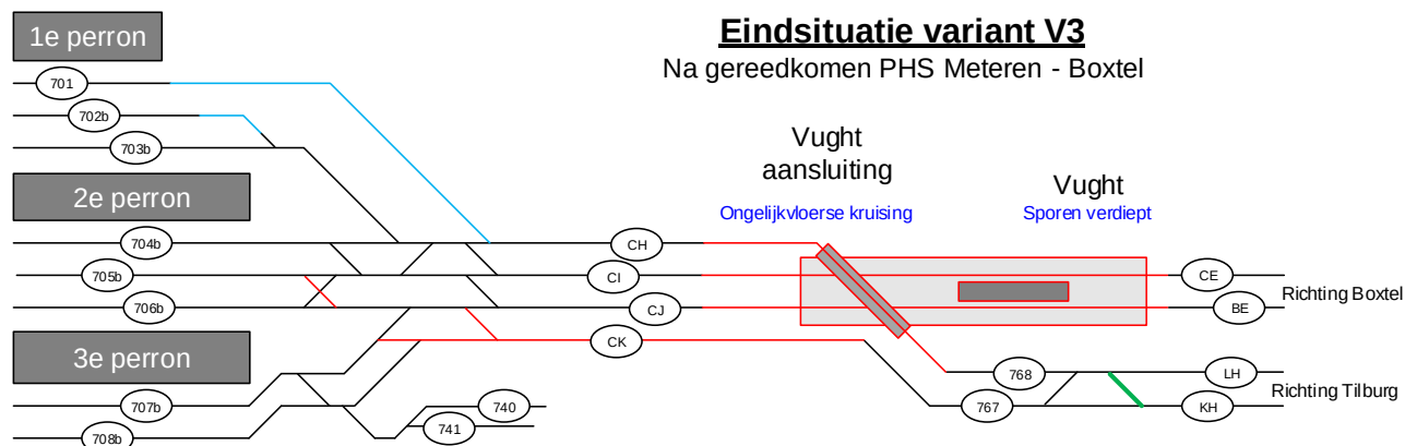
Figuur 2 | Schema huidige sporen (zwart), tijdelijke sporen (paars) en toekomstige sporen (rood) voor het tracé 's-Hertogenbosch – Vught.
